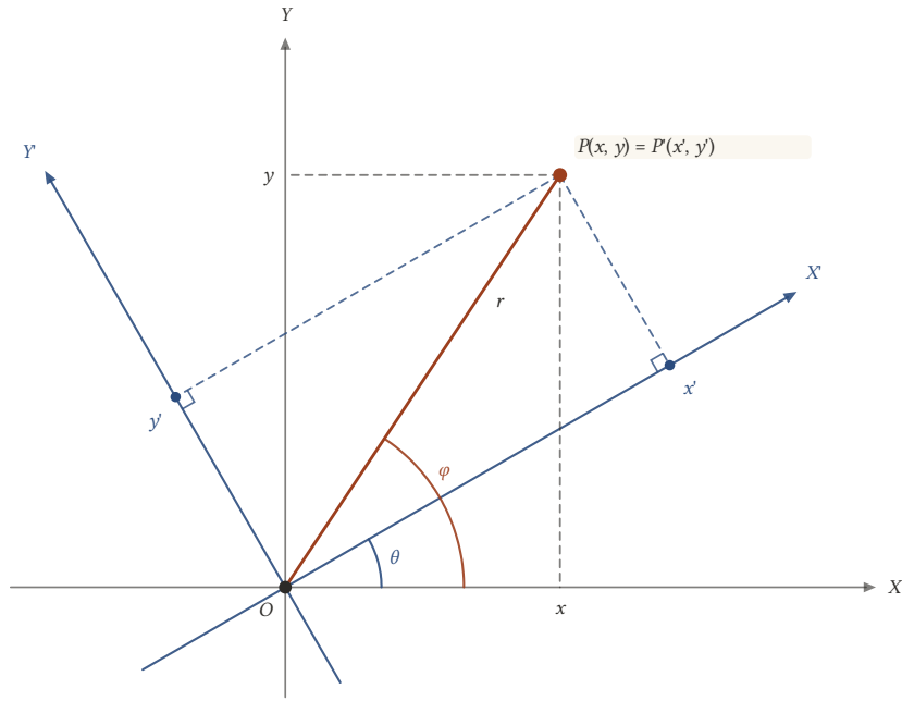
Şekil 17.9: Aynı P noktası: XY sisteminde kutupsal açısı \varphi , X'Y' sisteminde \varphi - \theta ; O'ya uzaklığı iki sistemde de r 'dir.
