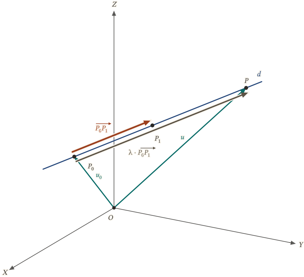
Şekil 10.5: P_0 ile P_1 'den geçen d doğrusunun doğruiltmanı olarak P_0P_1 vektörü alınır; d 'nin her P noktası için u = u_0 + \lambda P_0P_1 olur.
