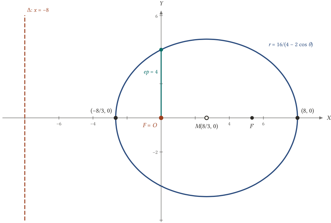
Şekil 20.13: r = 16/(4 - 2 \cos \theta) ; e = 1/2 , kutup sol odakta; Kartezyen denklem 3x^2 - 16x + 4y^2 = 64 .
