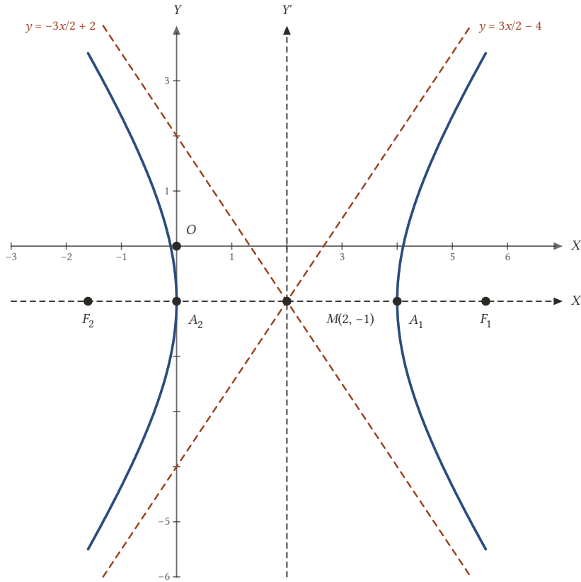
Şekil 19.7: Merkezi M(2, -1) olan hiperbol: öteleme ile x'^2/4 - y'^2/9 = 1 olur.
