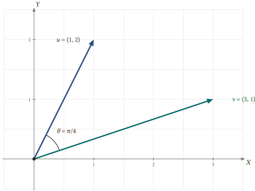
Şekil 9.12: u = (1, 2) ile v = (3, 1) arasındaki açı: \cos \theta = \sqrt{2}/2 , yani \theta = \pi/4 .
