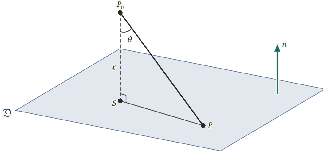
Şekil 14.9: P_0 'dan düzleme inen dikmenin ayağı S , düzlemin başka bir noktası P 'dir. P_0SP üçgeni S 'de dik açıdadır ve \ell = |P_0S| = |P_0P| |\cos \theta| olur.
