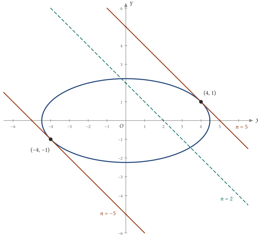
Şekil 18.29: y = -x + n doğruları x^2/20 + y^2/5 = 1 elipsine n = \pm 5 iken (4, 1) ve (-4, -1) noktalarında teğettir; n = 2 doğrusu elipsi keser.
