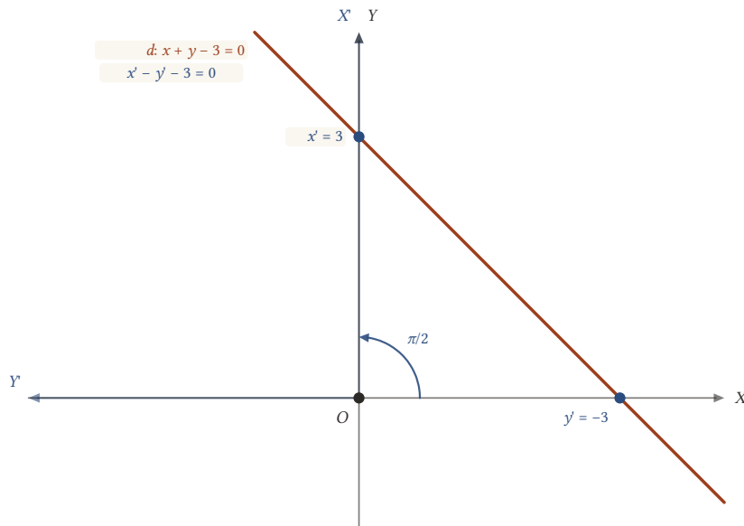
Şekil 17.22: Eksenler \pi/2 döndürülünce x + y - 3 = 0 doğrusu X'Y' sisteminde x' - y' - 3 = 0 olur ve eğimi 1'dir.
