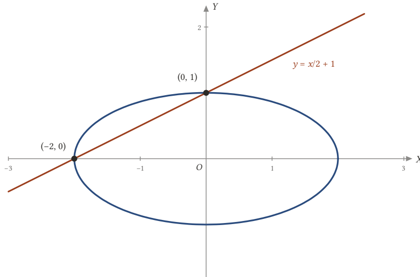
Şekil 18.16: y = x/2 + 1 doğrusu x^2/4 + y^2 = 1 elipsini (0, 1) ve (-2, 0) noktalarında keser.
