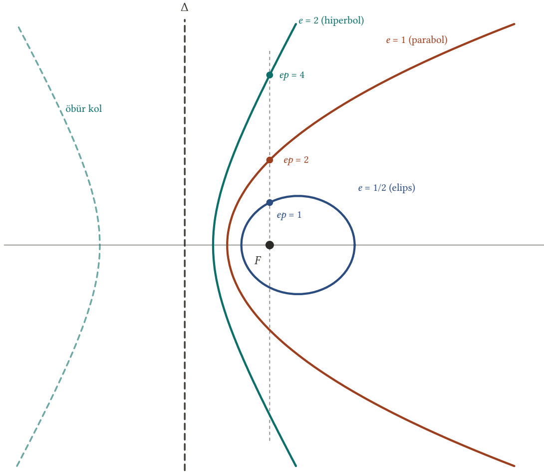
Şekil 20.11: Aynı odak F ve doğrultman \Delta ile üç konik ( p = 2 ): e < 1 elips, e = 1 parabol, e > 1 hiperbol. Kutupsal denklem \Delta 'nın F tarafında kalan kısmı verir; hiperbolün öbür kolu (kesikli) \Delta 'nın öbür yanındadır.
