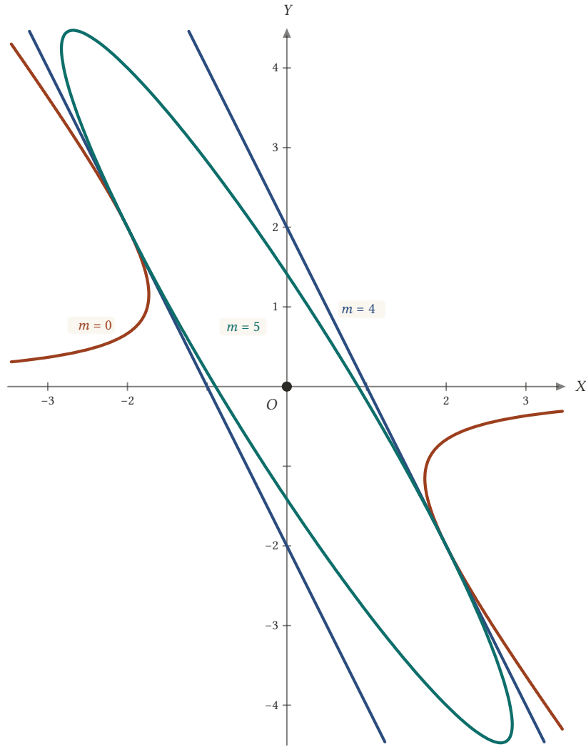
Şekil 21.17: mx^2 + 2(m-2)xy + (m-3)y^2 - 4 = 0 ailesi: m < 4 için hiperbol, m = 4 için paralel iki doğru, m > 4 için elips.
