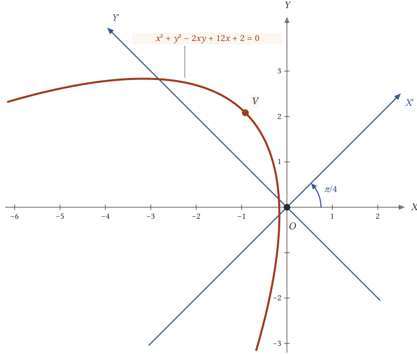
Şekil 21.2: Eksenler \pi/4 döndürülünce karma terim kaybolur: y'^2 + 3\sqrt{2}x' - 3\sqrt{2}y' + 1 = 0 .
