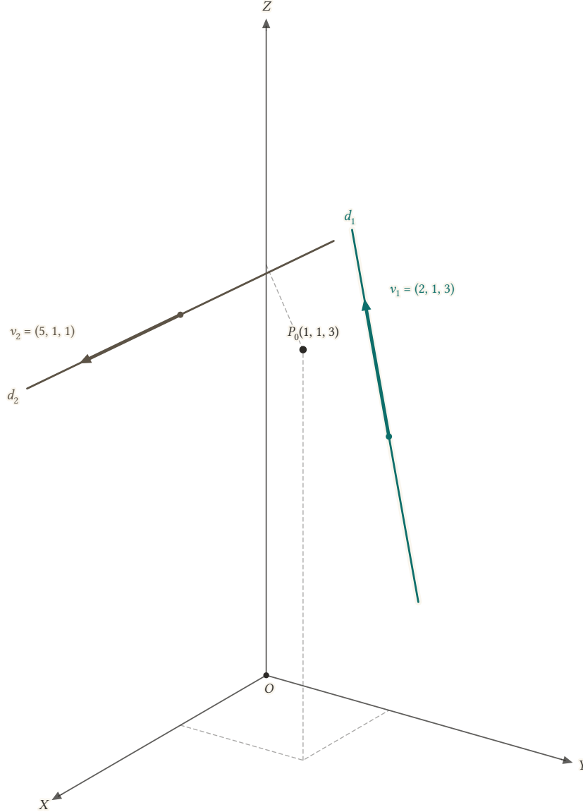
Şekil 12.6: Aykırı d_1 ve d_2 doğruları, doğrultmanları ve P_0(1, 1, 3) noktası. Doğrular kesişmez; şekilde çakışır gibi göründükleri yerde arkadaki doğru kesintilidir.
