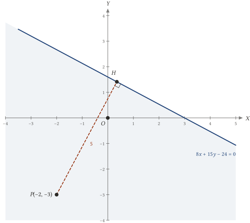
Şekil 3.13: P(-2, -3) noktasının 8x + 15y - 24 = 0 doğrusuna uzaklığı |PH| = 5 'tir. Taralı yarı düzlem doğrunun orijin tarafıdır; s = -5 < 0 olduğundan P de bu taraftadır.
