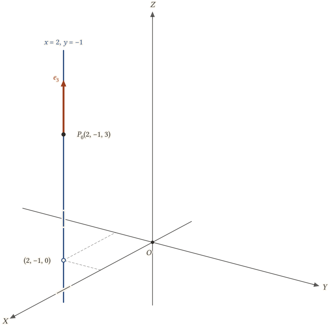
Şekil 12.18: P_0(2, -1, 3) noktasından geçen ve Z -eksenine paralel olan doğru; doğrultmanı e_3 'dir. Doğru XY -düzlemini (2, -1, 0) noktasında dik keser.
