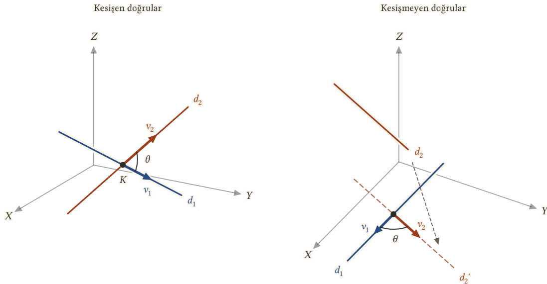
Şekil 11.1: Solda d_1 ile d_2 K noktasında kesişir; aralarındaki açı, K 'dan çizilen doğrultman vektörleri v_1 , v_2 arasındaki \theta açısıdır. Sağda doğrular kesişmez: d_2 kendine paralel kaydırılarak d_1 'i kesen d_2' konumuna getirilir; doğrultman vektörü, dolayısıyla açı değişmez.
