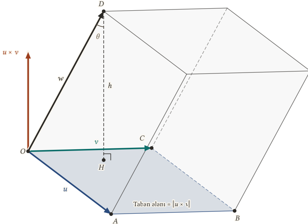
Şekil 9.9: u, v, w üzerine kurulan paralelyüz. Taban OABC 'nin alanı \|u \times v\| , yükseklik h = |HD| = \|w\| \cos \theta 'dir; \theta, w ile tabana dik u \times v arasındaki açıdır. Arkada kalan ayrıtlar kesiklidir.
