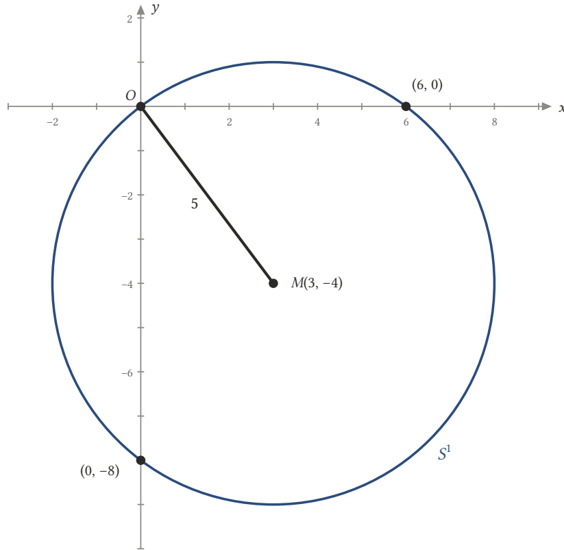
Şekil 4.4: x^2 + y^2 - 6x + 8y = 0 çemberinin merkezi M(3, -4) , yarıçapı 5'tir. F = 0 olduğundan çember orijinden geçer; eksenleri (6, 0) ve (0, -8) noktalarında da keser.
