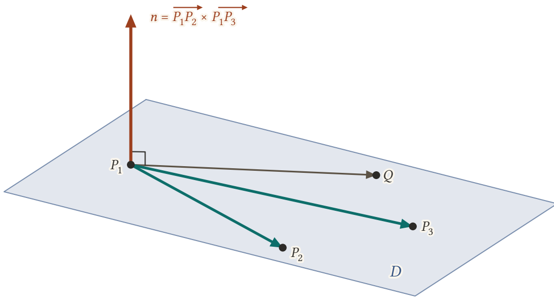
Şekil 12.9: Doğrudaş olmayan P_1, P_2, P_3 noktaları ve düzlemin herhangi bir Q noktası. P_1 'den çıkan üç vektör de düzlemin içindedir; normal, ilk ikisinin vektörel çarpımıdır.
