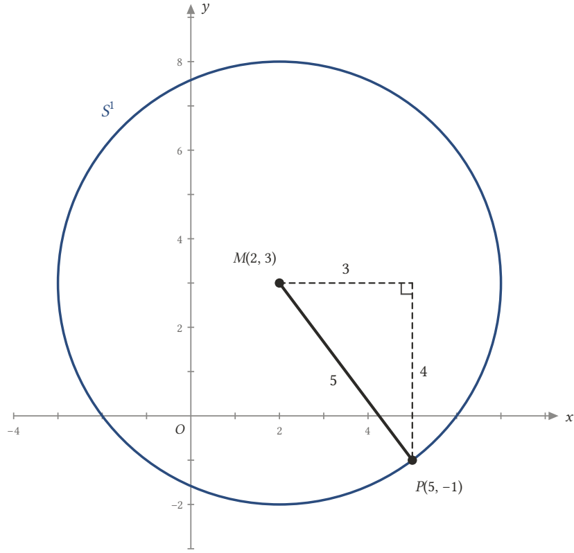
Şekil 4.23: Yarıçap |MP| , dik kenarları 3 ve 4 olan dik üçgenin hipotenüsüdür: r = 5 .
