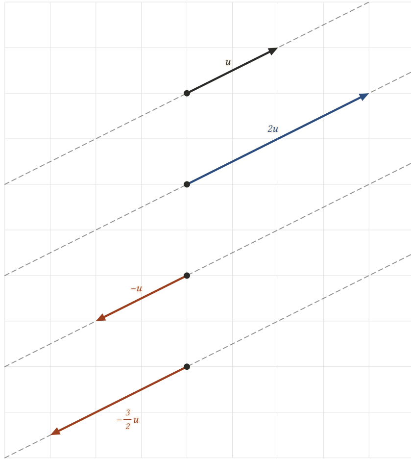
Şekil 7.11: u = (2, 1) ve katları kendi paralel doğruları üzerinde: pozitif katlar u ile aynı yönü (sağı), negatif katlar ters yönü (solu) gösterir.
