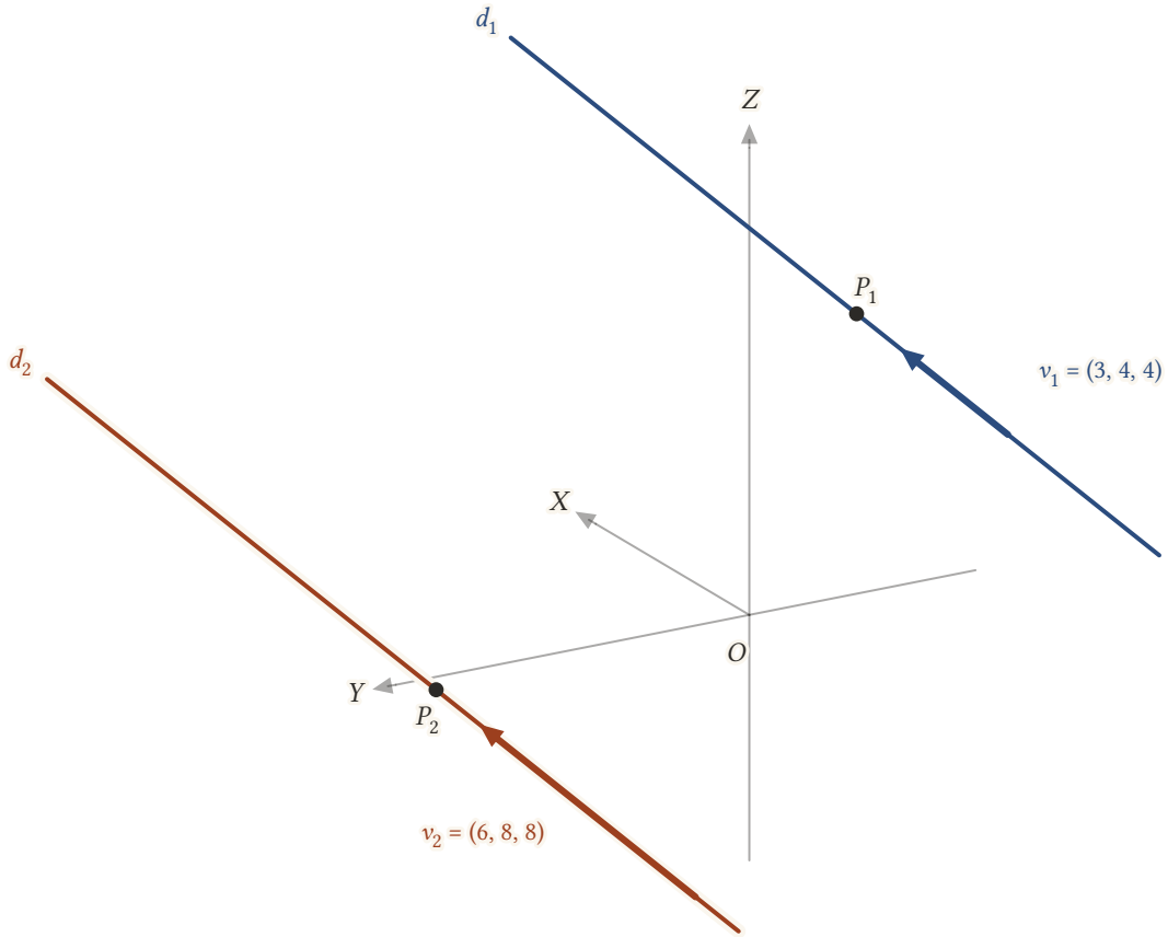
Şekil 11.15: m = 4, n = 8 için d_1 ile d_2 paralel ve farklıdır: v_2 = 2v_1 , ama P_2 d_1 üzerinde değildir. Oklar, doğrultman vektörlerinin aynı oranda kısaltılmış halleridir.
