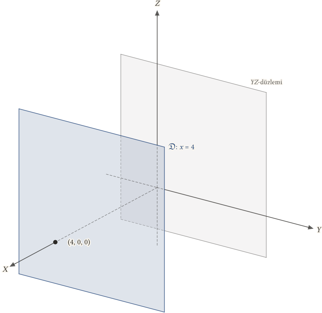
Şekil 13.17: x = 4 düzlemi YZ-düzlemine paraleldir ve X-eksenini (4, 0, 0) 'da dik keser; eksenin düzlemin arkasında kalan kısmı kesiklidir.
