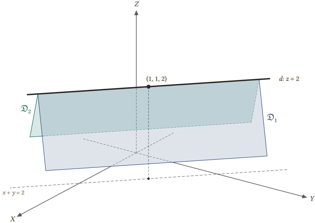
Şekil 13.6: Arakesit doğrusu d her noktasında z = 2 olan yatay bir doğrudur; bu yüzden z parametre olarak seçilemez. Kesikli doğru, d 'nin XY -düzlemindeki izdüşümü x + y = 2 'dir.
