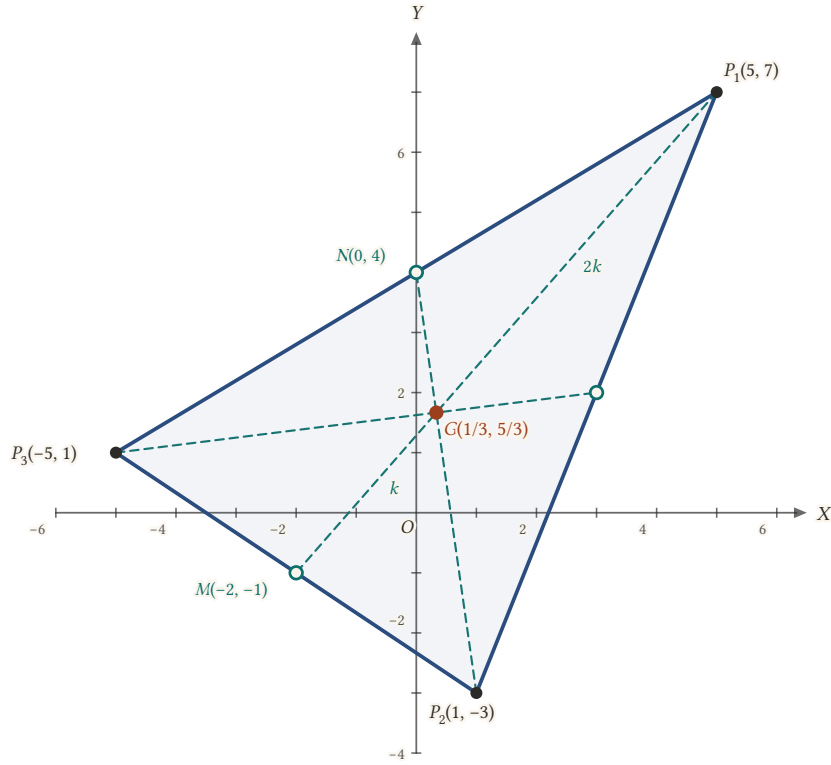
Şekil 1.30: Kenarortaylar G(1/3, 5/3) 'te kesişir; G her kenarortayı köşeden itibaren 2 : 1 oranında böler.
