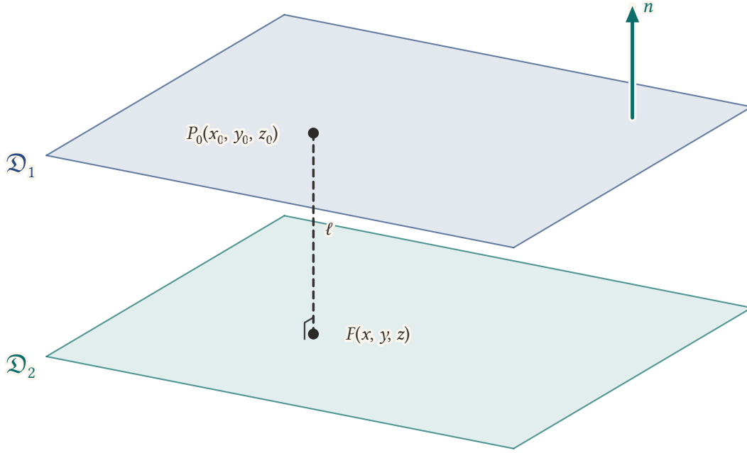
Şekil 14.11: Paralel iki düzlemin normali ortaktır: ikisi de aynı n vektörüne diktir. Üstteki düzlemin P_0 noktasından alttaki düzleme inen dikmenin uzunluğu \ell , iki düzlem arasındaki uzaklıktır.
