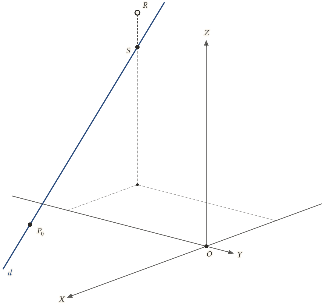
Şekil 10.3: d üzerindeki S = (-3, -5, 4) noktası ilk iki koordinatı R = (-3, -5, 5) ile aynı olan tek noktadır; R onun 1 birim üstündedir, yani d üzerinde değildir.
