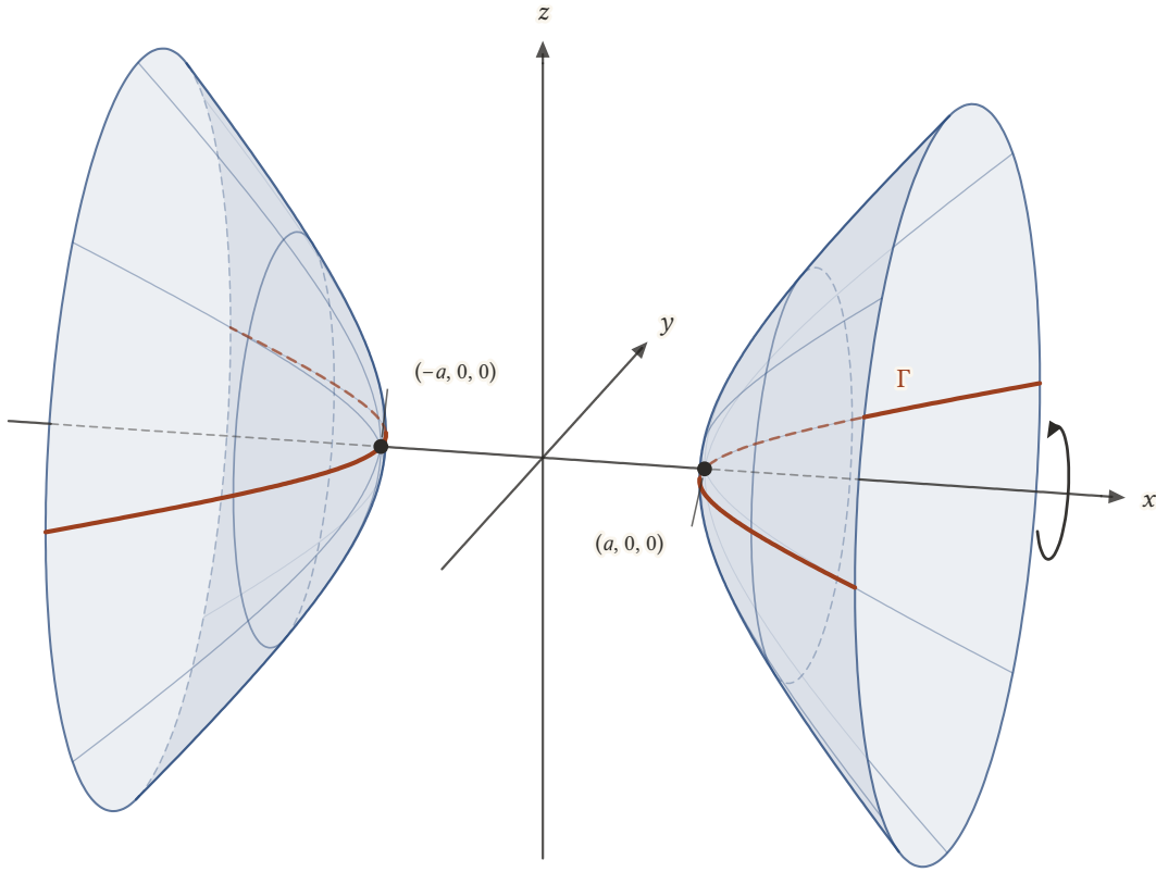
Şekil 23.16: a = b = 1 için x^2 - y^2 = 1 hiperbolünün (kırmızı, \Gamma ) x -ekseni etrafında döndürülmesiyle oluşan iki kanatlı hiperboloid x^2 - y^2 - z^2 = 1 , |x| \leq 2,5 . Kanatlar köşelerde başlar; -1 < x < 1 bölgesinde yüzey yoktur.
