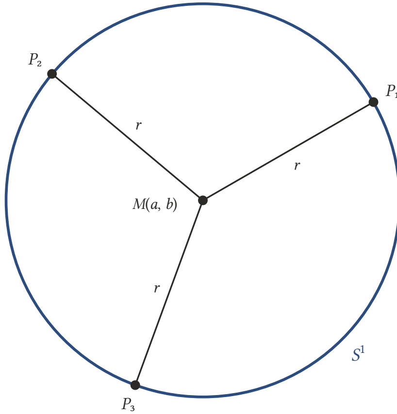
Şekil 4.1: Merkezi M , yarıçapı r olan S^1 çemberi. Çemberin her noktası merkezden aynı r uzaklığındadır.
