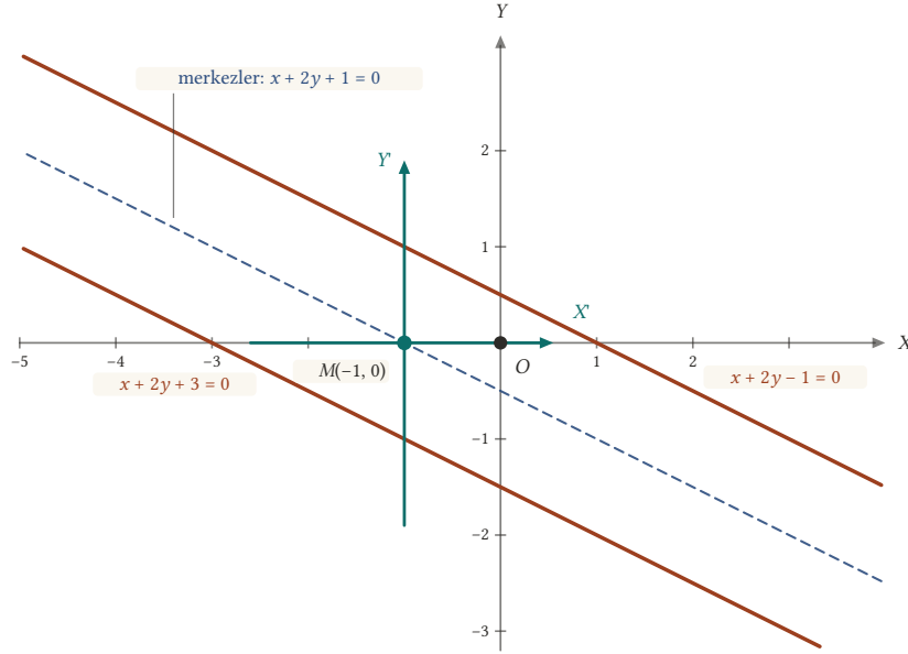
Şekil 21.9: d = D = 0 ve a'_{33} = -4 < 0 : denklem paralel iki doğrudur; merkezler aralarındaki orta doğrudur.
