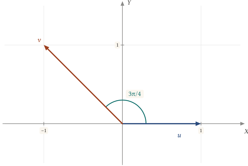
Şekil 8.5: u = (1, 0, 0) ve v = (-1, 1, 0) vektörleri XY-düzleminde yatar. Aralarındaki açı 3\pi/4 'tür; iç çarpımları negatif, açı geniştir.
