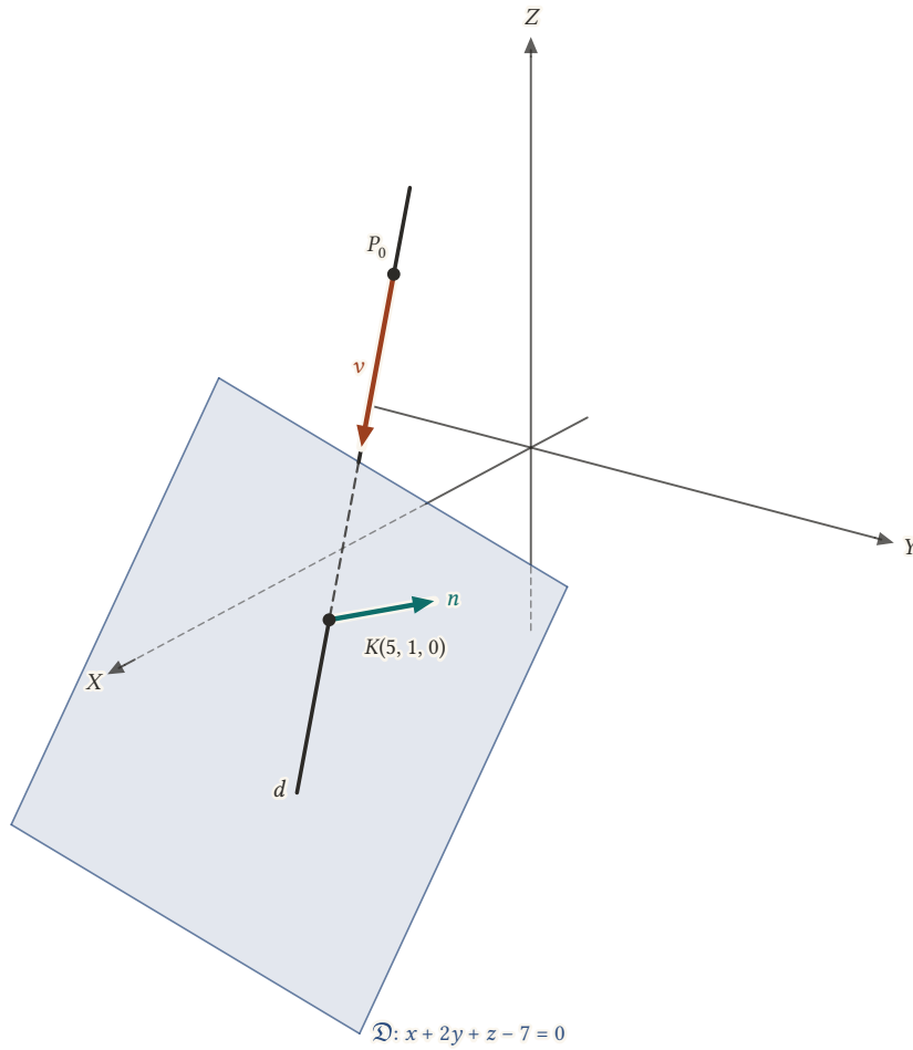
Şekil 14.5: d doğrusu düzlemi K(5, 1, 0) noktasında keser: \langle n, v \rangle = 3 \neq 0 'dır. v = (2, 1, -1) , P_0(1, -1, 2) 'dan; n = (1, 2, 1) , K 'dan çizilmiştir. Doğrunun ve eksenlerin düzlemin arkasında kalan kısımları kesiklidir.
