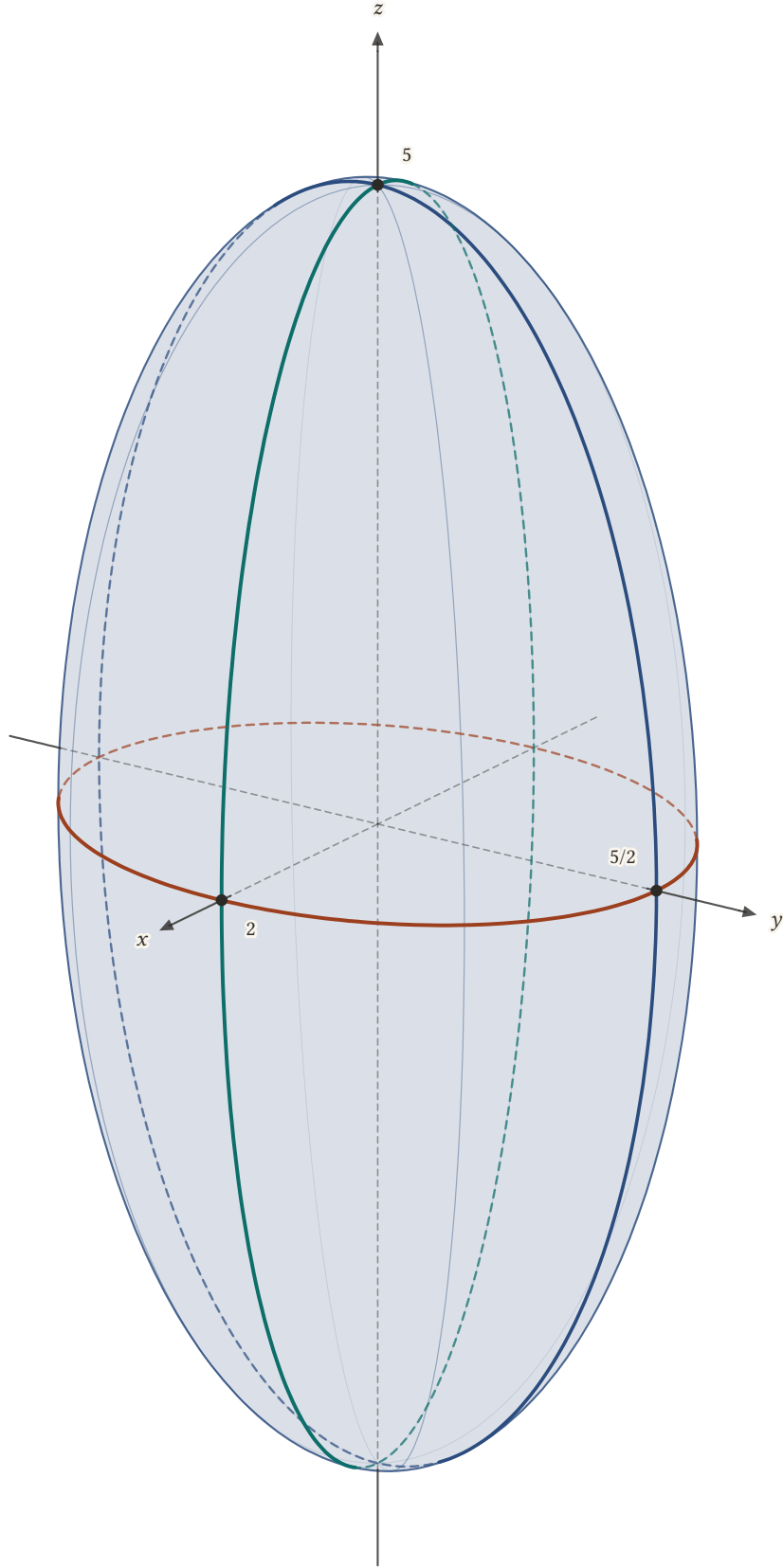
Şekil 23.26: Elipsoid x^2/4 + y^2/(25/4) + z^2/25 = 1 (yarı eksenler 2, 5/2, 5) ve koordinat düzlemlerindeki izleri: z = 0 (kırmızı), y = 0 (yeşil), x = 0 (mavi). Yüzey z doğrultusunda uzamıştır.
