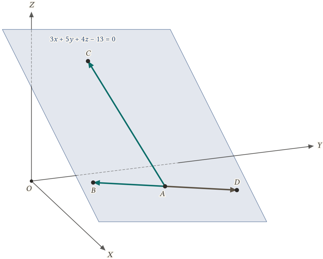
Şekil 12.12: A, B, C, D noktaları aynı düzlemde: AB, AC ve AD vektörleri düzlemin içinde kalır.
