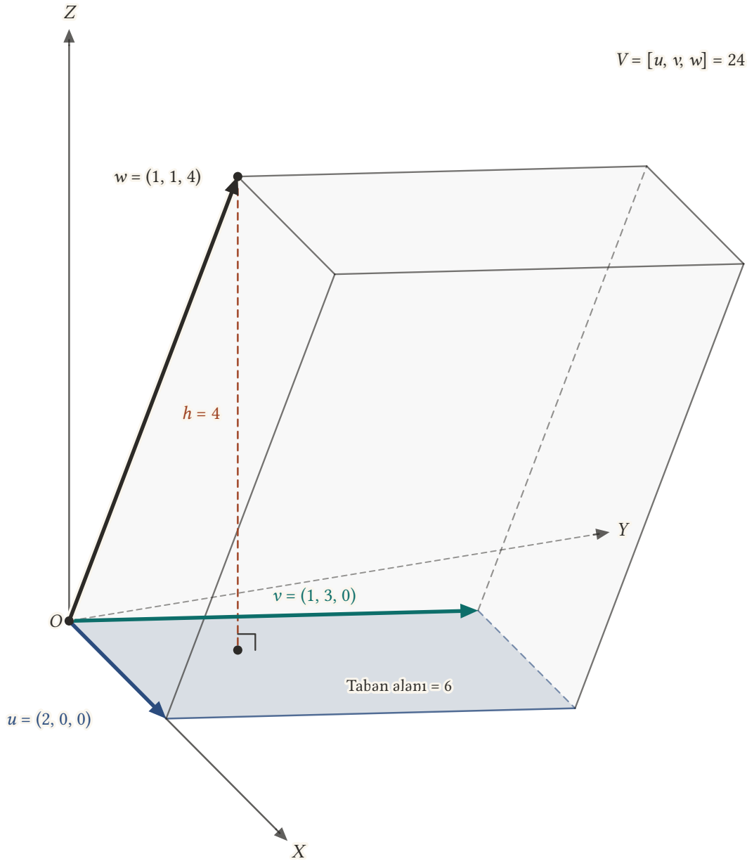
Şekil 9.10: u = (2, 0, 0) , v = (1, 3, 0) , w = (1, 1, 4) üzerine kurulan paralelyüz. Taban XY düzleminde ve alanı 6'dır; w 'nin ucu düzlemden 4 birim yukarıdadır. Hacim 6 \cdot 4 = 24 = [u, v, w] .
