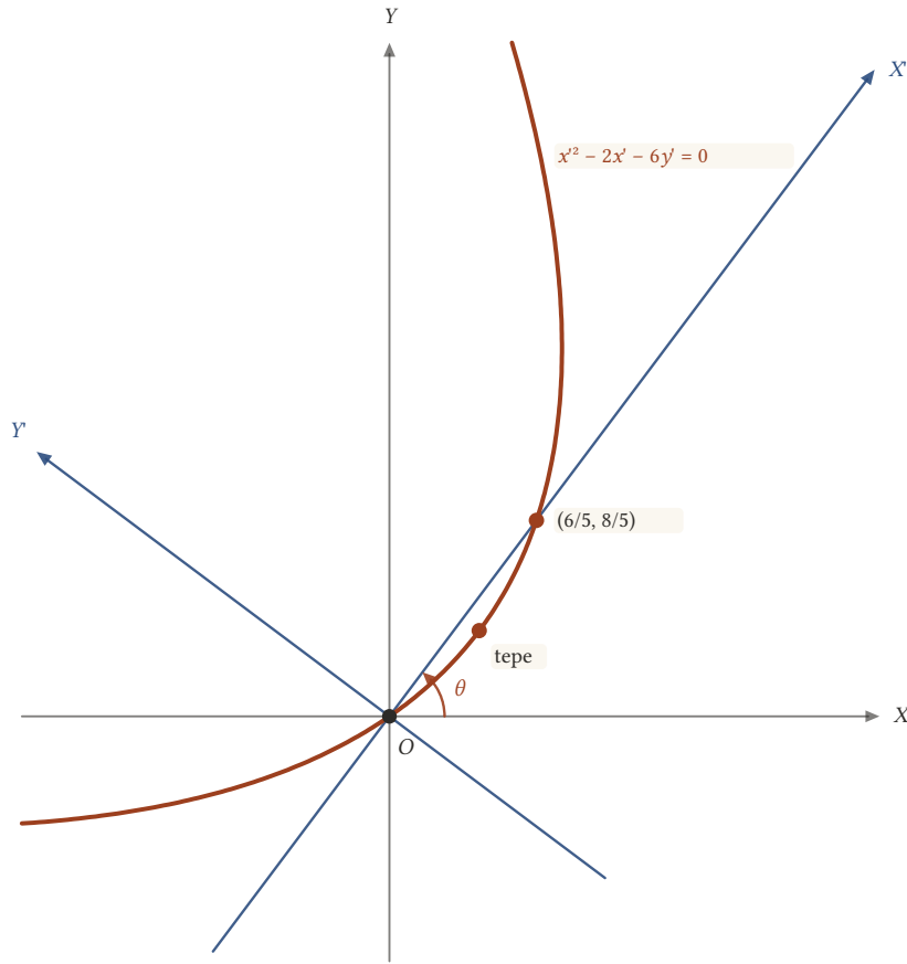
Şekil 17.24: Eksenler \theta = \arctan(4/3) kadar döndürülünce 9x^2 + 24xy + 16y^2 + 90x - 130y = 0 eğrisi x'^2 - 2x' - 6y' = 0 olur; eğrinin simetri eksenini Y' -eksenine paraleldir.
