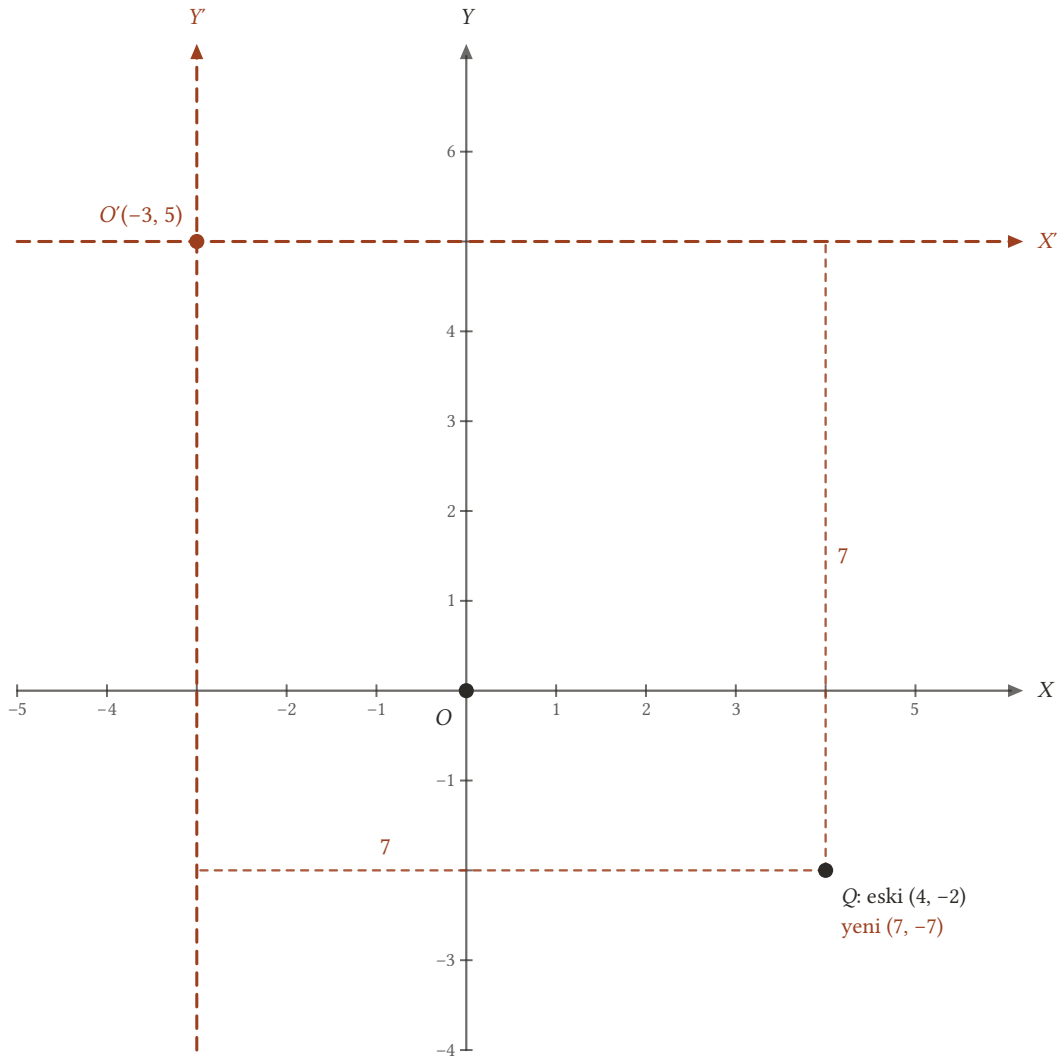
Şekil 16.9: Başlangıç noktası O'(-3, 5) olan yeni sistemde Q(4, -2) noktasının koordinatları (7, -7) 'dir.
