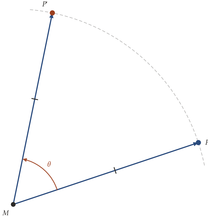
Şekil 17.1: M merkezli \theta radyanlık dönme P 'yi, M 'ye uzaklığı aynı kalacak ve MP 'den MP' 'ne açı \theta olacak biçimde P 'ne götürür.
