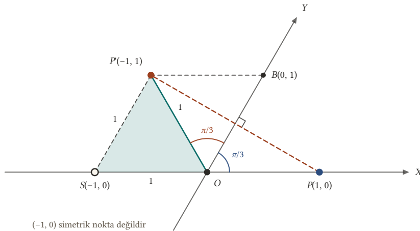
Şekil 5.3: \alpha = \pi/3 olan eğik sistemde Y -eksenine göre yansıma. P(1, 0) 'ın simetriği P(-1, 1) 'dir; OSP eşkenar üçgendir ve OSPB bir paralelkenardır.
