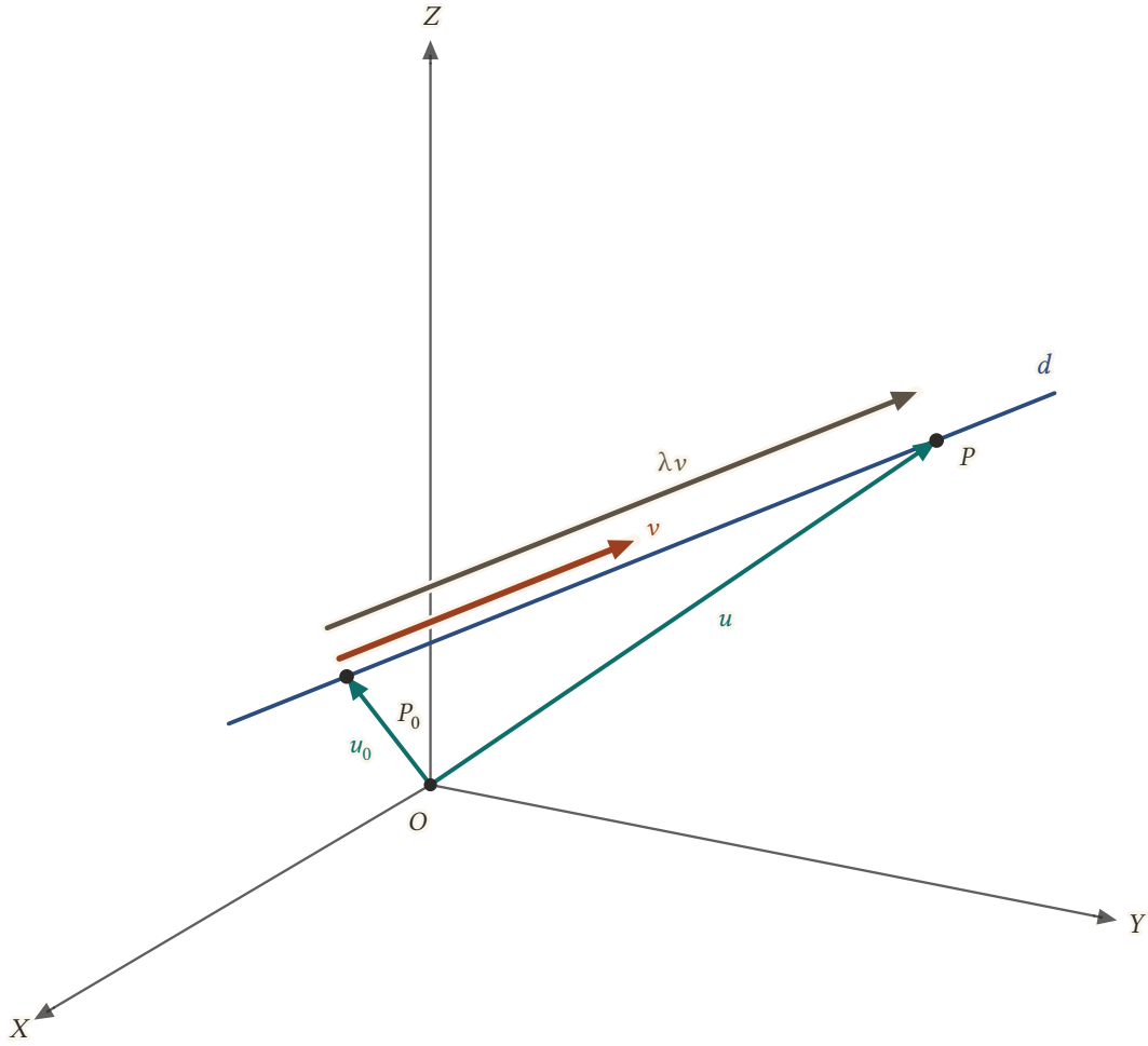
Şekil 10.1: d doğrusu P_0 'dan geçer ve doğrultmanı v 'dir. P 'ye O 'dan doğrudan ( u ) ya da önce P_0 'a ( u_0 ), sonra doğru boyunca \lambda v kadar giderek varılır: u = u_0 + \lambda v .
