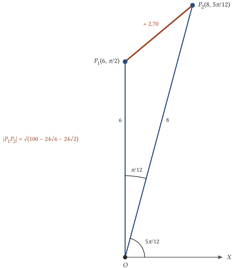
Şekil 5.21: (6, \pi/2) ve (8, 5\pi/12) noktaları kutuptan \pi/12 = 15^\circ farklı yönlerde görünür; aralarındaki uzaklık yaklaşık 2,70'tir.
