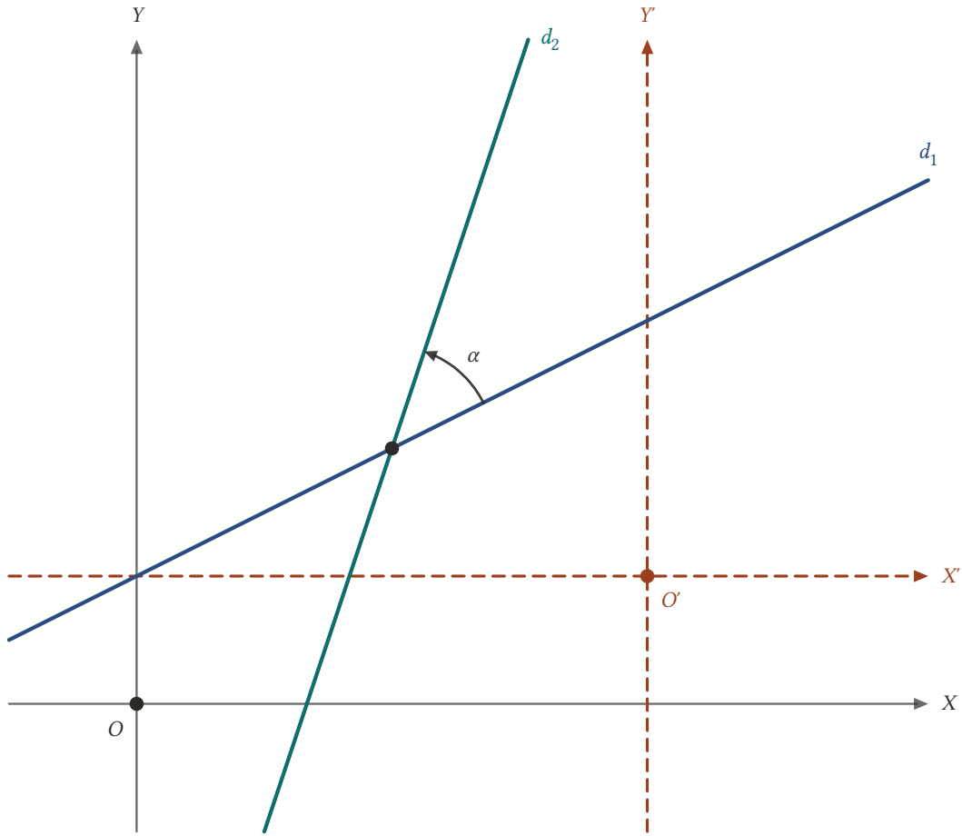
Şekil 16.11: Eksenler ötelenince d_1 ile d_2 doğrularının denklemleri değişir, eğimleri ve aralarındaki \alpha açısı değişmez.
