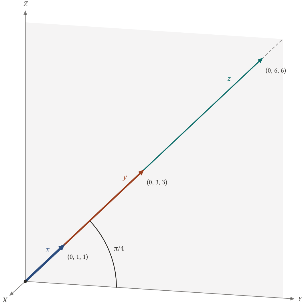
Şekil 8.22: x = (0, 1, 1) , y = (0, 3, 3) , z = (0, 6, 6) YZ -düzleminde, y = z açkırtay doğrusu üzerindedir; bu doğru Y -ekseniyle \pi/4 açı yapar. Kısa oklar uzunların üstüne daha kalın çizilmiştir.
