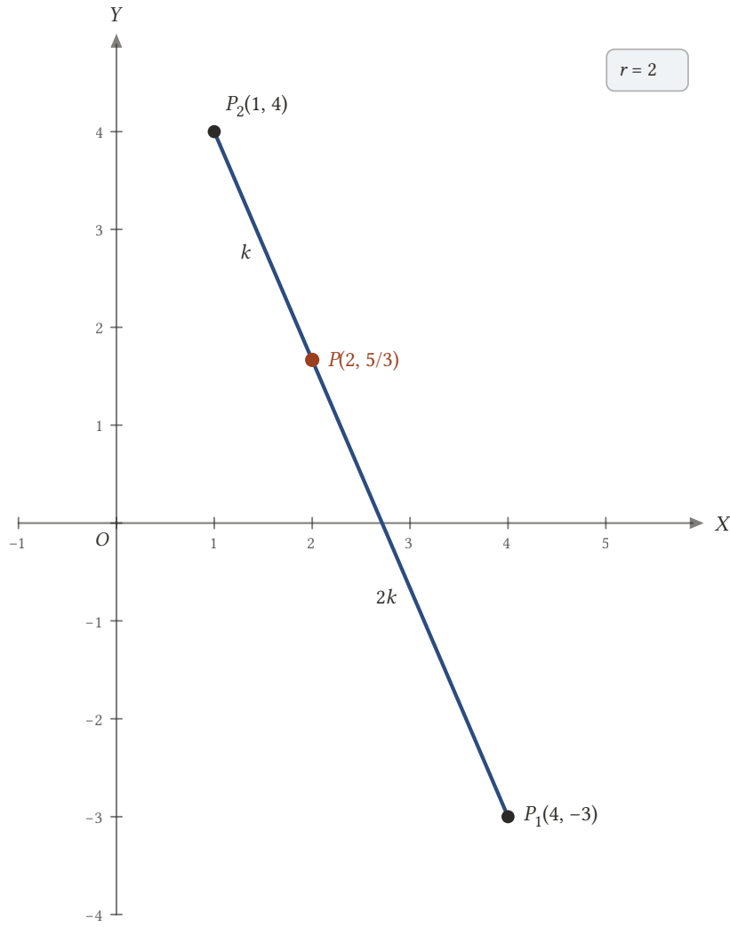
Şekil 2.6: P_1(4, -3) ve P_2(1, 4) uç noktalı parçayı r = 2 oranında bölen nokta P(2, 5/3) ; |P_1P| , |PP_2| uzunluğunun iki katıdır.
