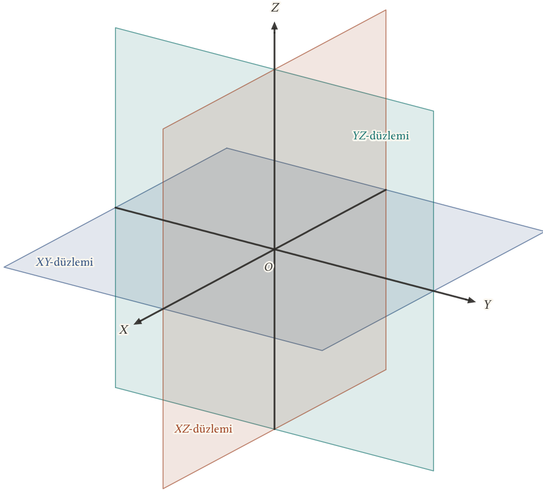
Şekil 6.2: Üç koordinat düzlemi: XY-düzlemi ( z = 0 , mavi), YZ-düzlemi ( x = 0 , yeşil) ve XZ-düzlemi ( y = 0 , turuncu). İkişer ikişer kesişme doğruları koordinat eksenleridir; düzlemlerin yalnız -3 ile 3 arasındaki parçaları çizilmiştir.
