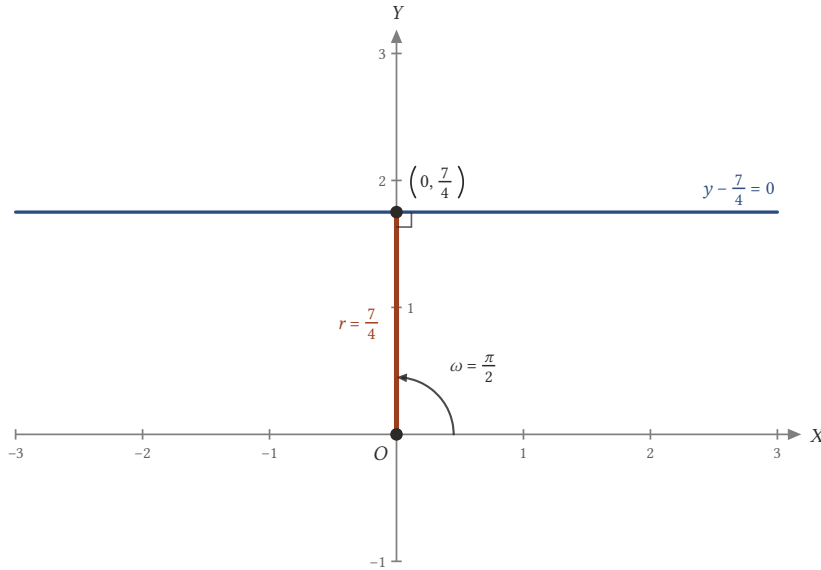
Şekil 3.9: 4y - 7 = 0 doğrusuna orijinden inen dikme Y -ekseninin pozitif yarısı üzerindedir: r = 7/4, \omega = \pi/2 .
