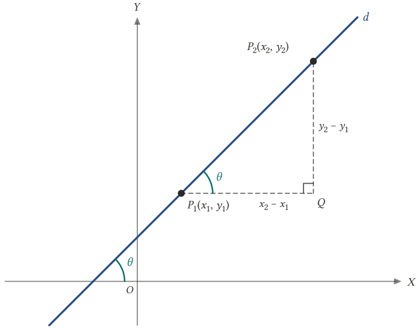
Şekil 2.11: Dar eğim açısında P_1QP_2 dik üçgeninin P_1 köşesindeki açı \theta 'dır (yöndeş açı); bu yüzden \tan \theta = (y_2 - y_1) / (x_2 - x_1) .
