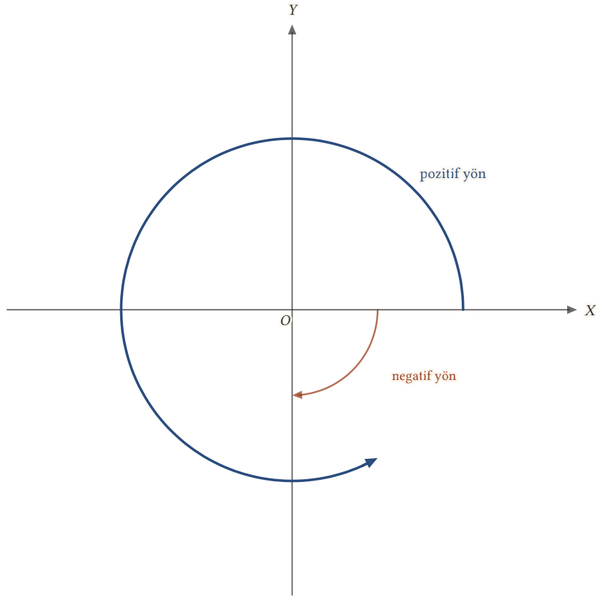
Şekil 1.5: Saat yönünün tersi pozitif yön, saat yönü negatif yöndür.
