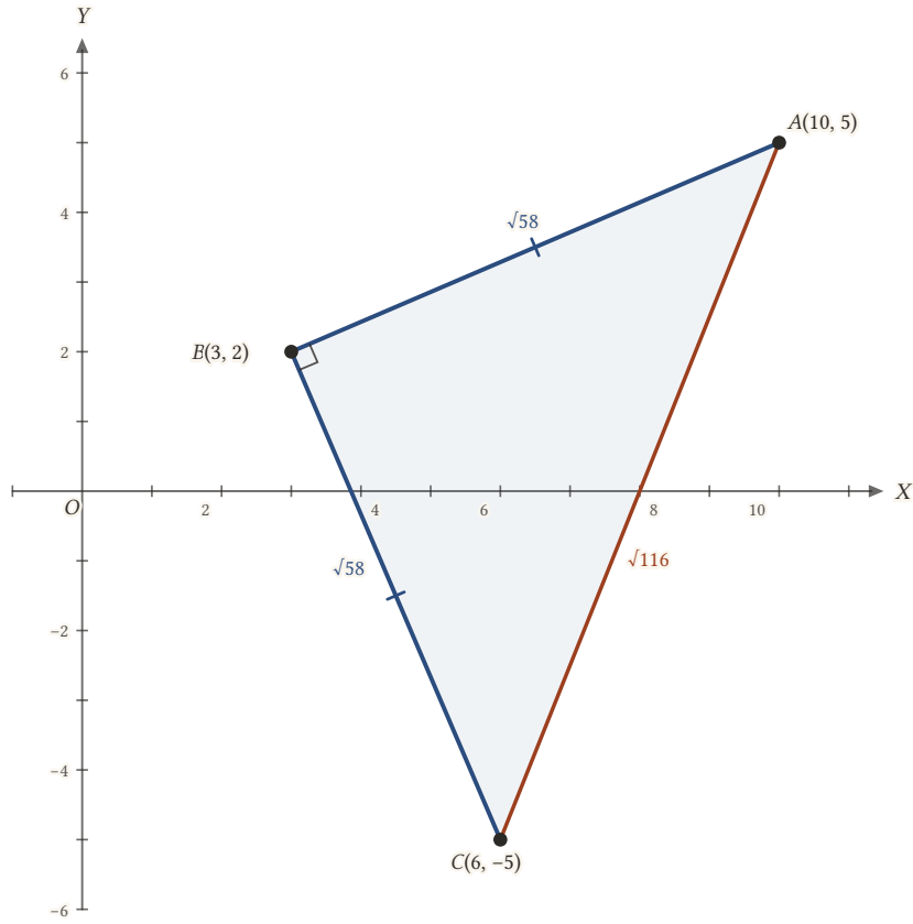
Şekil 1.24: 58 + 58 = 116 olduğundan B açısı diktir; üçgen ikizkenar dik üçgendir.
