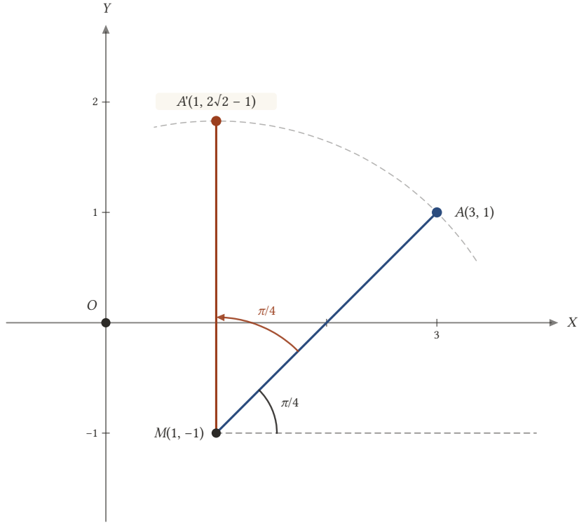
Şekil 17.7: A(3, 1) , M(1, -1) etrafında \pi/4 döndürülünce A'(1, 2\sqrt{2} - 1) olur; MA' düşeydir.
