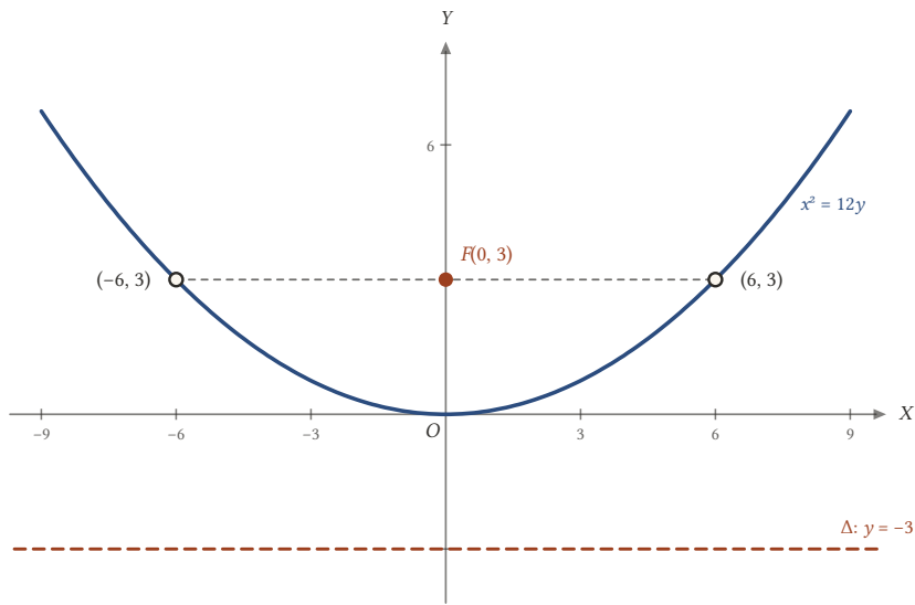
Şekil 20.4: x^2 = 12y köşe O , odak F(0, 3) , doğrultman y = -3 ; odak hizasındaki kirişin uzunluğu 2p = 12 .
