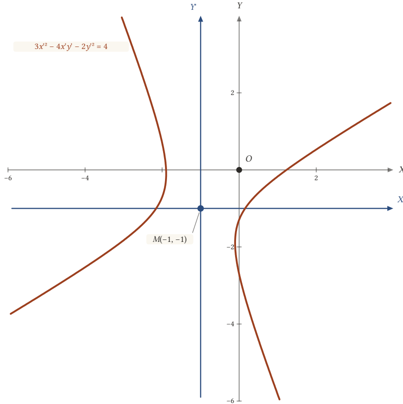
Şekil 21.18: Hiperbolün merkezi M(-1, -1) ; eksenler M 'ye ötelenince birinci dereceden terimler kaybolur.
