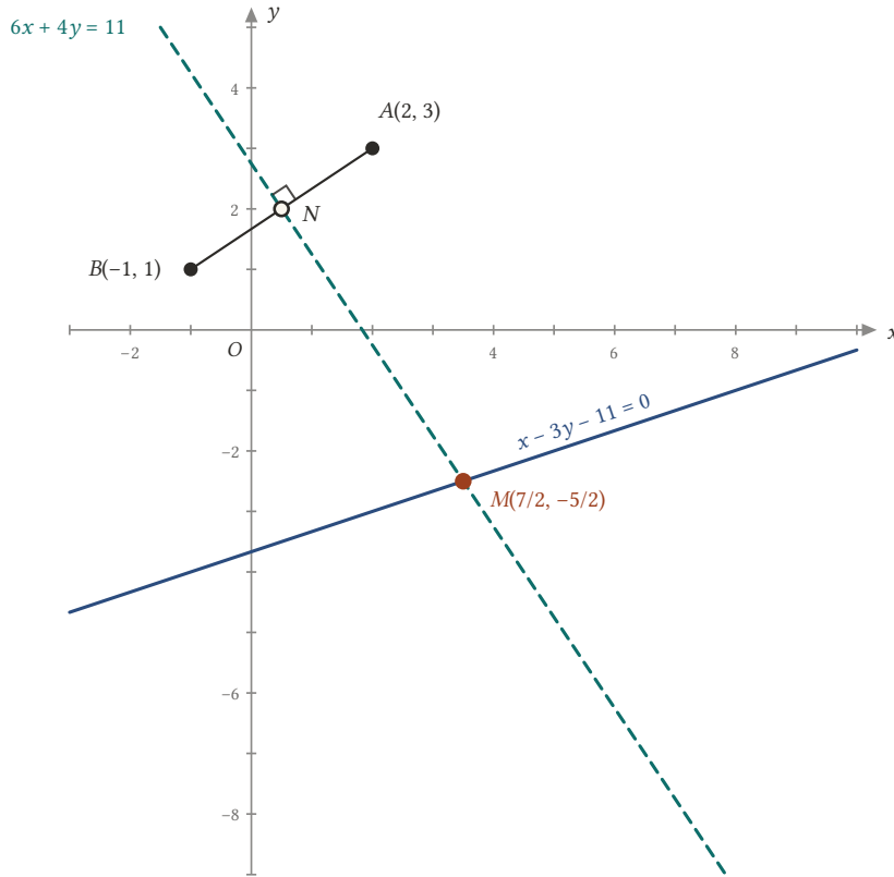
Şekil 4.6: A ile B 'ye eşit uzaklıktaki noktalar, AB 'nin orta noktası N 'den geçen dik doğru 6x + 4y = 11 'dir. Merkez hem bu doğru hem de x - 3y - 11 = 0 doğrusu üzerinde olduğundan ikisinin kesişimidir.
