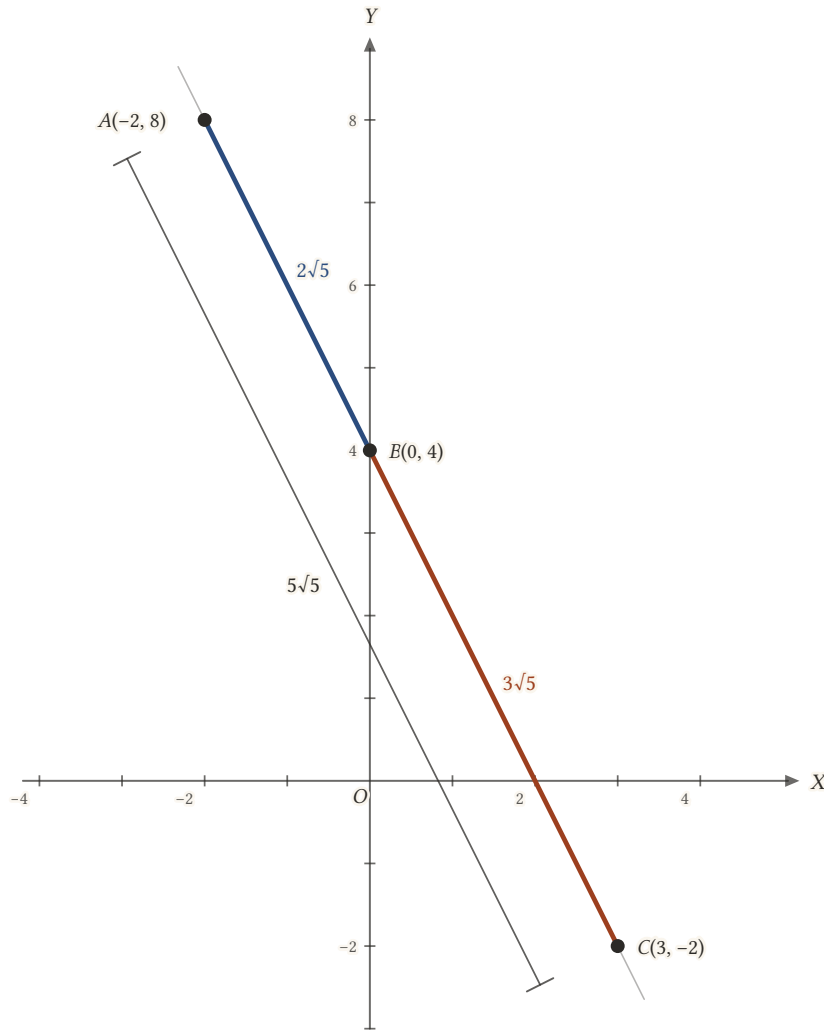
Şekil 1.18: |AB| + |BC| = 2\sqrt{5} + 3\sqrt{5} = 5\sqrt{5} = |AC| : B , AC doğru parçası üzerindedir.
