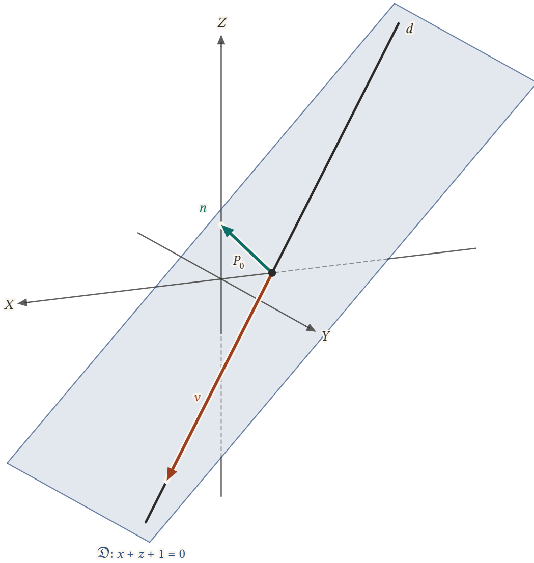
Şekil 14.4: d doğrusu düzlemin içinde yatar: doğrultman vektörü v = (3, 2, -3) , düzlemin normali n = (1, 0, 1) 'e diktir ve P_0(-1, 0, 0) düzlemin üzerindedir. Eksenlerin düzlemin arkasında kalan kısımları kesiklidir.
