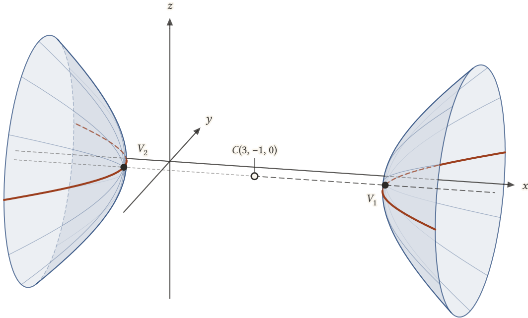
Şekil 23.33: İki kanatlı hiperboloid (x - 3)^2/18 - (y + 1)^2/12 - z^2/9 = 1 , -4 \leq x \leq 10 . Merkez C(3, -1, 0) (içi boş nokta; yüzeyde değildir), eksen C 'den geçen ve x -eksenine paralel kesikli doğrudur. Köşeler V_1(3 + 3\sqrt{2}, -1, 0) ve V_2(3 - 3\sqrt{2}, -1, 0) ; kırmızı eğri z = 0 düzlemindeki hiperbolün kollarıdır.
