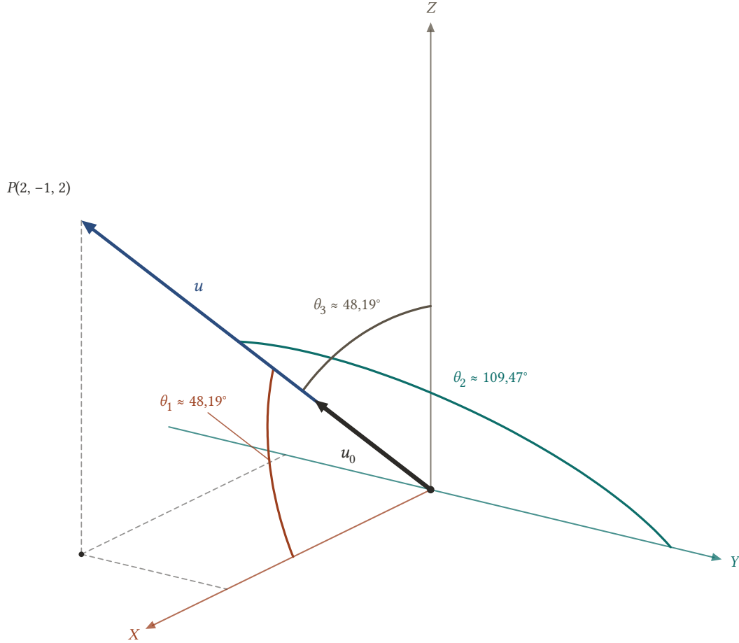
Şekil 8.13: u = (2, -1, 2) ve u yönündeki birim vektör u_0 = (2/3, -1/3, 2/3) . u , Y -ekseninin pozitif yönüyle geniş açı, öteki iki eksenle eşit dar açılar yapar.
