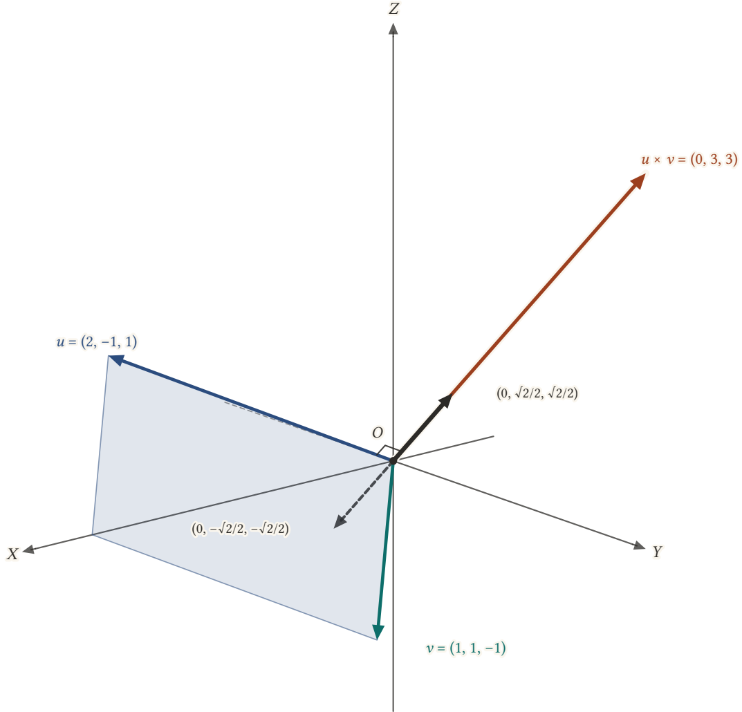
Şekil 9.4: u = (2, -1, 1) ile v = (1, 1, -1) vektörlerinin düzlemi ve ona dik u \times v = (0, 3, 3) . Bu doğrultudaki iki birim vektör (0, \sqrt{2}/2, \sqrt{2}/2) ve düzlemin arkasına düşen, kesikli çizilen (0, -\sqrt{2}/2, -\sqrt{2}/2) 'dir.
