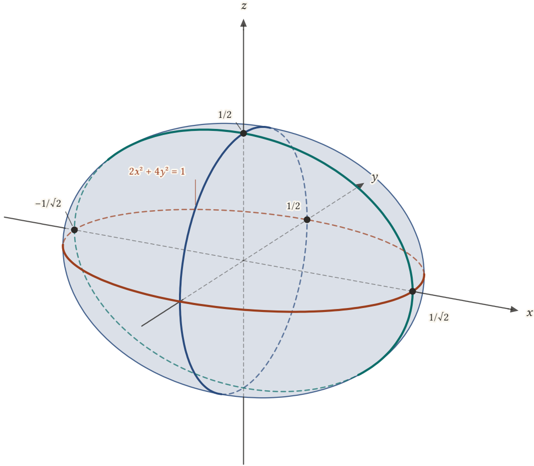
Şekil 23.13: Dönel elipsoid 2x^2 + 4y^2 + 4z^2 = 1 : xy -düzlemindeki iz 2x^2 + 4y^2 = 1 elipsi (kırmızı, üreteç), xz -düzlemindeki iz 2x^2 + 4z^2 = 1 elipsi (yeşil), yz -düzlemindeki iz yarıçapı 1/2 olan çember (mavi). Yüzey x -ekseni boyunca \pm 1/\sqrt{2} 'ye uzanır.
