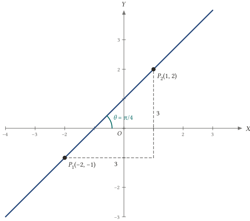
Şekil 2.13: P_1(-2, -1) ve P_2(1, 2) 'den geçen doğruya yatay ve düşey değişim 3'er birimdir; eğim 1, eğim açısı \pi/4 'tür.
