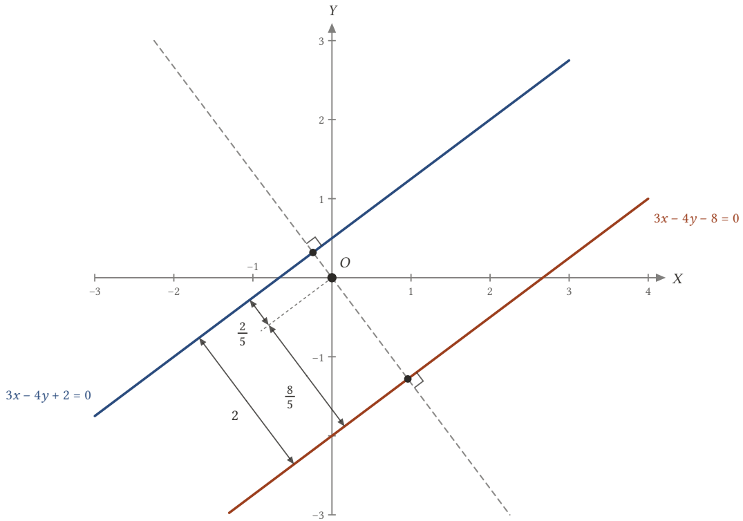
Şekil 3.22: Paralel 3x - 4y + 2 = 0 ve 3x - 4y - 8 = 0 doğruları orijinin iki yanındadır: orijine uzaklıkları 2/5 ve 8/5 , aralarındaki uzaklık 2/5 + 8/5 = 2 'dir. Ölçüler, ortak dikme doğrultusunda çizilmiştir.
