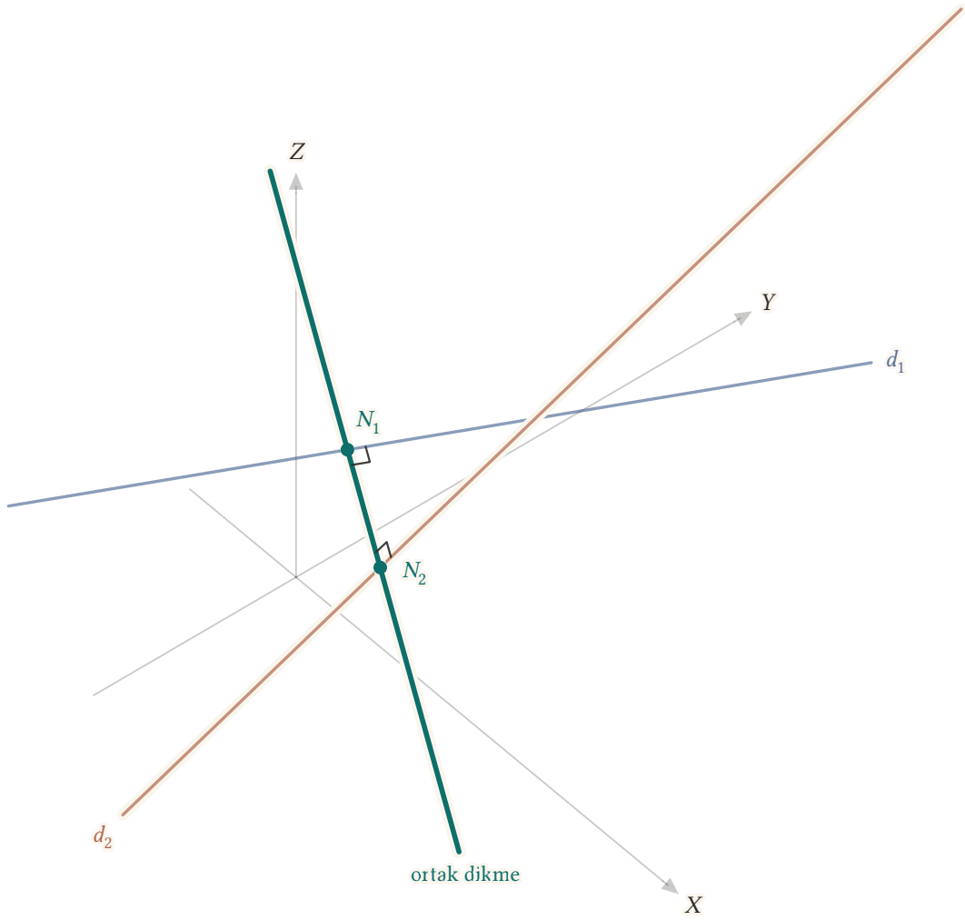
Şekil 11.18: N_1 ve N_2 'den geçen ortak dikme doğrusu; doğrultman vektörü (4, -2, -1) , v_1 \times v_2 'ye paraleldir ve doğru iki doğruyu da dik keser.
