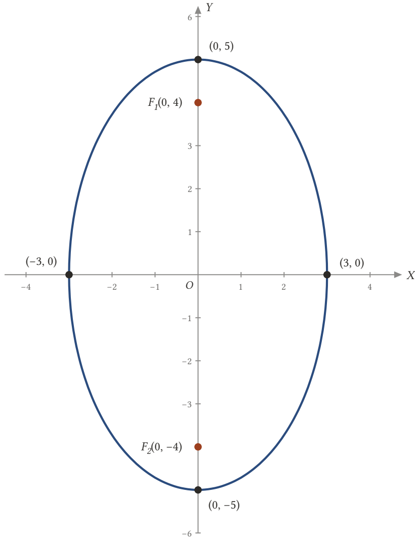
Şekil 18.10: x^2/9 + y^2/25 = 1 elipsinin asal eksenini Y -eksenidir: uzak köşeler (0, \pm 5) , yakın köşeler (\pm 3, 0) , odaklar (0, \pm 4) .
