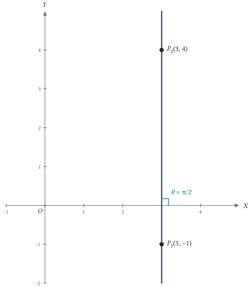
Şekil 2.15: P_1(3, -1) ve P_2(3, 4) 'ten geçen doğru düşeydir: eğim açısı \pi/2 , eğimi tanımsızdır.
