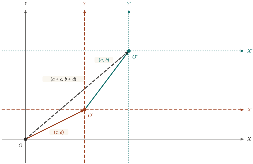
Şekil 16.22: Önce (c, d) , sonra (a, b) kadar ötelenen eksenler, (a + c, b + d) kadar tek ötelemeye aynı yere gelir.
