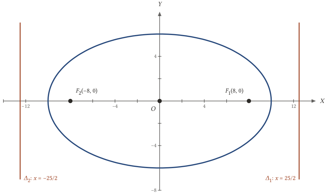
Şekil 19.17: Elipsin doğrultmanları elipsin dışında, x = \pm 25/2 'de durur.
