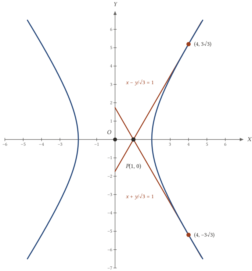
Şekil 19.11: P(1, 0) 'dan hiperbole çizilen iki teğet, sağ kola (4, \pm 3\sqrt{3}) 'te değer.
