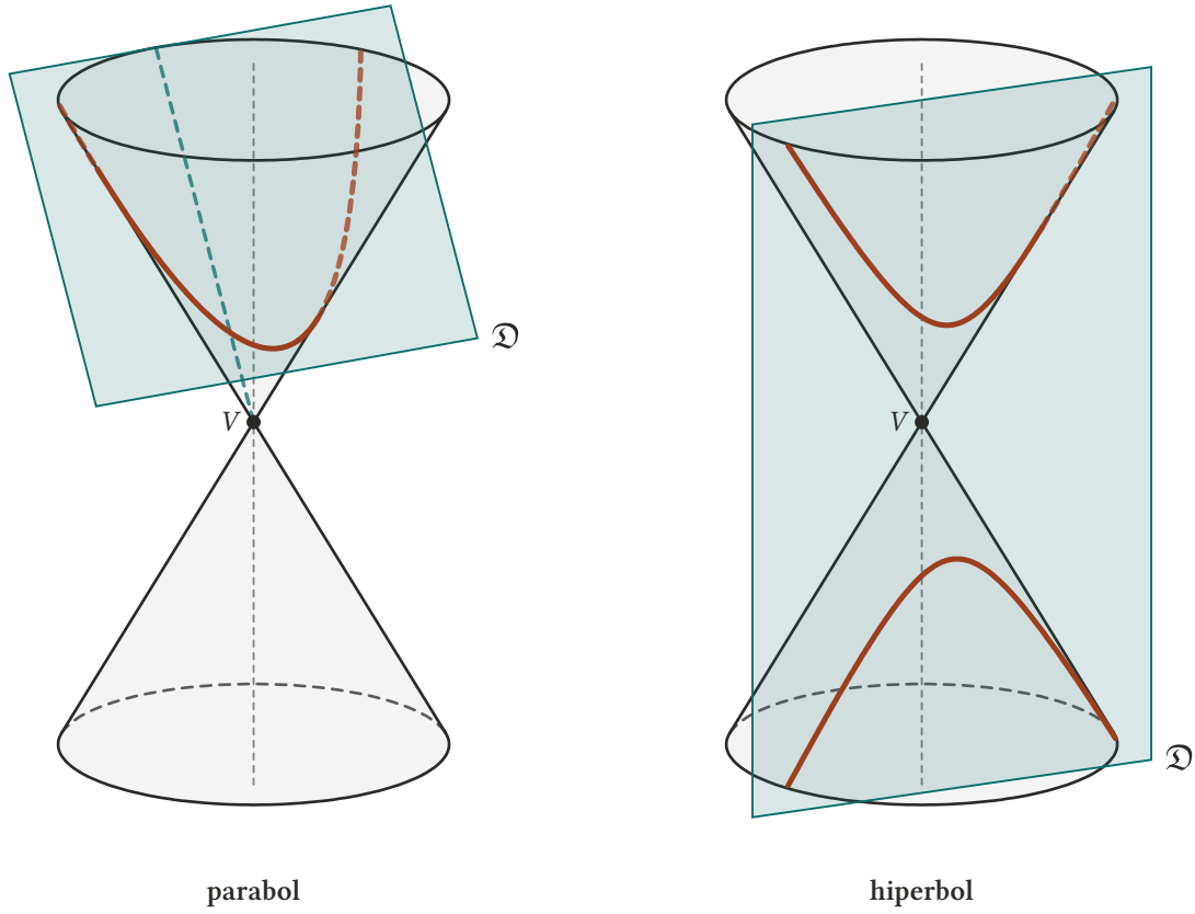
Şekil 18.2: Bir ana doğruya paralel düzlem koniyi kapanmayan tek kollu bir eğri, parabol boyunca keser; eksene paralel düzlem ise iki parçayı birden keser ve iki kollu hiperbolü verir.
