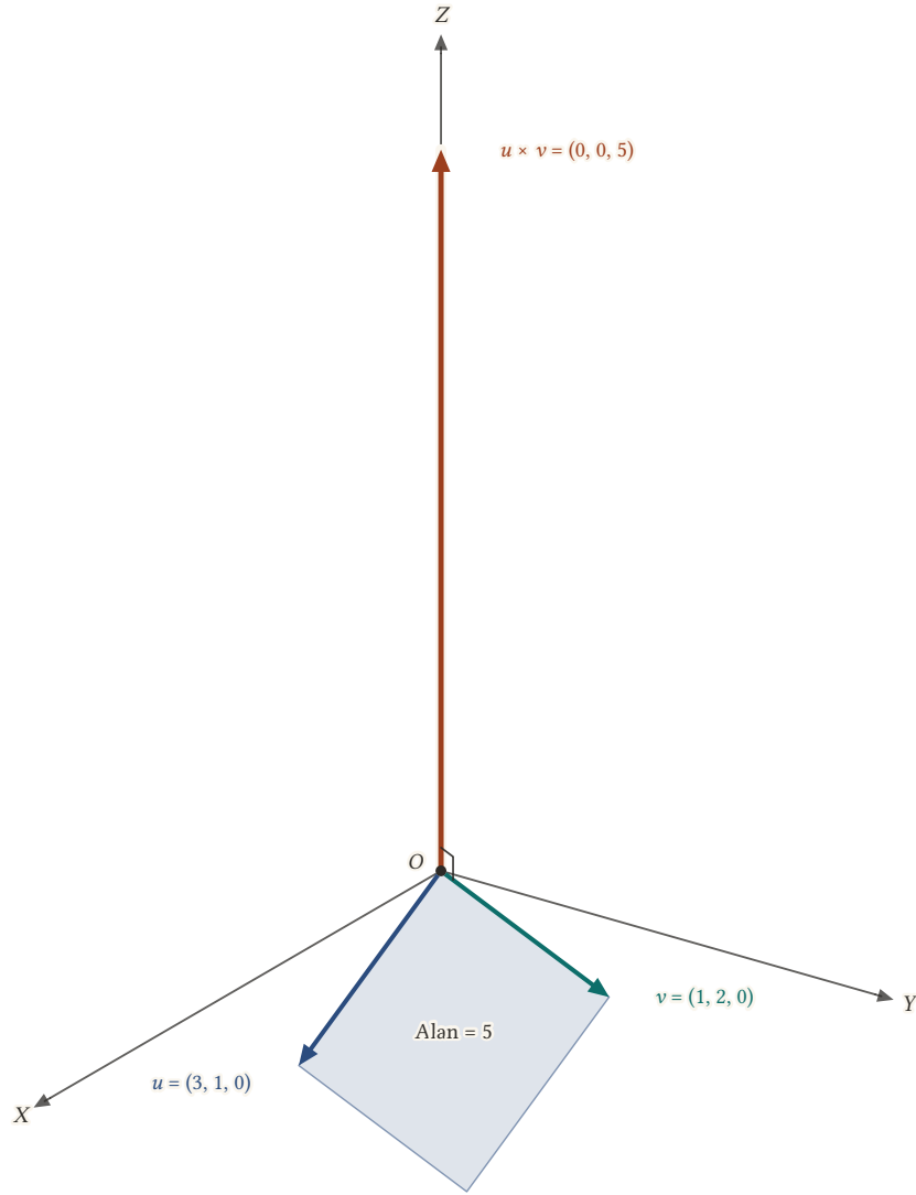
Şekil 9.13: XY düzlemindeki u = (3, 1, 0) ve v = (1, 2, 0) üzerine kurulan paralelkenar. u \times v = (0, 0, 5) Z eksenini üzerindedir ve uzunluğu alana, 5'e eşittir.
