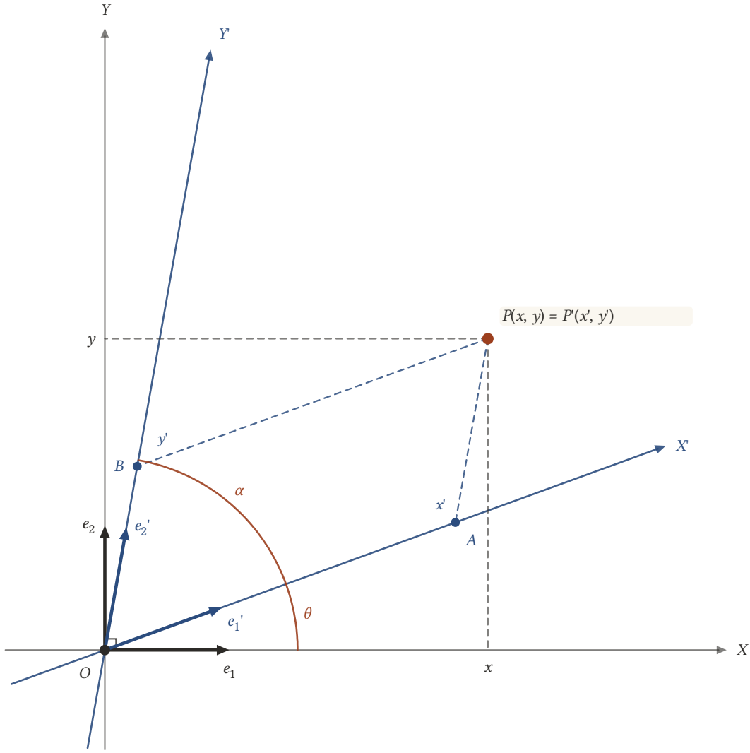
řekil 17.15: Dik sistemde P'nin koordinatları dikmelerle (x, y) , eğik sistemde eksenlere paralellerle (x', y') okunur; OP = x e_1 + y e_2 = x' e_1' + y' e_2' .
