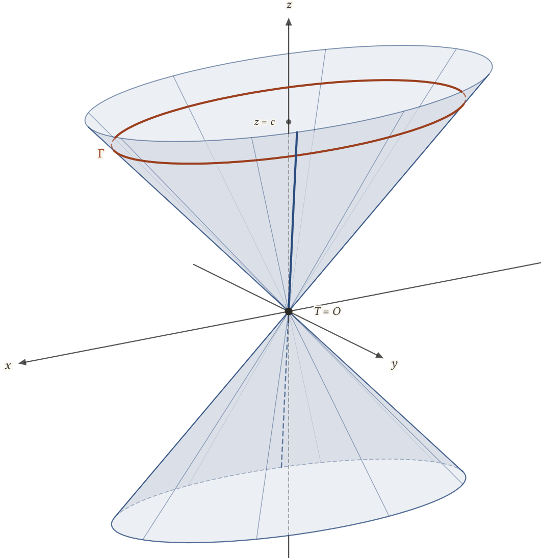
Şekil 23.10: a = 2, b = 1, c = 2 için tepe noktası başlangıç noktası olan eliptik koni x^2/4 + y^2 = z^2/4 . Dayanak elipsi \Gamma (kırmızı) z = c düzleminindedir; üreteçler O 'dan geçip alt kanada uzanır, alt kanattaki elips z = -2 kesitidir.
