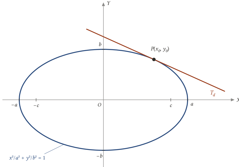
Şekil 18.13: Elipsin P(x_0, y_0) noktasındaki teğeti x_0 x/a^2 + y_0 y/b^2 = 1 doğrusudur; elipsle yalnız bu noktada buluşur.
