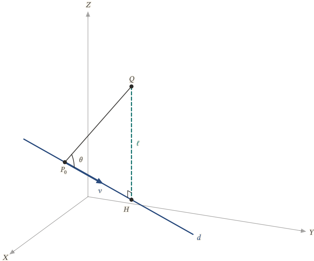
Şekil 11.3: Q noktasından d doğrusuna inilen dikme QH ; uzunluğu \ell = |QH| , Q 'nın d 'ye uzaklığıdır. \theta , d 'nin doğrultman vektörü v ile P_0Q arasındaki açıdır.
