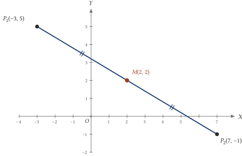
Şekil 2.3: P_1(-3, 5) ve P_2(7, -1) uç noktalı parçanın orta noktası M(2, 2) ; çift çentikler |P_1M| = |MP_2| eşitliğini gösterir.
