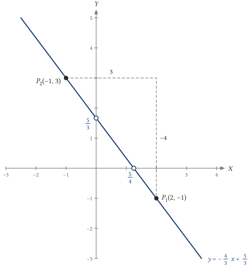
Şekil 3.3: P_1(2, -1) ve P_2(-1, 3) 'ten geçen doğru. Eğim üçgeninde x 3 artarken y 4 azalır; doğru eksenleri (\frac{5}{4}, 0) ve (0, \frac{5}{3}) noktalarında keser.
