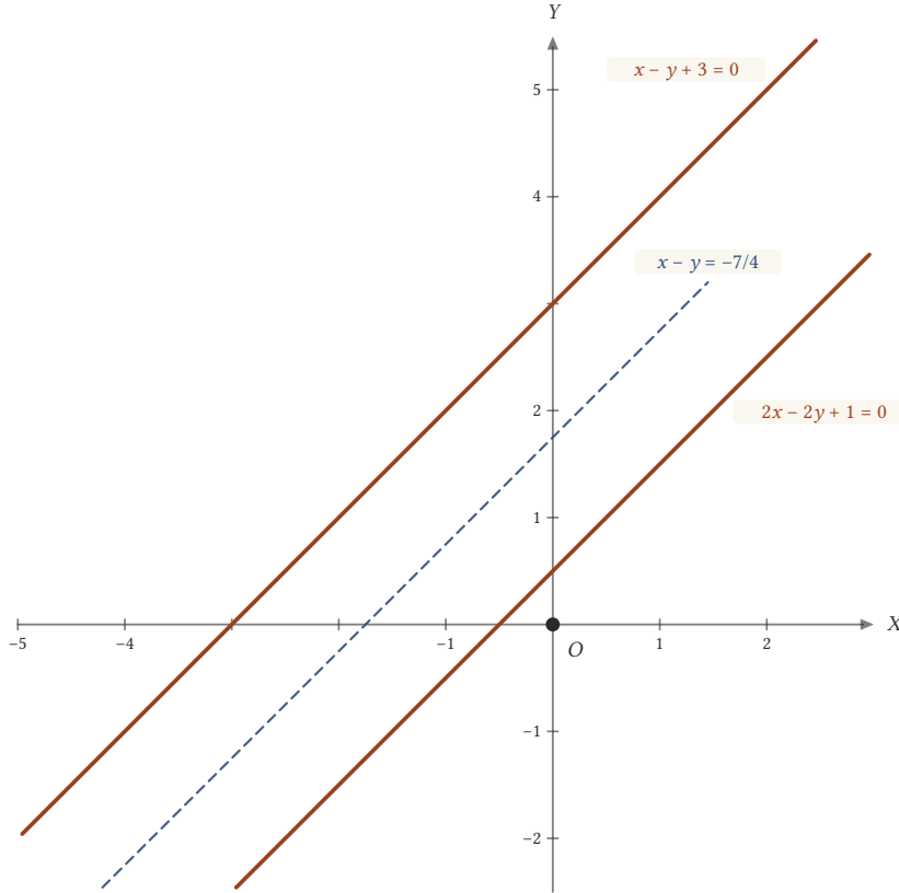
Şekil 21.21: d = D = 0 ve a'_{33} = -25/8 < 0 : denklem paralel iki doğrudur.
