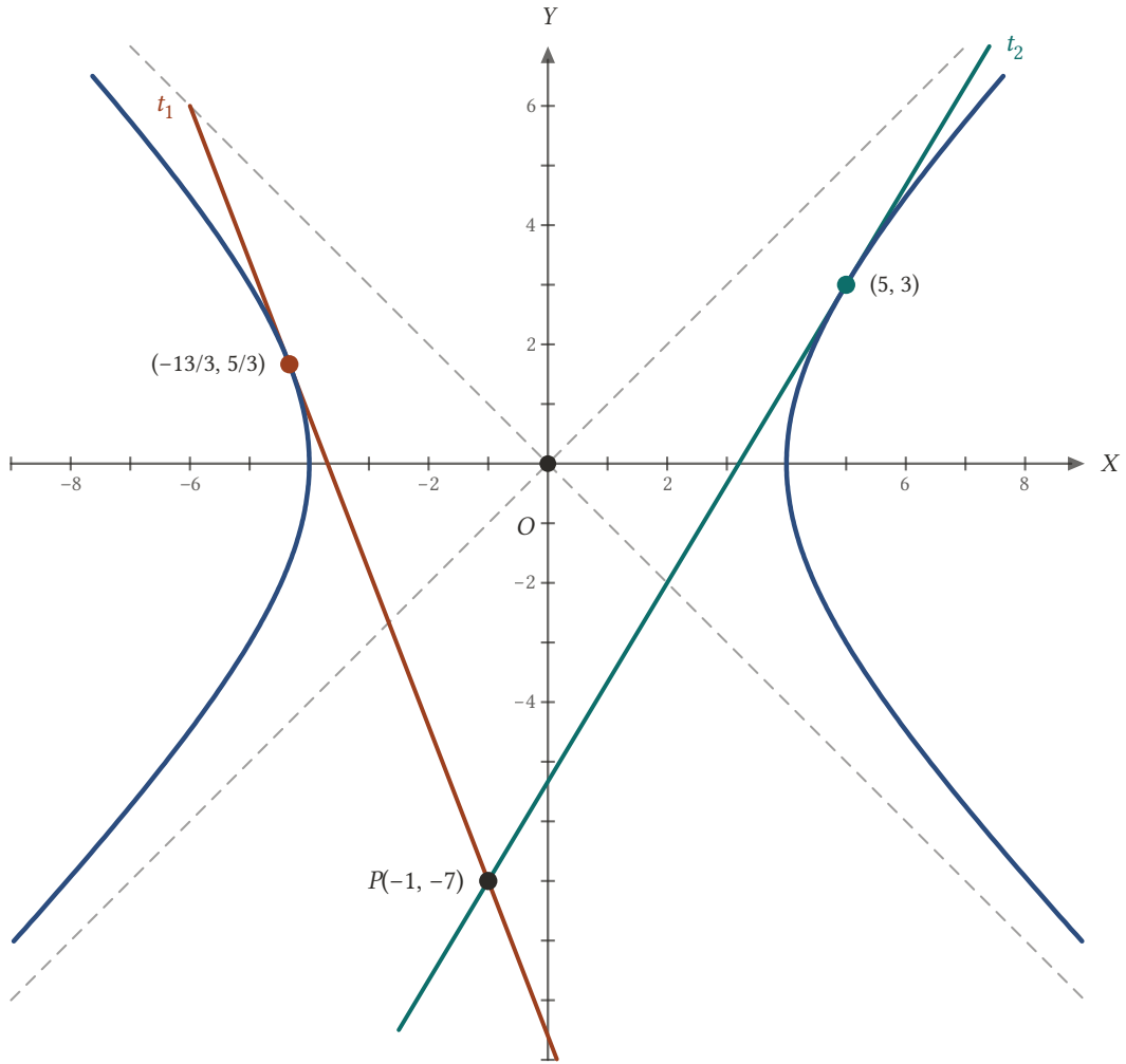
Şekil 19.25: P(-1, -7) 'den çizilen iki teğetten biri sol kola, öteki sağ kola değer.
