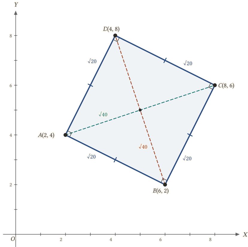
Şekil 1.35: Dört kenarı \sqrt{20} , köşegenleri \sqrt{40} olan ve açıları dik olan ABCD bir karedir.
