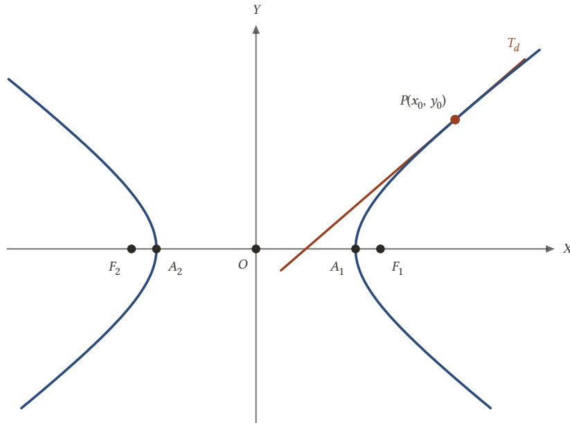
Şekil 19.10: P(x_0, y_0) noktasındaki teğet: x_0 x / a^2 - y_0 y / b^2 = 1 .
