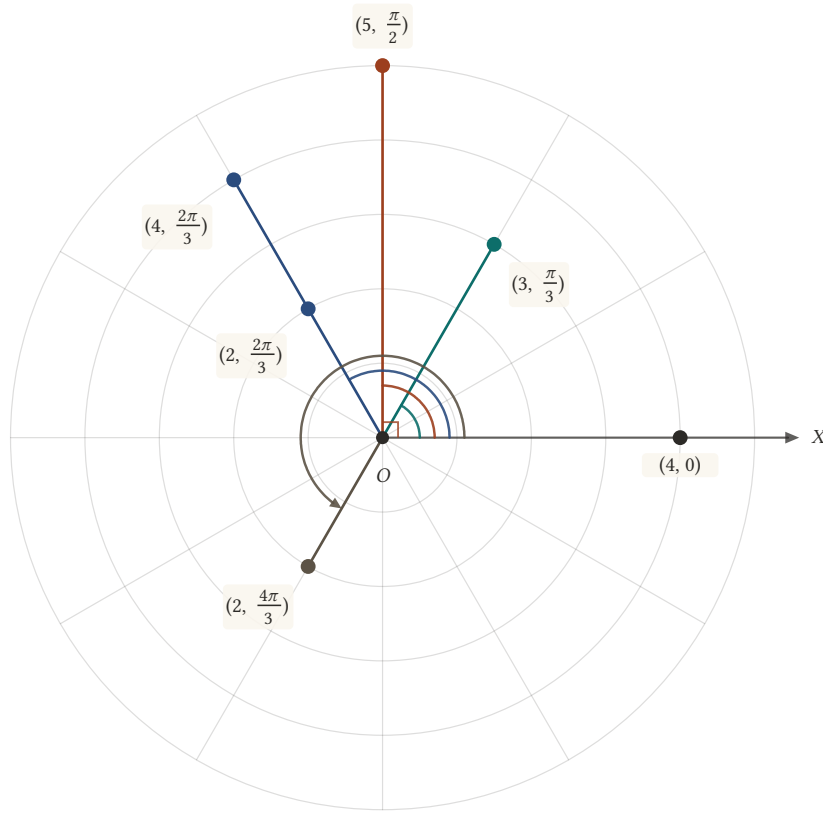
Şekil 5.6: Altı noktanın kutupsal düzlemdeki yeri. Soluk çemberler r = 1, \dots, 5 ; soluk ışınlar her \pi/6 'da bir. O 'daki renkli yaylar her noktanın kutupsal açısını gösterir.
