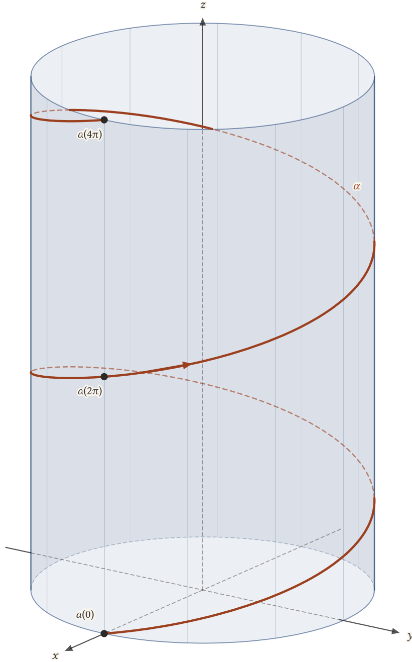
Şekil 23.2: Helis \alpha(t) = (2 \cos t, 2 \sin t, t/2) , t \in [0, 4\pi] , x^2 + y^2 = 4 silindirin üzerinde iki tur atarak yükselir; ok, t artarken hareket yönünü gösterir. \alpha(0) , \alpha(2\pi) ve \alpha(4\pi) aynı düşey doğru üzerindedir; eğrinin silindirin arkasında kalan kısımları kesiklidir.
