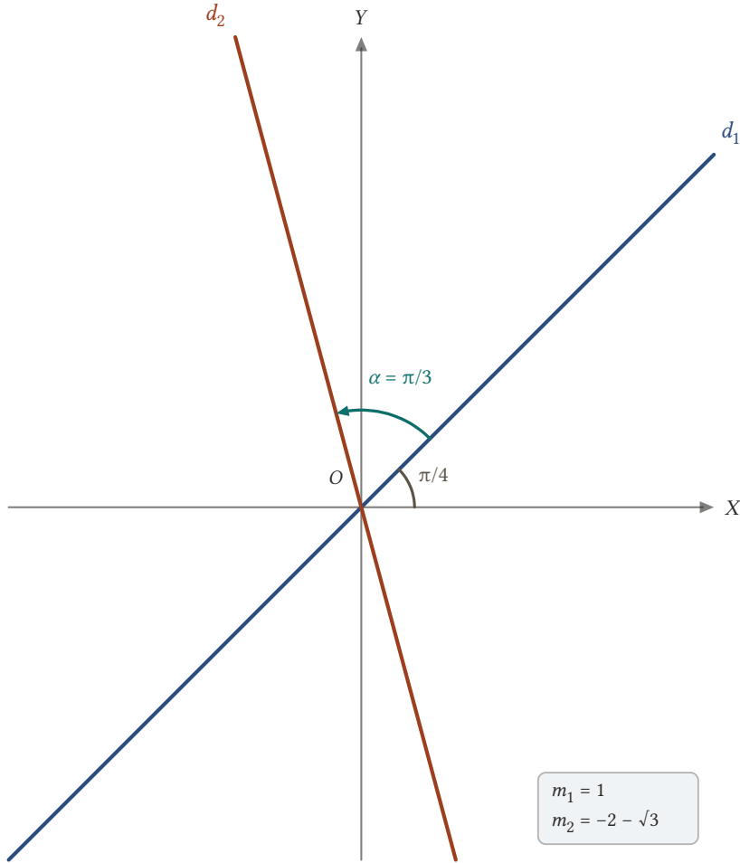
Şekil 2.30: Eğimi 1 olan d_1 doğrusu \pi/3 döndürülünce eğim açısı \pi/4 + \pi/3 = 7\pi/12 olan d_2 doğrusuna paralel olur; d_2 'nin eğimi -2 - \sqrt{3} 'tür.
