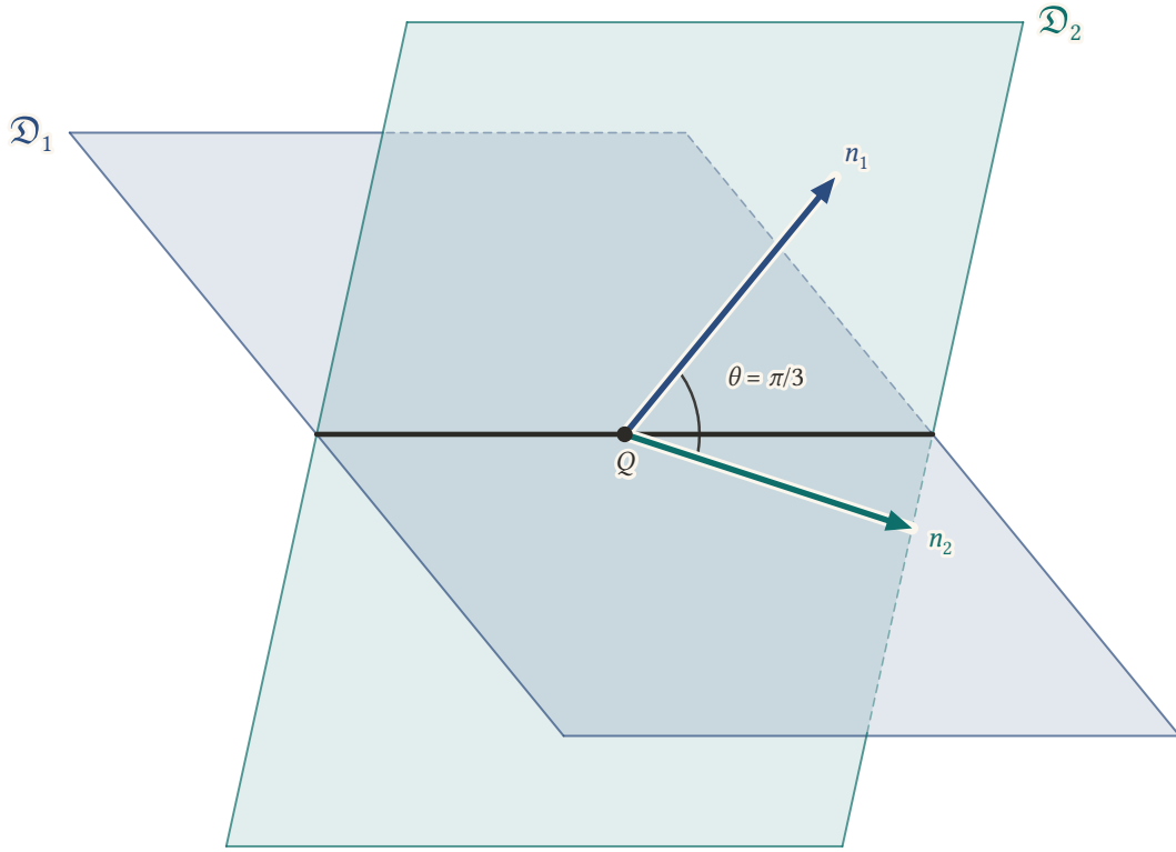
Şekil 14.12: İki düzlem arakesit doğrusu boyunca kesişir. Arakesit üzerindeki Q(6, 5, 0) noktasından çizilen n_1 = (2, -1, 1) ve n_2 = (1, 1, 2) normalleri arasındaki açı \theta = \pi/3 'tür; düzlemler arasındaki açı da budur.
