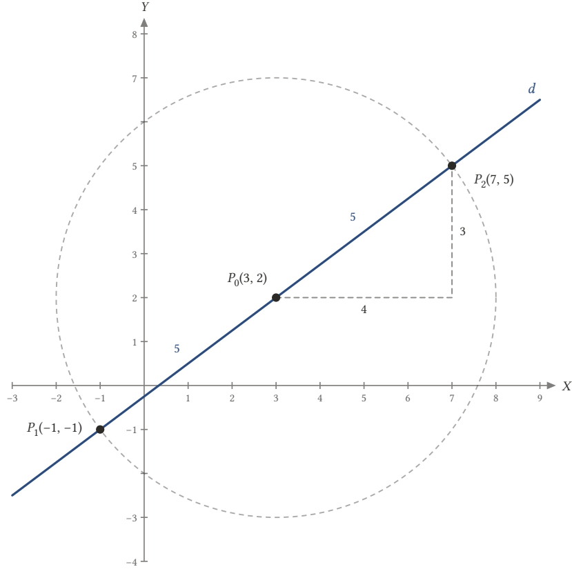
Şekil 3.7: P_0(3, 2) 'den geçen, eğimi 3/4 olan d doğrusu. Merkezi P_0 , yarıçapı 5 olan çember doğruyu aranan P_1(-1, -1) ve P_2(7, 5) noktalarında keser; yatay 4, dikey 3 birimlik adımın uzunluğu 5'tir.
