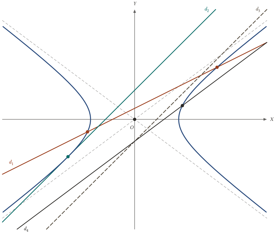
Şekil 19.13: Bir doğru hiperbolü iki noktada kesebilir ( d_1 ), ona teğet olabilir ( d_2 ), onunla hiç buluşmayabilir ( d_3 ); bir asimptota paralelse tek noktada keser ( d_4 ).
