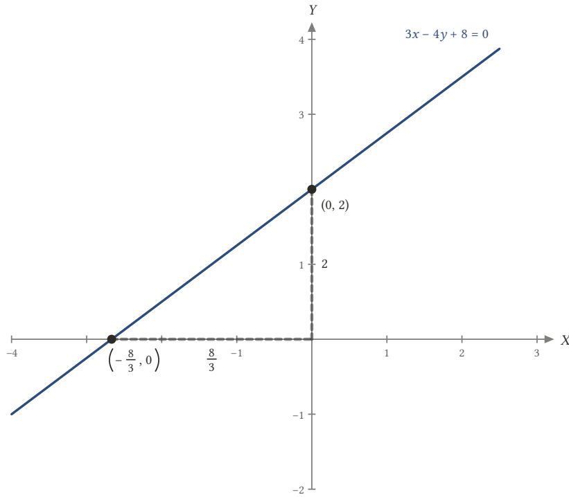
Şekil 3.6: 3x - 4y + 8 = 0 doğrusu eksenleri (-8/3, 0) ve (0, 2) 'de keser; eğim üçgeninin kenarları 8/3 ve 2 olduğundan eğim 2 : 8/3 = 3/4 'tür.
