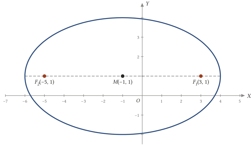
Şekil 18.25: F_1(3, 1) ve F_2(-5, 1) noktalarına uzaklıkları toplamı 10 olan noktalar: merkezi M(-1, 1) olan (x + 1)^2/25 + (y - 1)^2/9 = 1 elipsi.
