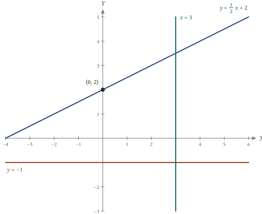
Şekil 3.2: Üç tür doğru: eğimi 1/2 olup Y -eksenini (0, 2) 'de kesen y = x/2 + 2 doğrusu, yatay y = -1 doğrusu ve düşey x = 3 doğrusu.
