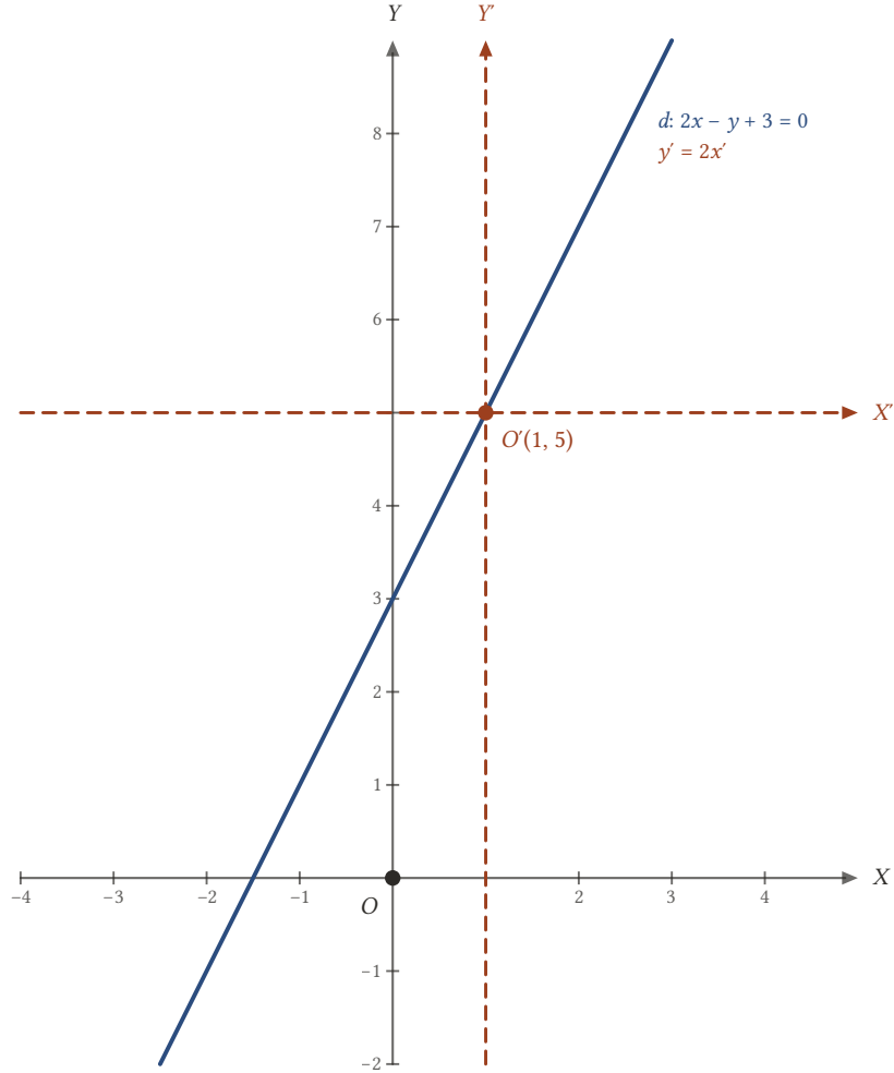
Şekil 16.13: d doğrusu yeni başlangıç noktası O'(1, 5) 'ten geçtiği için yeni denkleminde sabit terim yoktur.
