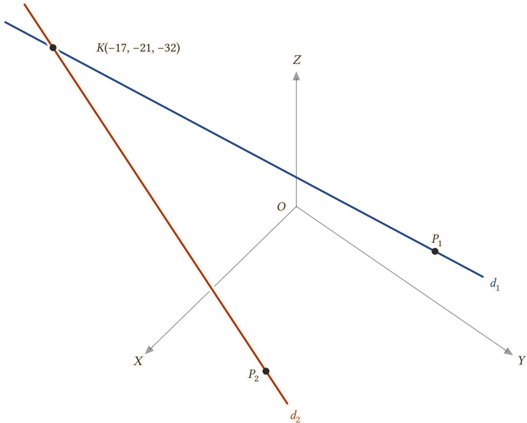
Şekil 11.7: d_1 ile d_2 K(-17, -21, -32) noktasında kesişir. Doğrultman vektörleri arasındaki açı küçük olduğundan doğrular kesişim noktasına doğru yavaşça yaklaşır; eksenler başlangıç noktası çevresinde, ölçek için çizilmiştir.
