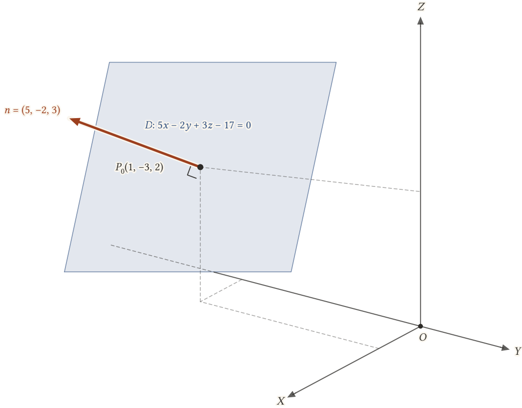
Şekil 12.2: 5x - 2y + 3z - 17 = 0 düzleminin P_0(1, -3, 2) çevresindeki parçası ve normali n = (5, -2, 3) (0,4 katı çizildi).
