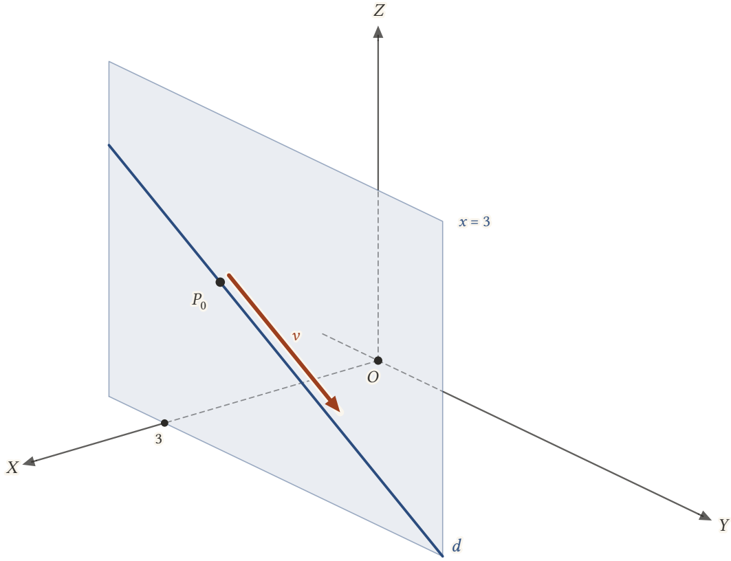
Şekil 10.13: Doğrultmanı v = (0, 2, -1) olan d doğrusu x = 3 düzleminde yatar. Bu düzlem YZ düzlemine paraleldir ve X eksenini 3'te dik keser.
