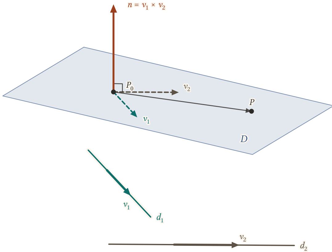
Şekil 12.5: Altta doğrultmanları v_1 ve v_2 olan aykırı d_1, d_2 doğruları; üstte P_0 'dan geçip ikisine de paralel olan düzlem. Kesikli oklar v_1 ve v_2 'nin P_0 'a taşınmış temsilcileridir; normal n = v_1 \times v_2 ikisine de diktir.
