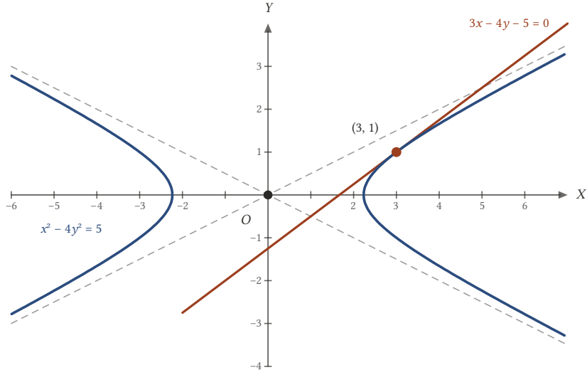
Şekil 19.23: 3x - 4y - 5 = 0 doğrusu hiperbole (3, 1) noktasında teğettir.
