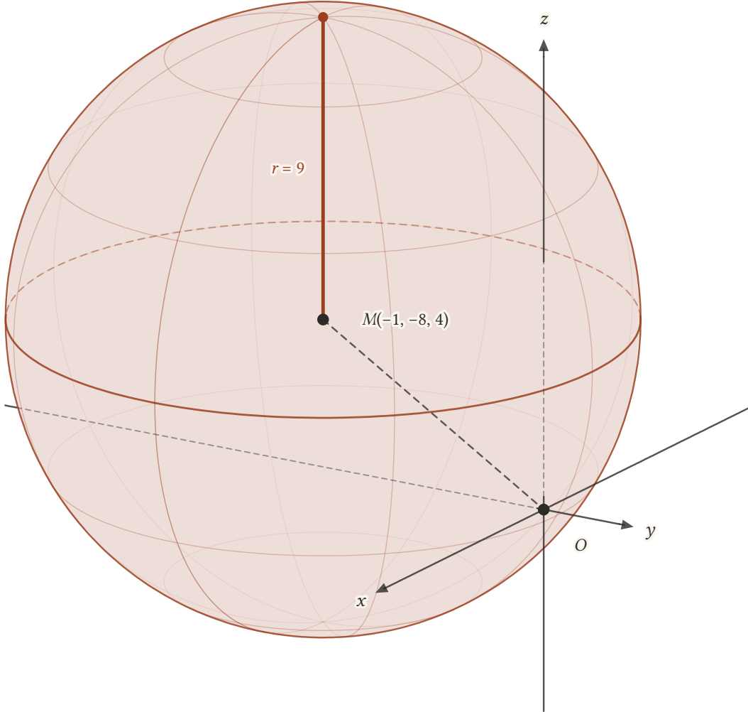
Şekil 23.1: Merkezi M(-1, -8, 4) ve yarıçapı 9 olan küre. Kırmızı doğru parçası yarıçaptır; |OM| = 9 olduğundan başlangıç noktası O küre üzerindedir (kesikli MO parçası). Eksenlerin kürenin arkasında ya da içinde kalan kısımları kesiklidir.
