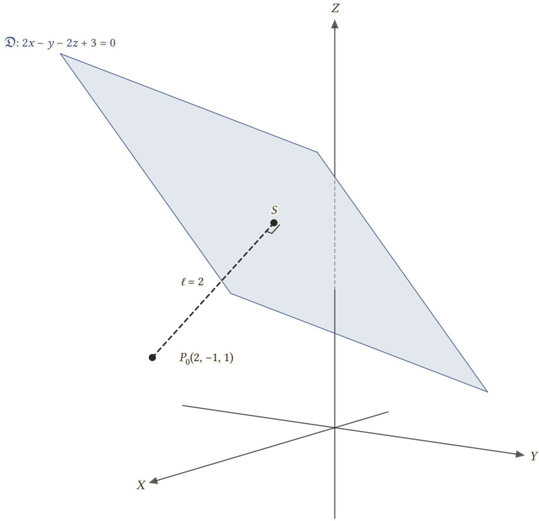
Şekil 14.10: P_0(2, -1, 1) 'dan düzleme inen dikmenin ayağı S(2/3, -1/3, 7/3) 'tür ve |P_0S| = 2 'dir. P_0 , normal n = (2, -1, -2) 'nin gösterdiği taraftadır.
