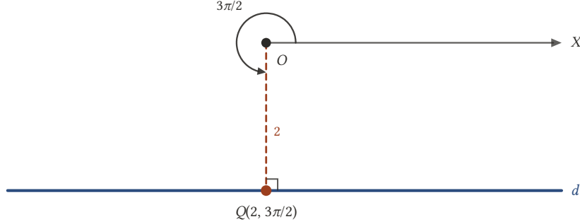
Şekil 5.16: r \sin \theta = -2 doğrusu: kutuptan inilen dikmenin ayağı Q(2, 3\pi/2) 'dir ve doğru kutupsal eksene paraleldir.
