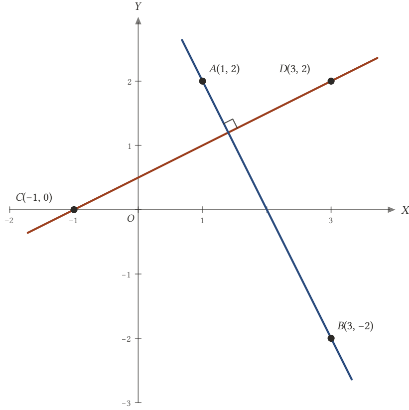
Şekil 2.22: k = -2 için AB doğrusu (eğim -2 ) CD doğrusuna (eğim 1/2 ) diktir; iki doğru (7/5, 6/5) noktasında kesişir.
