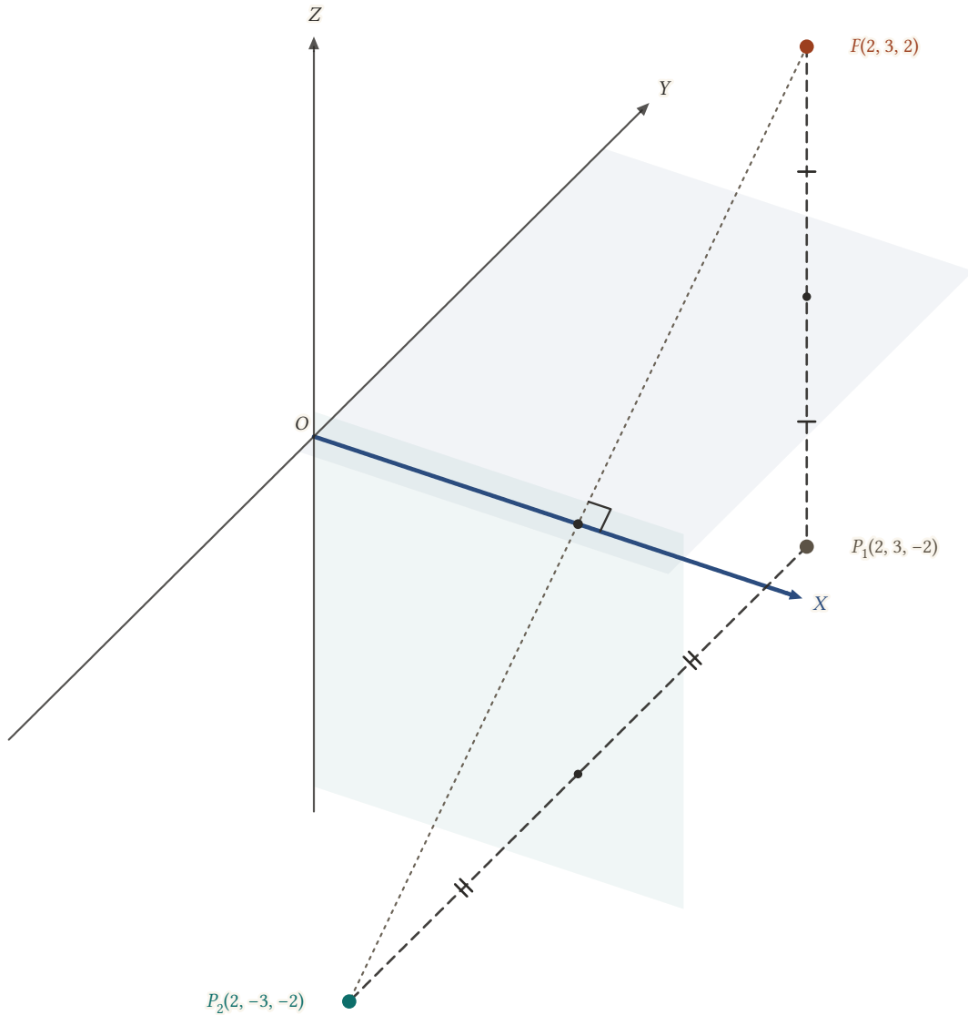
Şekil 15.14: P(2, 3, 2) noktasının XY -düzlemine göre simetriği P_1(2, 3, -2) , onun da XZ -düzlemine göre simetriği P_2(2, -3, -2) 'dir. Noktalı PP_2 parçası X -eksenini (2, 0, 0) 'da dik keser: P_2 , P 'nin X -eksenine göre simetriğidir.
