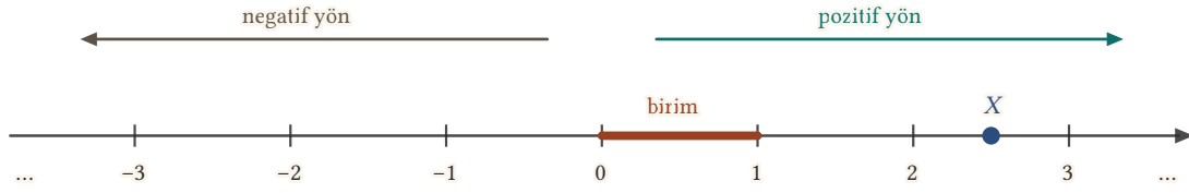
Şekil 1.1: Sayı doğrusu: 0 başlangıcı, 1 ise hem birimi hem de pozitif yönü belirler. 0'ın 2,5 birim sağındaki X noktasının sayısı 2,5'tir.
