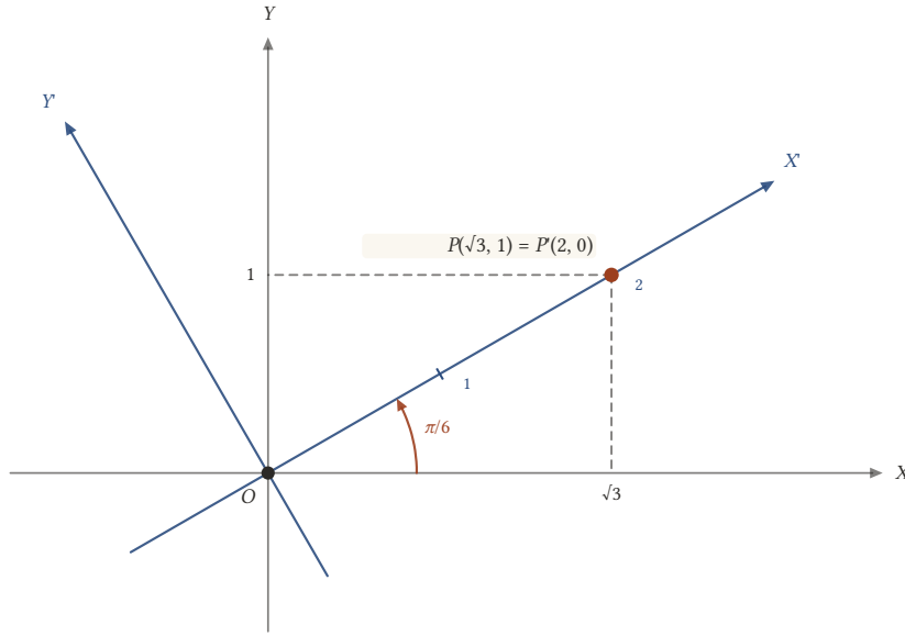
Şekil 17.10: Eksenler \pi/6 döndürülünce P(\sqrt{3}, 1) yeni X' -ekseni üzerine düşer ve yeni koordinatları (2, 0) olur.
