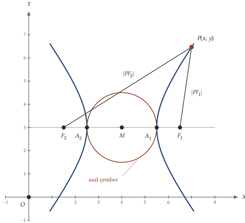
Şekil 19.1: Odakları F_1, F_2 olan hiperbol: sağ kolun her P noktasında |PF_2| - |PF_1| = 2a .
