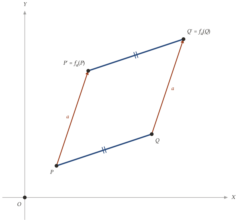
Şekil 16.5: PQ parçası a kadar ötelenince uzunluğu değişmez: |P'Q'| = |PQ| .
