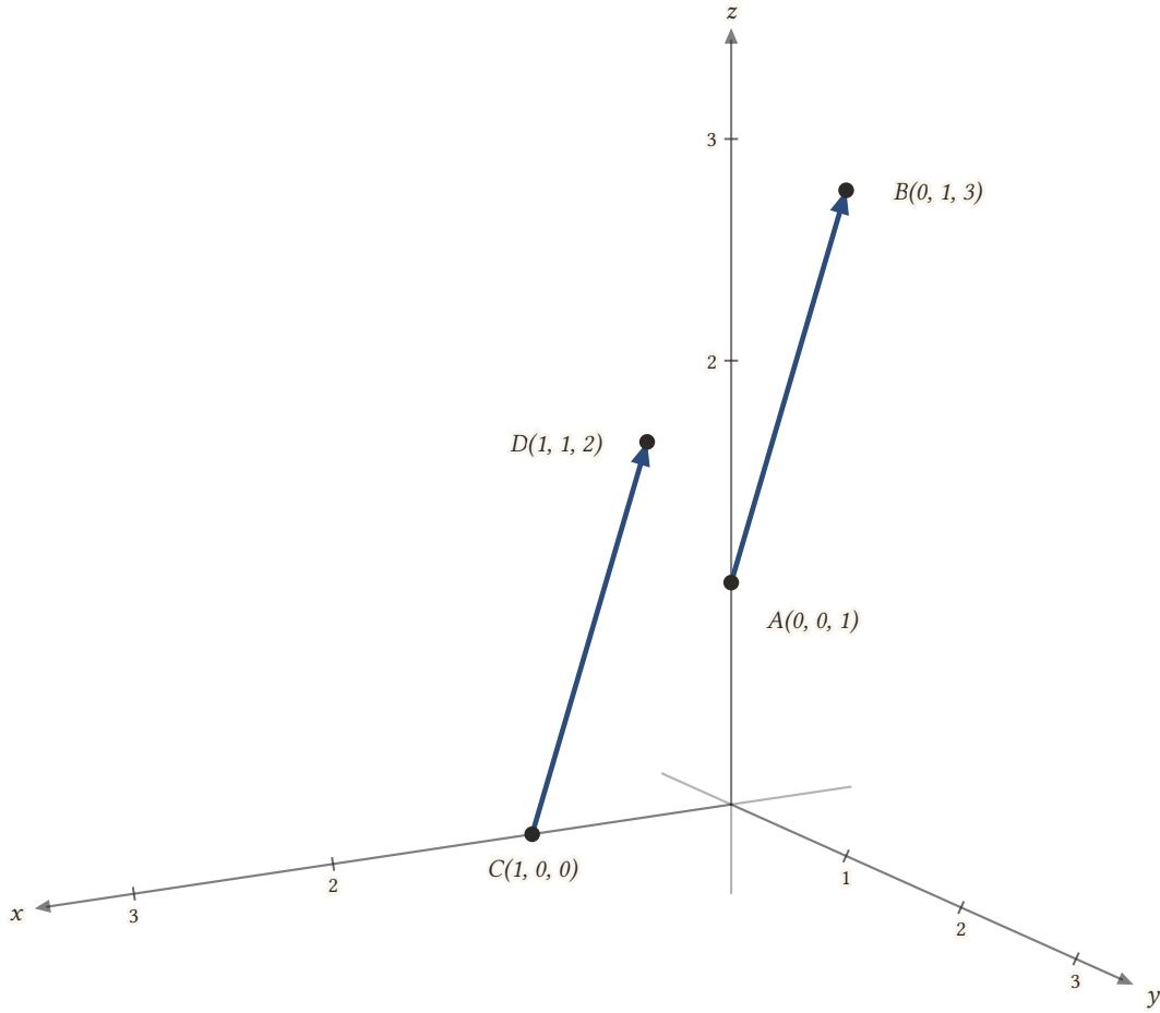
Şekil 7.5: AB ve CD yönlü doğru parçaları paralel, aynı yönlü ve eşit uzunluktadır; ikisi de (0, 1, 2) üçlüsüne gider.
