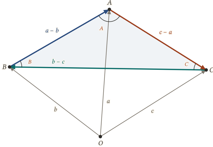
Şekil 9.15: A, B, C noktalarının yer vektörleri a, b, c ve kenar vektörleri a - b, b - c, c - a . Üçünün toplamı sıfırdır; köşelerdeki yaylar iç açıları gösterir.
