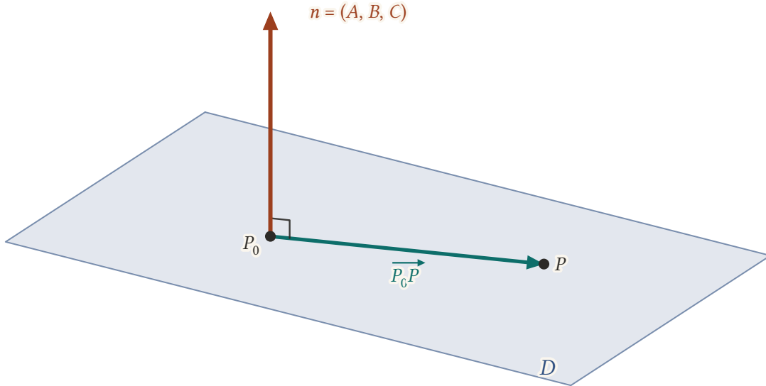
Şekil 12.1: Düzlemin bir P_0 noktası ve normali n . Düzlemin her P noktası için P_0P vektörü düzlemin içindedir ve n 'ye diktir.
