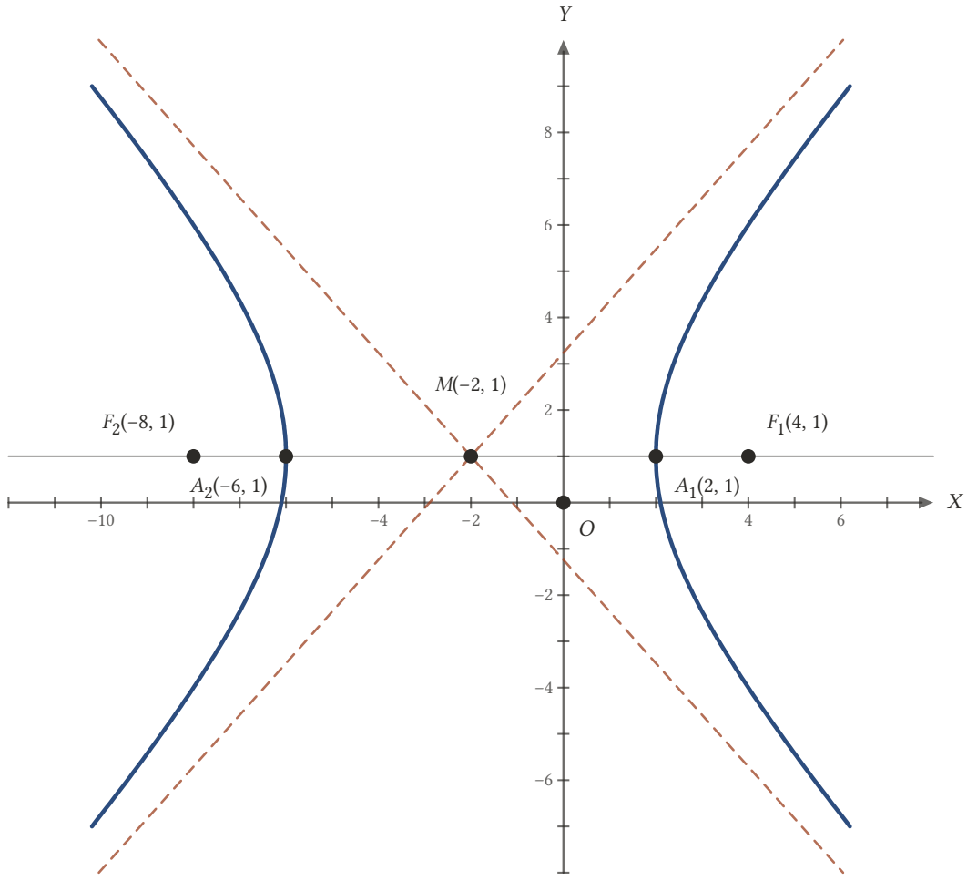
Şekil 19.19: Odakları ve köşeleri y = 1 doğrusu üzerinde olan, merkezi M(-2, 1) hiperbol.
