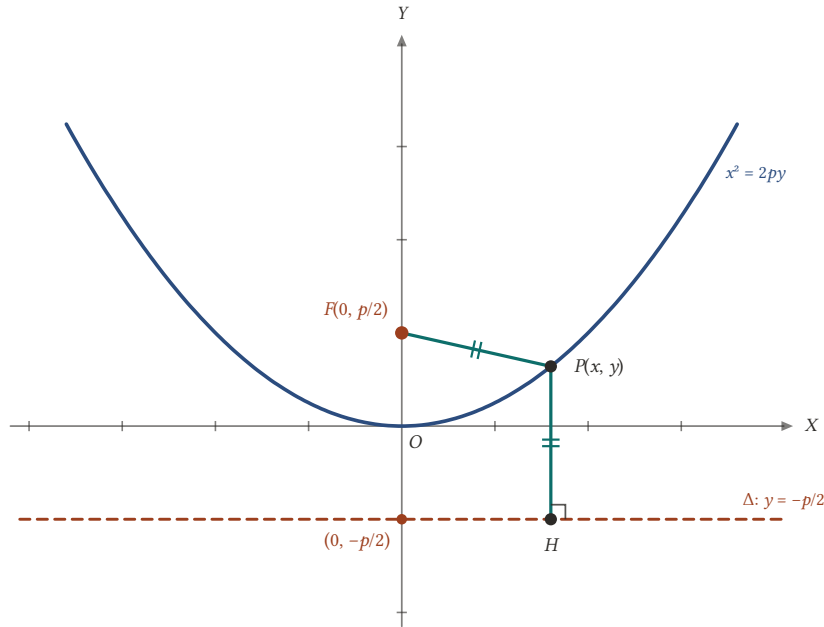
Şekil 20.2: Asal eksen Y-ekseni olan parabol: |PF| = |PH| koşulu x^2 = 2py denklemine denktir.
