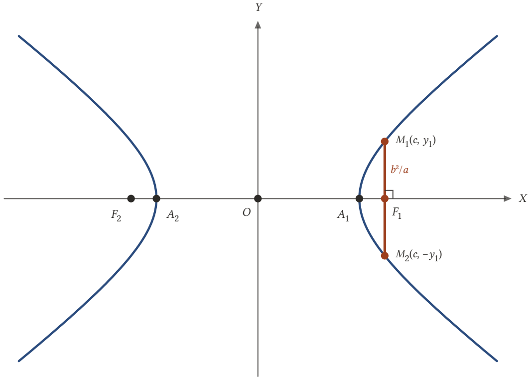
Şekil 19.9: Odaktan asal eksene dik kiriş: |M_1M_2| = 2b^2/a .
