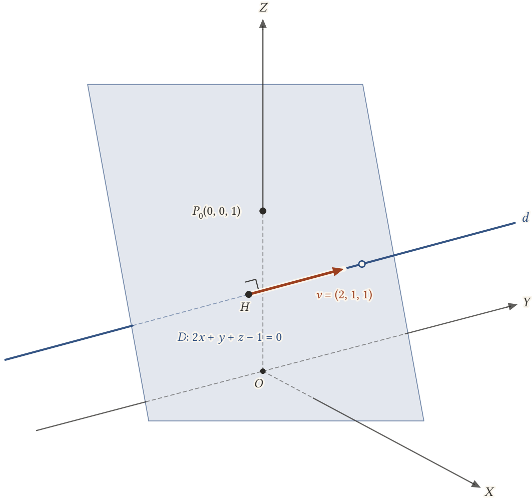
Şekil 12.4: 2x + y + z - 1 = 0 düzlemi ve ona dik d doğrusu. d düzlemi H(1/3, -1/3, 2/3) noktasında dik keser; boş daire d 'nin (1, 0, 1) noktasıdır.
