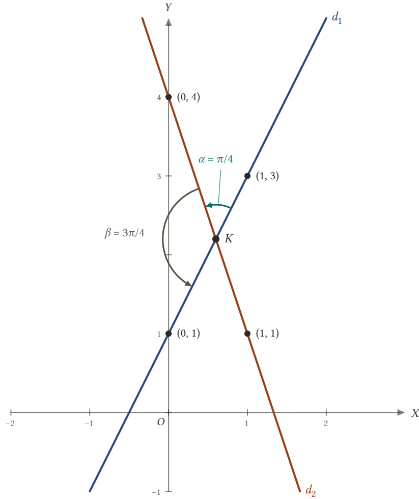
Şekil 2.25: d_1 (eğim 2) ve d_2 (eğim -3) doğruları K(3/5, 11/5) noktasında kesişir; d_1 'den d_2 'ye yönelmiş açı \alpha = \pi/4 , ters yöndeki açı \beta = 3\pi/4 'tür.
