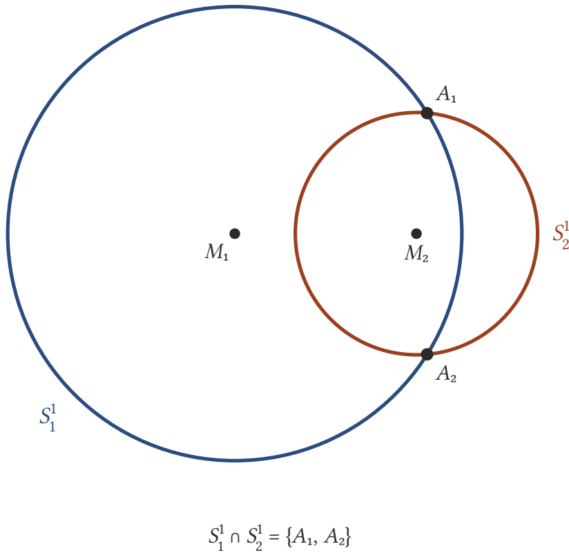
Şekil 4.14: |r_1 - r_2| < |M_1M_2| < r_1 + r_2 : çemberler iki noktada kesişir. Burada küçük çemberin merkezi büyük çemberin içindedir.
