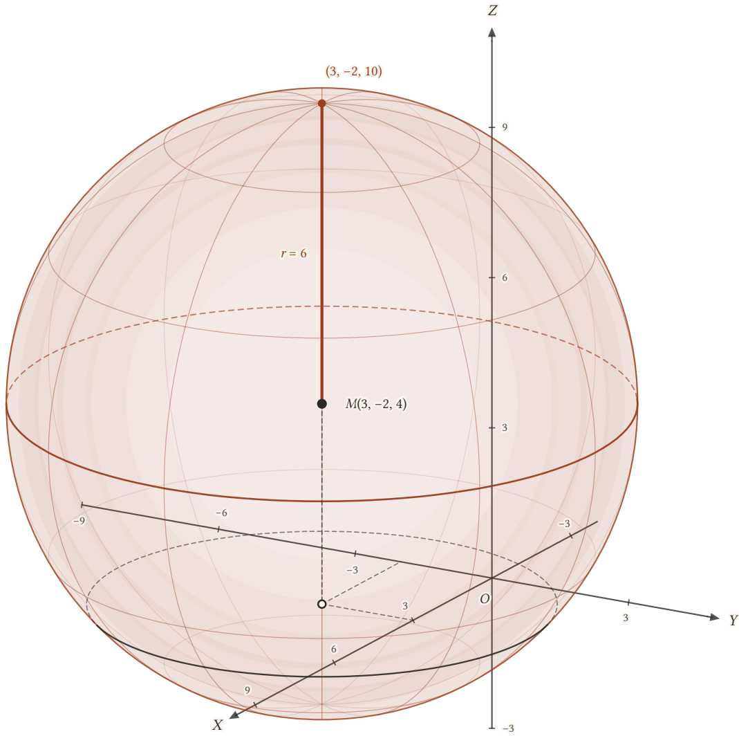
Şekil 6.15: Merkezi M(3, -2, 4) ve yarıçapı 6 olan küre. Kürenin en üst noktası (3, -2, 10) 'dur; küre z = -2 'ye kadar indiğinden XY -düzlemini, merkezi (3, -2, 0) ve yarıçapı \sqrt{20} olan çember boyunca keser (siyah çember).
