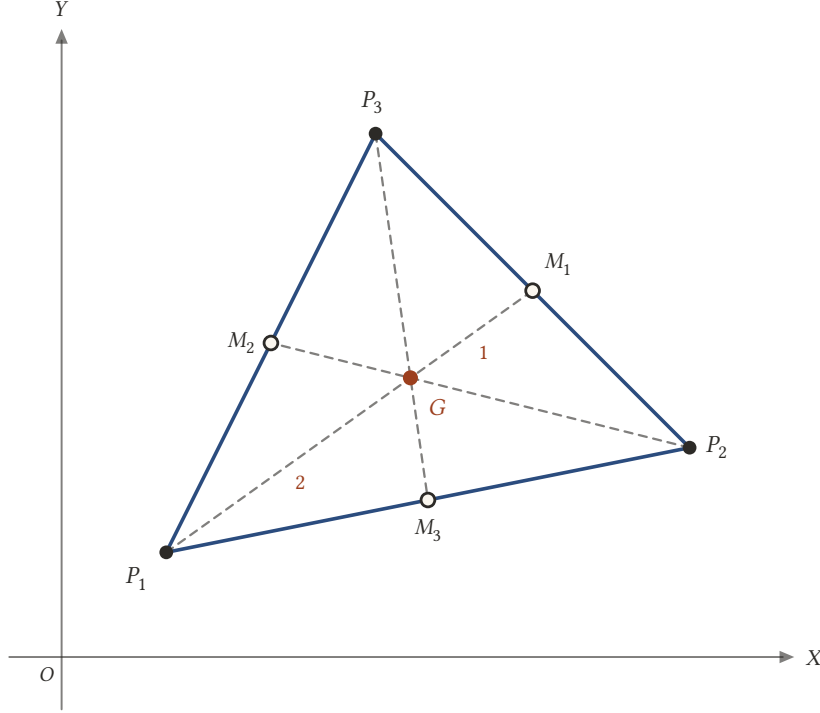
Şekil 2.4: Üç kenarortay P_1M_1, P_2M_2, P_3M_3 aynı G noktasından geçer; G her kenarortayı köşeden itibaren 2 : 1 oranında böler.
