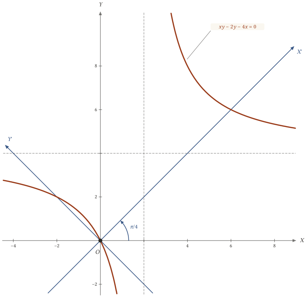
Şekil 21.12: Eksenler \pi/4 döndürülünce karma terim kaybolur: x'^2 - y'^2 - 6\sqrt{2}x' + 2\sqrt{2}y' = 0 .
