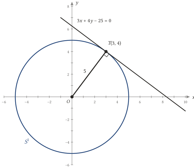
Şekil 4.12: 3x + 4y - 25 = 0 doğrusu x^2 + y^2 = 25 çemberine T(3, 4) noktasında teğettir; OT yarıçapı teğete diktir. ■
