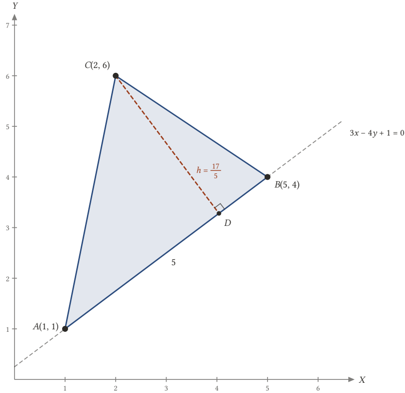
Şekil 3.23: A(1, 1) , B(5, 4) , C(2, 6) üçgeninde C 'den AB 'ye inen yükseklik h = 17/5 'tir; taban |AB| = 5 olduğundan alan 17/2 'dir.
