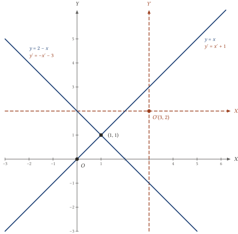
Şekil 16.18: Eğri y = x ve y = 2 - x doğrularından oluşur; yeni sistemde bu doğrular y' = x' + 1 ve y' = -x' - 3 olur.
