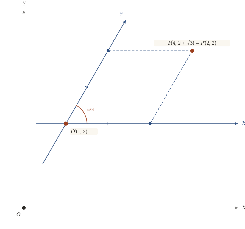
Şekil 17.19: Başlangıcı O'(1, 2) ve eksen açısı \pi/3 olan eğik sistemde P(4, 2 + \sqrt{3}) noktasının paralel koordinatları (2, 2) 'dir.
