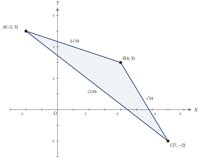
Şekil 1.12: Kenarları 2\sqrt{10} , \sqrt{34} ve \sqrt{130} olan üçgen.
