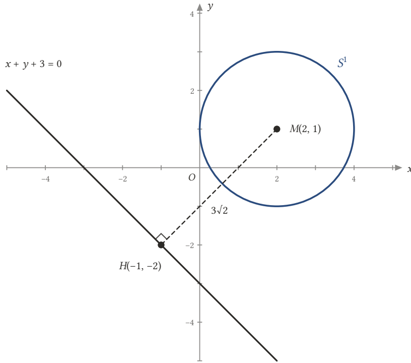
Şekil 4.13: Merkez M(2, 1) 'in x + y + 3 = 0 doğrusuna uzaklığı 3\sqrt{2} \approx 4,24 'tür; bu, yarıçap 2'den büyük olduğundan doğru çemberle buluşmaz.
