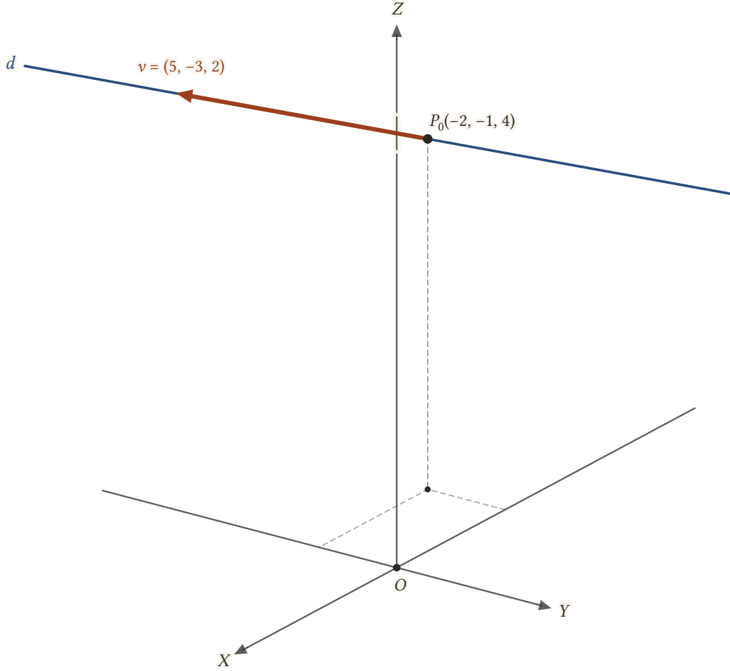
Şekil 12.14: P_0(-2, -1, 4) noktasından geçen ve v = (5, -3, 2) vektörüne paralel olan d doğrusu; kesikli çizgi P_0 'ın XY -düzlemine dikmesidir.
