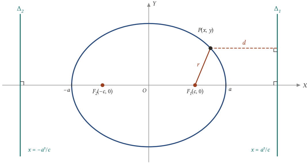
Şekil 18.22: x^2/25 + y^2/16 = 1 elipsinin doğrultmanları x = \pm 25/3 . Elipsin her P noktası için r/d = |PF_1|/d(P, \Delta_1) = e = 3/5 .
