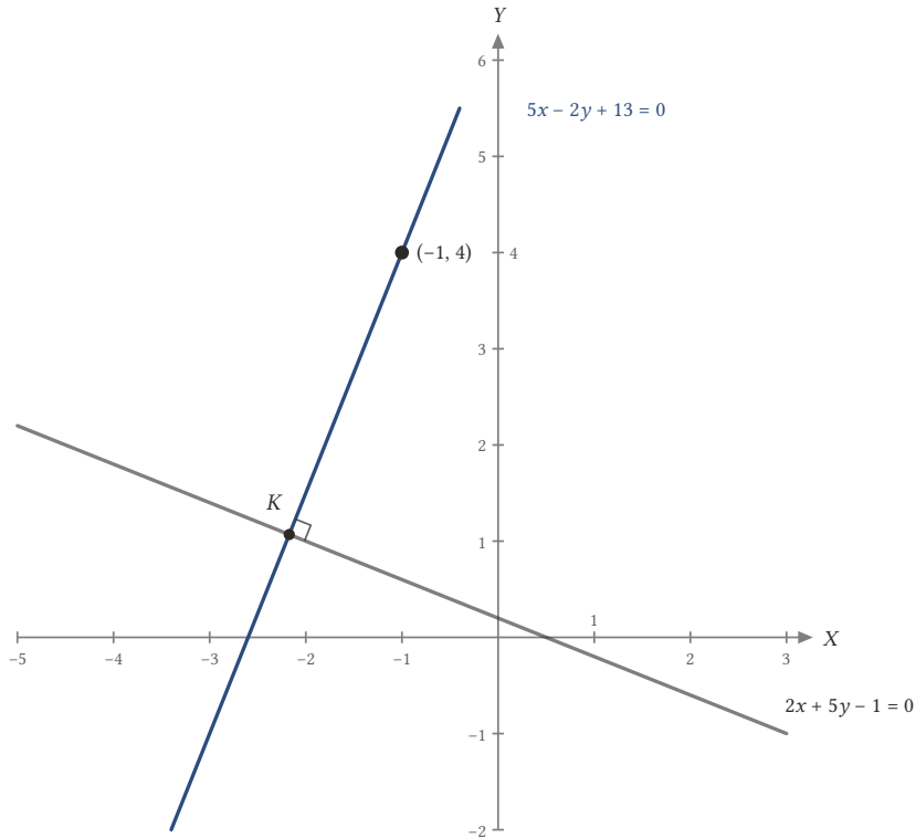
Şekil 3.20: (-1, 4) 'ten geçen ve 2x + 5y - 1 = 0 'a dik olan doğru 5x - 2y + 13 = 0 'dır; iki doğru K(-\frac{63}{29}, \frac{31}{29}) noktasında dik kesişir.
