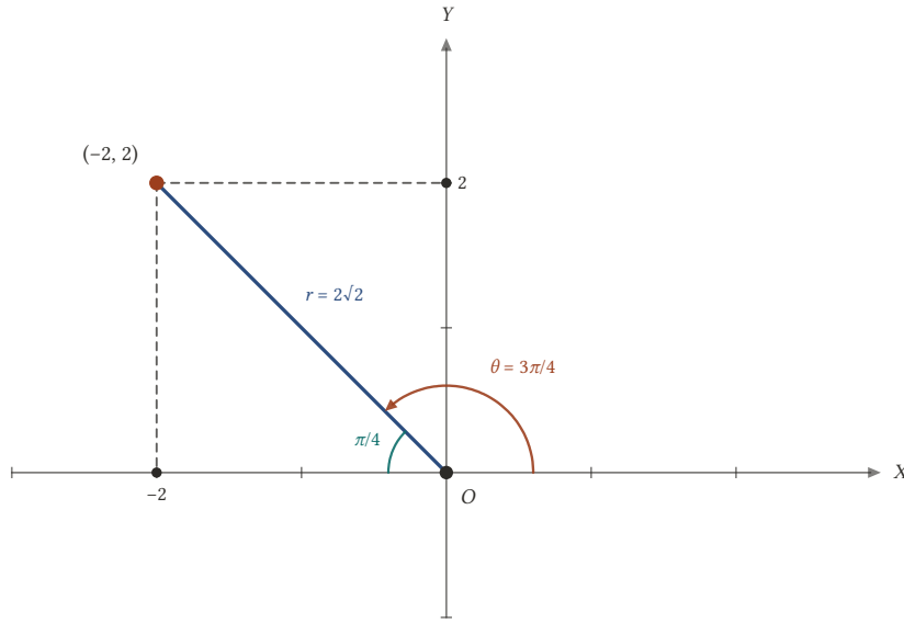
Şekil 5.8: (-2, 2) noktası ikinci bölgededir: r = 2\sqrt{2} ve \theta = 3\pi/4 . OP negatif X yönüyle \pi/4 açı yapar.
