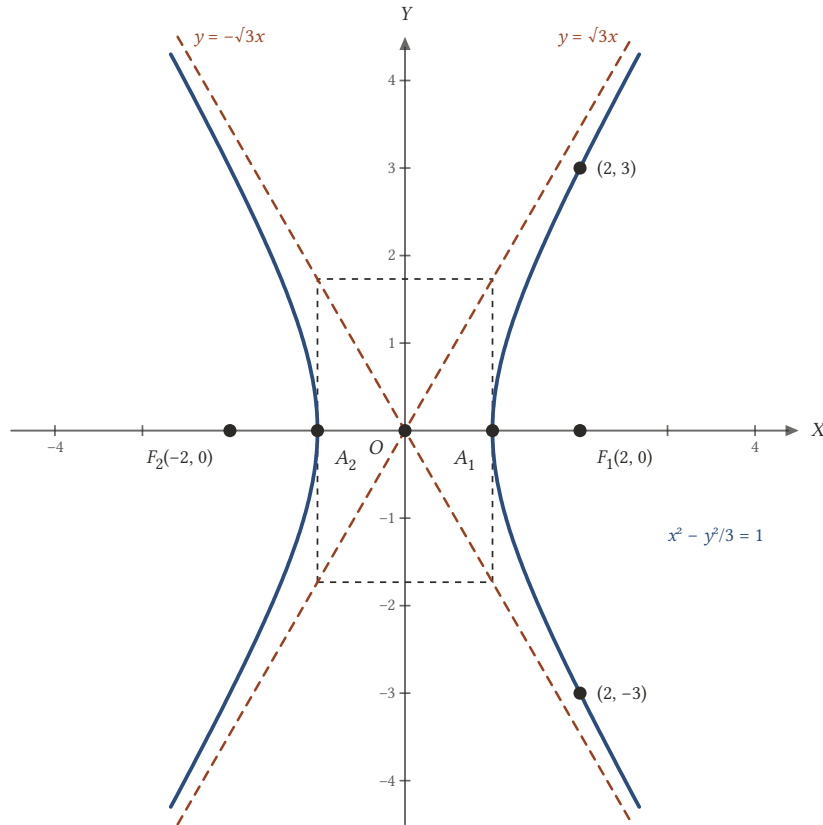
Şekil 19.5: x^2 - y^2/3 = 1 hiperbolü: köşeler (\pm 1, 0) , odaklar (\pm 2, 0) , asimptotlar y = \pm \sqrt{3}x .
