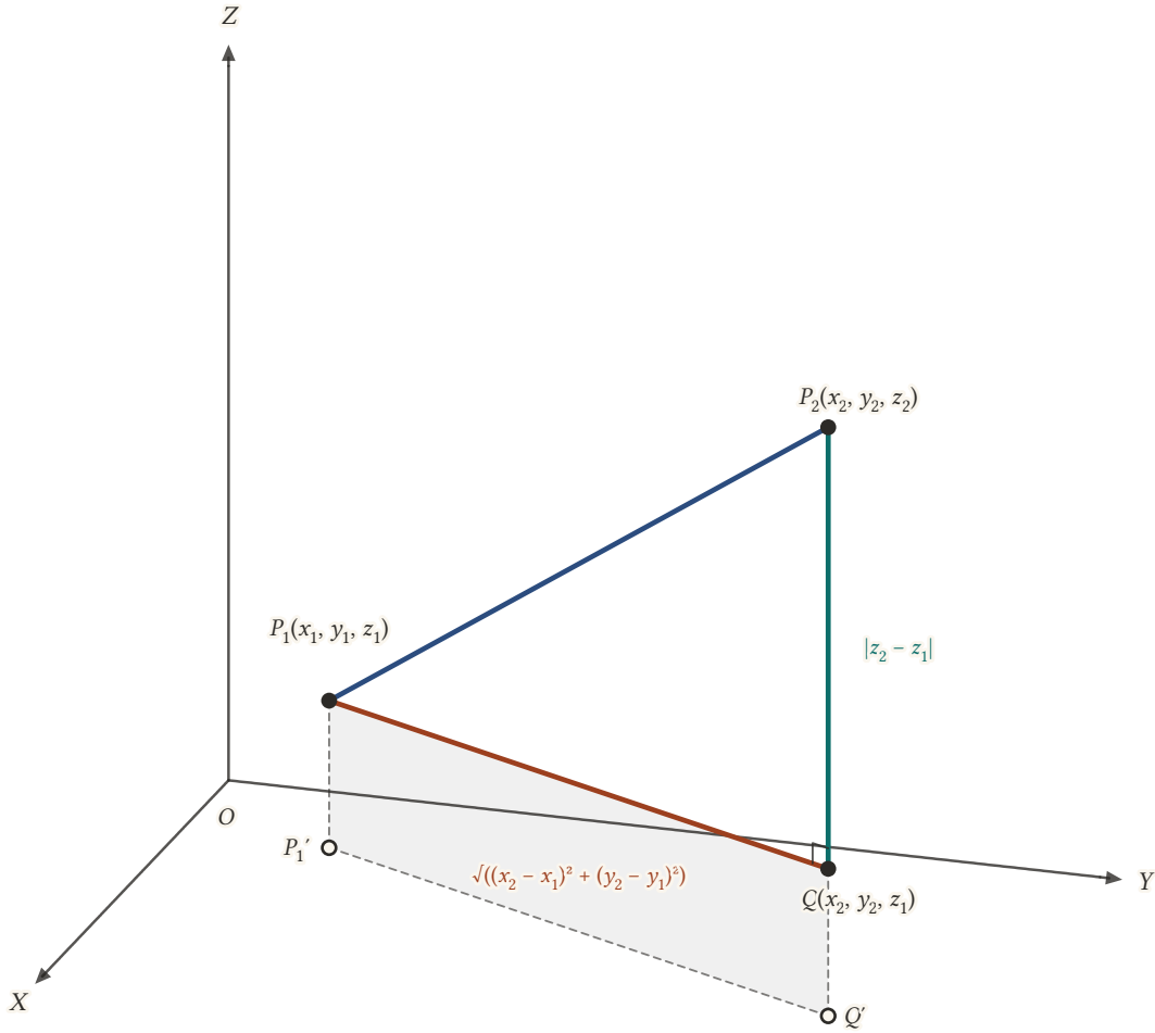
Şekil 6.11: Uzaklık formülünün ispatı: Q yardımcı noktasıyla P_1QP_2 üçgeni Q'da diktir. Yatay kenar P_1Q (turuncu), XY-düzlemindeki P_1'Q' ile aynı uzunlukta; düşey kenar QP_2 (yeşil) kotların farkıdır; hipotenüs P_1P_2 (mavi) aranan uzaklıktır.
