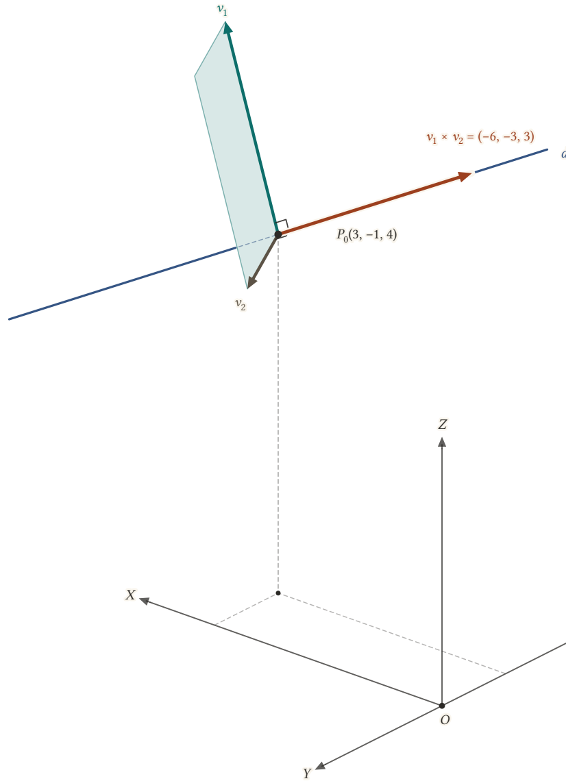
Şekil 12.19: v_1 ve v_2 'nin gerdiği paralelkenar (0,6 katı) ve P_0(3, -1, 4) 'ten geçip ikisine de dik olan d doğrusu; doğrultmanı v_1 \times v_2 = (-6, -3, 3) (0,3 katı çizildi).
