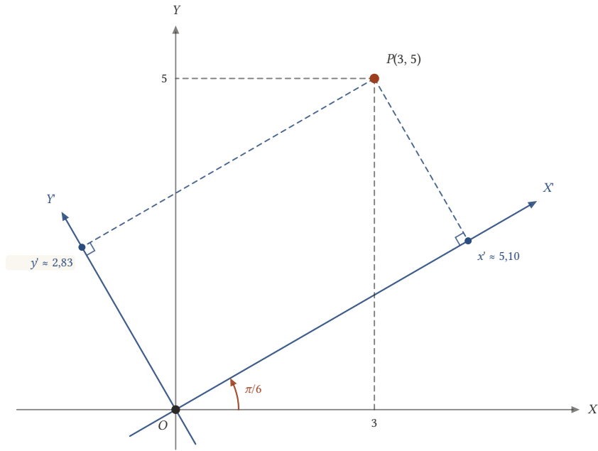
Şekil 17.21: Eksenler \pi/6 döndürülünce P(3, 5) 'in yeni koordinatları ((3\sqrt{3} + 5)/2, (5\sqrt{3} - 3)/2) \approx (5,10; 2,83) olur.
