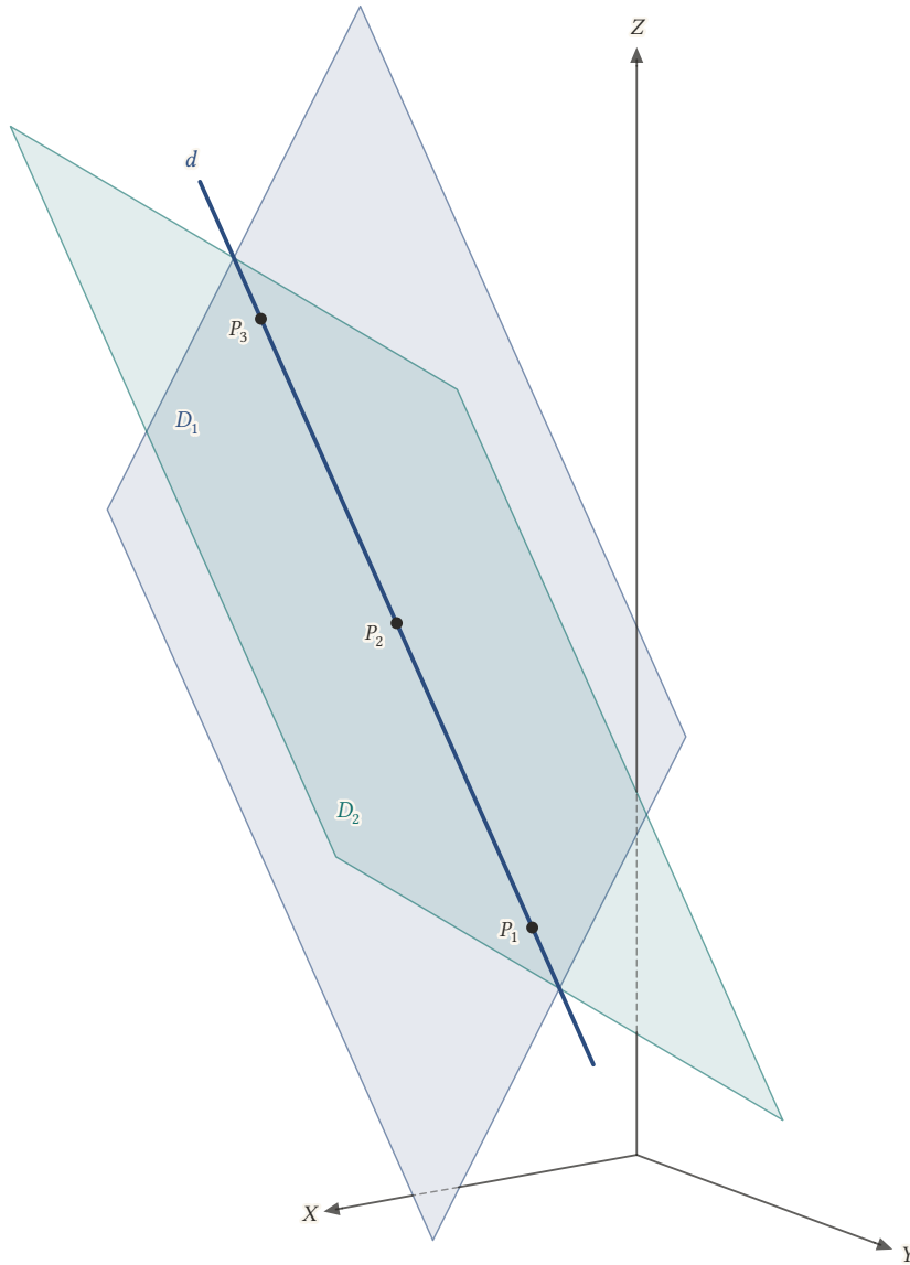
Şekil 12.11: Doğrudaş P_1, P_2, P_3 noktalarından geçen d doğrusu ve d 'yi içeren iki düzlem: x - 2y - 1 = 0 ve 3x - 2z + 1 = 0 . Üç nokta tek bir düzlem belirtmez.
