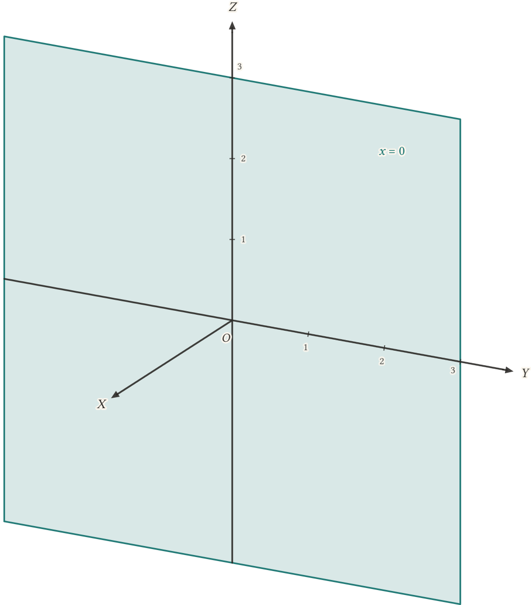
Şekil 6.6: x = 0 denklemini sağlayan noktalar YZ -koordinat düzlemini oluşturur; düzlemin -3 \leq y \leq 3 , -3 \leq z \leq 3 karesiyle sınırlı parçası çizilmiştir. Pozitif X -ekseni düzlemden okuyucuya doğru çıkar.
