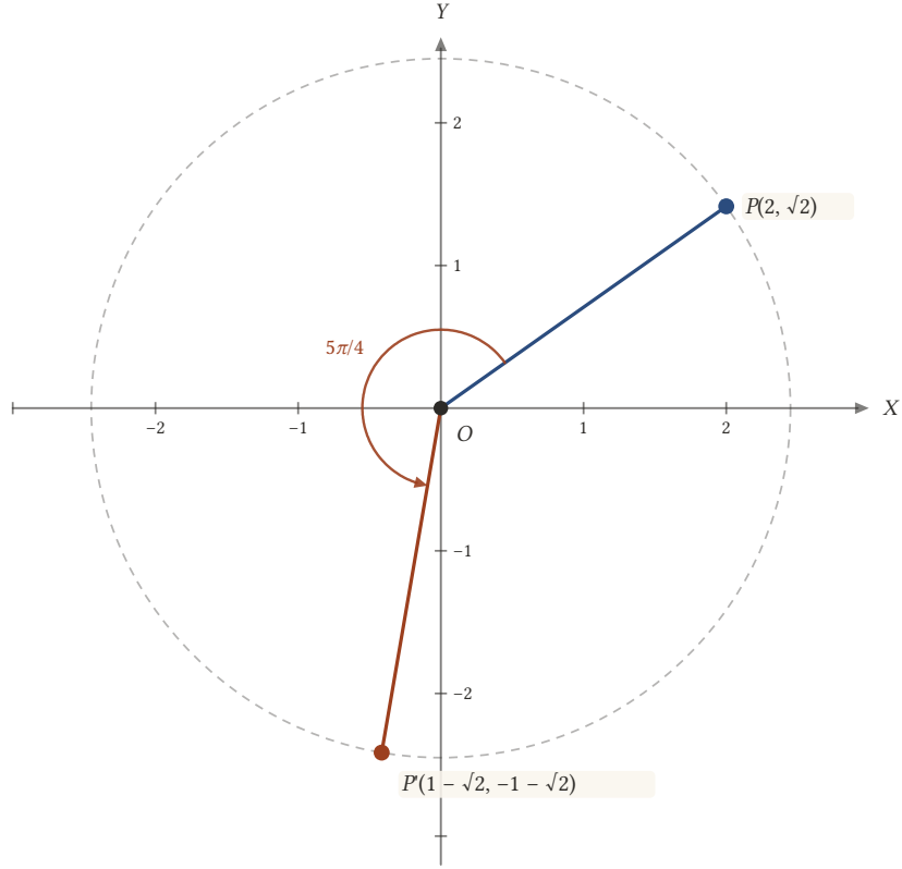
Şekil 17.3: P(2, \sqrt{2}) noktası O etrafında 5\pi/4 döndürülünce P(1 - \sqrt{2}, -1 - \sqrt{2}) noktasına gider; iki nokta da yarıçapı \sqrt{6} olan çember üzerindedir.
