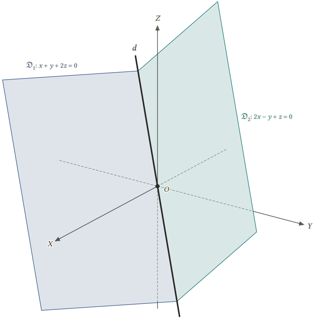
Şekil 13.5: Orijinden geçen iki düzlemin arakesiti de orijinden geçer: d , O 'dan geçen ve (-1, -1, 1) doğrultusundaki doğrudur. Her düzlemin yalnız d 'nin bir yanında kalan yarısı çizilmiştir.
