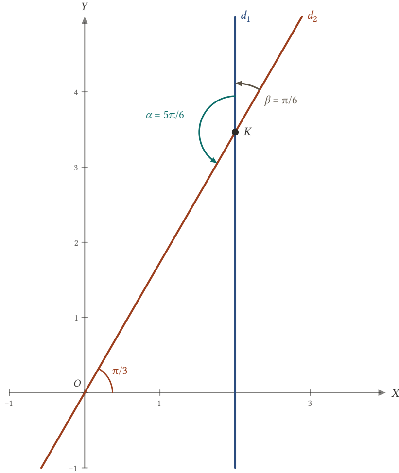
Şekil 2.26: Düşey d_1 ile eğimi \sqrt{3} olan d_2 doğrusu: d_1 'den d_2 'ye yönelmiş açı \alpha = 5\pi/6 , d_2 'den d_1 'e yönelmiş açı \beta = \pi/6 'dır.
