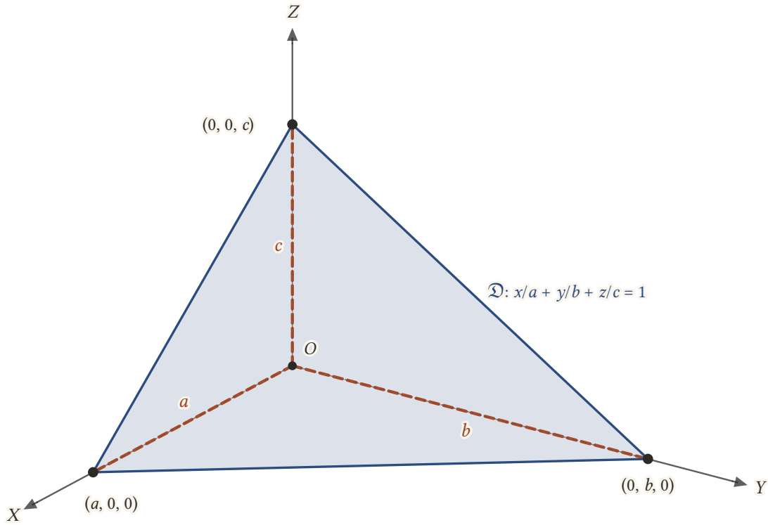
Şekil 13.9: Düzlem eksenleri (a, 0, 0) , (0, b, 0) , (0, 0, c) noktalarında keser; kalın parçalar eksen parçalarıdır. Bu üç noktanın üçgeni düzlemin bir parçasıdır.
