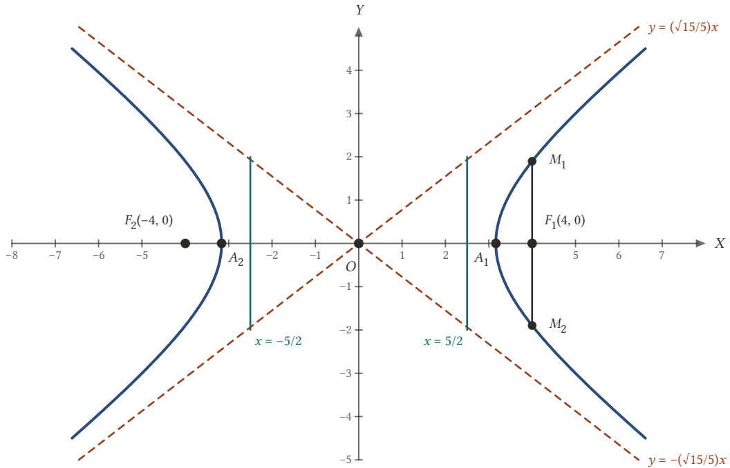
Şekil 19.21: x^2/10 - y^2/6 = 1 : odaklar (\pm 4, 0) , asimptotlar y = \pm(\sqrt{15}/5)x , doğrultmanlar x = \pm 5/2 .
