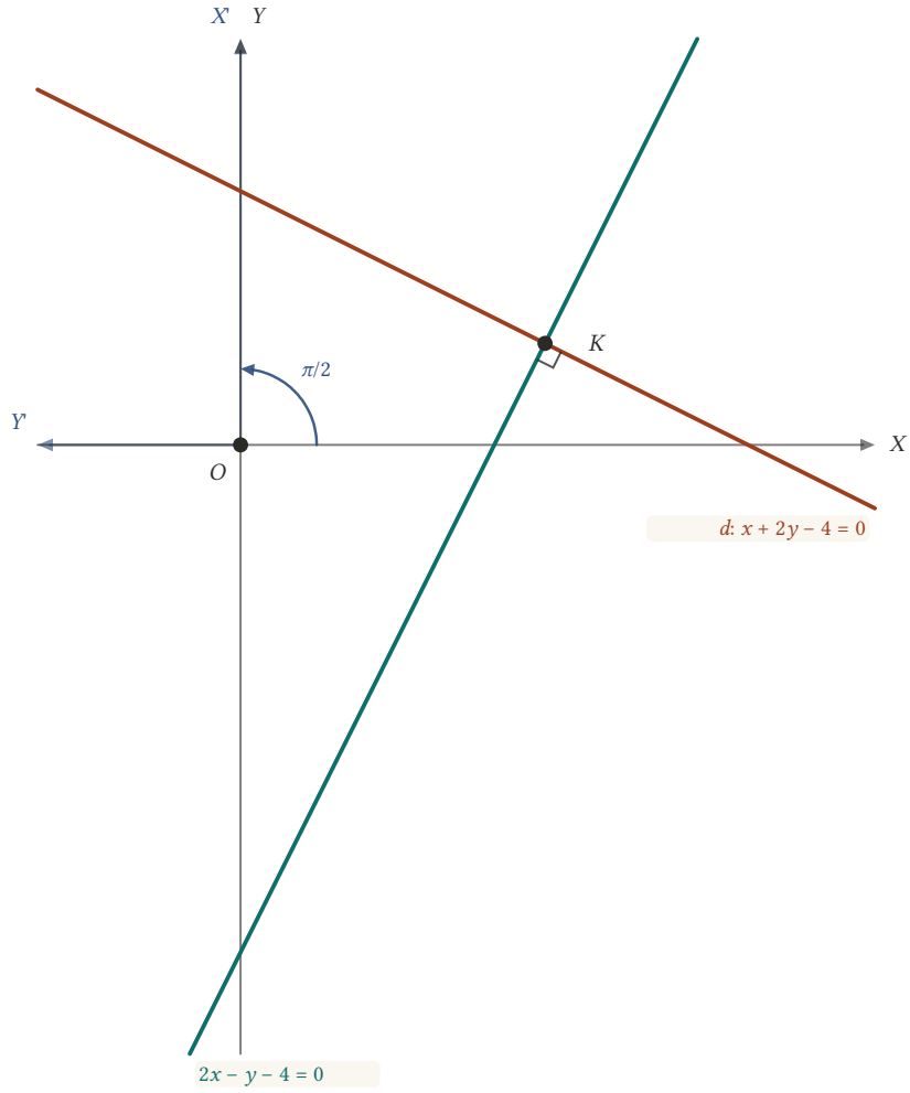
Şekil 17.13: Eksenler \pi/2 döndürülünce d 'nin yeni denklemi 2x' - y' - 4 = 0 olur; bu denklem XY 'de okunduğunda d 'ye dik bir doğru belirtir. İki doğru K(12/5, 4/5) 'te dik kesişir.
