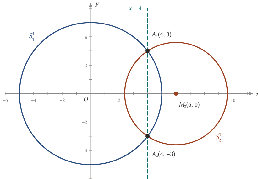
Şekil 4.21: x^2 + y^2 = 25 ile (x - 6)^2 + y^2 = 13 çemberleri A_1(4, 3) ve A_2(4, -3) noktalarında kesişir; ortak kiriş x = 4 doğrusu üzerindedir.
