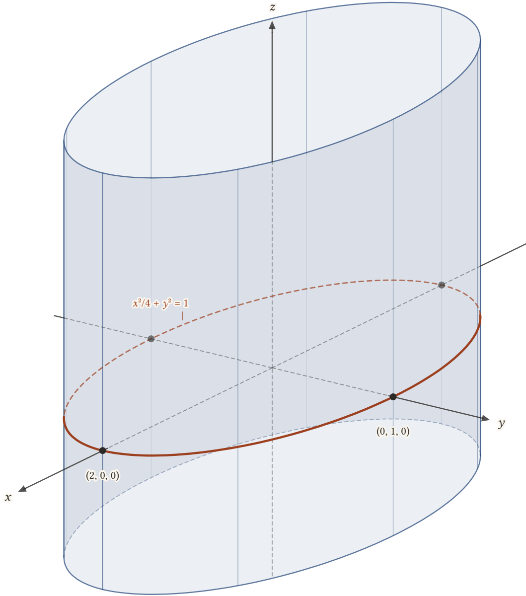
Şekil 23.6: Eliptik silindir x^2/4 + y^2 = 1 ( -1 \leq z \leq 2 parçası). Her z = k düzlemi yüzeyi aynı elips boyunca keser; kırmızı elips xy -düzlemindeki dayanak eğrisidir ve eksenleri (\pm 2, 0, 0) ile (0, \pm 1, 0) noktalarında keser.
