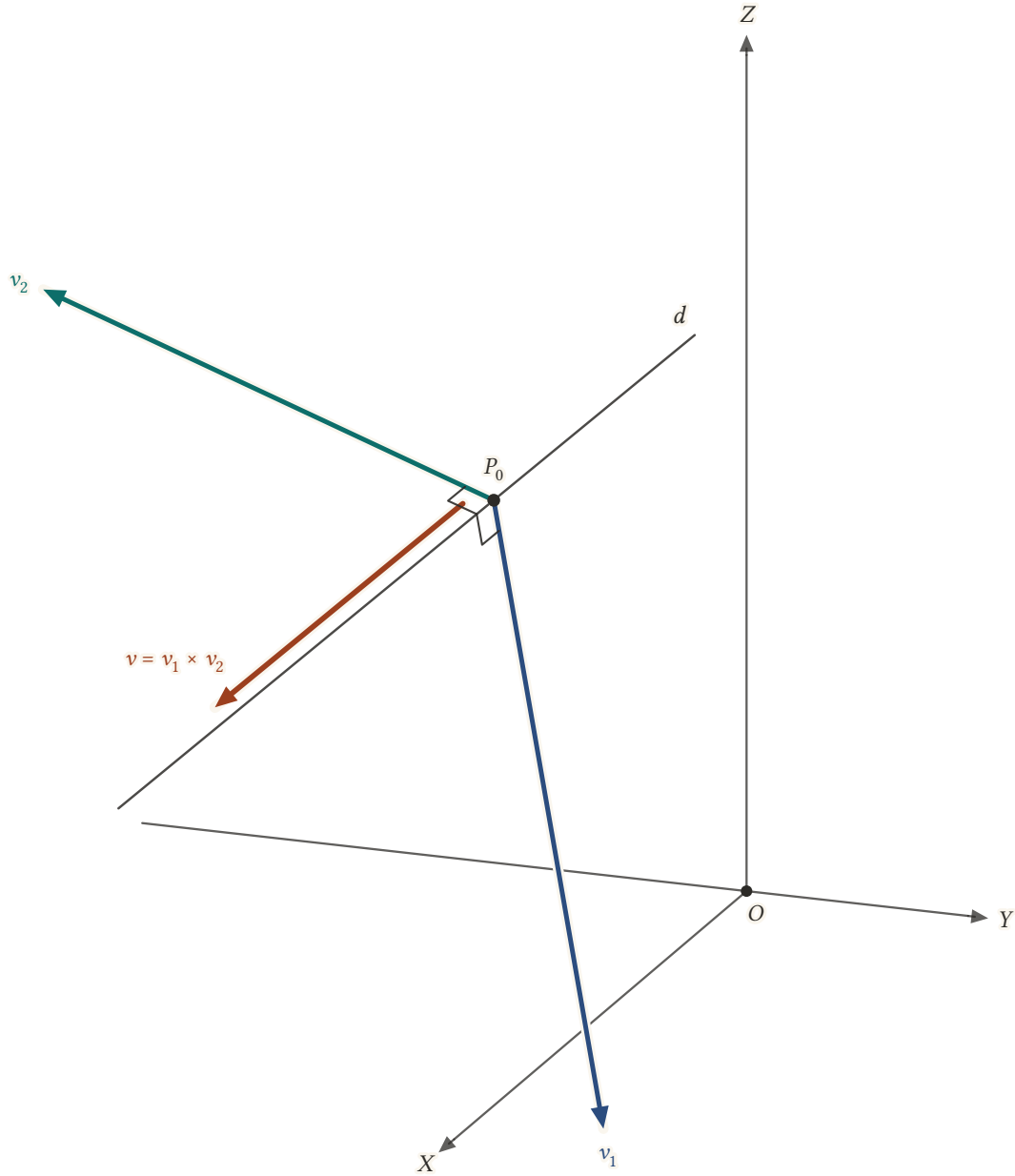
Şekil 10.12: P_0 = (3, -1, 4) noktasından çizilen v_1 , v_2 ve bunların vektörel çarpımı v = (-8, -14, -13) ; v kısaltılarak, yalnız yönü gösterilecek biçimde çizildi. v her ikisine de diktir ve aranan d doğrusunun doğrultmanıdır.
