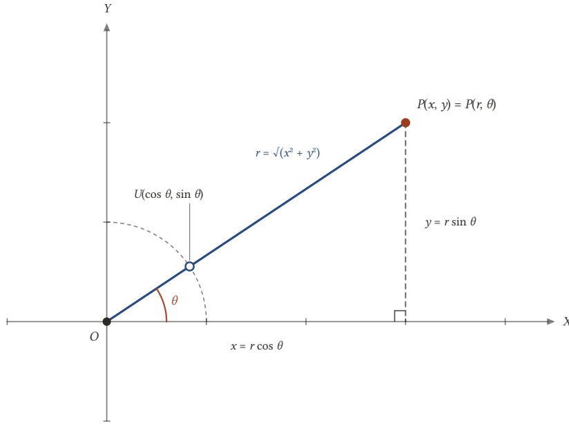
Şekil 5.7: Dik ve kutupsal koordinatlar: OHP dik üçgeninden x = r \cos \theta , y = r \sin \theta . Birim çember üzerindeki U noktası (\cos \theta, \sin \theta) 'dir.
