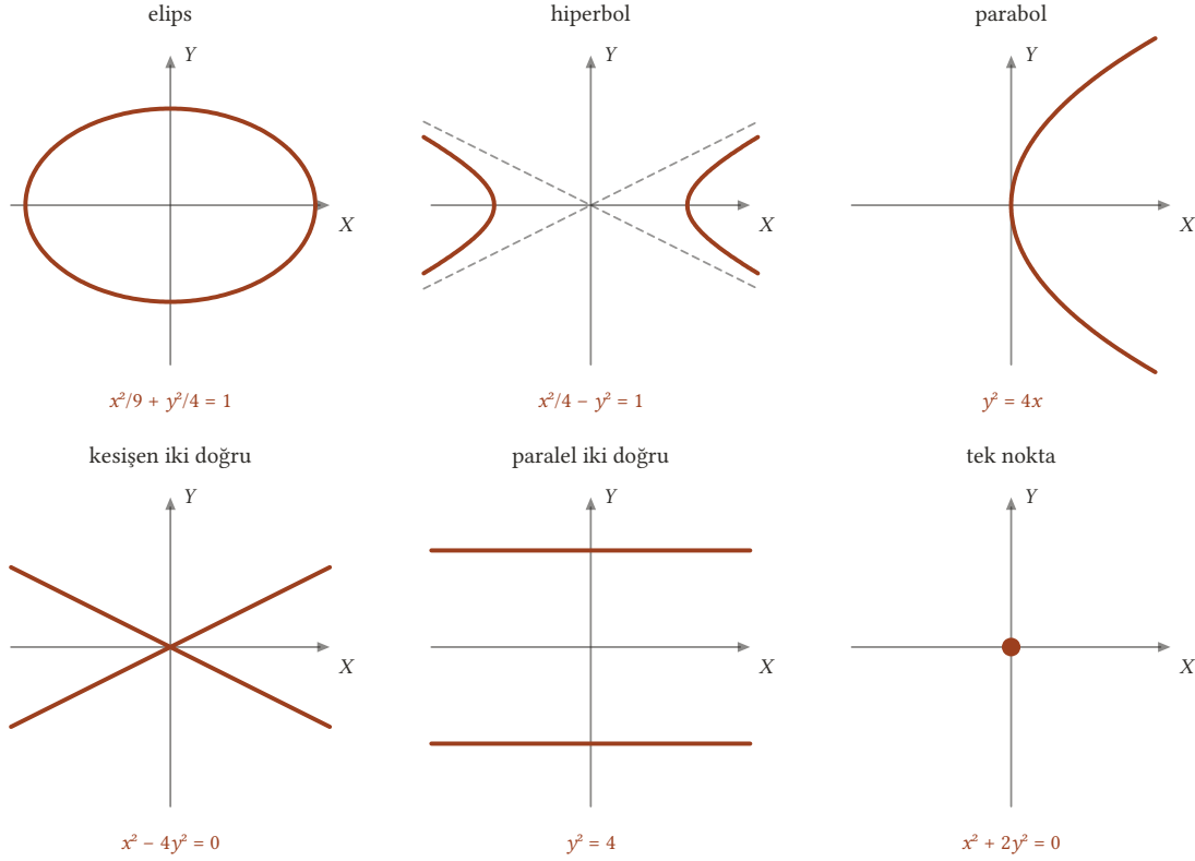
Şekil 21.4: İkinci dereceden denklemlerin belirttiği kümeler: üç konik ve üç yozlaşmış durum (sanal elips ile sanal iki doğru boş kümedir, çizilmez).
