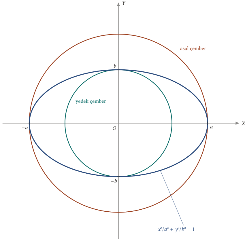
Şekil 18.20: Elipsin asal çemberi x^2 + y^2 = a^2 , yedek çemberi x^2 + y^2 = b^2 ; elips ikisinin arasında kalır.
