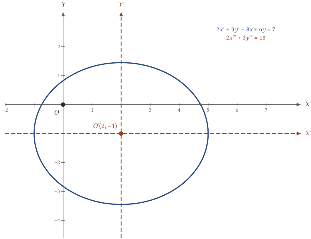
Şekil 16.17: Eksenler (2, -1) kadar ötelenince eğrinin denklemi 2x'^2 + 3y'^2 = 18 olur; eğri O' etrafında simetriktr.
