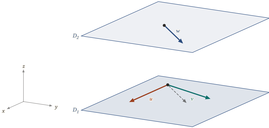
Şekil 7.17: Düzlemdeş vektörler: u ile v alt düzlemde, w ona paralel üst düzlemde çizilmiştir. w 'nın ortak başlangıç noktasından çizilen kopyası (kesikli) da alt düzlemde kalır.
