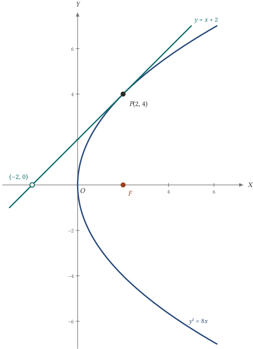
Şekil 20.9: y^2 = 8x parabolünün P(2, 4) noktasındaki teğeti y = x + 2 .
