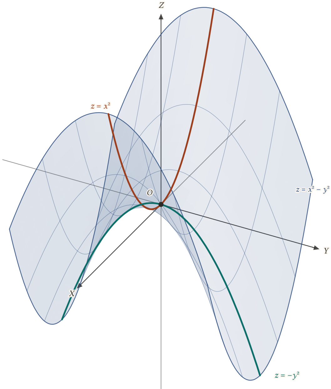
Şekil 22.10: z = x^2 - y^2 eyer yüzeyinin -1,5 \leq x, y \leq 1,5 parçası. XZ -düzlemiyle kesiti yukarı açılan z = x^2 parabolü, YZ -düzlemiyle kesiti aşağı açılan z = -y^2 parabolüdür; ikisi O eyer noktasında buluşur.
