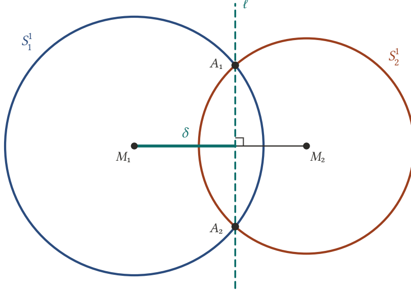
Şekil 4.20: İki çemberin denklemlerinin farkı, merkezleri birleştiren doğruya dik bir \ell doğrusudur; ortak noktalar S_1^1 ile \ell 'nin ortak noktalarıdır. Sayılarını M_1 'in \ell 'ye uzaklığı \delta belirler.
