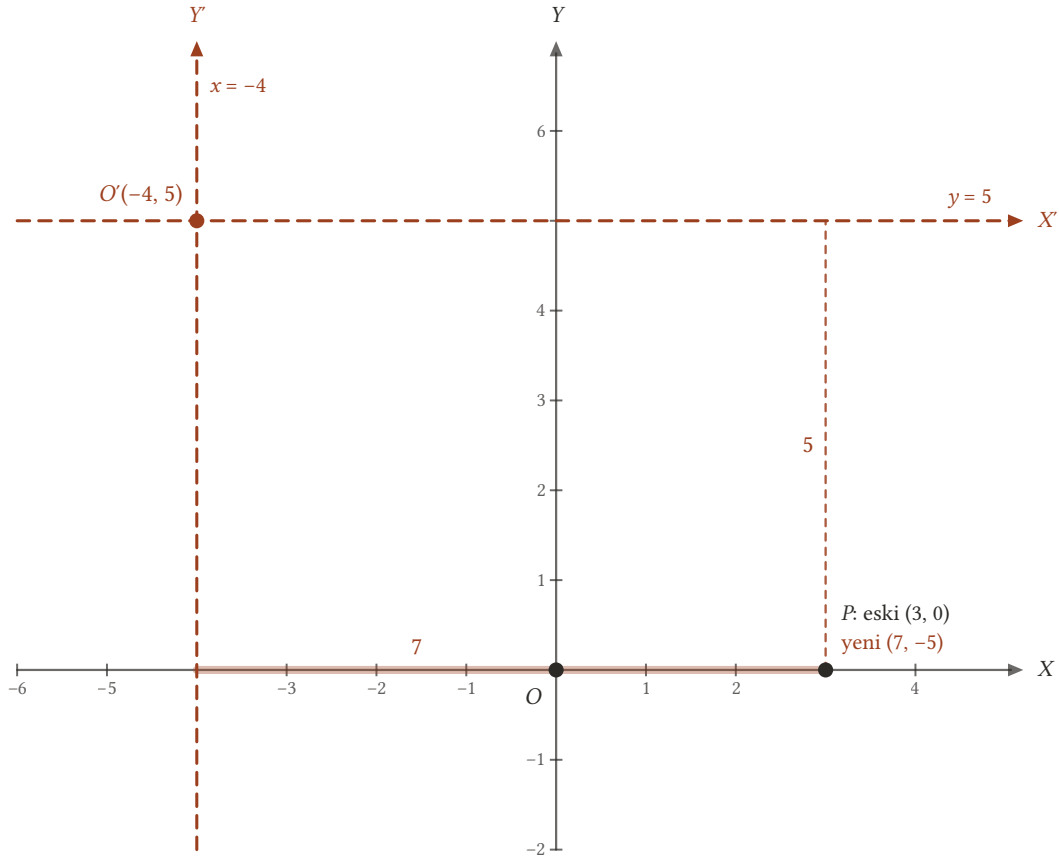
Şekil 16.16: y = 5 ve x = -4 doğruları yeni eksenler olunca başlangıç noktası O'(-4, 5) olur; P(3, 0) noktası yeni sistemde (7, -5) 'tir.
