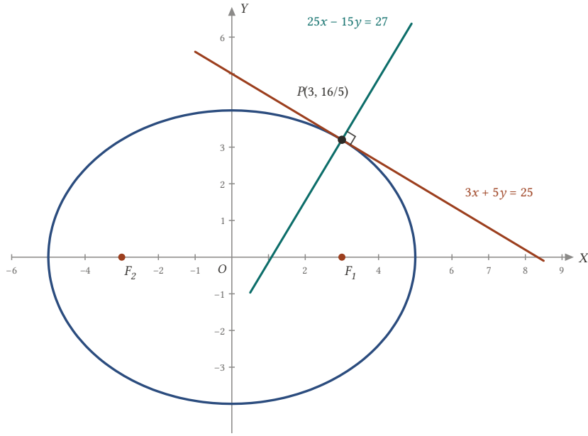
Şekil 18.14: x^2/25 + y^2/16 = 1 elipsinin P(3, 16/5) noktasındaki teğeti 3x + 5y = 25 , normali 25x - 15y = 27 'dir; eğimleri -3/5 ve 5/3 .
