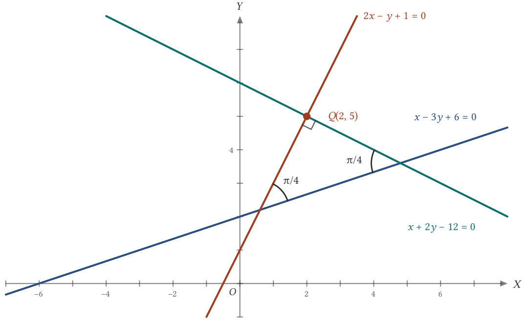
Şekil 2.32: Q(2, 5) 'ten geçen ve x - 3y + 6 = 0 doğrusuyla \pi/4 'lük açı yapan iki doğru: 2x - y + 1 = 0 ve x + 2y - 12 = 0 . İki çözüm doğrusu Q 'da dik kesişir.
