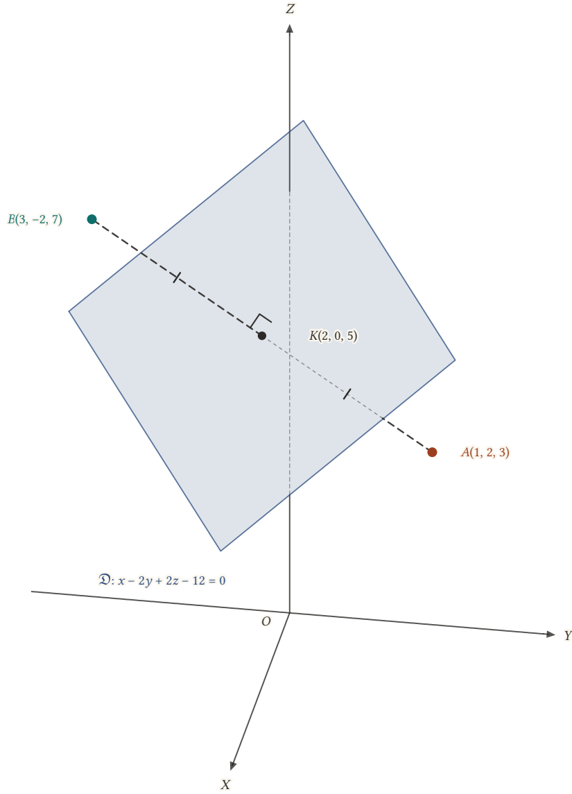
Şekil 15.11: A(1, 2, 3) ile simetriği B(3, -2, 7) arasındaki ayna, AB parçasının orta noktası K(2, 0, 5) 'ten geçen ve AB 'ye dik olan x - 2y + 2z - 12 = 0 düzlemidir. Düzlemin arkasında kalan parça kesikli ve soluktur.
