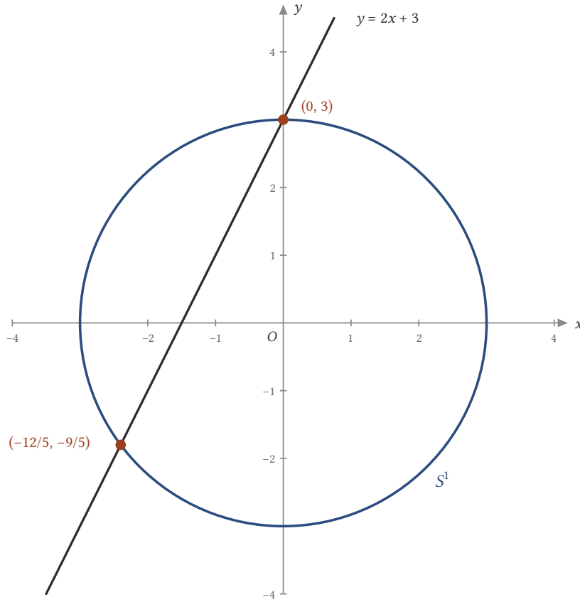
Şekil 4.26: y = 2x + 3 doğrusu x^2 + y^2 = 9 çemberini (0, 3) ve (-12/5, -9/5) noktalarında keser.
