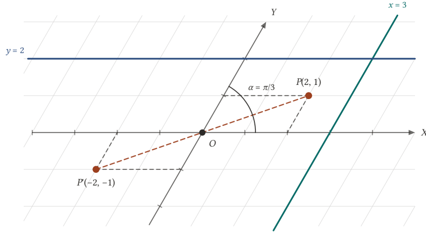
Şekil 5.2: \alpha = \pi/3 olan eğik sistemde P(2, 1) ile P'(-2, -1) noktaları O 'ya göre simetriktir (kesikli paralellere). x = 3 doğrusu Y -eksenine, y = 2 doğrusu X -eksenine paraleldir.
