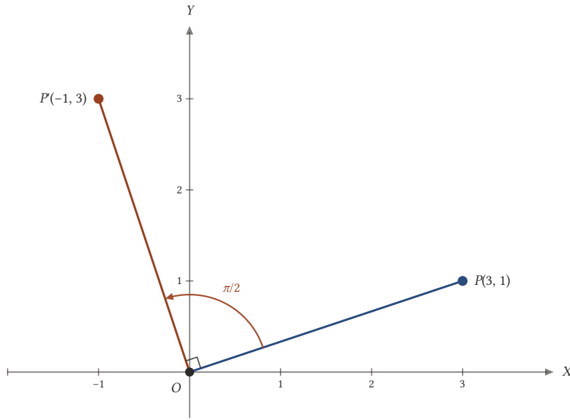
Şekil 17.4: \pi/2 radyanlık dönme P(3, 1) 'i P(-1, 3) 'e götürür; (2) formülleri P 'nden P' 'ye geri döndürür.
