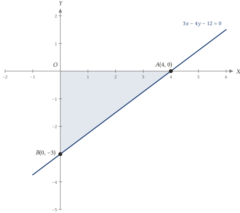
Şekil 3.4: X-eksenini A(4, 0) , Y-eksenini B(0, -3) noktasında kesen doğru: x/4 - y/3 = 1 , yani 3x - 4y - 12 = 0 .
