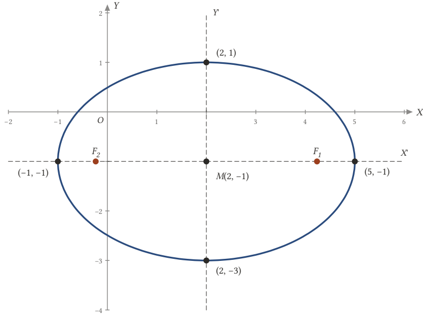
Şekil 18.11: 4x^2 + 9y^2 - 16x + 18y - 11 = 0 elipsi: merkez M(2, -1) , a = 3 , b = 2 , odaklar (2 \pm \sqrt{5}, -1) . Kesikli doğrular merkeze ötelenmiş X'Y' eksenleridir.
