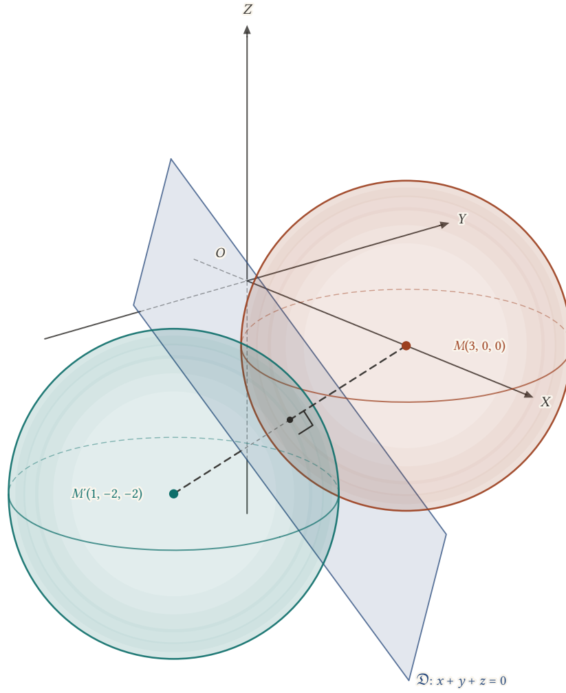
Şekil 15.8: (x - 3)^2 + y^2 + z^2 = 4 küresi (turuncu) ve x + y + z = 0 düzlemine göre simetriği (yeşil). Merkez M(3, 0, 0) merkeze, M'(1, -2, -2) 'ye gider; MM' parçası düzlemi orta noktası (2, -1, -1) 'de dik keser ve yarıçap 2 olarak kalır.
