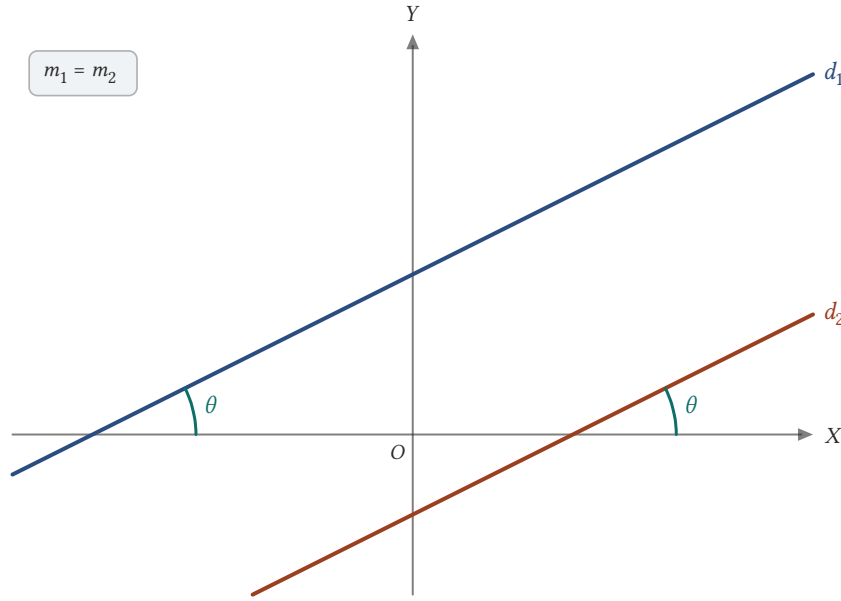
Şekil 2.17: Paralel d_1 ve d_2 doğruları X -ekseniyle aynı \theta açısını yapar; bu yüzden eğimleri eşittir.
