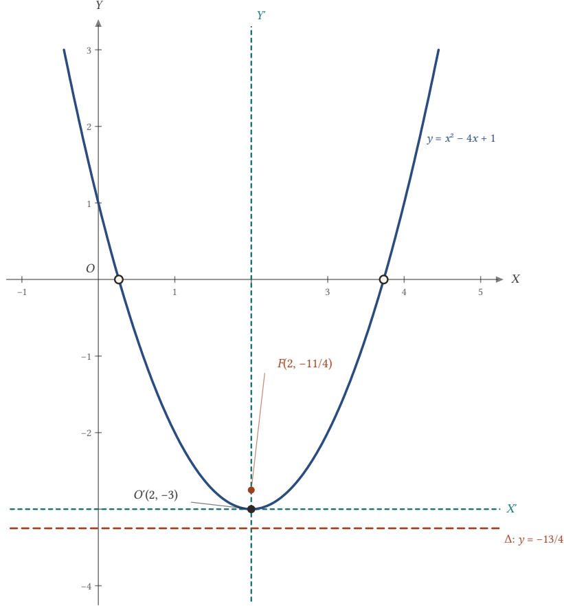
Şekil 20.7: Eksenleri köşe O'(2, -3) 'e ötelemek denklemi x'^2 = y' standart biçimine getirir; odak F(2, -11/4) , doğrultman y = -13/4 .
