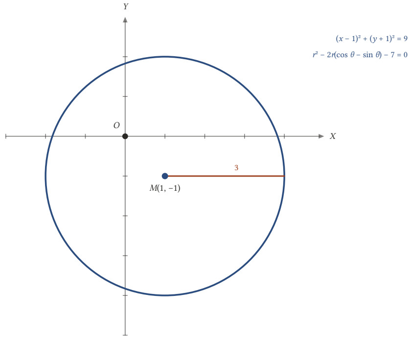
Şekil 5.25: r^2 - 2r(\cos \theta - \sin \theta) - 7 = 0 eğrisi, merkezi M(1, -1) ve yarıçapı 3 olan çemberdir; kutup çemberin içinde kalır.
