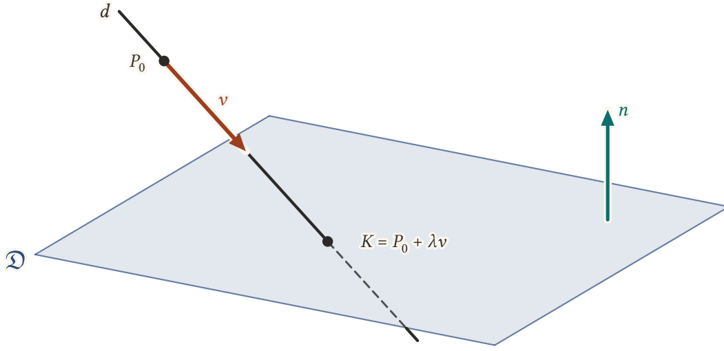
Şekil 14.2: d doğrusunun noktaları P_0 + \lambda v biçimindedir. Bu noktalardan düzlemin denklemini sağlayan tek nokta K 'dir; \lambda değeri (1)'den bulunur. Doğrunun düzlemin arkasında kalan parçası kesiklidir.
