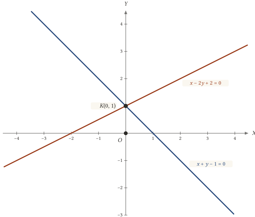
Şekil 21.5: d > 0 ve D = 0 : x^2 - xy - 2y^2 + x + 4y - 2 = 0 denklemi K(0, 1) 'de kesişen iki doğrudur.
