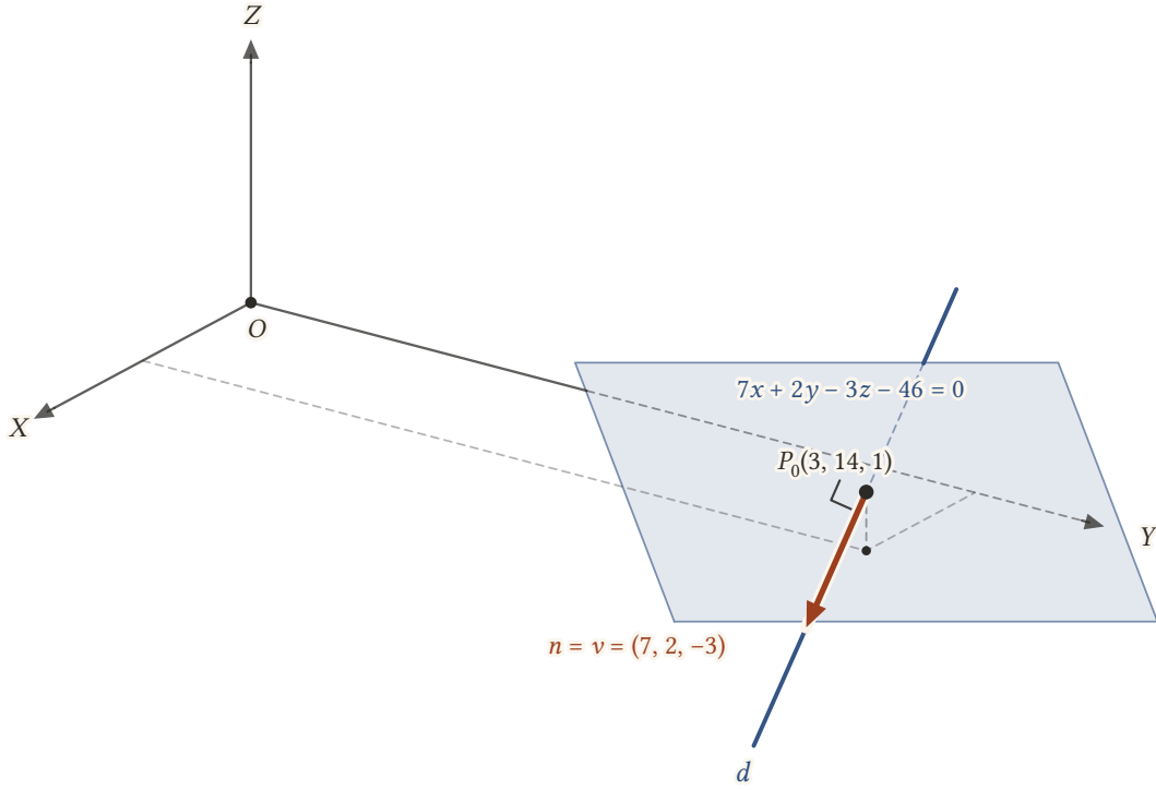
Şekil 12.20: P_0(3, 14, 1) noktasından geçen ve doğrultmanı (7, 2, -3) olan d doğrusuna dik düzlem: 7x + 2y - 3z - 46 = 0 . Doğrunun düzlemin arkasında kalan kısmı kesiklidir.
