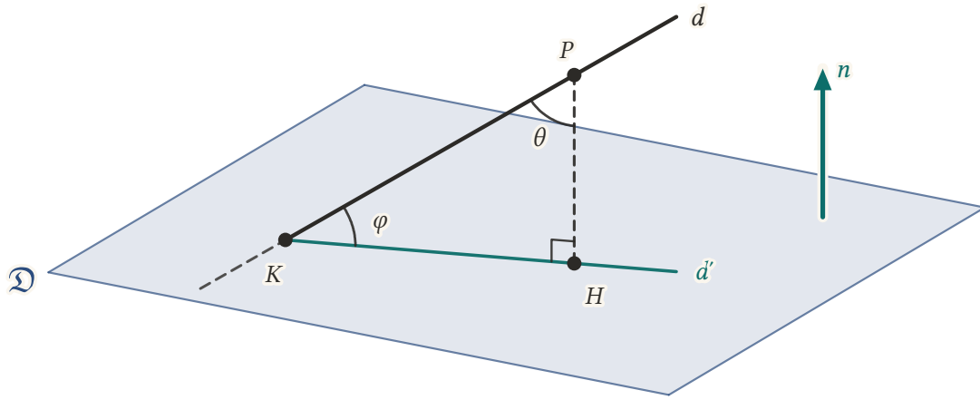
Şekil 14.8: Doğru ile düzlem arasındaki açı: P den inen dikmenin ayağı H 'dir ve d' = KH , d' nin düzlemdeki izdüşümüdür. \varphi , d ile d' arasındaki açıdır; PHK dik üçgeninde \varphi + \theta = \pi/2 olur.
