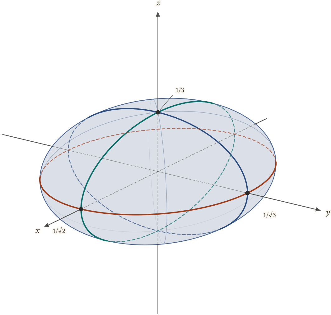
Şekil 23.18: Elipsoid 2x^2 + 3y^2 + 9z^2 = 1 ve koordinat düzlemlerindeki izleri: 2x^2 + 3y^2 = 1 (kırmızı, z = 0 ), 2x^2 + 9z^2 = 1 (yeşil, y = 0 ), 3y^2 + 9z^2 = 1 (mavi, x = 0 ). c = 1/3 küçük olduğundan yüzey z doğrultusunda basıktır.
