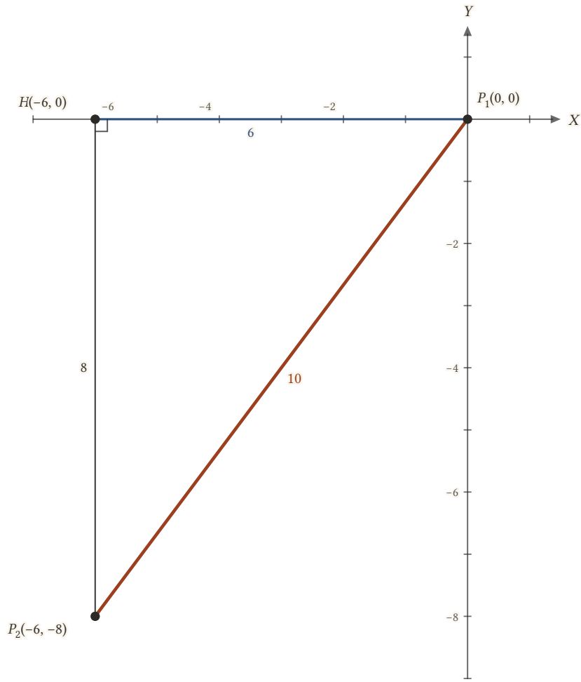
Şekil 1.9: Başlangıç noktasına uzaklık: dik kenarları 6 ve 8 olan dik üçgenin hipotenüsü 10'dur.
