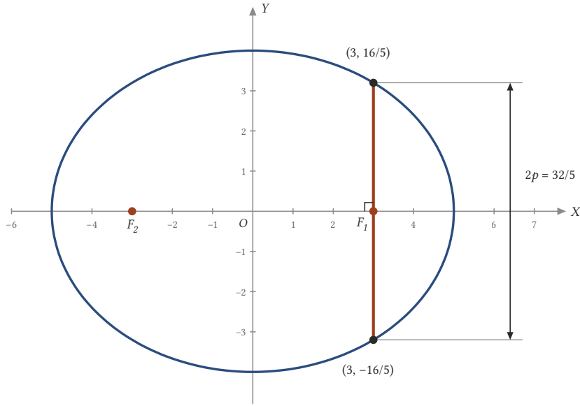
Şekil 18.12: x^2/25 + y^2/16 = 1 elipsinde F_1(3, 0) odağından asal eksene dik kirişin uzunluğu 2p = 2b^2/a = 32/5 'tir.
