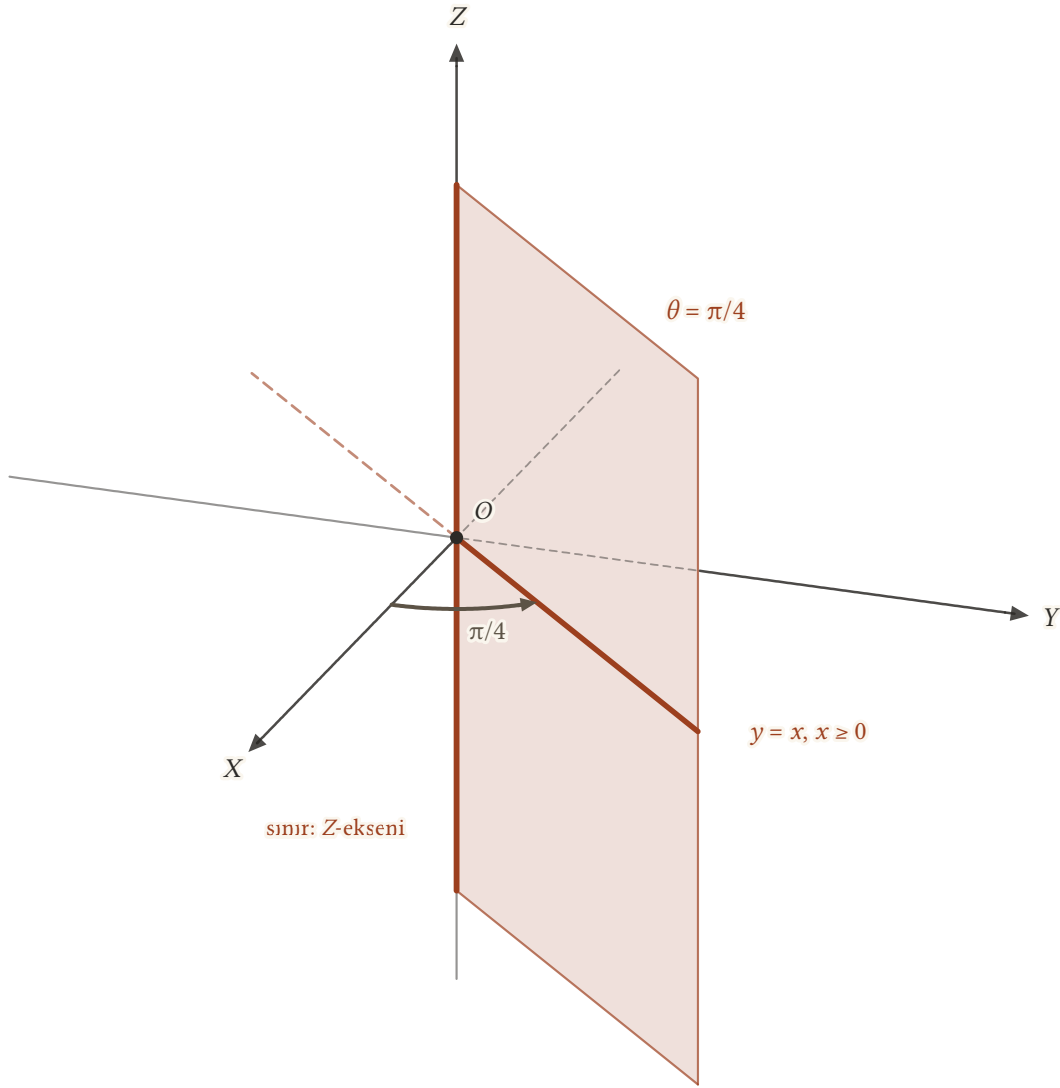
Şekil 22.3: \theta = \pi/4 denkleminin grafiği: Z-ekseniyle sınırlanan yarım düzlem ( -2 \leq z \leq 2 parçası). XY-düzlemindeki izi y = x, x \geq 0 yarı doğrusudur; kesikli yarı doğru y = x doğrusunun öbür yarısıdır ve \theta = 5\pi/4 yarım düzlemine aittir.
