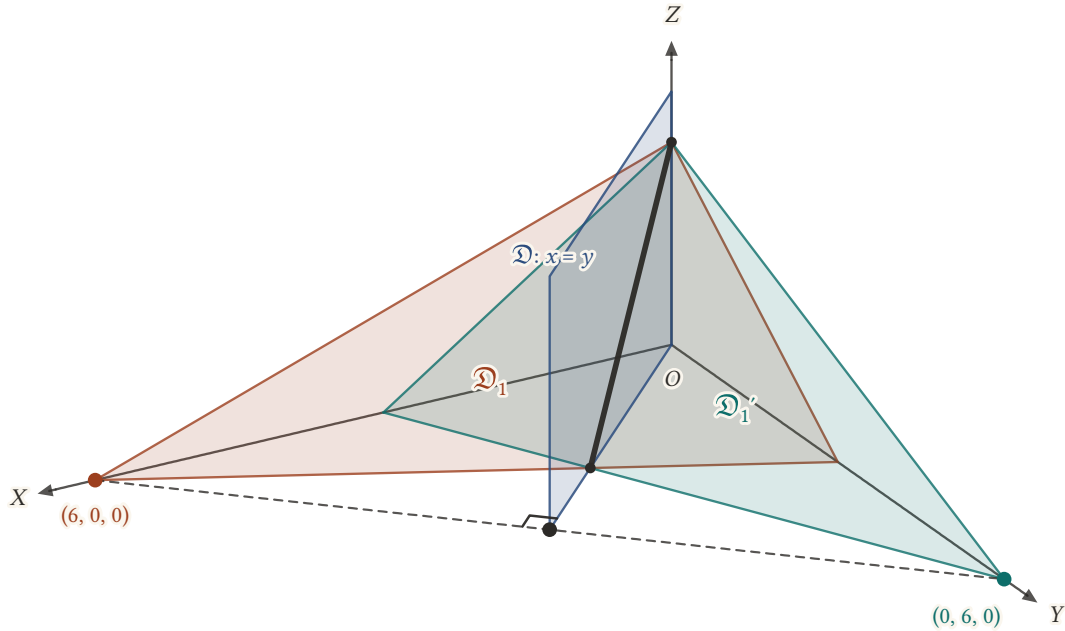
Şekil 15.13: Birinci bölgedeki parçalar: x + 2y + 3z = 6 (turuncu), simetriği 2x + y + 3z = 6 (yeşil) ve ayna x = y (mavi). Üç düzlem kalın çizilen ortak doğru boyunca kesişir; (6, 0, 0) noktasının görüntüsü (0, 6, 0) 'dır.
