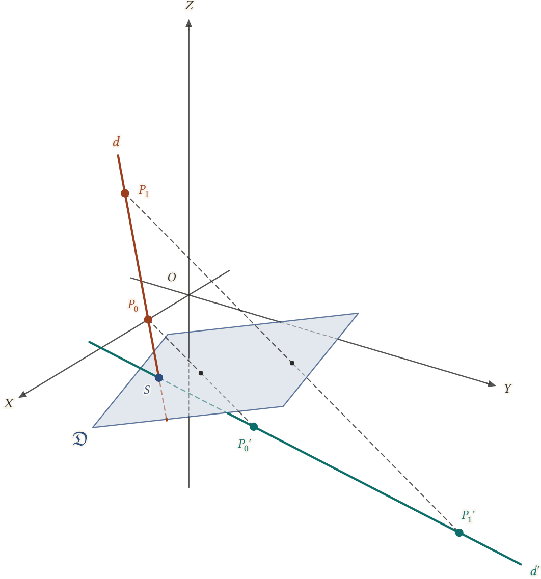
Şekil 15.9: d doğrusu (turuncu) ve 2x - 3y + 4z + 4 = 0 düzlemine göre simetriği d' (yeşil). P_0(1, 0, 0) ve P_1(3, 1, 3) noktalarının simetrikleri P_0'(5/29, 36/29, -48/29) ve P_1'(11/29, 143/29, -65/29) 'dir; iki doğru düzlemi aynı S(1/13, -6/13, -18/13) noktasında keser. Düzlemin arkasında kalan parçalar kesiklidir.
