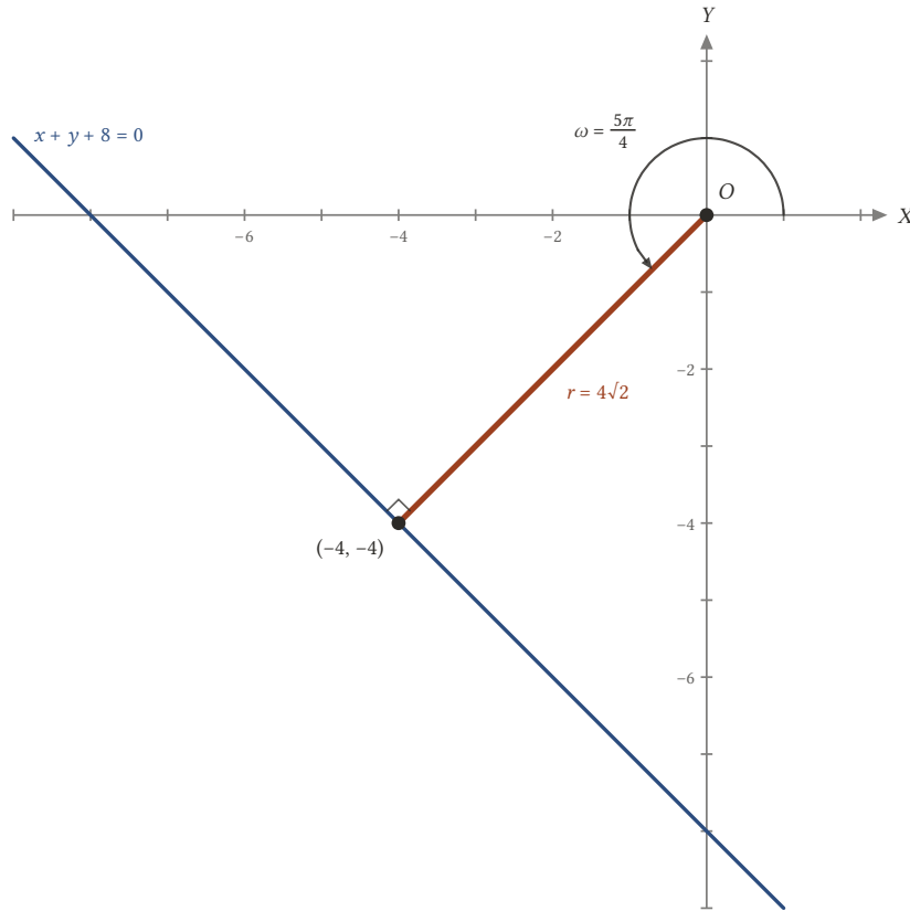
Şekil 3.14: x + y + 8 = 0 doğrusuna orijinden inen dikmenin ayağı (-4, -4) 'tür: r = 4\sqrt{2} , \omega = 5\pi/4 .
