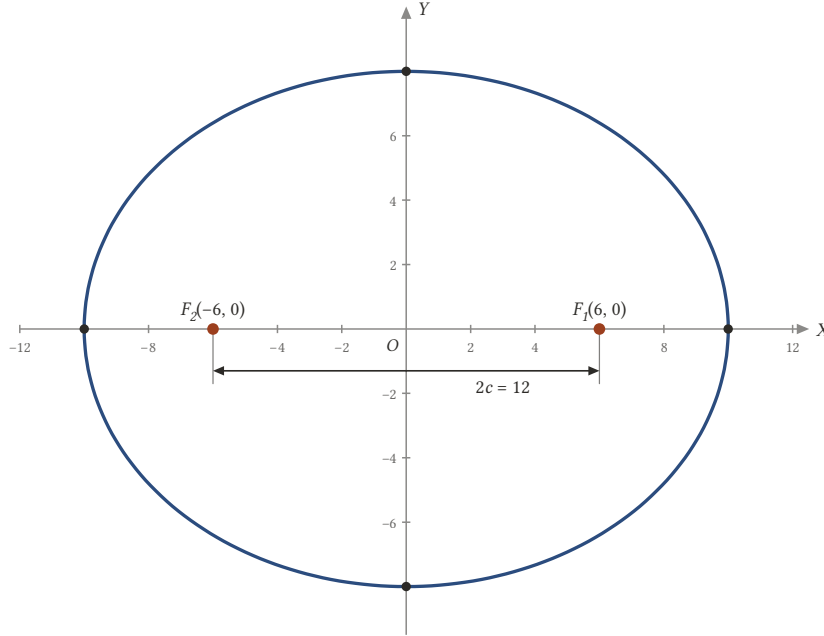
Şekil 18.9: x^2/100 + y^2/64 = 1 elipsinde c = 6 : odaklar F_1(6, 0) ve F_2(-6, 0) , aralarındaki uzaklık 2c = 12 .
