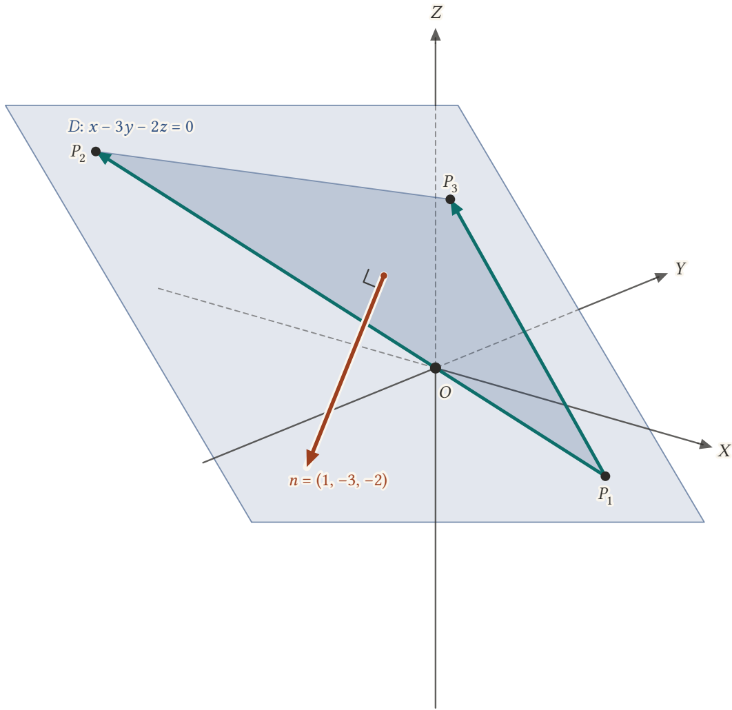
Şekil 12.10: P_1(1, 1, -1) , P_2(-2, -2, 2) , P_3(1, -1, 2) noktalarından geçen x - 3y - 2z = 0 düzlemi; düzlem orijinden de geçer. Normal, üçgenin ağırlık merkezinden çizildi.
