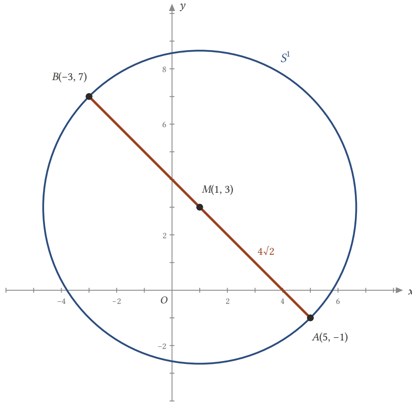
Şekil 4.5: Çapın orta noktası merkezdir: M(1, 3) . Yarıçap |MA| = 4\sqrt{2} olduğundan çemberin denklemi (x - 1)^2 + (y - 3)^2 = 32 'dir.
