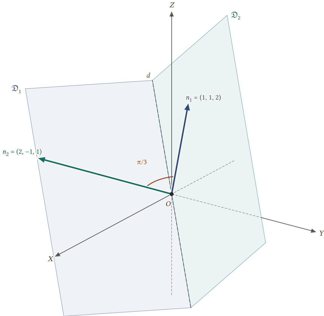
Şekil 13.8: n_1 = (1, 1, 2) ile n_2 = (2, -1, 1) arasındaki açı \pi/3 olup düzlemler arasındaki açı da budur. Soluk yarım düzlemler x + y + 2z = 0 ile 2x - y + z = 0 düzlemlerinin parçaları, kesikli doğru da onların arakesiti d 'dir.
