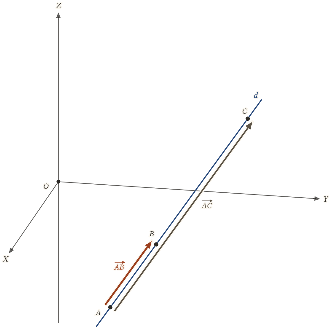
Şekil 10.15: A, B, C aynı d doğrusu üzerindedir: AC vektörü AB vektörünün 3 katıdır.
