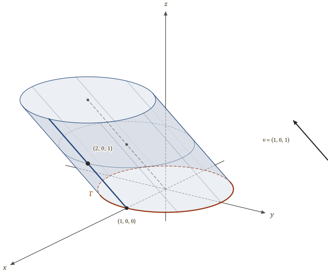
Şekil 23.5: Eğik silindir (x - z)^2 + y^2 = 1 , 0 \leq z \leq 2 . Dayanak çemberi \Gamma (kırmızı) xy -düzleminde; z = 1 ve z = 2 kesitleri merkezleri (1, 0, 1) ve (2, 0, 2) olan birim çemberlerdir. Kalın üreteç (1, 0, 0) 'dan v = (1, 0, 1) doğrultusunda çıkar ve (2, 0, 1) noktasından geçer.
