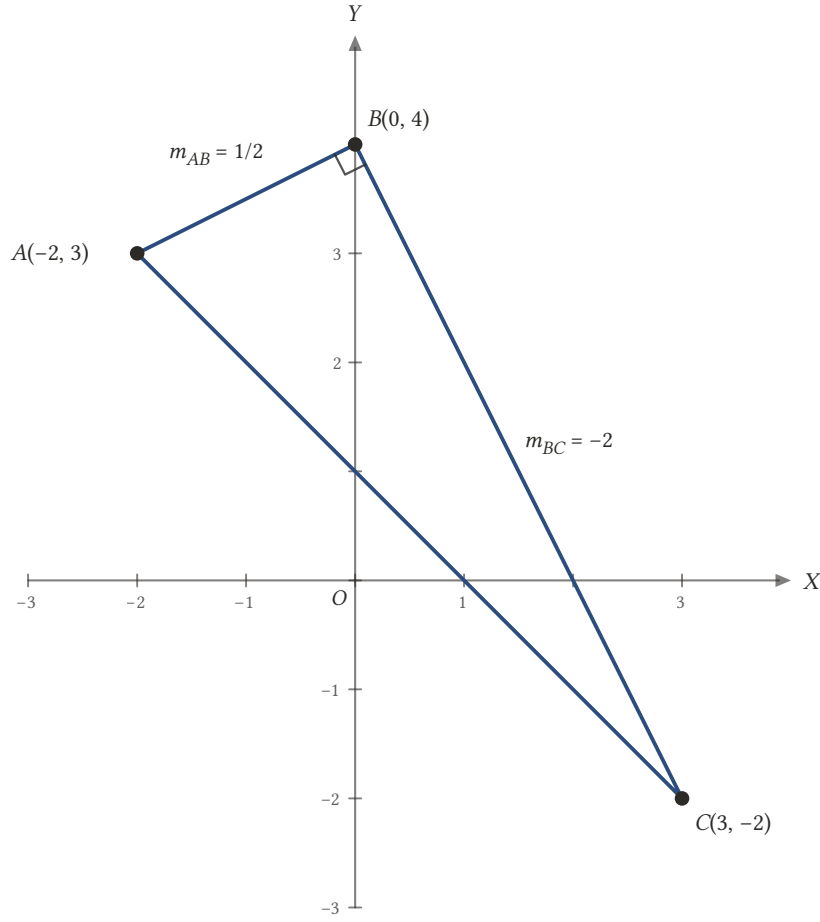
Şekil 2.20: A(-2, 3) , B(0, 4) , C(3, -2) üçgeninde m_{AB} \cdot m_{BC} = (1/2)(-2) = -1 ; dik açı B köşesindedir.
