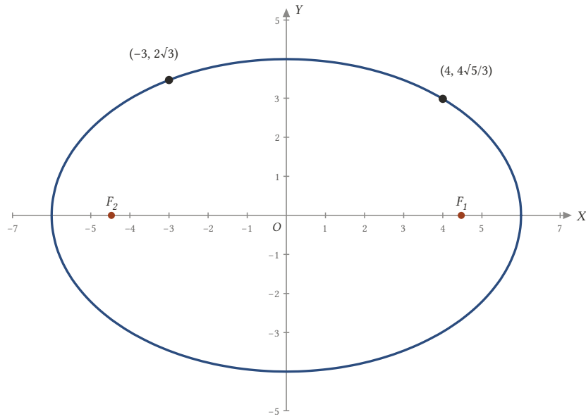
Şekil 18.24: (-3, 2\sqrt{3}) ve (4, 4\sqrt{5}/3) noktalarından geçen x^2/36 + y^2/16 = 1 elipsi; odakları (\pm 2\sqrt{5}, 0) .
