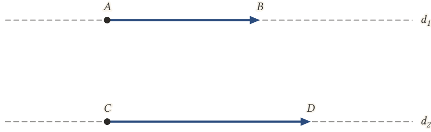
Şekil 7.2: d_1 \parallel d_2 olduğundan AB ve CD yönlü doğru parçaları aynı doğrultuludur.
