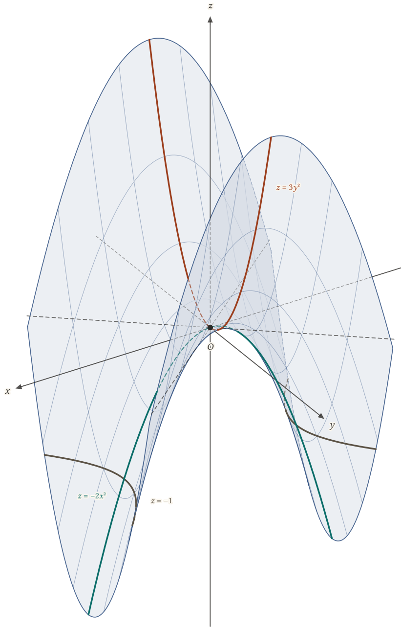
Şekil 23.23: Hiperbolik paraboloid (eyer) -2x^2 + 3y^2 = z , |x| \leq 1 , |y| \leq 0,8 . yz -düzlemindeki iz yukarı açılan z = 3y^2 (kırmızı), xz -düzlemindeki iz aşağı açılan z = -2x^2 (yeşil) parabolüdür; z = 0 izi kesikli doğru çiftidir, z = -1 izi köşeleri (\pm 1/\sqrt{2}, 0, -1) olan bir hiperboldür (kahverengi). O eyer noktasıdır.
