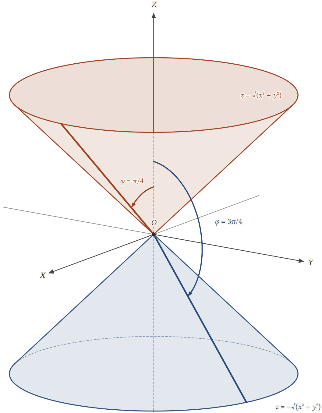
Şekil 22.12: x^2 + y^2 = z^2 çift konisi ( |z| \leq 2,2 parçası): üstteki \varphi = \pi/4 konisi ile alttaki \varphi = 3\pi/4 konisinin birleşimi. İki açı da pozitif Z -ekseninden ölçülür; koninin arkasında kalan çizgiler kesiklidir.
