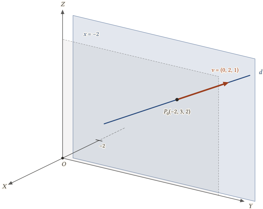
Şekil 12.15: v = (0, 2, 1) vektörüne paralel olan d doğrusu x = -2 düzleminin içinde kalır; bu düzlem YZ -düzlemine (soluk) paraleldir.
