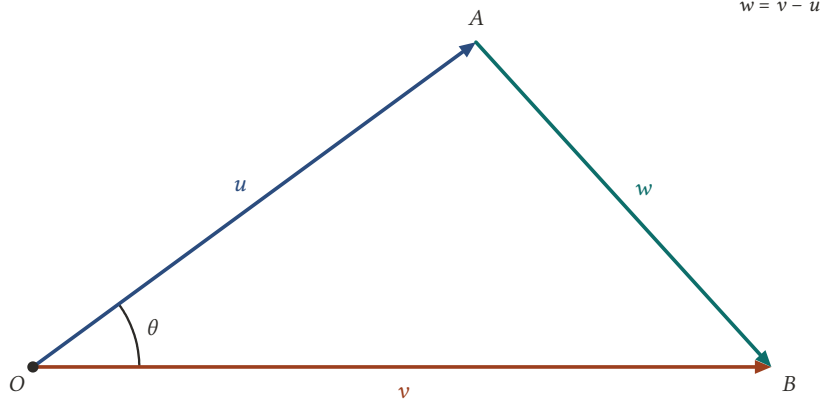
Şekil 8.2: u ile v aynı O noktasından çizilir; A 'dan B 'ye giden üçüncü kenar w = v - u olur. O köşesindeki açı \theta 'dır ve Kosinüs Teoremi bu üçgene uygulanır.
