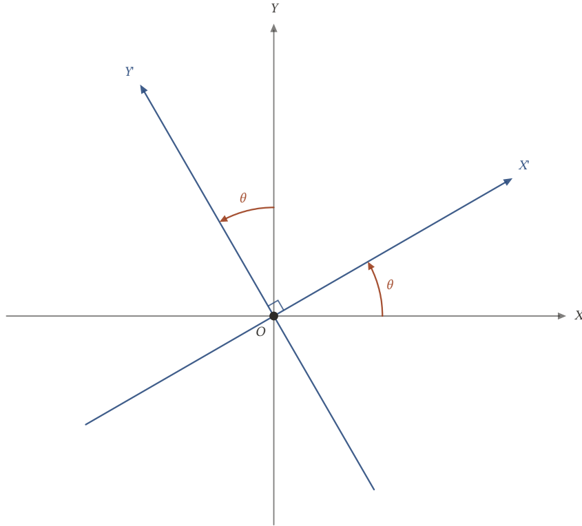
Şekil 17.8: XY sistemi \theta kadar döndürülünce X'Y' sistemi elde edilir; yeni eksenler de birbirine diktir.
