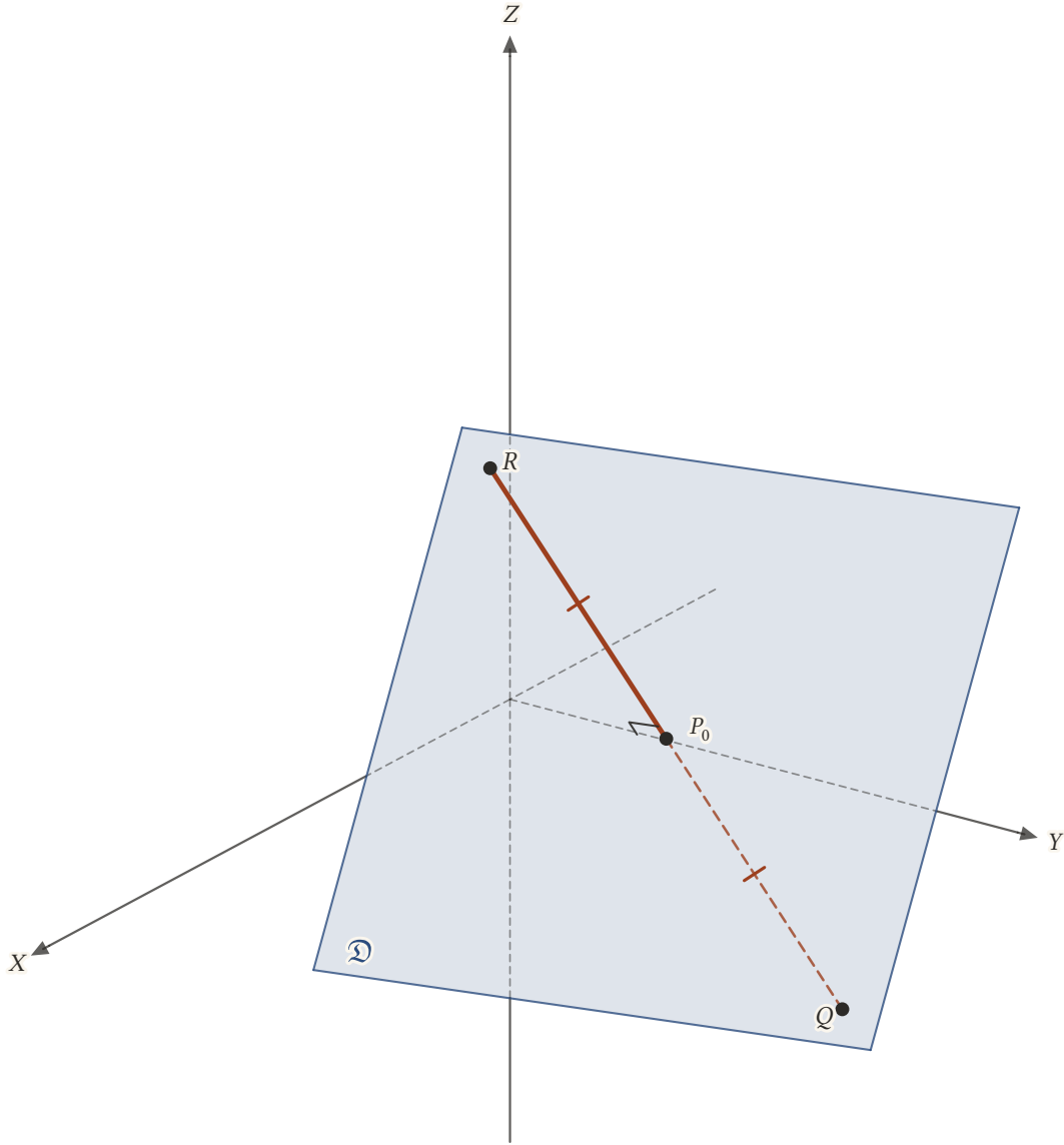
Şekil 13.18: [QR] doğru parçasının orta dikme düzlemi 4x + y + 4z - 15 = 0 : orta nokta P_0(2, 3, 1) 'den geçer ve QR 'ye diktir. Doğru parçasının düzlemin arkasında kalan kısmı kesiklidir.
