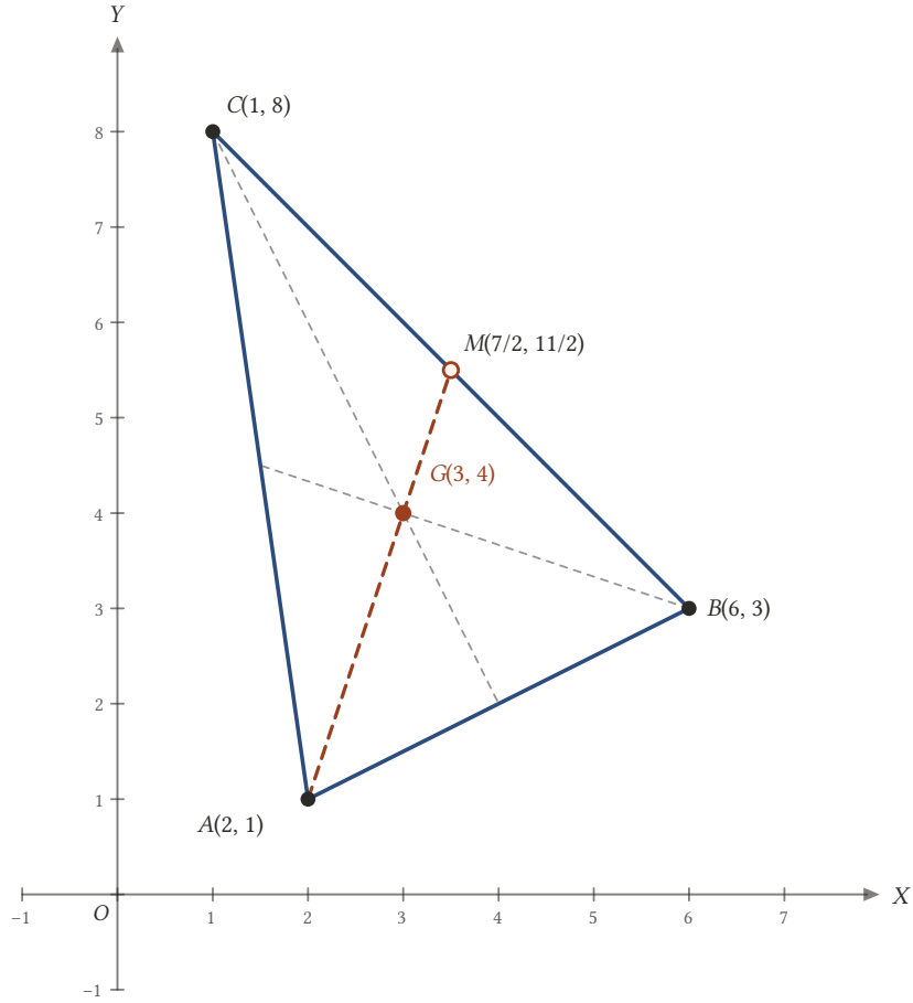
Şekil 2.5: A(2, 1) , B(6, 3) , C(1, 8) üçgeninin ağırlık merkezi G(3, 4) . Turuncu AM kenarortayı G tarafından 2 : 1 oranında bölünür; diğer iki kenarortay da G den geçer.
