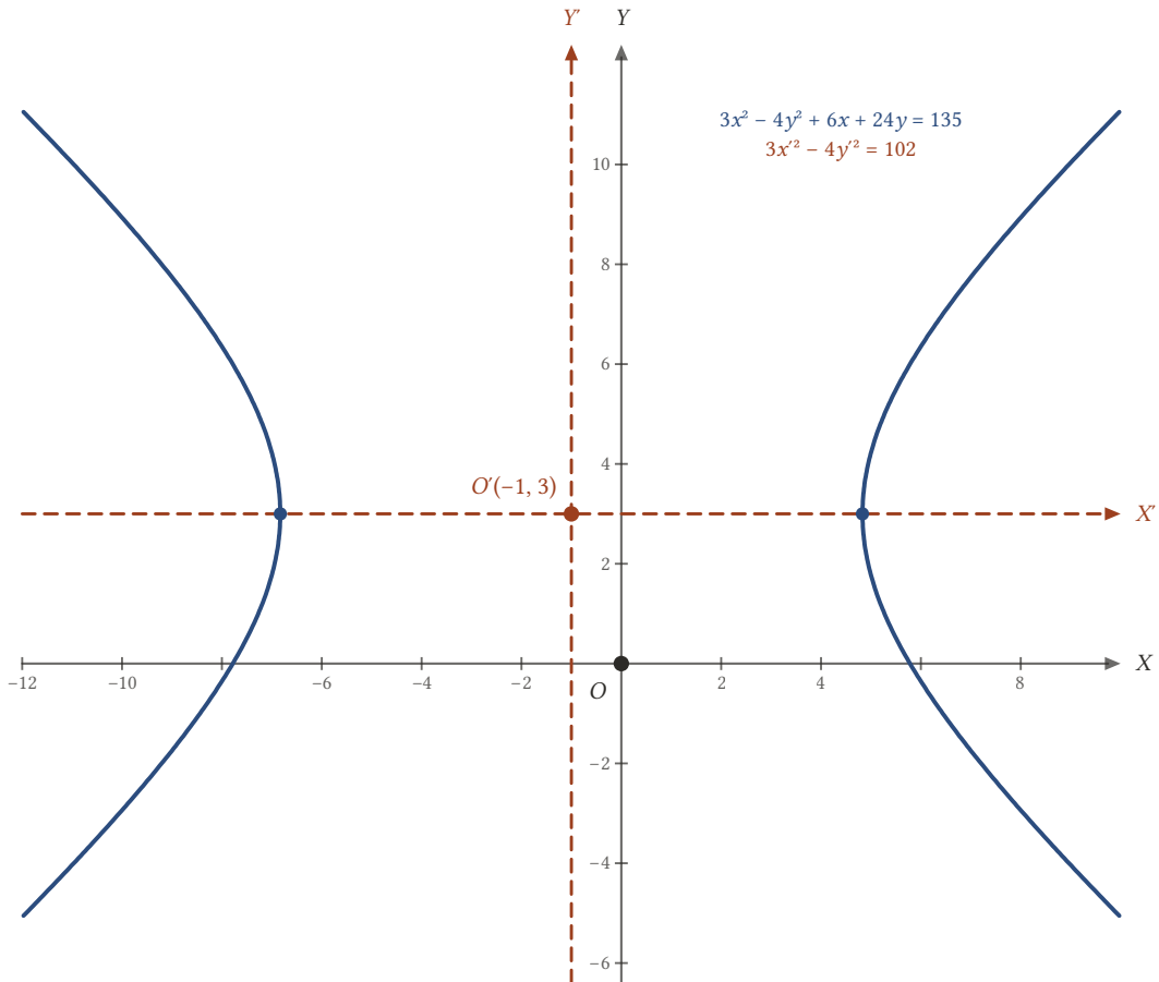
Şekil 16.20: Eksenler O'(-1, 3) noktasına ötelenince eğrinin denklemi 3x'^2 - 4y'^2 = 102 olur.
