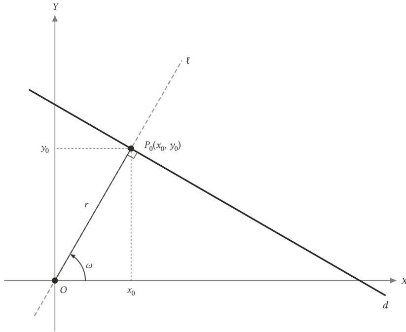
Şekil 3.8: Normal denklemin kuruluşu: orijinden d 'ye inen dikme \ell doğrusu üzerindedir, uzunluğu r , X -ekseniyle yaptığı açı \omega 'dır. Dikmenin ayağı P_0 = (r \cos \omega, r \sin \omega) noktasıdır.
