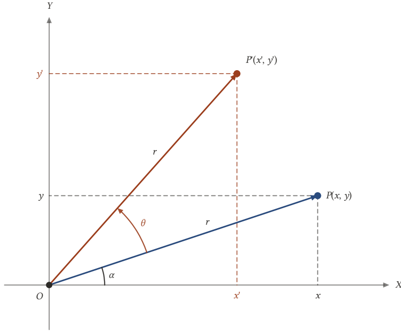
Şekil 17.2: P'nin kutupsal açısı \alpha , P'nünkü \alpha + \theta 'dir; ikisinin de O'ya uzaklığı r 'dir.
