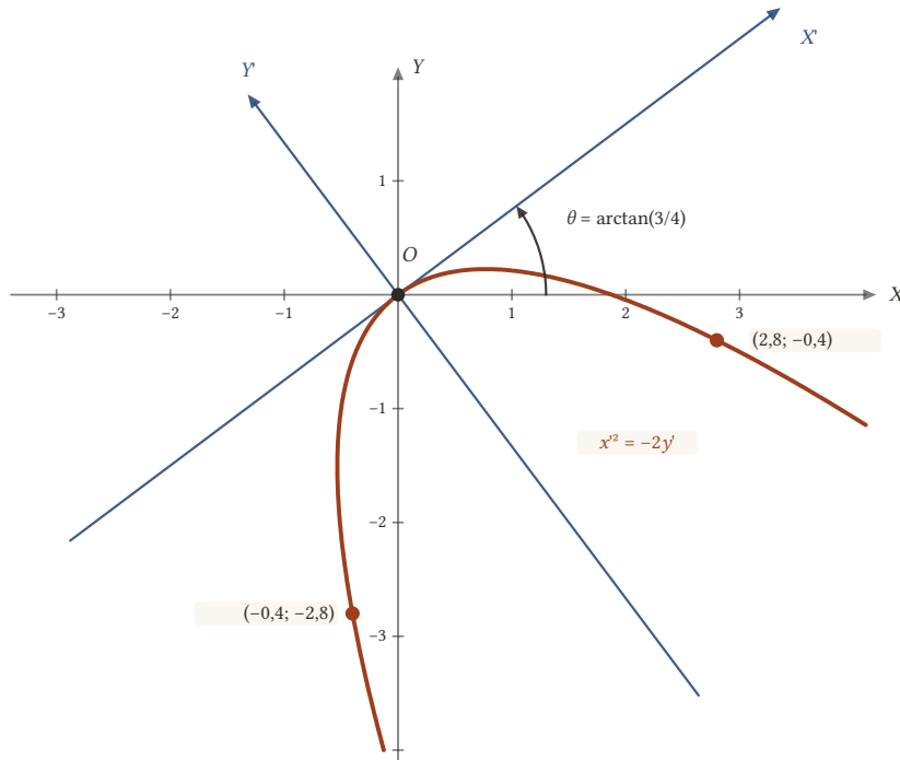
Şekil 21.16: Eksenler \arctan(3/4) döndürülünce 16x^2 + 24xy + 9y^2 - 30x + 40y = 0 parabolü x'^2 = -2y' olur.
