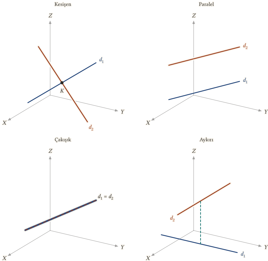
Şekil 11.6: Uzayda iki doğrunun dört durumu: kesişen doğrular (tek ortak nokta K ), paralel ve farklı doğrular, çakışık doğrular ve aykırı doğrular. Aykırı doğrular ne kesişir ne de paraleldir; kesikli parça ikisine birden diktir.
