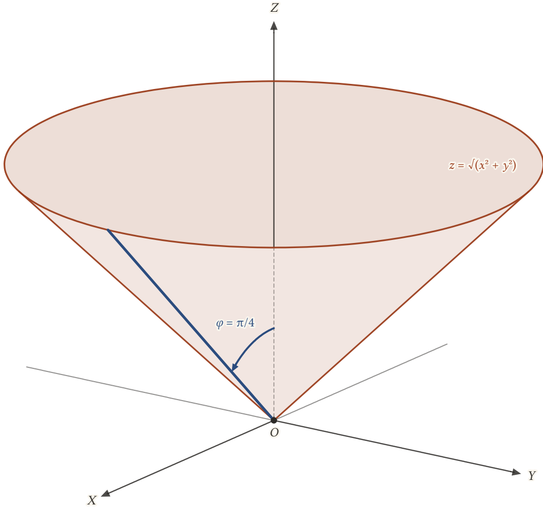
Şekil 22.7: \varphi = \pi/4 denkleminin grafiği: tepesi O 'da, eksen Z -ekseni olan ve XY -düzleminin üstünde kalan z = \sqrt{x^2 + y^2} konisi ( 0 \leq z \leq 2,5 parçası). Mavi ana doğru Z -ekseniyle \pi/4 açı yapar; koninin arkasında kalan çizgiler kesiklidir.
