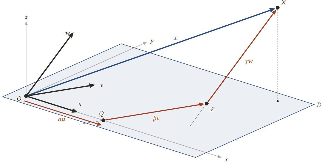
Şekil 7.19: X'ten w'ya paralel çizilen doğru u ile v'nin düzlemini P'de, P'den v'ye paralel çizilen doğru u doğrusunu Q'da keser; böylece x = \alpha u + \beta v + \gamma w olur.
