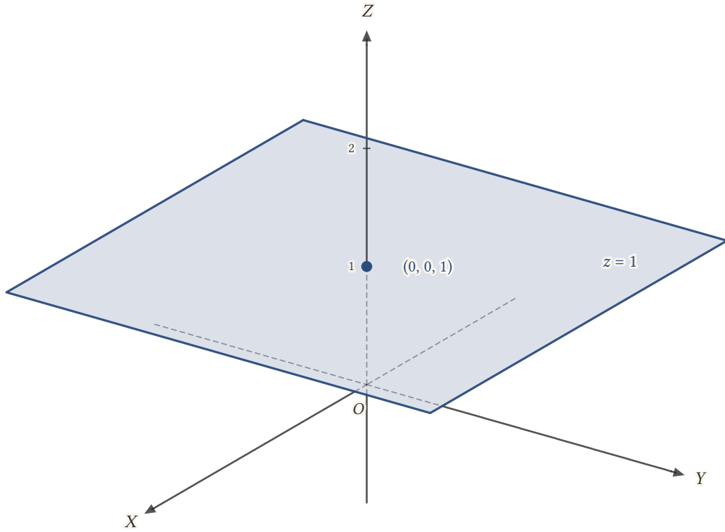
Şekil 6.7: z = 1 düzlemi: XY -düzleminin 1 birim yukarısında ve ona paralel. Z -ekseni düzlemi (0, 0, 1) noktasında deler; düzlemin arkasında kalan eksen parçaları kesikli ve soluktur.
