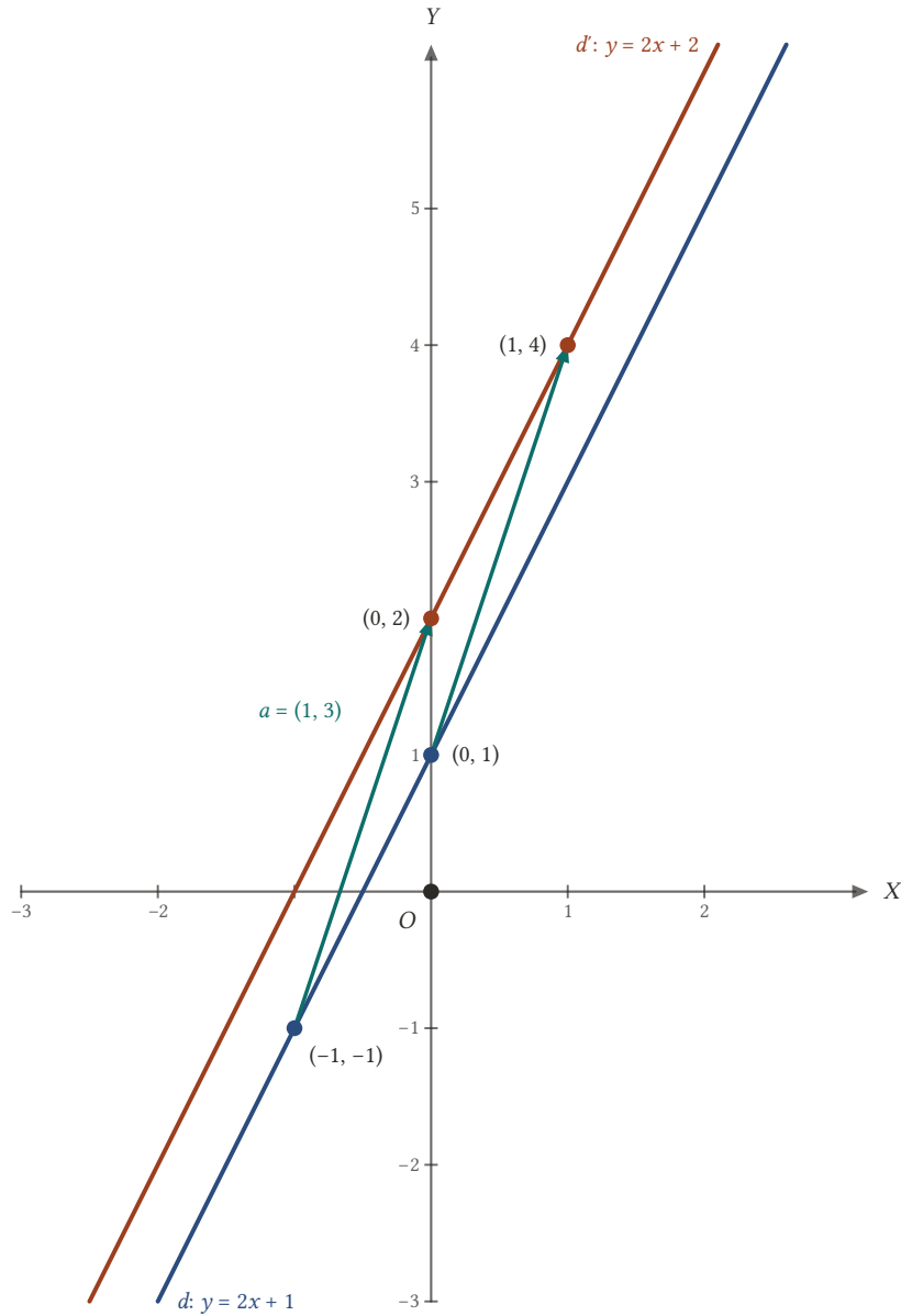
Şekil 16.7: d doğrusunun her noktası a = (1, 3) kadar ötelenince d' doğrusu oluşur; iki doğrunun eğimi aynıdır.
