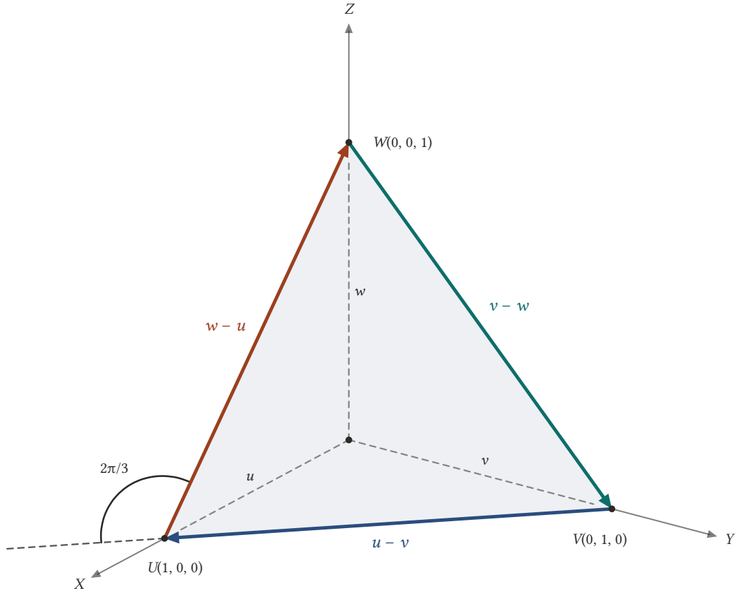
Şekil 8.18: u = e_1, v = e_2, w = e_3 için UVW eşkenar bir üçgendir. Fark vektörleri üçgenin kenarlarını sırayla dolaşır; ardışık iki kenar vektörü arasındaki açı, dış açı olan 2\pi/3 'tür.
