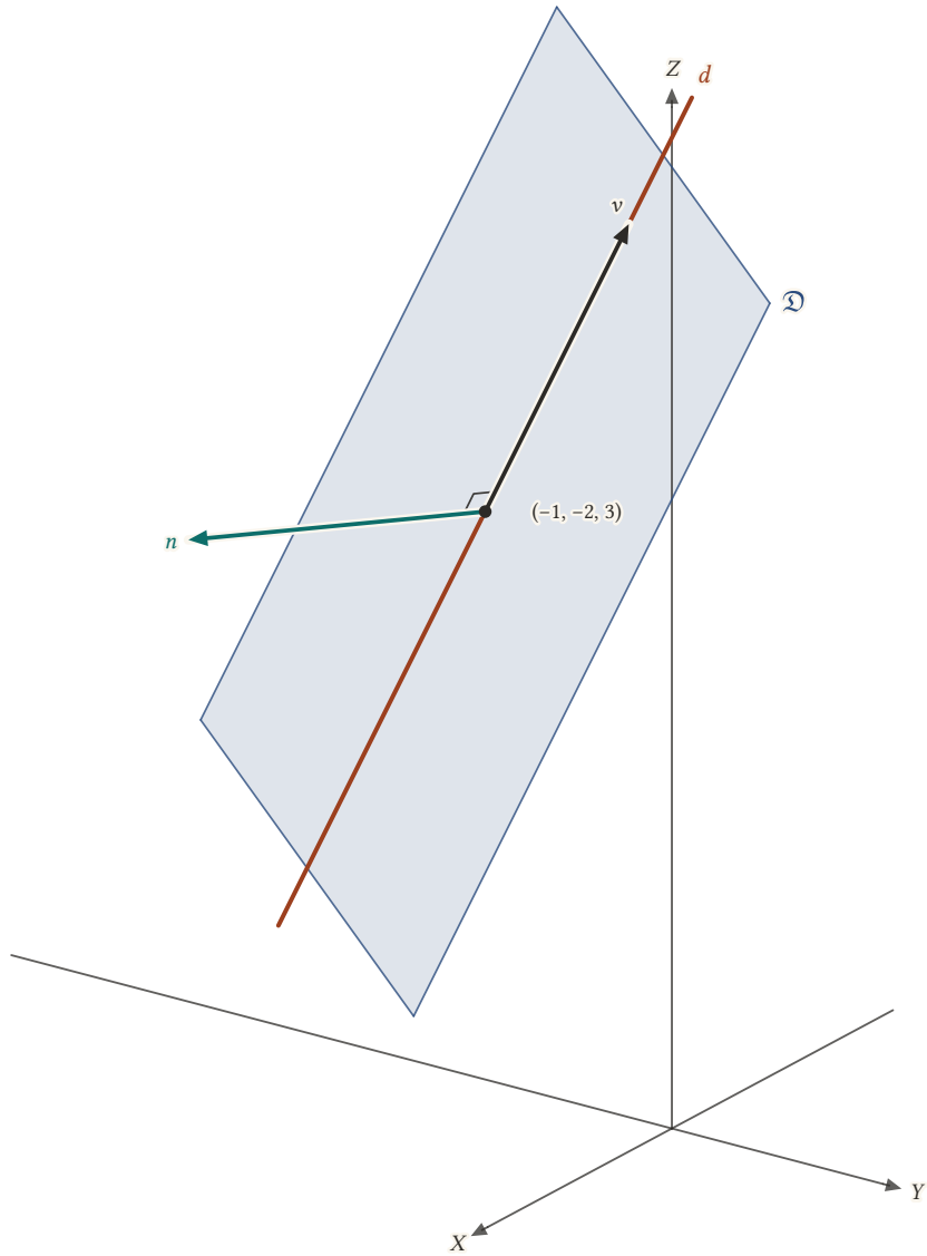
Şekil 13.16: d doğrusu 6x - 2y + z - 1 = 0 düzleminin içinde yatar: doğrultusu v = (0, 2, 4) normal n = (6, -2, 1) 'e diktir ve (-1, -2, 3) noktası düzlemedir. Oklar v/2 ve n/3 boyunda çizilmiştir.
