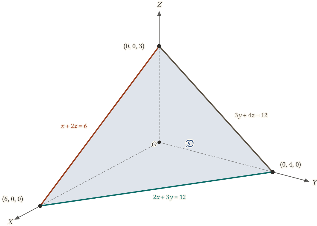
Şekil 13.10: 2x + 3y + 4z - 12 = 0 düzleminin birinci bölgedeki parçası. Üçgenin kenarları düzlemin izleri üzerindedir: XY -düzleminde 2x + 3y = 12 , XZ -düzleminde x + 2z = 6 , YZ -düzleminde 3y + 4z = 12 .
