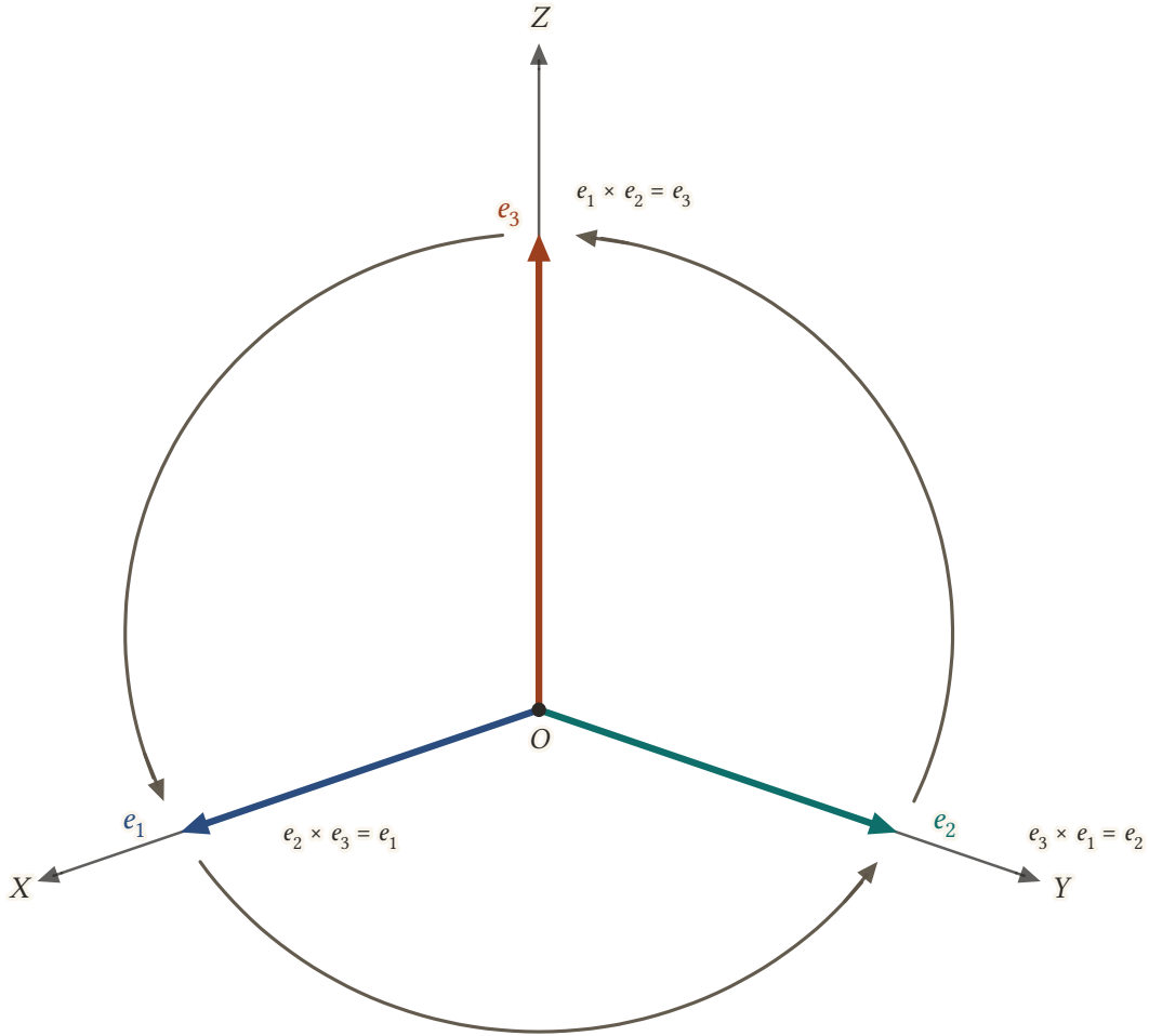
Şekil 9.1: Standart baz vektörleri ve döngü: e_1 \rightarrow e_2 \rightarrow e_3 \rightarrow e_1 sırasında ardışık iki vektörün vektörel çarpımı döngüdeki bir sonraki vektördür; her yazı, sonucu olan vektörün ucunun yanındadır.
