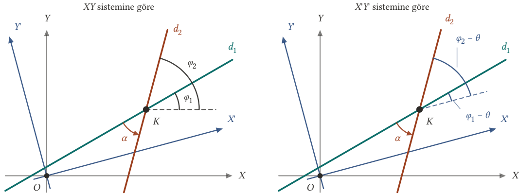
Şekil 17.11: Eksenler \theta döndürülünce her doğrunun eğim açısı \theta kadar azalır; d_1 'den d_2 'ye yönelmiş açı \alpha değişmez.
