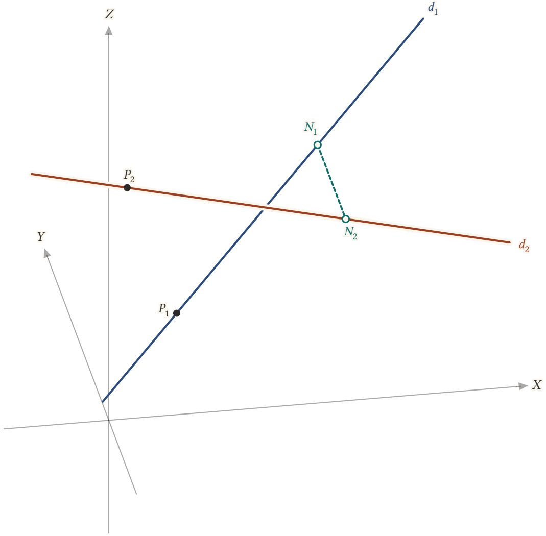
Şekil 11.10: Aykırı iki doğru: sayfada kesişiyormuş gibi görünseler de önde kalan doğru arkadakinin üzerinden geçer. En yakın noktaları N_1(15/7, 6/7, 16/7) ile N_2(16/7, 1/7, 13/7) arasındaki kesikli parça iki doğruya da diktir; uzunluğu \sqrt{35}/7 'dir.
