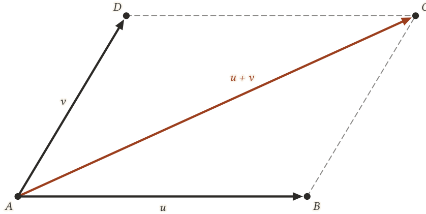
Şekil 7.10: Paralelkenar kuralı: u ve v ortak A noktasından çizilince toplamı, üzerlerine kurulan paralelkenarın AC köşegenidir.
