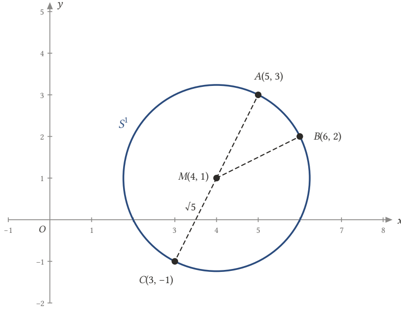
Şekil 4.24: A(5, 3) , B(6, 2) ve C(3, -1) noktalarından geçen çemberin merkezi M(4, 1) , yarıçapı \sqrt{5} 'tir.
