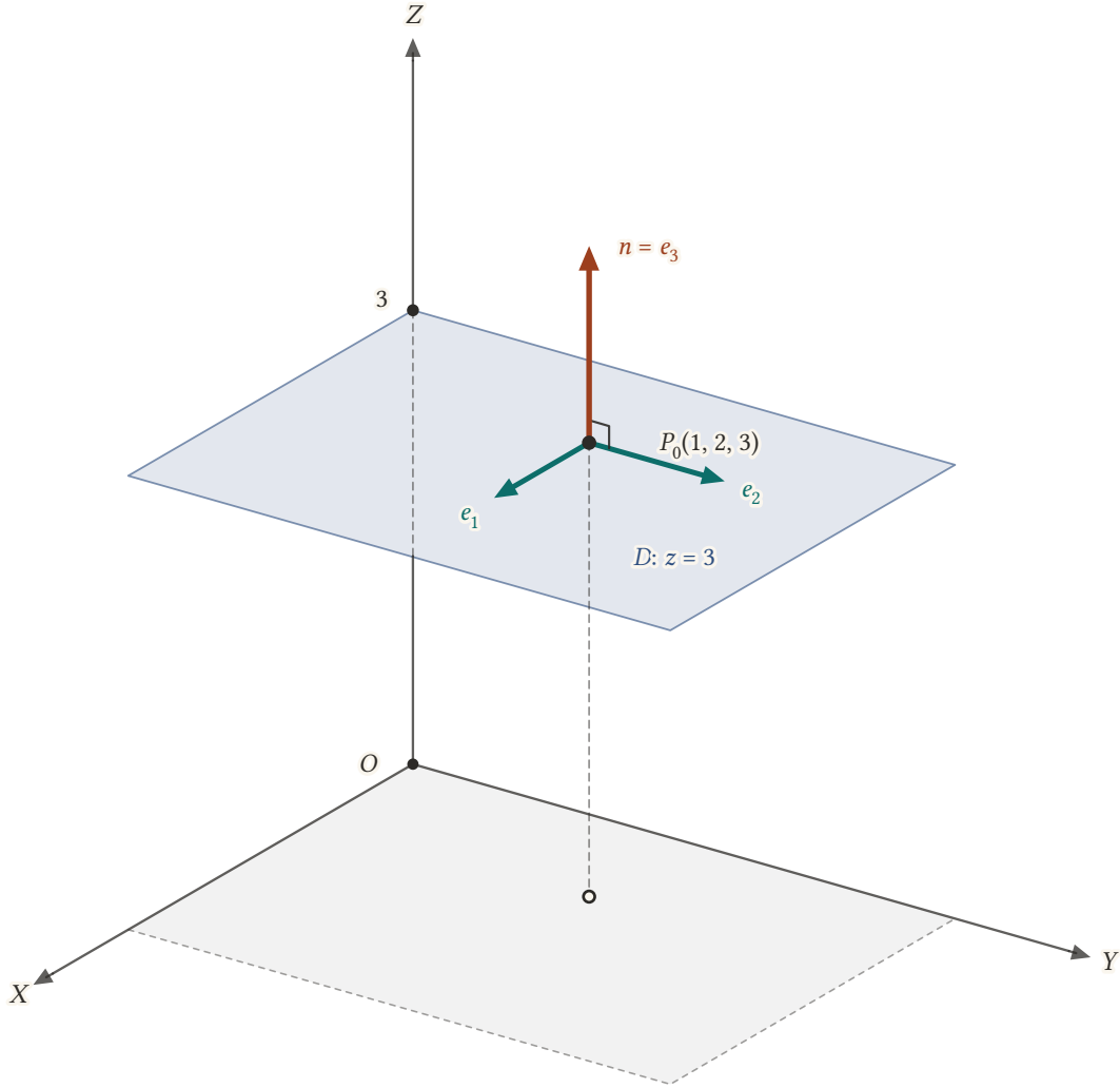
Şekil 12.8: X - ve Y -eksenine paralel olup P_0(1, 2, 3) 'ten geçen z = 3 düzlemi: XY -düzlemine (soluk) paraleldir, normali e_3 'tür.
