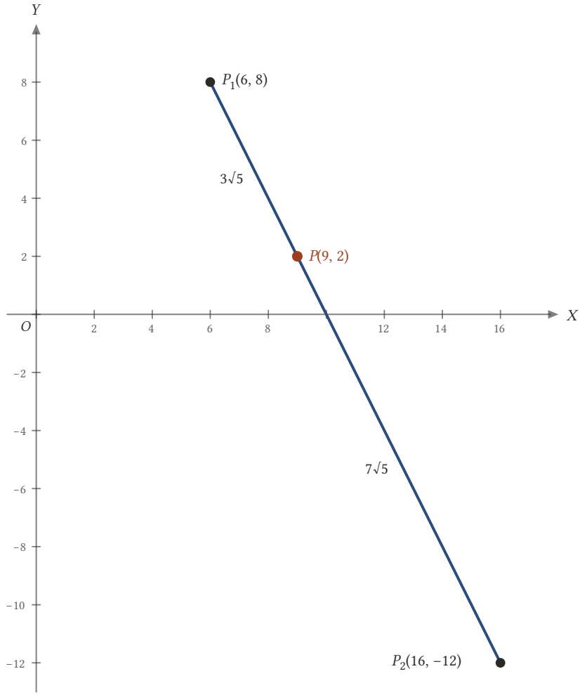
Şekil 2.28: P_1(6, 8) ile P_2(16, -12) arasındaki P(9, 2) noktası parçayı |P_1P| : |PP_2| = 3\sqrt{5} : 7\sqrt{5} = 3 : 7 oranında böler.
