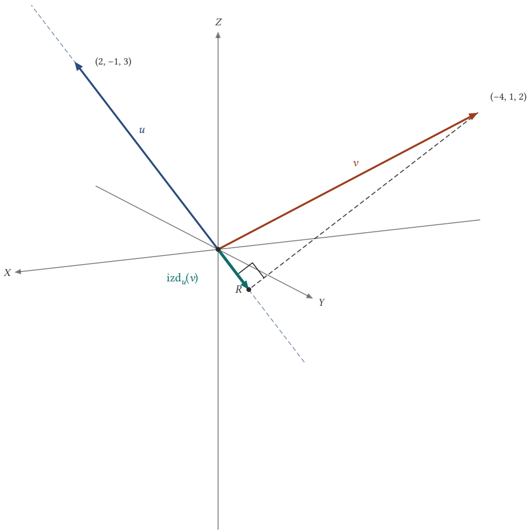
Şekil 8.10: v = (-4, 1, 2) 'nin u = (2, -1, 3) üzerine izdüşümü \text{izd}_u(v) = (-3/7, 3/14, -9/14) 'tür. İç çarpım negatif olduğundan izdüşüm u 'ya zıt yönlüdür ve u 'nun kesikli uzantısı üzerinde kalır.
