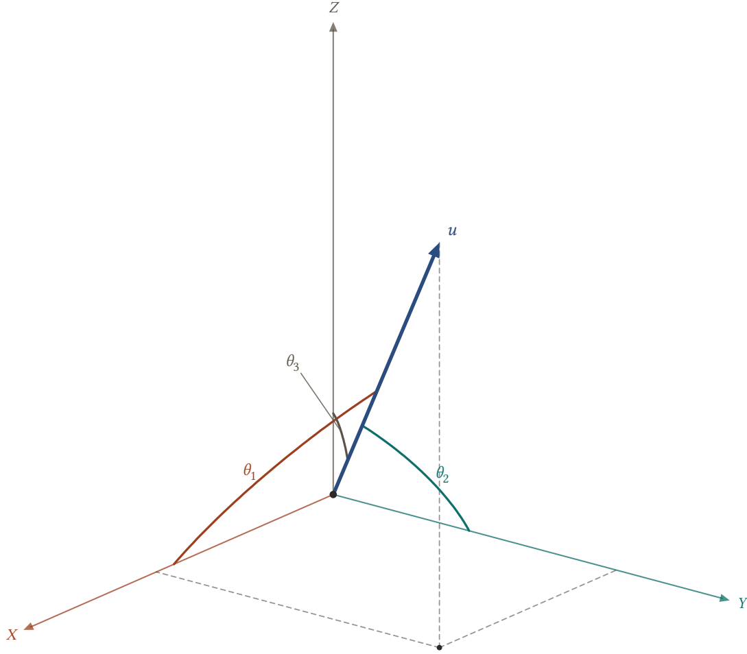
Şekil 8.12: u vektörünün doğrultu açıları: \theta_1 , \theta_2 , \theta_3 sırasıyla u 'nın X -, Y - ve Z -eksenlerinin pozitif yönleriyle yaptığı açılardır.
