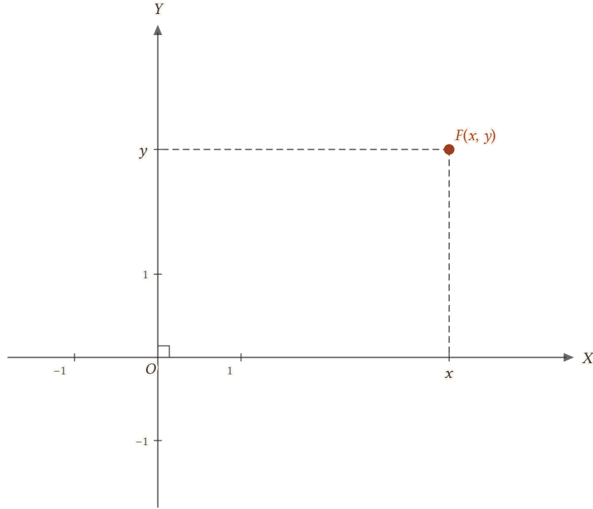
Şekil 1.2: Dik koordinat düzlemi. P den eksnlere inilen dikmeler X -eksenini x 'te, Y -eksenini y 'de keser; P nin dik koordinatları (x, y) 'dir.
