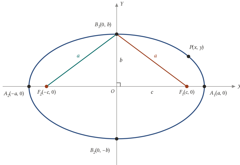
Şekil 18.6: Uzak köşeler (-a, 0) , (a, 0) ; yakın köşeler (0, \pm b) . B_1 'den iki odağa uzaklık a 'dır; OB_1F_1 dik üçgeni b^2 + c^2 = a^2 bağıntısını verir.
