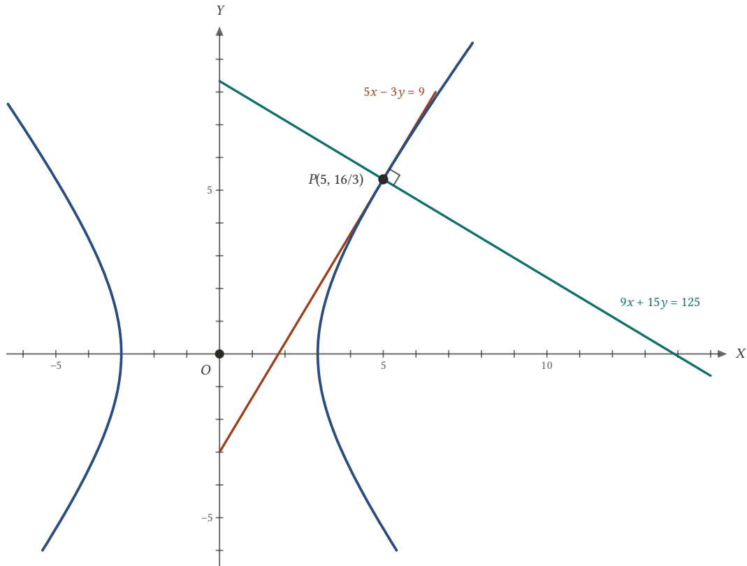
Şekil 19.12: P deki teğet ve normal birbirine diktir.
