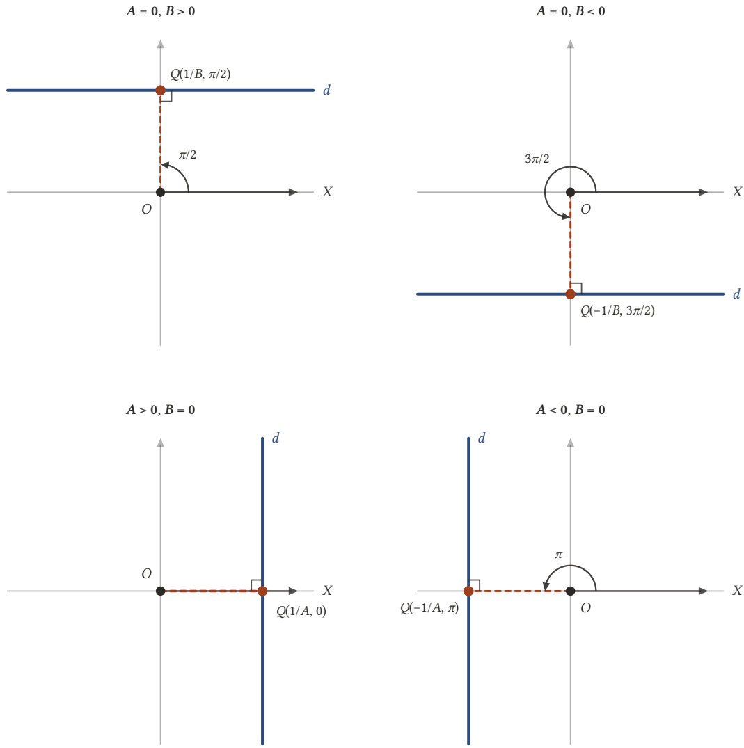
Şekil 5.15: A \cos \theta + B \sin \theta = 1/r doğrusunun dört özel durumu (örneklerde |A| ya da |B| = 1/2 ). Üst sıradaki ( A = 0 ) doğrular kutupsal eksene paralel, alt sıradaki ( B = 0 ) doğrular kutupsal eksene diktir.
