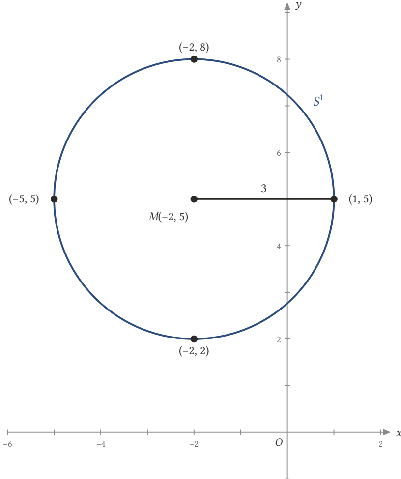
Şekil 4.3: Merkezi M(-2, 5) , yarıçapı 3 olan çember: (x + 2)^2 + (y - 5)^2 = 9 . Merkezden dört yöne 3 birim gidilerek çemberin dört noktası bulunur.
