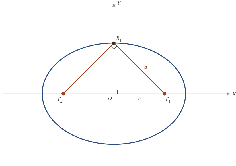
Şekil 18.31: B_1, F_2F_1 parçasını dik açı altında görür; OB_1F_1 ikizkenar dik üçgeninde \sin(\pi/4) = c/a = e = \sqrt{2}/2 .
