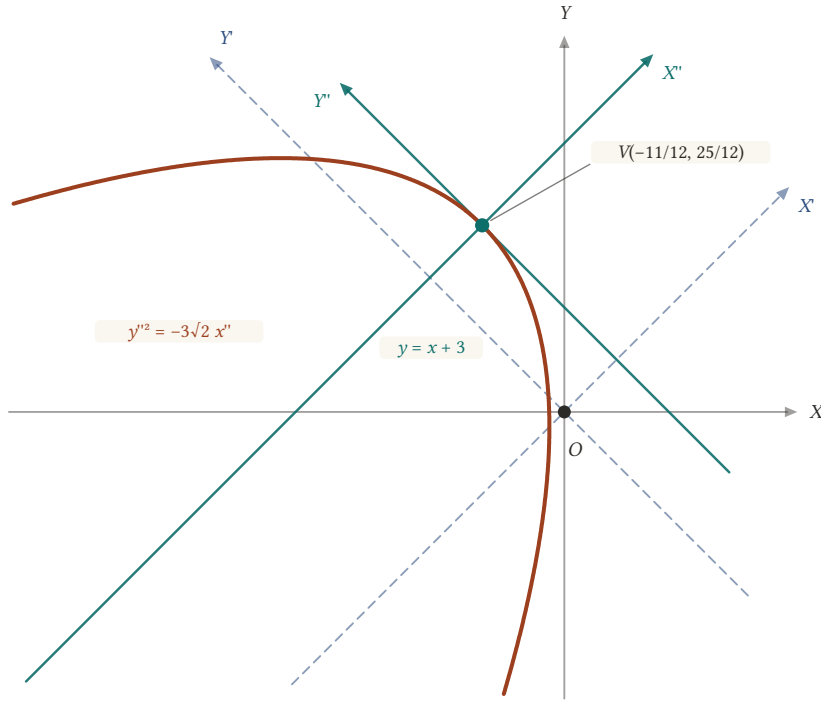
Şekil 21.3: Eksenler tepe noktasına ötelenince parabolün standart denklemi y''^2 = -3\sqrt{2} x'' elde edilir.
