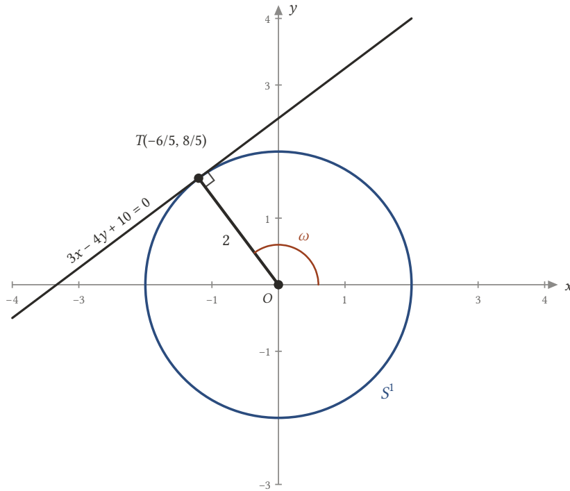
Şekil 4.25: Orijinin 3x - 4y + 10 = 0 doğrusuna uzaklığı 2'dir; merkezi orijin olan ve bu doğruya teğet çember x^2 + y^2 = 4 , değme noktası T(-6/5, 8/5) 'tir.
