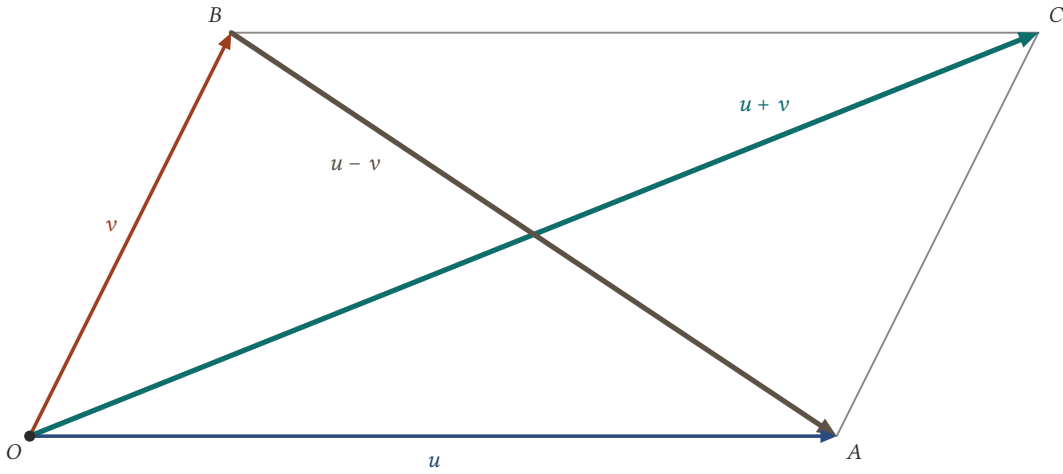
Şekil 8.16: Kenarları u ve v olan paralelkenarın köşegenleri u + v ve u - v 'dir. Köşegenlerin kareleri toplamı dört kenarın kareleri toplamına eşittir.
