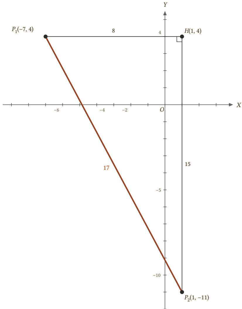
Şekil 1.22: Dik kenarları 8 ve 15 olan dik üçgenin hipotenüsü 17'dir.
