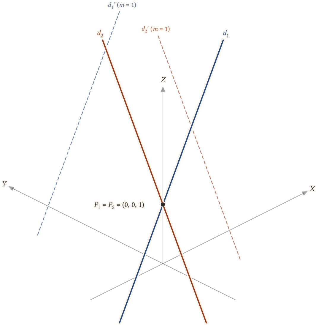
Şekil 11.8: m = 0 için d_1 ile d_2 (0, 0, 1) noktasında kesişir. Kesikli çizilen d_1' ve d_2' ise m = 1 için aynı doğrulardır; bunlar kesişmez, aykırıdır.
