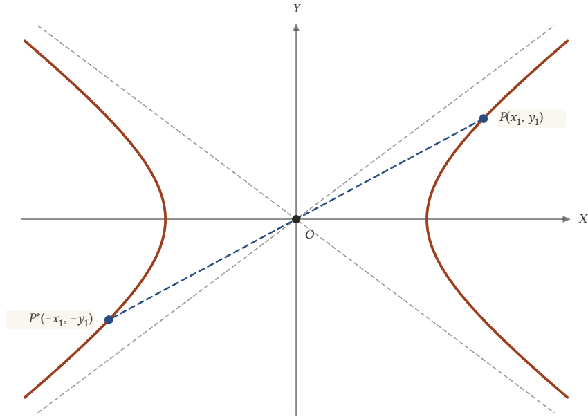
Şekil 21.8: Hiperbolün bir kolundaki her noktanın O 'ya göre simetriği öbür koldadır.
