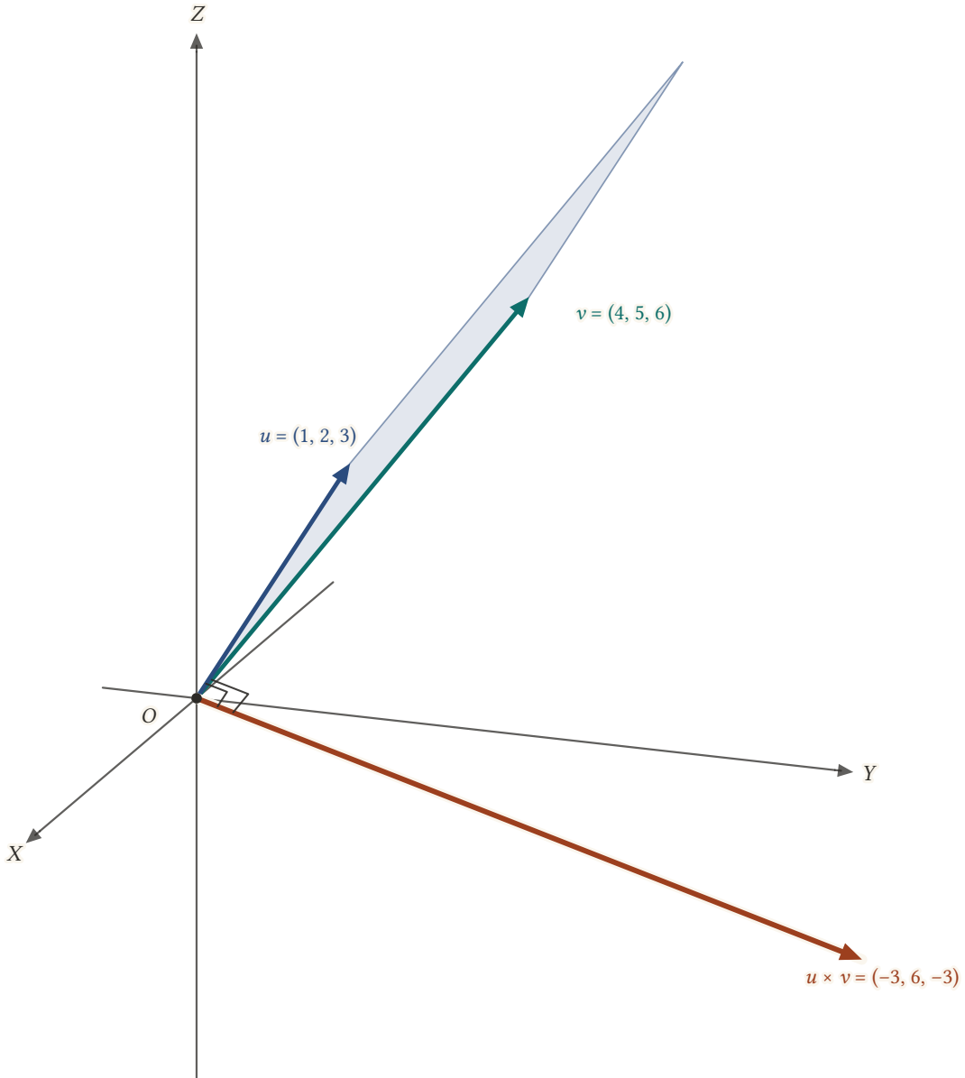
Şekil 9.2: u = (1, 2, 3) ve v = (4, 5, 6) vektörlerinin gerdiği paralelkenar ve u \times v = (-3, 6, -3) . Vektörel çarpım hem u 'ya hem v 'ye diktir, yani iki vektörün düzlemine diktir.
