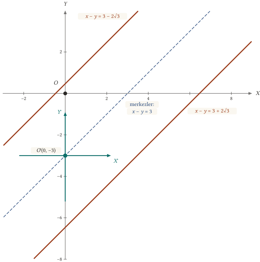
Şekil 21.20: d = D = 0 : konik paralel iki doğrudur ve (t, t - 3) biçimindeki her nokta bir merkezdır.
