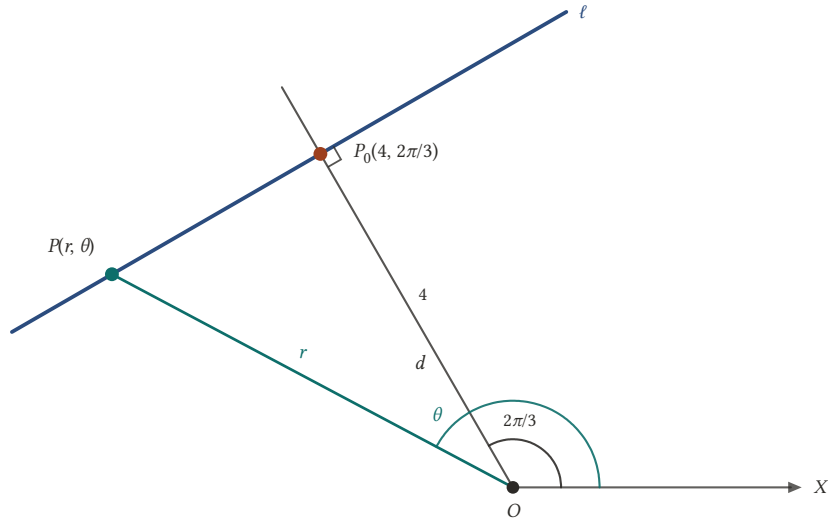
Şekil 5.27: OP_0 'a P_0 'da dik olan \ell doğrusu. Kutuptan \ell 'ye inilen dikmenin ayağı P_0 'ın kendisidir; denklem r \cos(\theta - 2\pi/3) = 4 .
