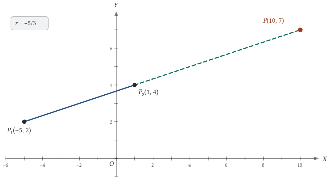
Şekil 2.9: r = -5/3 için bölünme noktası P(10, 7) , parçanın P_2 tarafındaki uzantısı (kesikli) üzerindedir.
