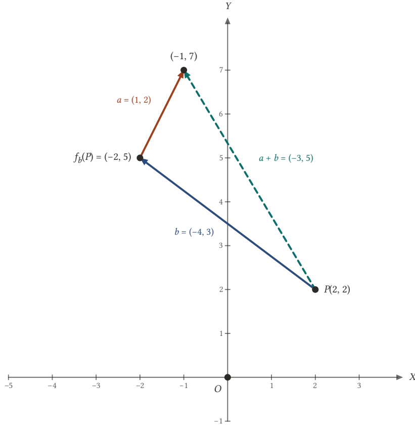
Şekil 16.4: P(2, 2) noktasına önce b = (-4, 3) , sonra a = (1, 2) ötelemesi uygulanır; sonuç, a + b = (-3, 5) ötelemesinin verdiği (-1, 7) noktasıdır.
