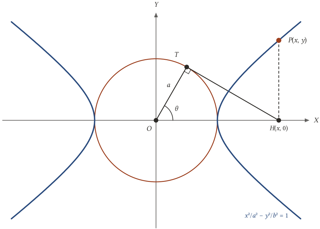
Şekil 19.16: OTH dik üçgeninde \cos \theta = a/x olduğundan x = a \sec \theta , y = b \tan \theta .
