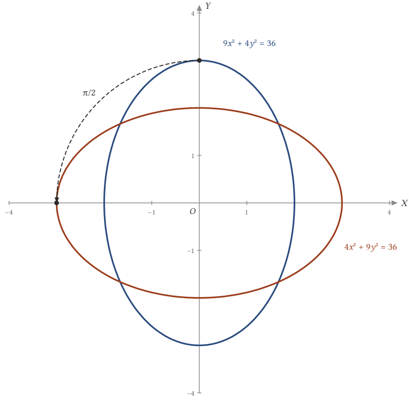
Şekil 18.33: 9x^2 + 4y^2 = 36 elipsi başlangıç noktası etrafında \pi/2 döndürülünce 4x^2 + 9y^2 = 36 elipsine gelir; (0, 3) noktası (-3, 0) noktasına taşınır.
