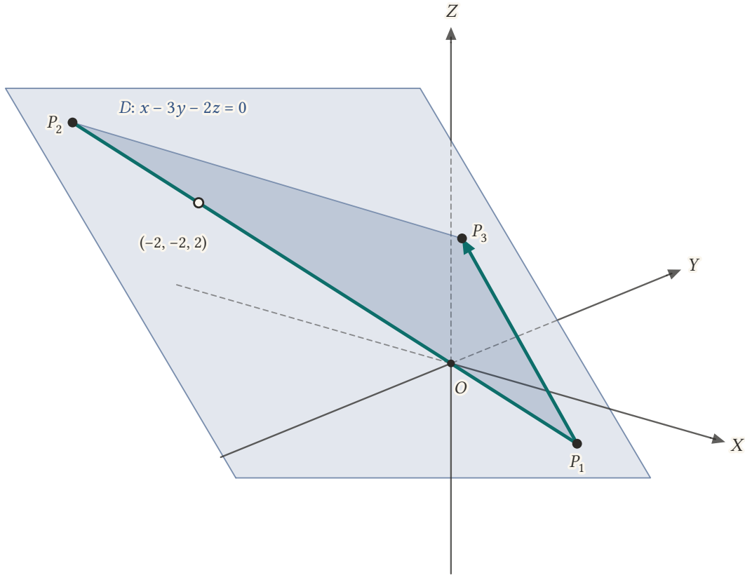
Şekil 12.21: P_1(1, 1, -1) , P_2(-3, -3, 3) , P_3(1, -1, 2) noktalarından geçen x - 3y - 2z = 0 düzlemi. Önceki örneğin (-2, -2, 2) noktası (boş daire) P_1P_2 doğrusu üzerindedir.
