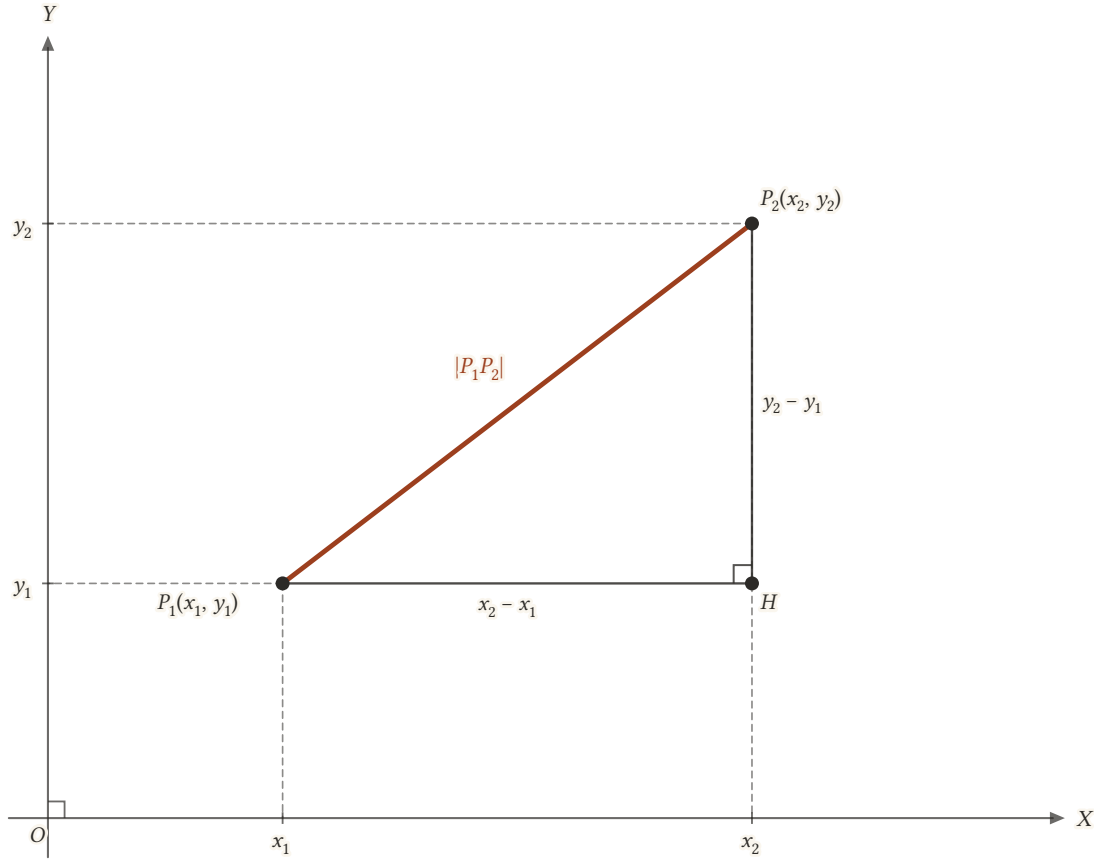
Şekil 1.6: P_1HP_2 dik üçgeninin dik kenarları |x_2 - x_1| ve |y_2 - y_1| 'dir; hipotenüs |P_1P_2| Pisagor bağıntısıyla bulunur.
