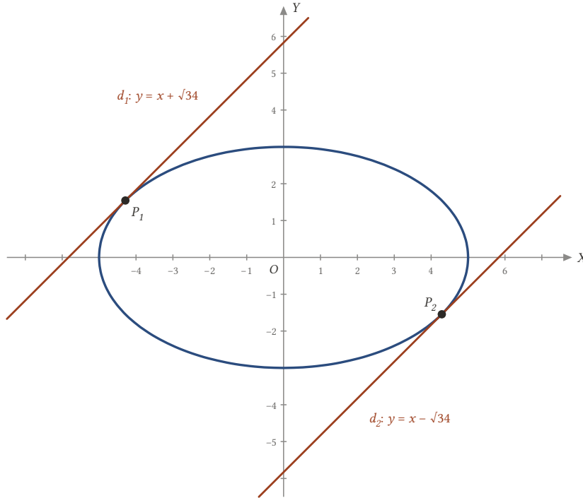
Şekil 18.17: y = x \pm \sqrt{34} doğruları x^2/25 + y^2/9 = 1 elipsine P_1(-25/\sqrt{34}, 9/\sqrt{34}) ve P_2(25/\sqrt{34}, -9/\sqrt{34}) noktalarında teğettir.
