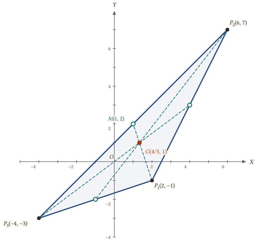
Şekil 1.31: Kenarortaylar G(4/3, 1) 'de kesişir; P_1M kenarortayında |P_1G| = 2|GM| 'dir.
