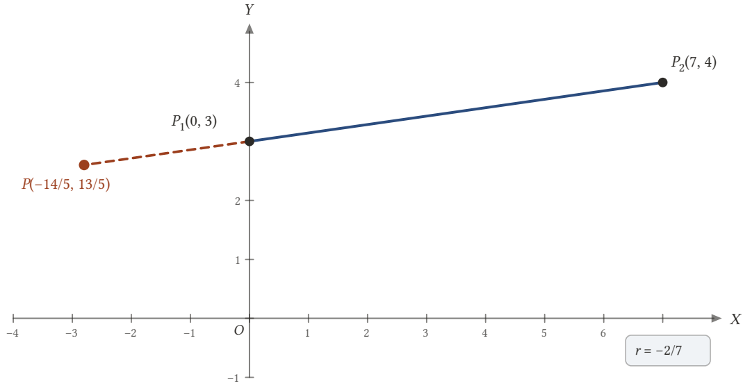
Şekil 2.7: r = -2/7 için bölünme noktası P(-14/5, 13/5) , parçanın P_1 tarafındaki uzantısı (kesikli) üzerindedir.
