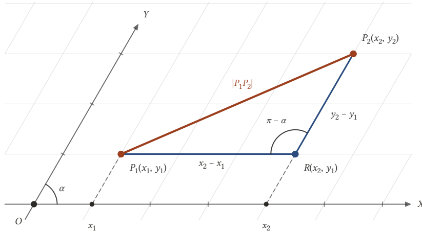
Şekil 5.20: Eğik sistemde uzaklık: P_1RP_2 üçgeninin kenarları |x_2 - x_1| ve |y_2 - y_1| , R 'deki açı \pi - \alpha 'dır; kosinüs teoremi uzaklığı verir.
