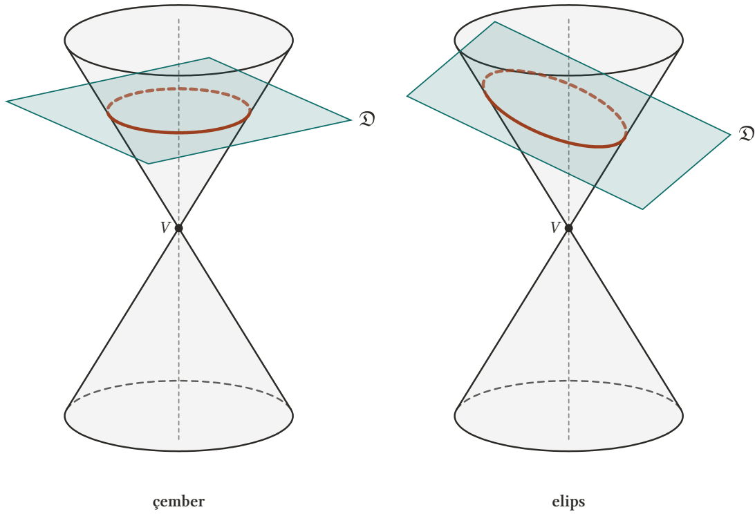
Şekil 18.1: Eksene dik bir düzlem koniyi çember boyunca, ana doğrulardan daha yatık bir düzlem ise kapalı bir eğri olan elips boyunca keser.
