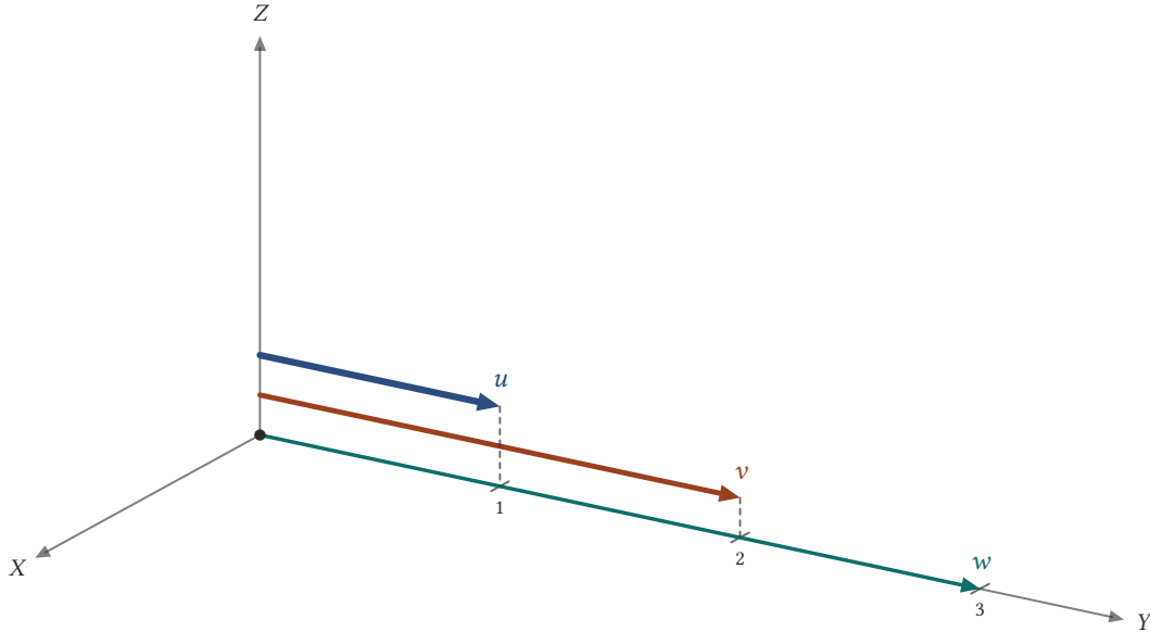
Şekil 8.21: u = (0, 1, 0) , v = (0, 2, 0) , w = (0, 3, 0) hepsi Y -ekseninin pozitif kısmı üzerindedir; aynı doğrultu ve yöndedirler. Görünsünler diye oklar biraz yukarı kaydırılarak çizilmiştir.
