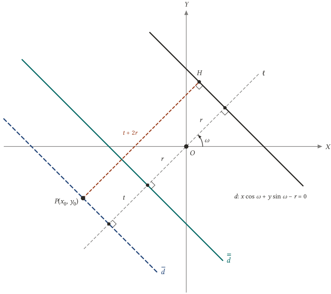
Şekil 3.12: İkinci konum: P orijinle aynı taraftadır ve orijinin ötesindedir. Yeşil doğru d'nin orijine göre simetriğidir; P'den geçen paralel \bar{d} ondan t kadar ötededir ve P'nin d'ye uzaklığı t + 2r'dir.
