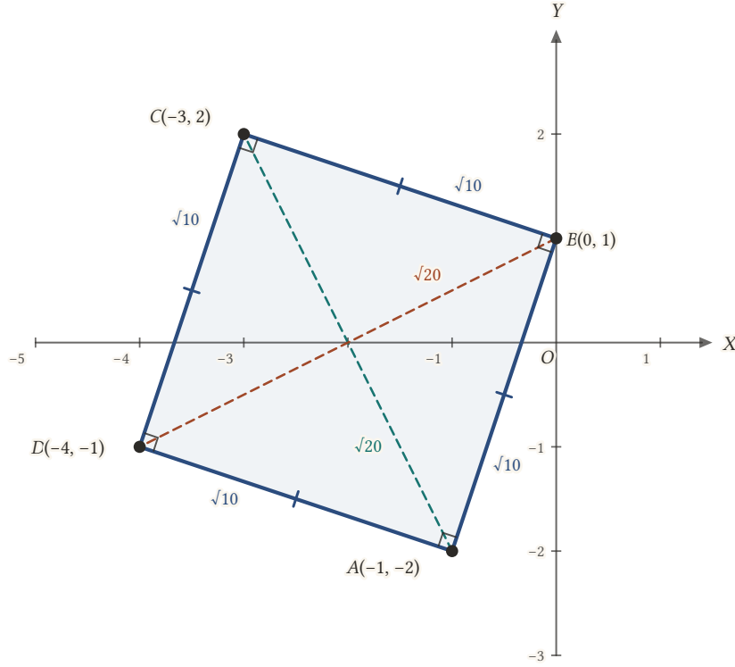
Şekil 1.17: Dört kenarı \sqrt{10} , iki köşegeni \sqrt{20} olan ABCD bir karedir.
