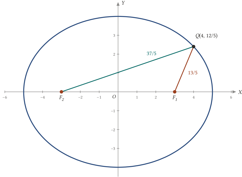
Şekil 18.5: Q(4, 12/5) noktasının odaklara uzaklıkları 13/5 ve 37/5 'tir; toplamı 10 = 2a olduğundan Q , x^2/25 + y^2/16 = 1 elipsinin üzerindedir.
