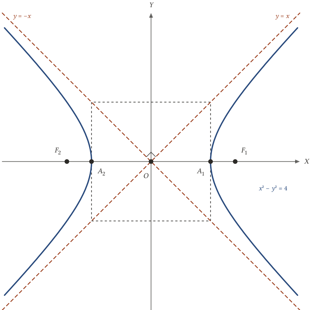
Şekil 19.8: İkizkenar hiperbolde temel dikdörtgen karedir ve asimptotlar birbirine diktir.
