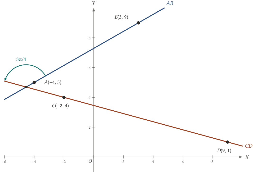
Şekil 2.29: A(-4, 5) ve B(3, 9) 'den geçen doğrudan C(-2, 4) ve D(9, 1) 'den geçen doğruya yönelmiş açı 3\pi/4 'tür.
