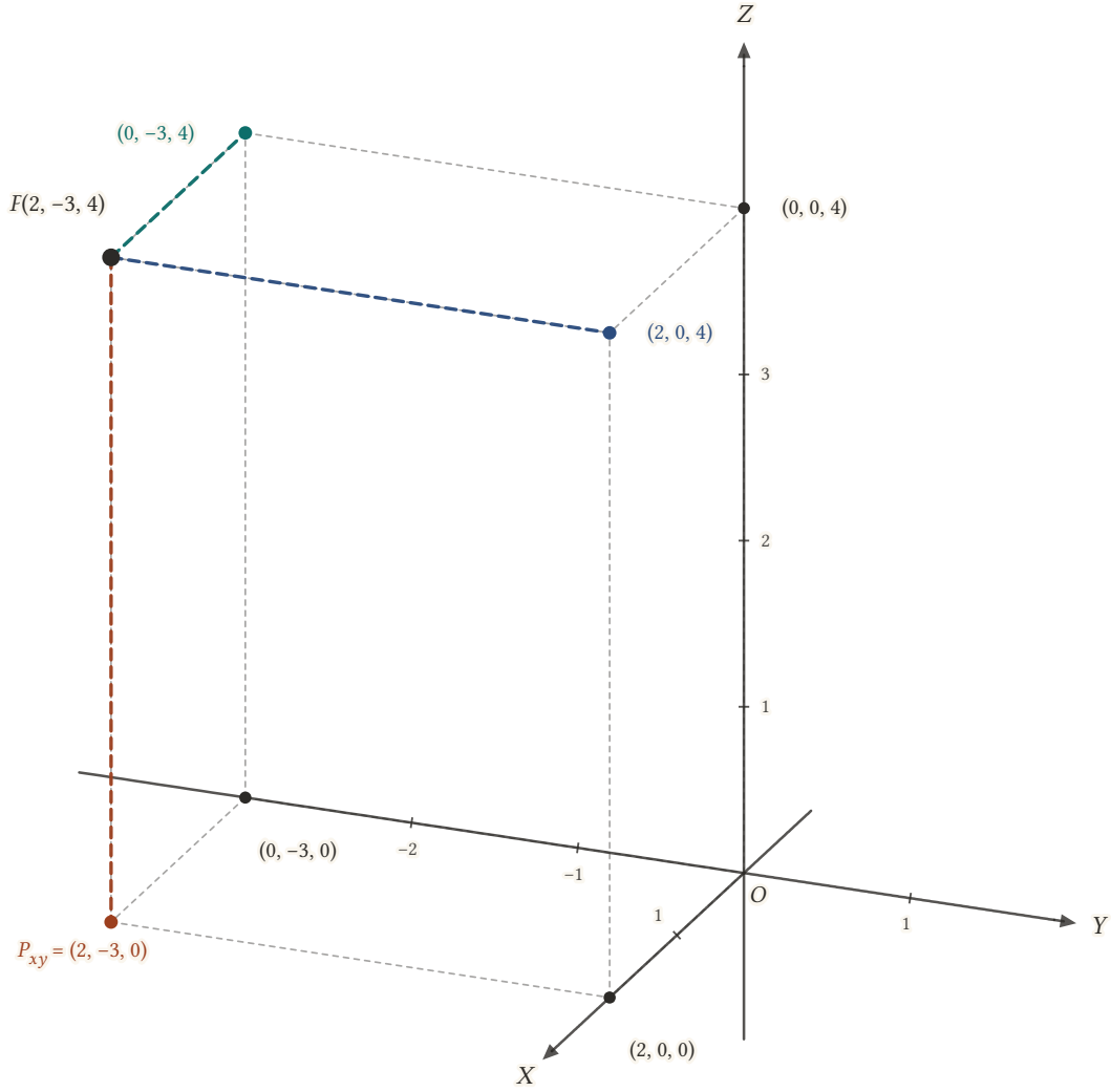
Şekil 6.5: P(2, -3, 4) noktası ve kenarları eksenlere paralel prizma. Renkli kesikli çizgiler P 'den XY -, YZ - ve XZ -düzlemlerine inilen dikmelerdir; eksenler üzerindeki üç nokta, eksenlere inilen dikmelerin ayaklarıdır.
