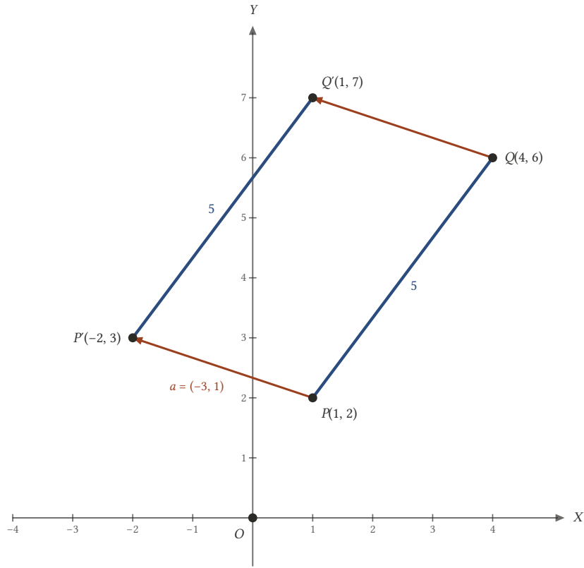
Şekil 16.6: a = (-3, 1) ötelemesinden önce ve sonra iki nokta arasındaki uzaklık 5'tir.
