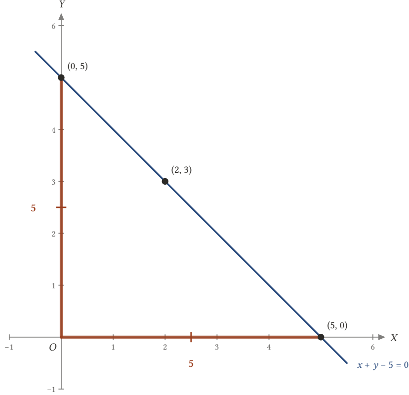
Şekil 3.21: (2, 3) 'ten geçen ve eksenlerin pozitif yarılarından eşit parçalar ayıran doğru x + y - 5 = 0 'dır; iki parçanın uzunluğu da 5'tir.
