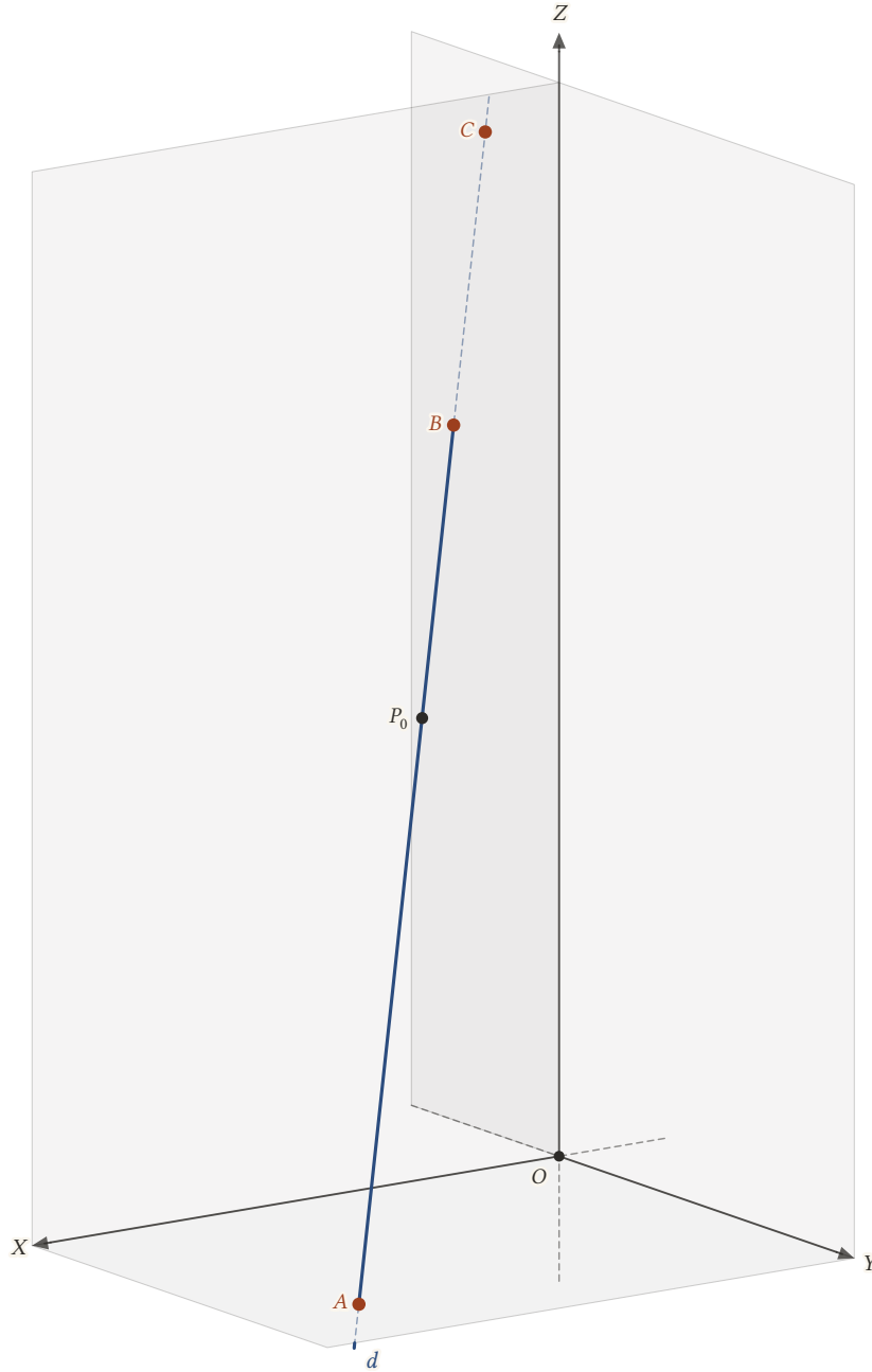
Şekil 10.4: d doğrusu YZ düzlemini C 'de, XZ düzlemini B 'de, XY düzlemini A 'da keser; parametre değerleri sırasıyla -2, -1, 2 'dir, P_0 ise \lambda = 0 noktasıdır.
