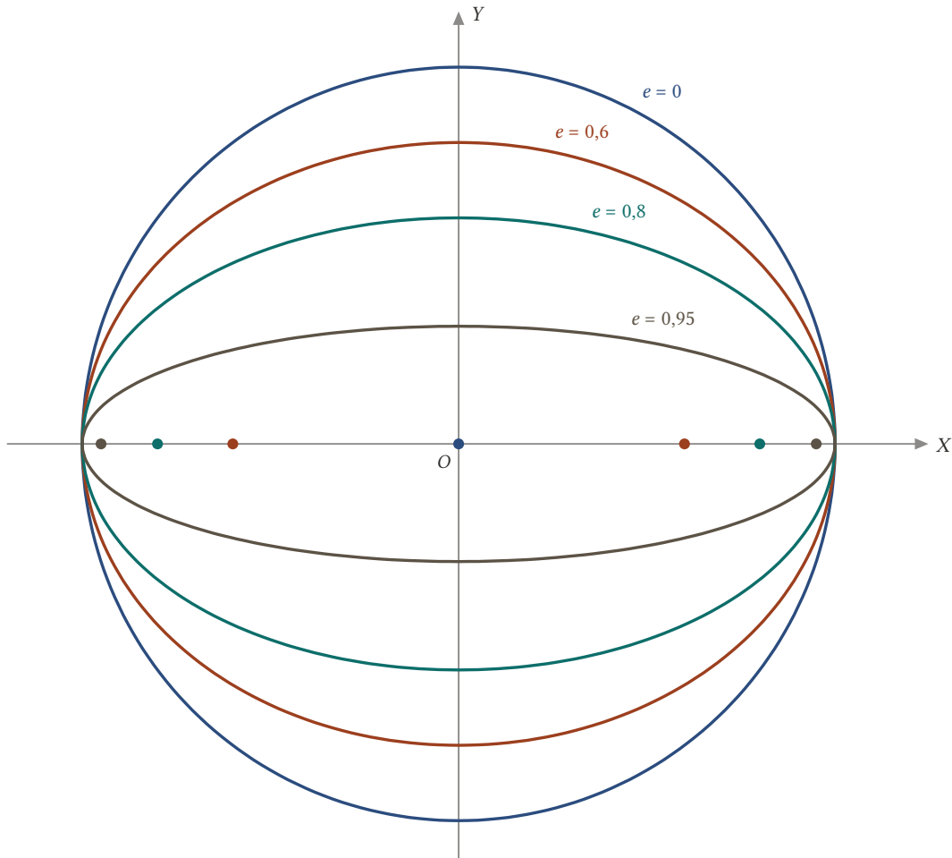
Şekil 18.19: Asal yarı eksen a = 5 olan elipsler: e büyüdükçe odaklar (\pm 5e, 0) uzak köşelere yaklaşır ve elips basıklaşır; e = 0 çemberdir.
