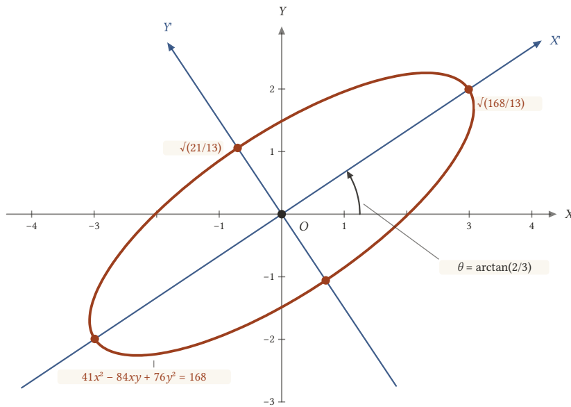
Şekil 21.15: Eksenler \arctan(2/3) döndürülünce elipsin denklemi 13x'^2 + 104y'^2 = 168 olur.
