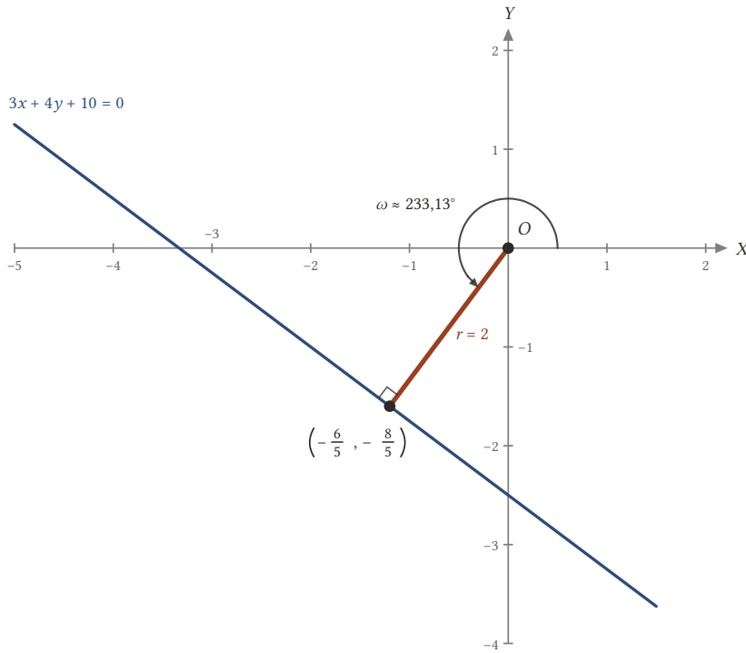
Şekil 3.10: 3x + 4y + 10 = 0 doğrusu: dikmenin ayağı (-6/5, -8/5) üçüncü bölgededir, r = 2 ve \omega = \pi + \arctan(4/3) \approx 233,13^\circ .
