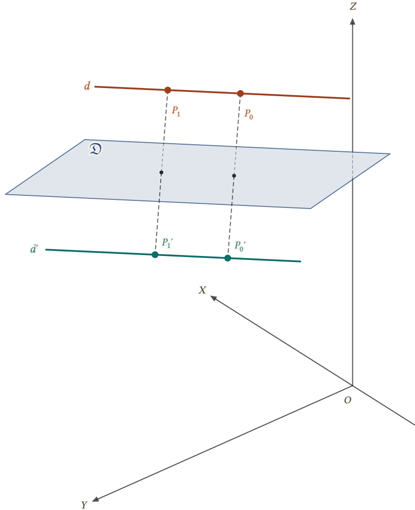
Şekil 15.12: x - y + z - 3 = 0 düzlemine paralel d doğrusu (turuncu) ve simetriği d' (yeşil). İki doğru da (1, 1, 0) doğrultusundadır ve düzlemin iki yanında, ona \sqrt{3} uzaklıktadır; kesikli dikmelerin ayakları (0, 3, 6) ve (1, 4, 6) 'dir.
