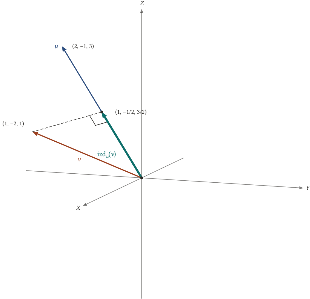
Şekil 8.11: v = (1, -2, 1) 'nin u = (2, -1, 3) üzerine izdüşümü \text{izd}_u(v) = (1, -1/2, 3/2) 'dir; dikmenin ayağı u 'nun tam ortasına düşer.
