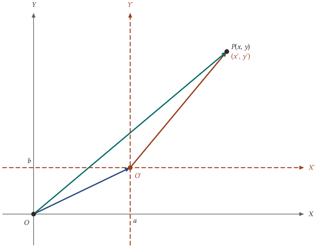
Şekil 16.8: Eksenler \overrightarrow{OO'} = (a, b) kadar ötelenir; \overrightarrow{OP} = \overrightarrow{OO'} + \overrightarrow{O'P} eşitliğinden x = x' + a , y = y' + b çıkar.
