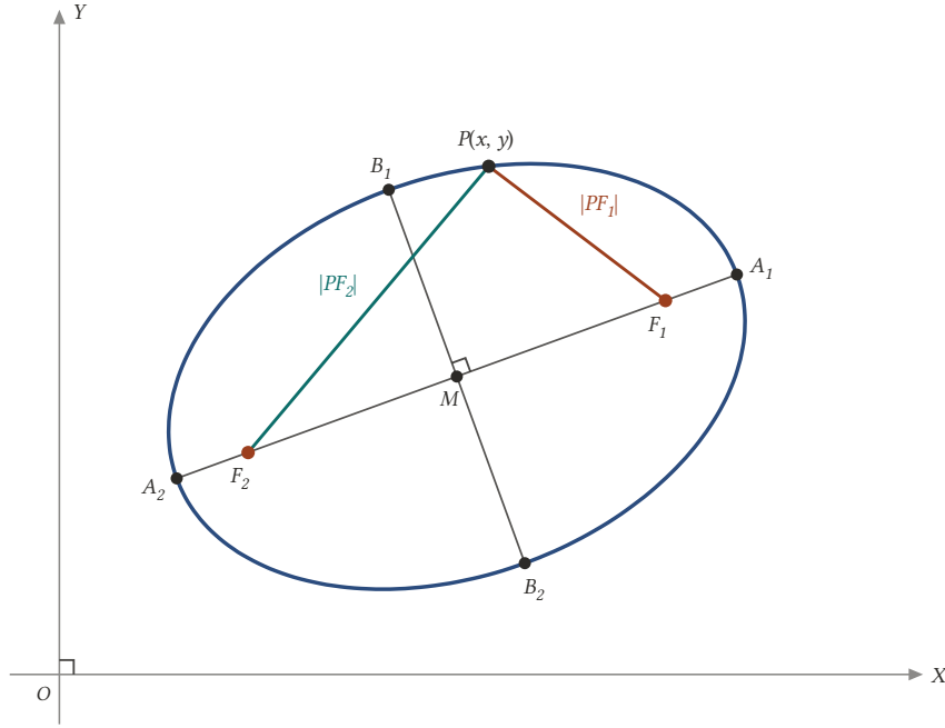
Şekil 18.4: F_1 ve F_2 odaklı elips: her P noktası için |PF_1| + |PF_2| = 2a . A_1A_2 ve B_1B_2 elipsin merkezi M 'de dik kesişen eksenlerdir.
