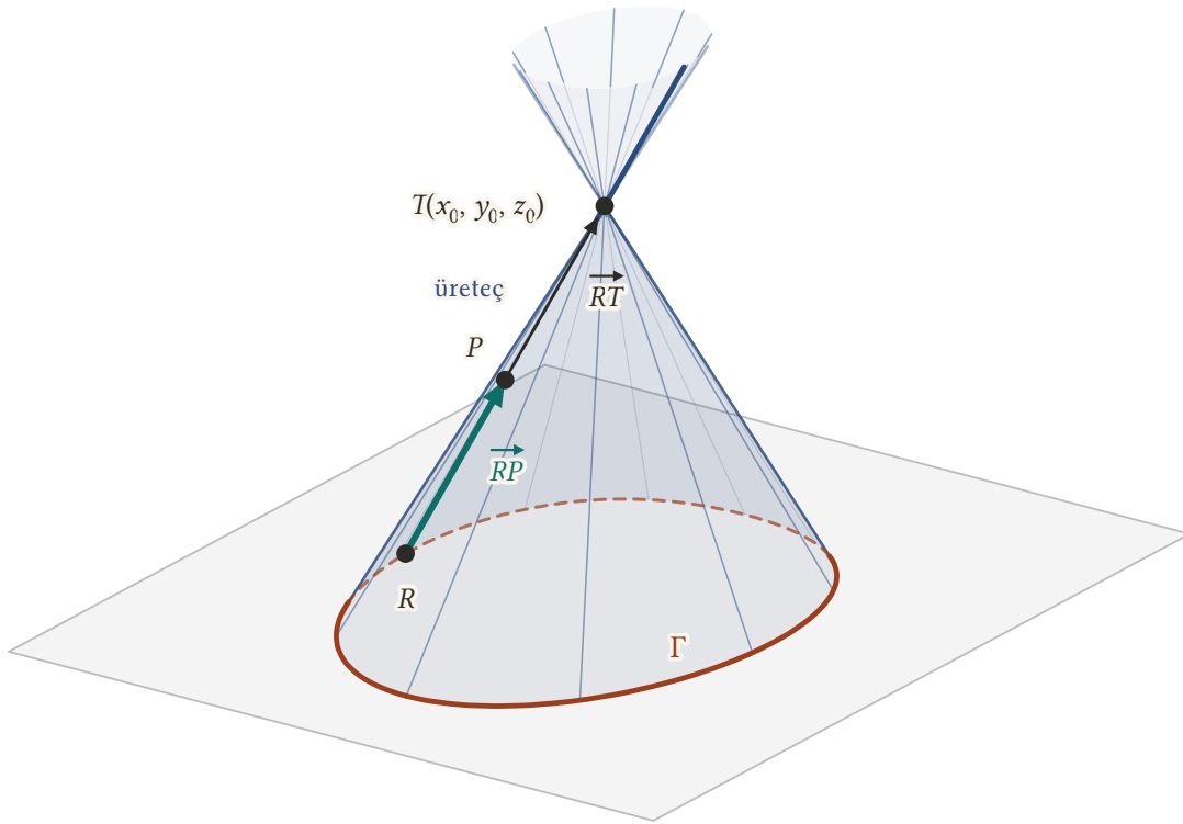
Şekil 23.8: Koni: dayanak eğrisi \Gamma (kırmızı) üzerindeki her noktayı T tepe noktasına birleştiren doğrular (üreteçler) yüzeyi örер; üreteçler T 'nin ötesine uzanarak öbür kanadı (soluk) oluşturur. R \in \Gamma ve P , RT üreteci üzerindeyken RP = \lambda RT olur.
