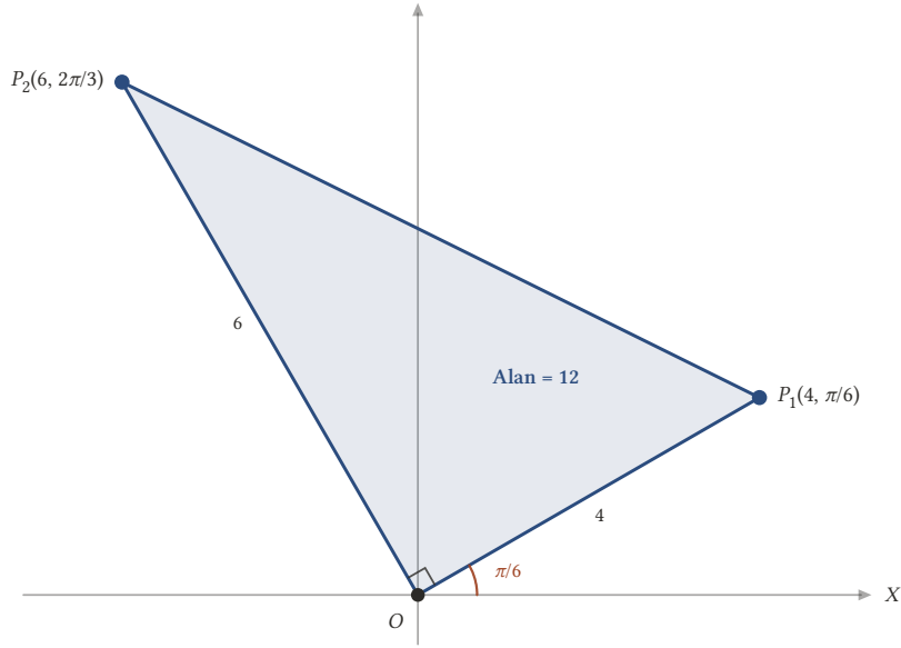
Şekil 5.13: O, P_1(4, \pi/6), P_2(6, 2\pi/3) üçgeni: açılar farkı \pi/2 olduğundan üçgen O 'da dik açıdır ve alanı 12'dir.
