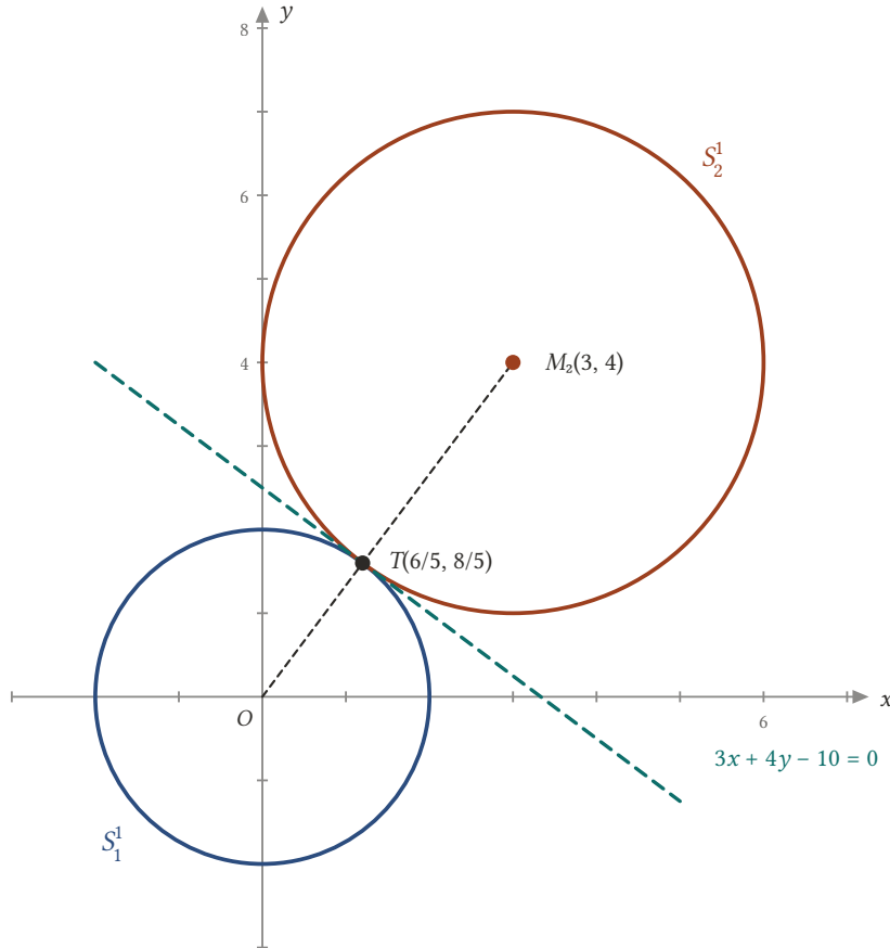
Şekil 4.22: x^2 + y^2 = 4 ile (x - 3)^2 + (y - 4)^2 = 9 çemberleri dıştan teğettir. Değme noktası T(6/5, 8/5) merkezleri birleştiren parça üzerindedir; ortak teğet 3x + 4y - 10 = 0 'dır.
