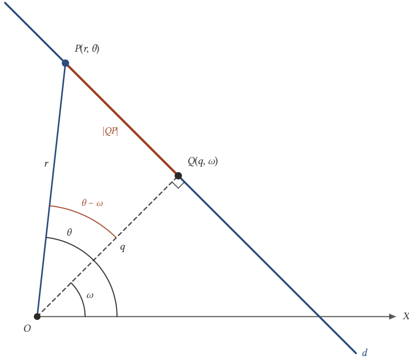
Şekil 5.14: Kutupsal doğru denklemi: Q(q, \omega) kutuptan d 'ye inilen dikmenin ayağıdır. OQP üçgeni Q 'da dik açı olduğu için r \cos(\theta - \omega) = q olur.
