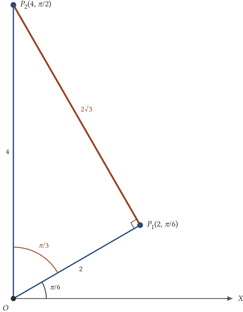
Şekil 5.11: P_1(2, \pi/6) ile P_2(4, \pi/2) arasındaki açı \pi/3 'tür ve uzaklık 2\sqrt{3} çıkar; üçgen P_1 'de dik açıdır.
