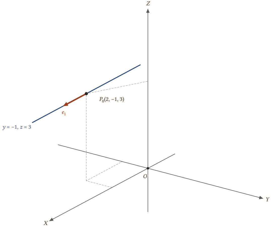
Şekil 12.16: P_0(2, -1, 3) noktasından geçen ve X -eksenine paralel olan doğru; doğrultmanı e_1 'dir.
