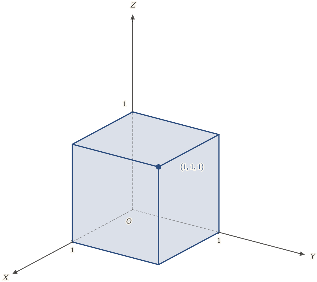
Şekil 6.10: Birim küp: 0 \leq x, y, z \leq 1 . O 'da buluşan üç ayrıtı eksenler üzerindedir ve arkada kaldıkları için kesiklidir; görünen üç yüz x = 1 , y = 1 ve z = 1 yüzleridir.
