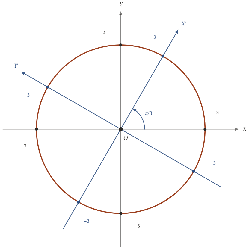
Şekil 17.12: x^2 + y^2 = 9 çemberi eksenler \pi/3 döndürüldükten sonra da x'^2 + y'^2 = 9 denklemiyle anlatılır.
