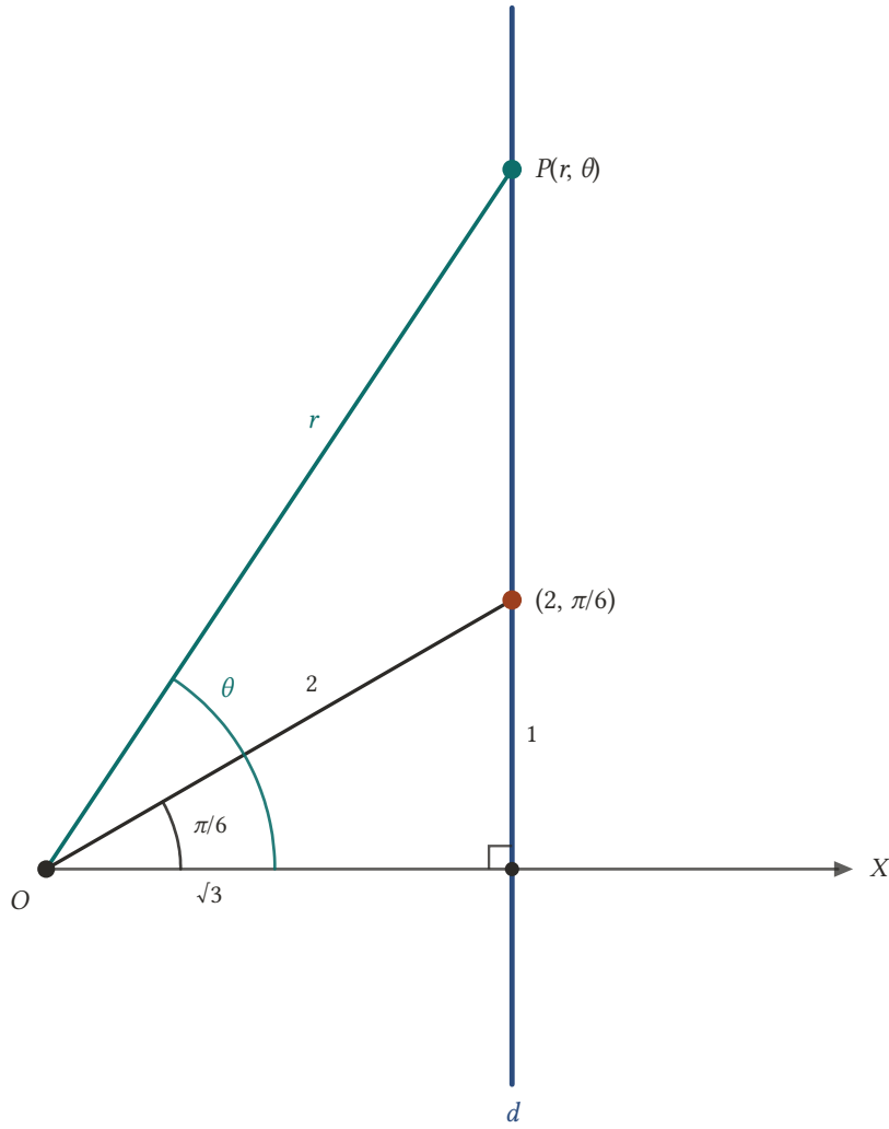
Şekil 5.17: (2, \pi/6) noktasından geçen ve OX e dik d doğrusu: OHK dik üçgeninden |OH| = \sqrt{3} , OHP dik üçgeninden r \cos \theta = \sqrt{3} .
