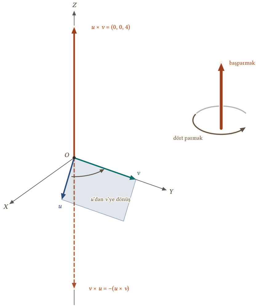
Şekil 9.5: Sağ el kuralı: sağ elin dört parmağı u'dan v'ye doğru kıvrıldığında başparmak u \times v = (0, 0, 4) 'ün yönünü gösterir (sağdaki şema). Çarpınların sırası değişince sonuç ters yöne döner: v \times u = (0, 0, -4) .
