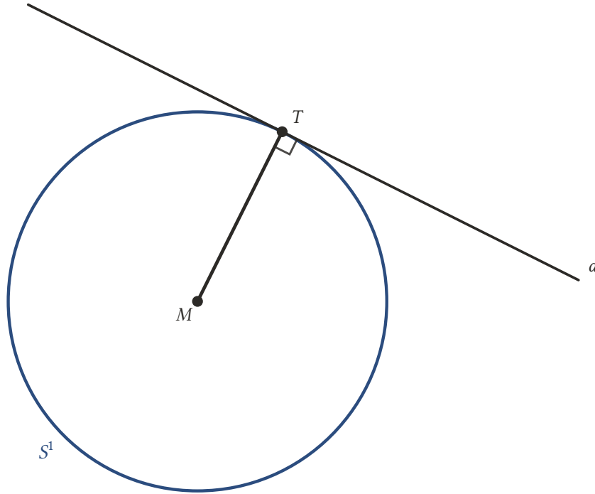
Şekil 4.11: Teğet d , değme noktası T 'deki MT yarıçapına diktir.
