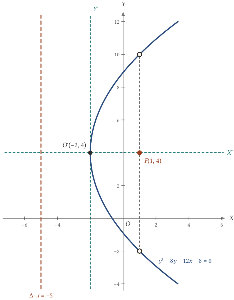
Şekil 20.15: Köşe O'(-2, 4) 'e öteleme denklemi y'^2 = 12x' yapar; odak F(1, 4) , doğrultman x = -5 .
