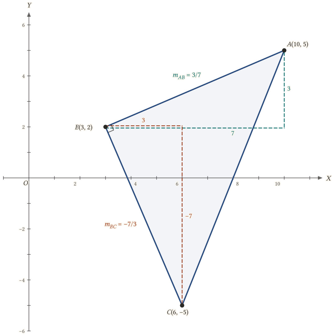
Şekil 1.33: Eğim üçgenleri: m_{AB} = 3/7 ve m_{BC} = -7/3 ; çarpımları -1 olduğundan AB \perp BC dir.
