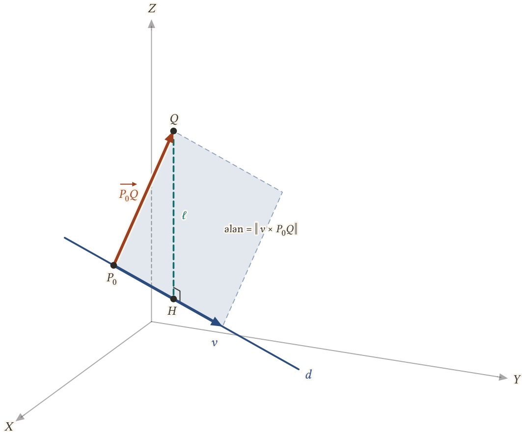
Şekil 11.4: v ile P_0Q vektörlerinin gerdiği paralelkenarın alanı \|v \times P_0Q\| , tabanı \|v\| , yüksekliği \ell = |QH| 'dir; bu yüzden \ell = \|v \times P_0Q\| / \|v\| .
