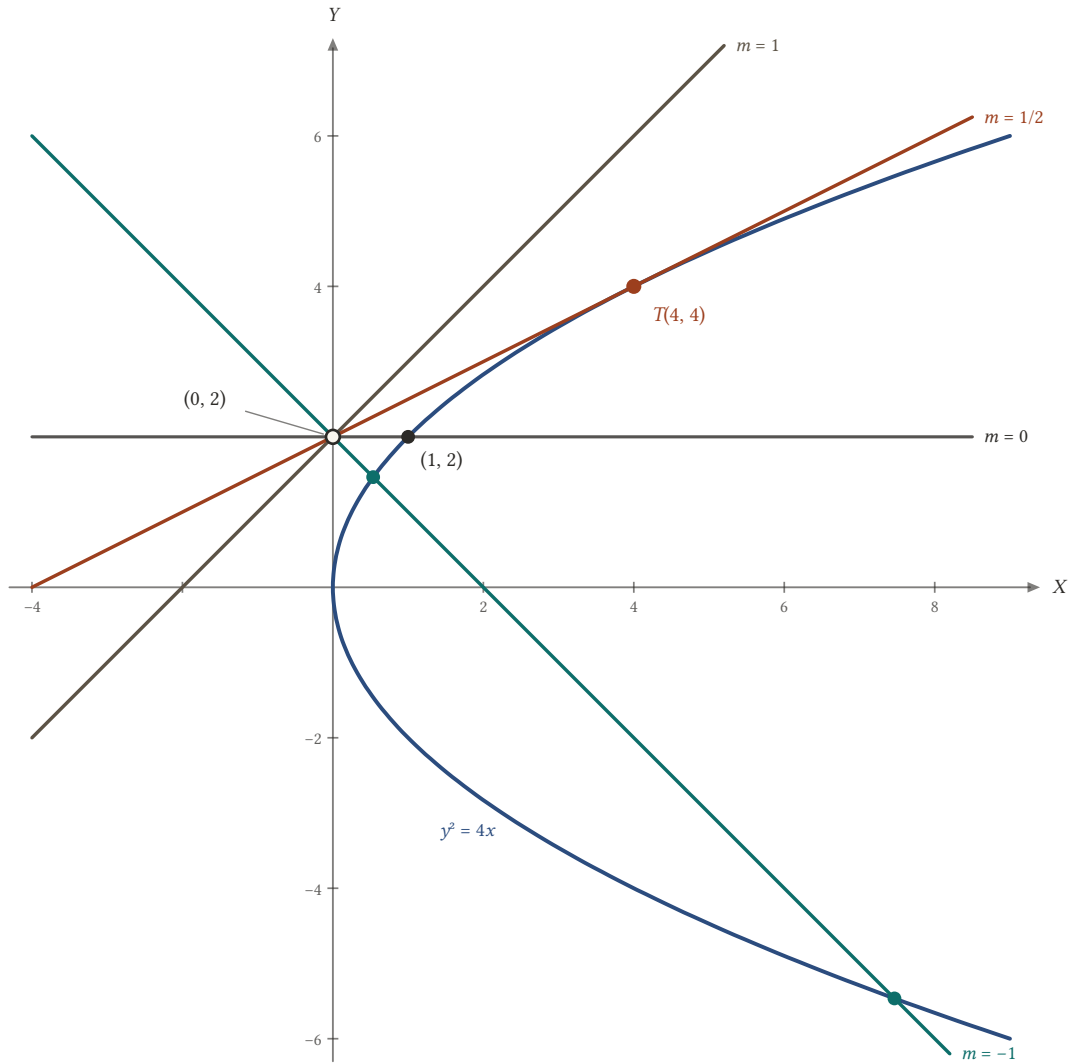
Şekil 20.17: y = mx + 2 doğruları: m > 1/2 kesmez, m = 1/2 teğet, m < 1/2 ( m \neq 0 ) iki noktada keser; m = 0 eksene paraleldir ve tek noktada keser.
