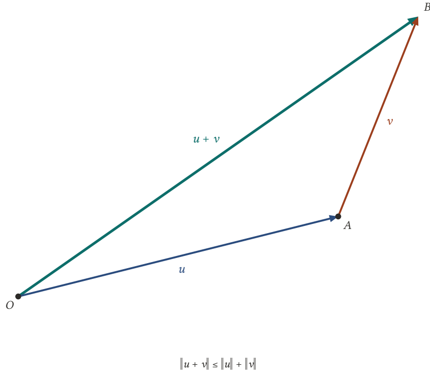
Şekil 8.1: u ile v uca eklenince u + v üçgenin üçüncü kenarı olur. Bu kenarın uzunluğu öteki iki kenarın uzunlukları toplamını aşamaz: \|u + v\| \leq \|u\| + \|v\| .
