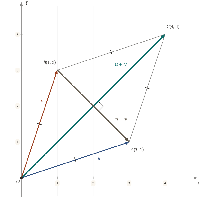
Şekil 8.19: u = (3, 1) ve v = (1, 3) eşit uzunlukludur; üzerlerine kurulan paralelkenar bir eşkenar dörtgendir. Köşegenleri u + v = (4, 4) ile u - v = (2, -2) birbirine diktir.
