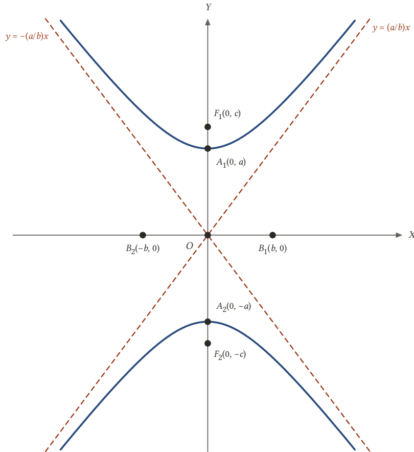
Şekil 19.6: Odakları Y-ekseninde olan hiperbol: kollar yukarı ve aşağı açılır.
