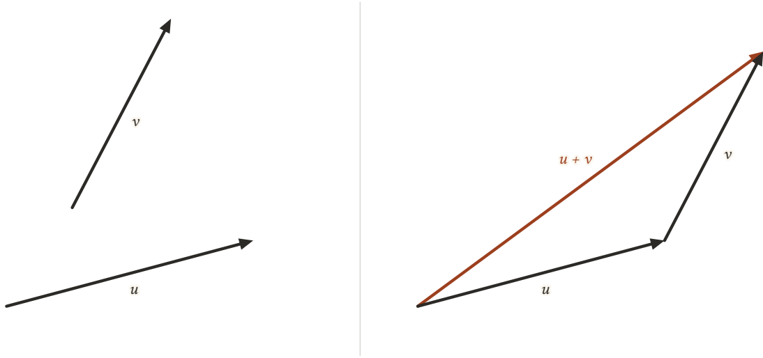
Şekil 7.8: Solda u ve v ; sağda v , u 'nun ucundan başlatılmıştır ve u 'nun başlangıcından v 'nin ucuna giden ok u + v 'dir.
