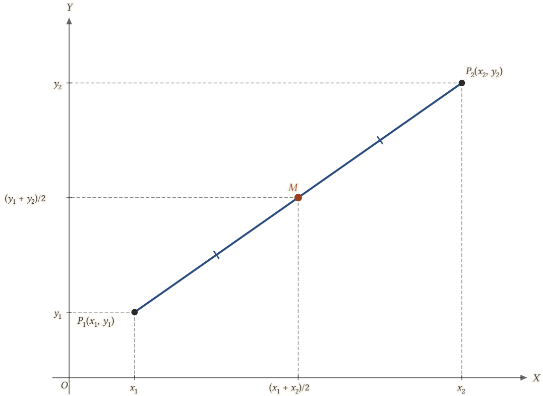
Şekil 1.27: Orta nokta: M 'nin koordinatları uç noktaların koordinatlarının ortalamasıdır ve |P_1M| = |MP_2| 'dir.
