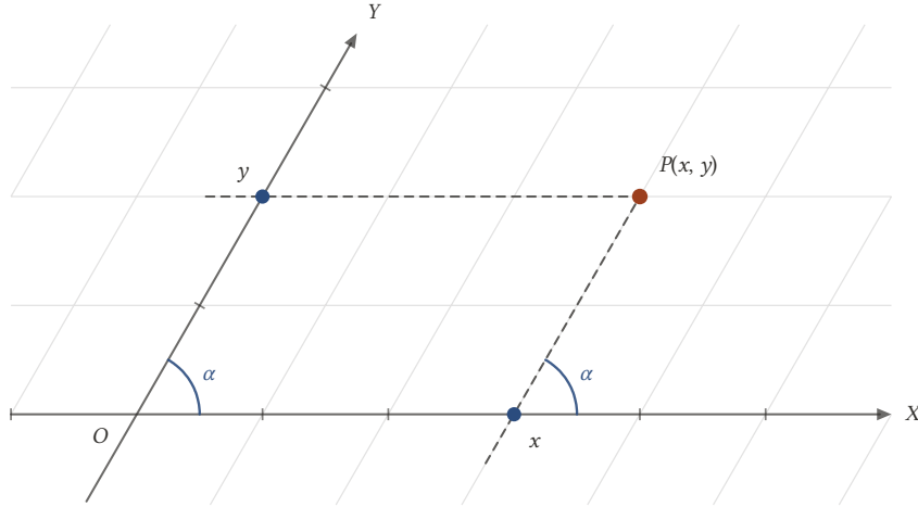
Şekil 5.1: Paralel koordinat sistemi: eksenler arasındaki açı \alpha . P den eksenlere paralel çizilen kesikli doğrular X -eksenini x 'te, Y -eksenini y 'de keser; P 'nin koordinatları (x, y) olur. Soluk ızgara çizgileri de eksenlere paraleldir.
