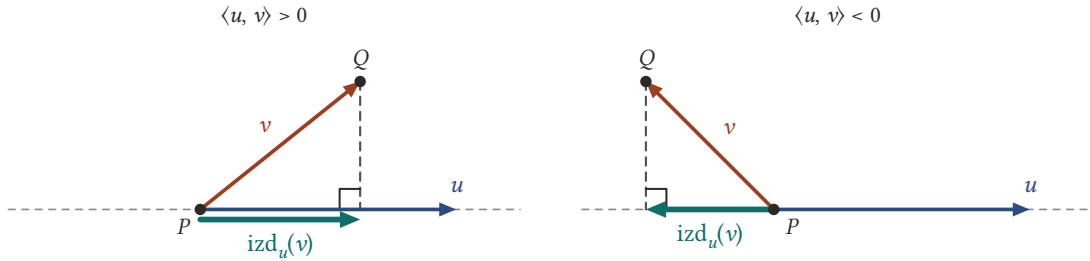
Şekil 8.8: Solda \langle u, v \rangle > 0 : izdüşüm u ile aynı yönlüdür. Sağda \langle u, v \rangle < 0 : izdüşüm u ile zıt yönlüdür.
