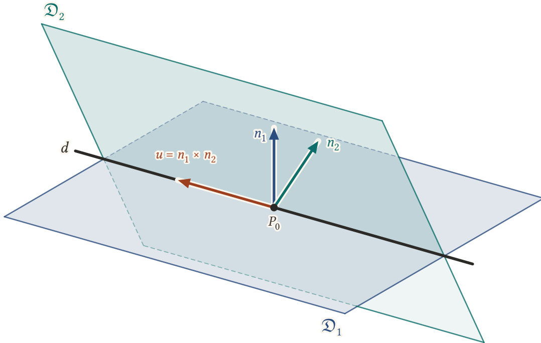
Şekil 13.3: Kesişen iki düzlem ortak bir d doğrusu boyunca buluşur. d , iki düzlemde de yattığı için iki normale de diktir; doğrultusu u = n_1 \times n_2 'dir. Düzlemlerin birbirinin arkasında kalan kenarları kesiklidir.
