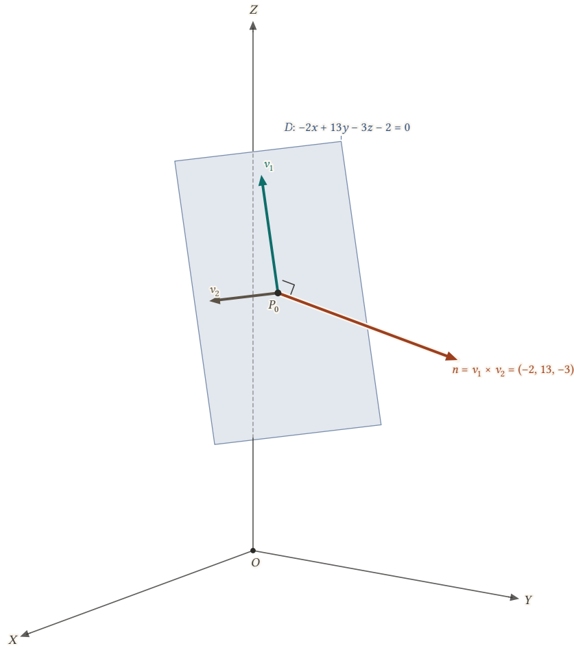
Şekil 12.7: -2x + 13y - 3z - 2 = 0 düzleminin kenarları v_1 ve v_2 doğrultusunda olan bir parçası ve normali n = v_1 \times v_2 = (-2, 13, -3) (0,15 katı çizildi).
