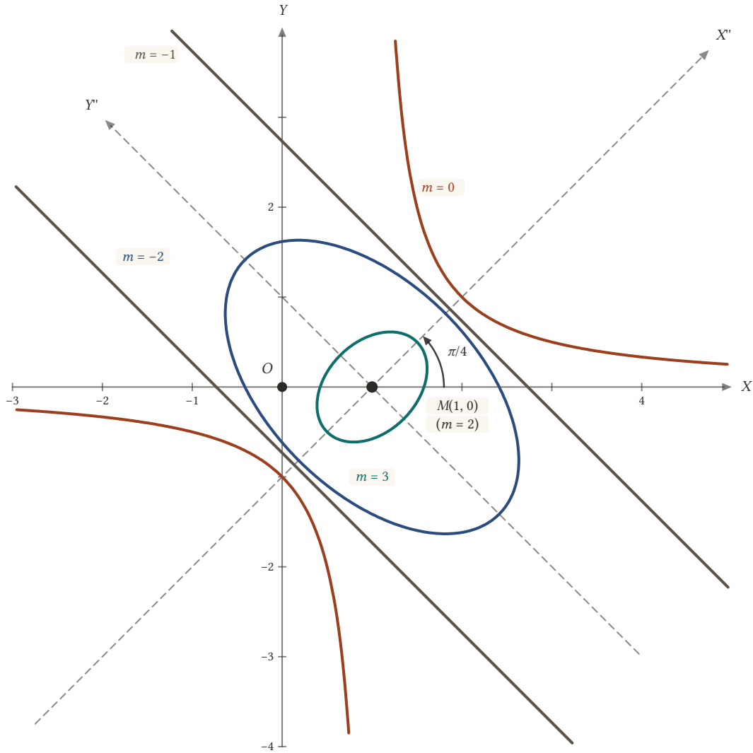
Şekil 21.10: mx^2 - 2xy + my^2 - 2mx + 2y + 2 = 0 ailesinin bazı üyeleri; merkezli üyelerin hepsi M(1, 0) merkezlidir ve eksenleri \pi/4 döndürülmüş doğrultudadır.
