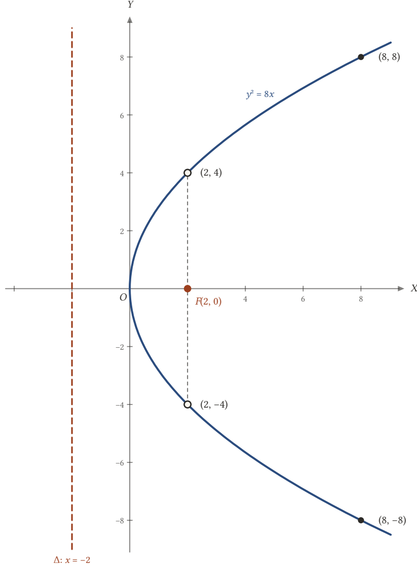
Şekil 20.5: y^2 = 8x : köşe O , odak F(2, 0) , doğrultman x = -2 .
