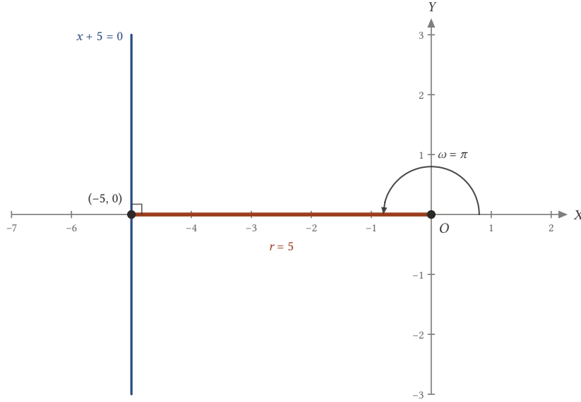
Şekil 3.15: x + 5 = 0 düşey doğrusuna orijinden inen dikme X -ekseninin negatif yarısı üzerindedir: ayağı (-5, 0) , r = 5 , \omega = \pi .
