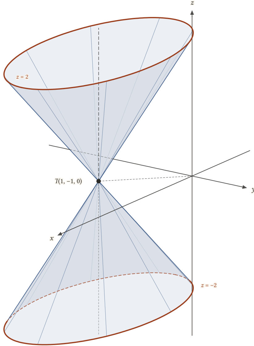
Şekil 23.24: Eliptik koni (x - 1)^2 + 4(y + 1)^2 = z^2 , |z| \leq 2 . Tepe noktası T(1, -1, 0) , eksenini T 'den geçen ve z -eksenine paralel kesikli doğrudur; z = \pm 2 'deki izler merkezi (1, -1, \pm 2) , yarı eksenleri 2 ve 1 olan elipslerdir.
