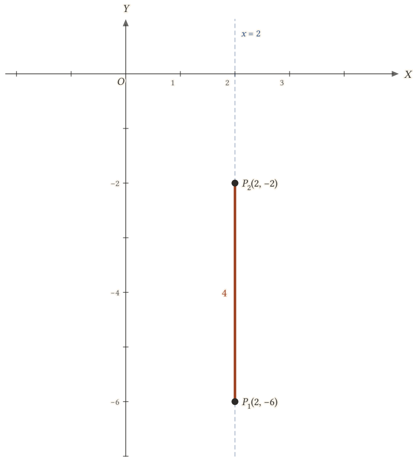
Şekil 1.8: Apsisleri eşit iki nokta x = 2 düşey doğrusu üzerindedir; aralarındaki uzaklık ordinatlar farkının mutlak değeri olan 4'tür.
