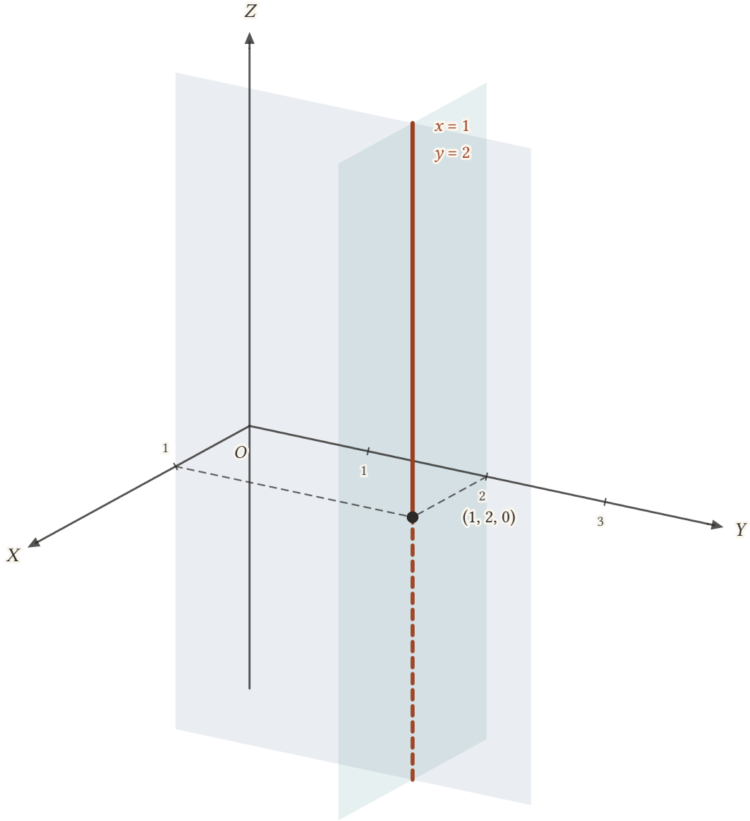
Şekil 6.8: x = 1 , y = 2 koşullarını sağlayan noktalar, (1, 2, 0) noktasından geçen ve Z -eksenine paralel olan doğruyu oluşturur. Soluk mavi ve yeşil parçalar x = 1 ve y = 2 düzlemleridir; doğru bu iki düzlemin kesişimidir. Doğrunun XY -düzleminin altındaki kısmı kesiklidir.
