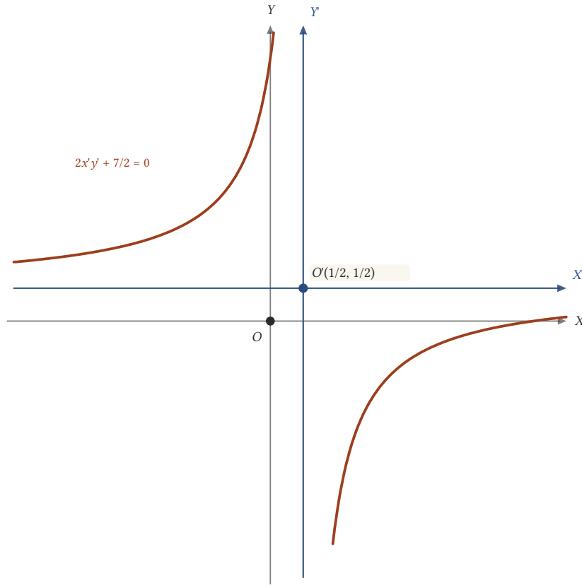
Şekil 17.26: Eksenler O(1/2, 1/2) 'ye ötelenince 2xy - x - y + 4 = 0 eğrisinin denklemi 2x'y' + 7/2 = 0 olur.
