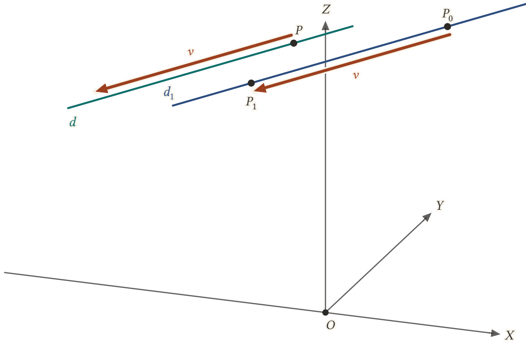
Şekil 10.9: P_0 ile P_1 'den geçen d_1 ve P 'den geçen, aynı v = (-3, -1, -1) doğrultmanlı d doğrusu. P , d_1 üzerinde olmadığından iki doğru çakışmaz.
