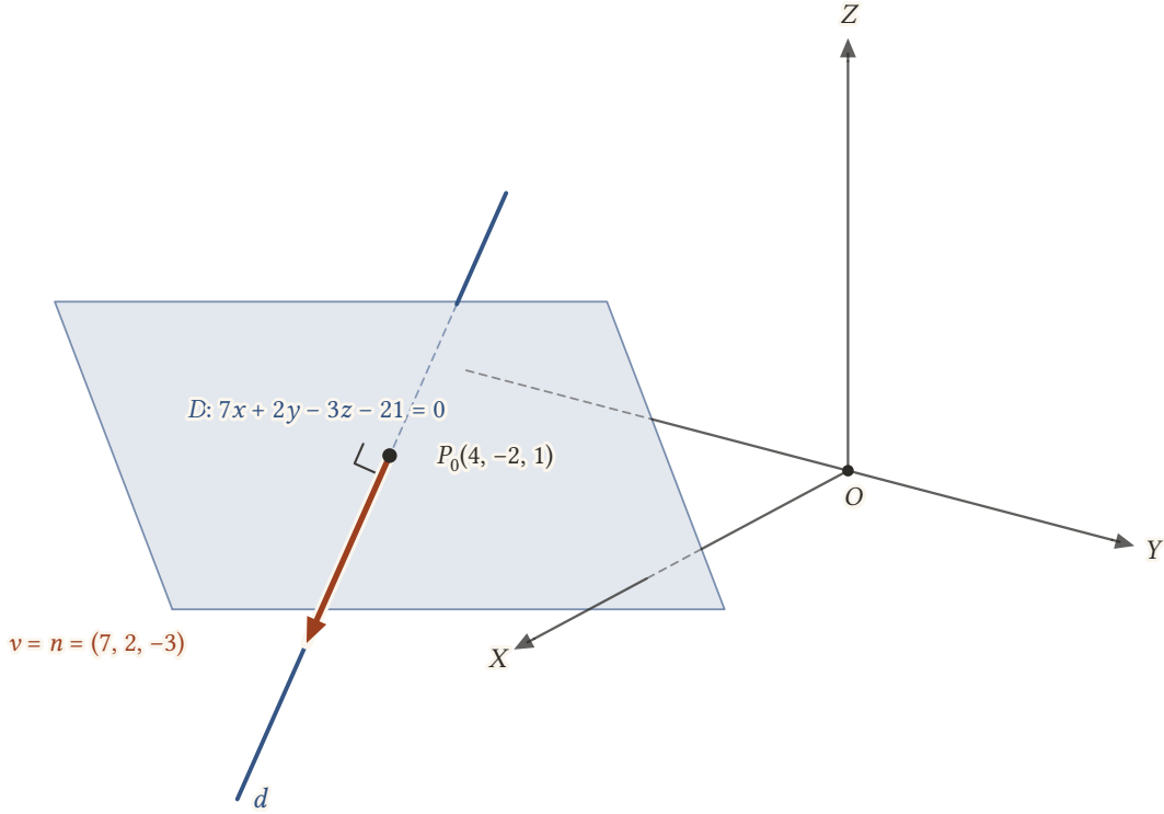
Şekil 12.3: P_0(4, -2, 1) noktasından geçen ve doğrultmanı v = (7, 2, -3) olan d doğrusuna dik düzlem. Doğrunun düzlemin arkasında kalan kısmı kesiklidir.
