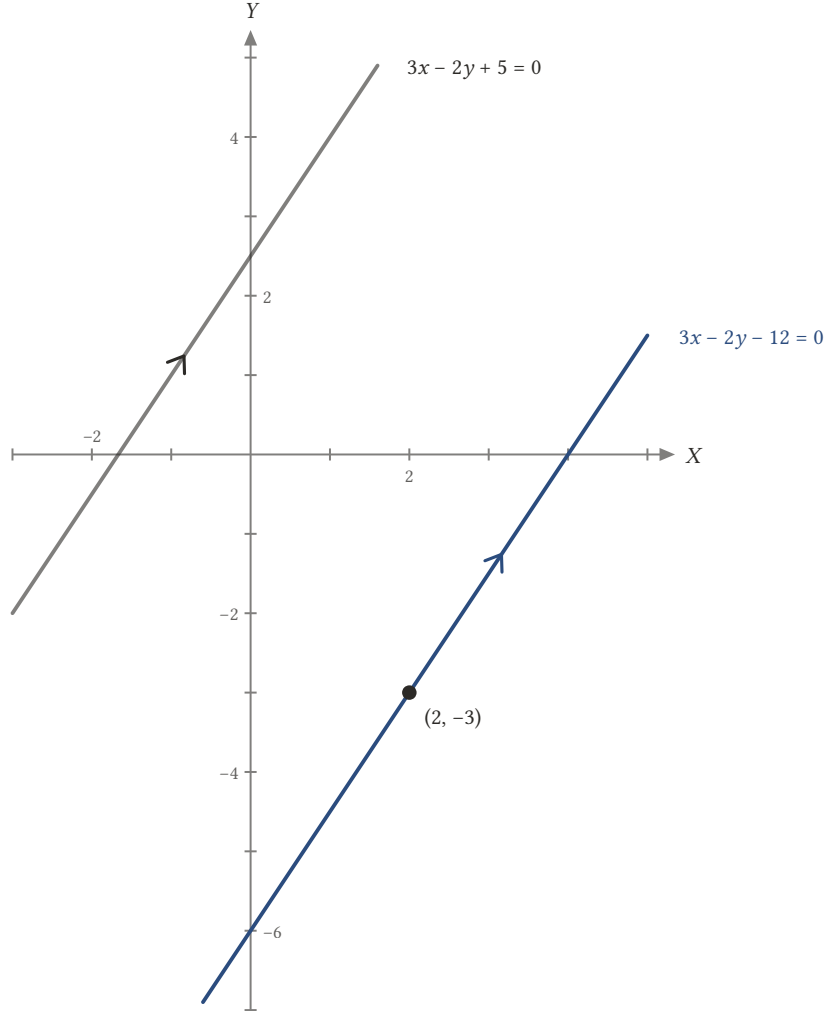
Şekil 3.19: (2, -3) 'ten geçen ve 3x - 2y + 5 = 0 'a paralel olan doğru 3x - 2y - 12 = 0 'dır; iki doğrunun eğimi de 3/2 'dir.
