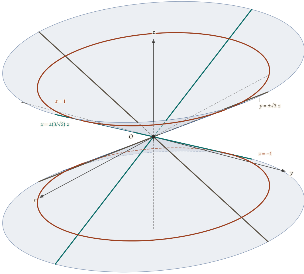
Şekil 23.20: Eliptik koni 2x^2 + 3y^2 = 9z^2 , |z| \leq 1,3 . z = \pm 1 düzlemlerindeki izler aynı 2x^2 + 3y^2 = 9 elipsidir (kırmızı); xz -düzlemindeki iz x = \pm(3/\sqrt{2})z (yeşil), yz -düzlemindeki iz y = \pm\sqrt{3}z doğru çiftidir. İki kanat O 'da birleşir.
