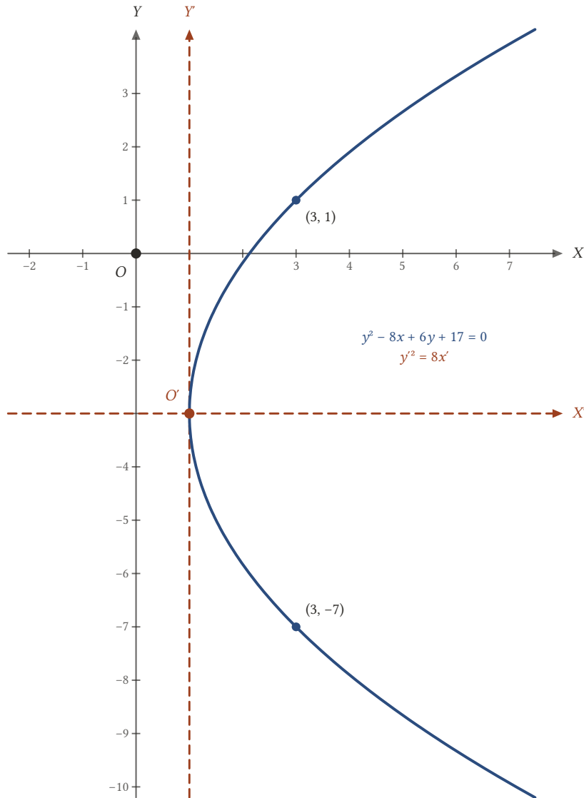
Şekil 16.21: Eksenler O'(1, -3) noktasına ötelenince denklem y'^2 = 8x' olur; eğri (3, 1) ve (3, -7) noktalarından geçer.
