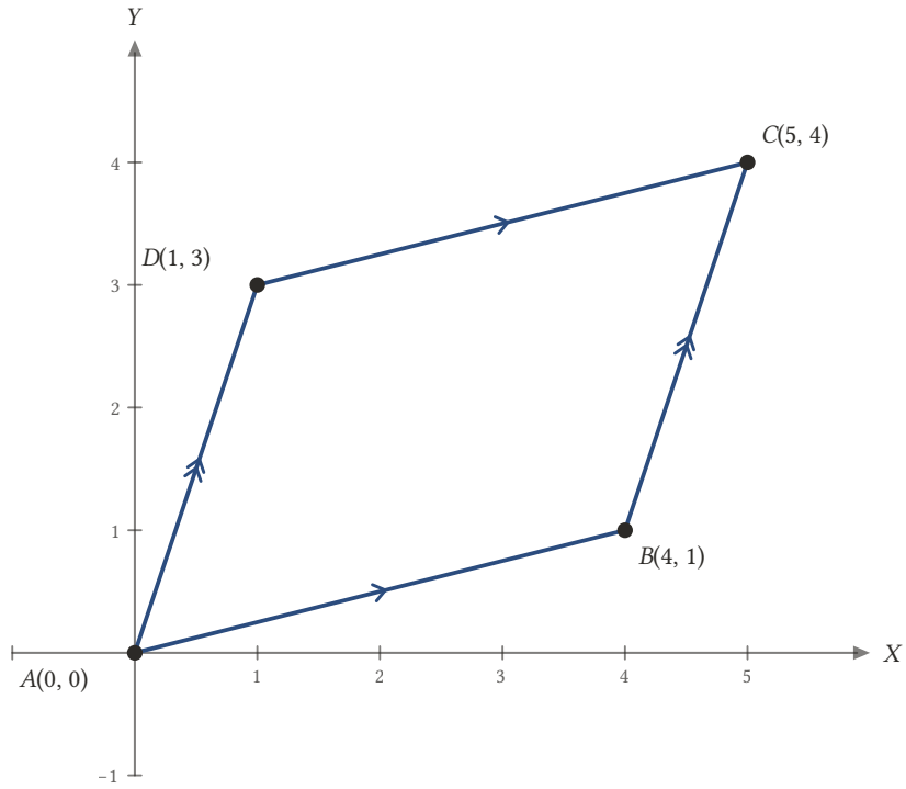
Şekil 2.21: ABCD dörtgeninde karşılıklı kenarların eğimleri eşittir: AB ve DC için 1/4 (tek ok), BC ve AD için 3 (çift ok). Dörtgen bir paralelkenardır.
