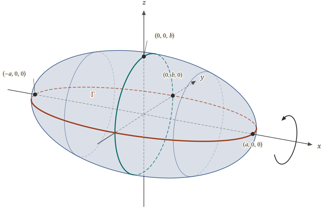
Şekil 23.12: a = 2 , b = 1 için x^2/4 + y^2 = 1 elipsi \Gamma 'nin (kırmızı) x -ekseni etrafında döndürülmesiyle oluşan dönel elipsoid x^2/4 + y^2 + z^2 = 1 . Yeşil çember x = 0 kesitidir; x = \pm 1 kesitleri yarıçapı \sqrt{3}/2 olan çemberlerdir.
