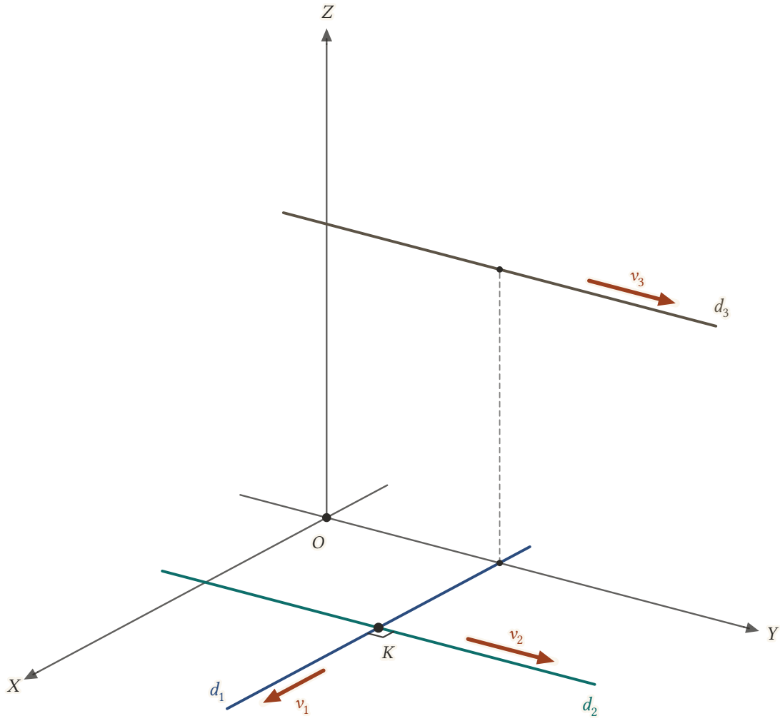
Şekil 10.10: d_1 \perp d_2 ve bu iki doğru K 'da kesişir. d_3 , d_1 'in 3 birim üstünden geçer: d_1 \perp d_3 olduğu hâlde bu iki doğru kesişmez.
