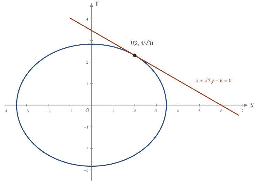
Şekil 18.28: x^2/12 + y^2/8 = 1 elipsinin P(2, 4/\sqrt{3}) noktasındaki teğeti x + \sqrt{3}y - 6 = 0 .
