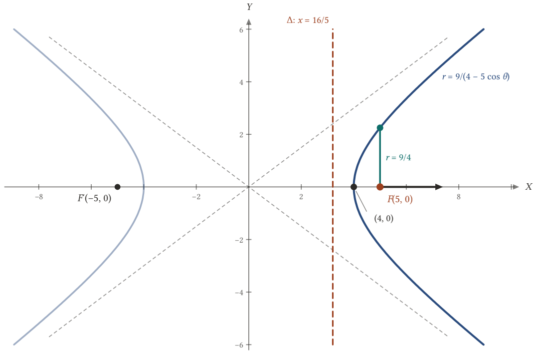
Şekil 20.14: Kutup sağ odakta: r = 9/(4 - 5 \cos \theta) sağ kolu verir; sol kol (soluk) doğrultmanın öbür yanındadır. Ok kutupsal eksenini gösterir.
