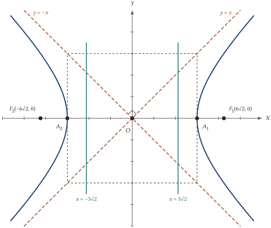
Şekil 19.22: x^2 - y^2 = 36 bir ikizkenar hiperboldür: a = b = 6 , asimptotlar y = \pm x .
