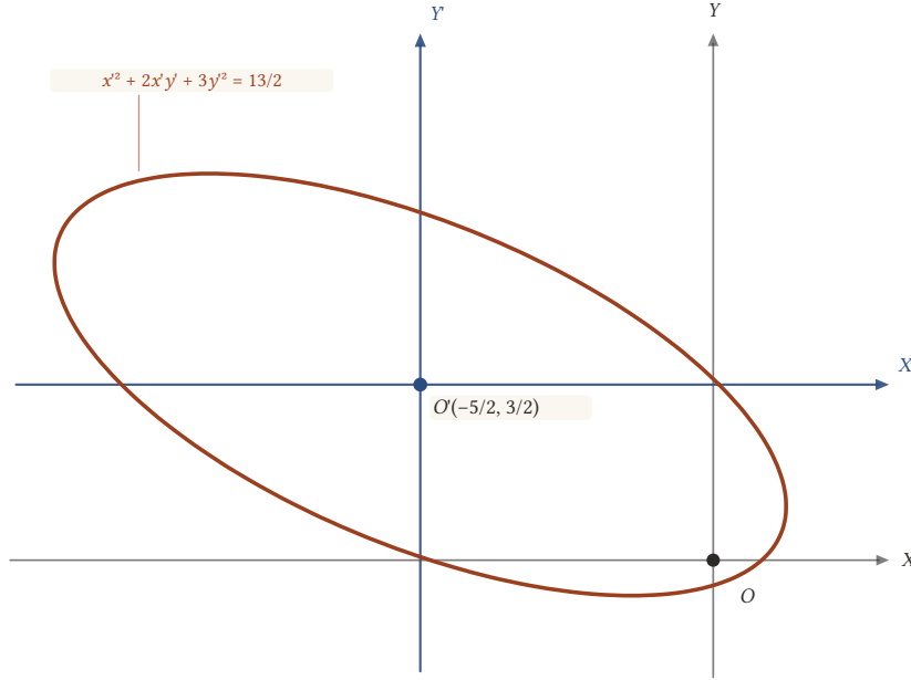
Şekil 17.27: Eksenler O'(-5/2, 3/2) 'ye ötelenince birinci dereceden terimler kaybolur; elipsin merkezi yeni başlangıç noktasıdır.
