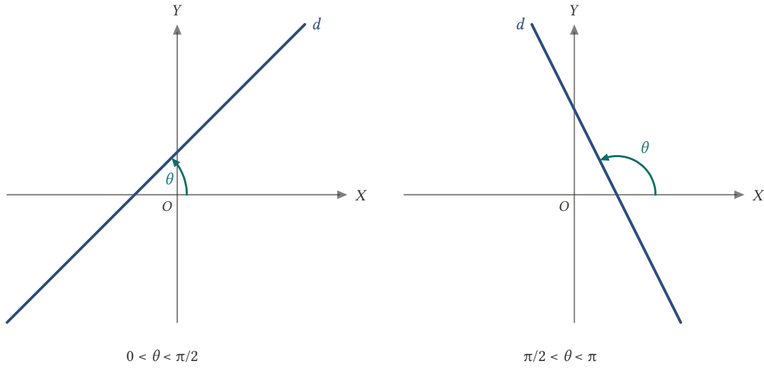
Şekil 2.10: Eğim açısı \theta , X-ekseninin pozitif yönünden doğruya saat yönünün tersine ölçülür. Solda sağa doğru yükselen doğru ( 0 < \theta < \pi/2 ), sağda sağa doğru alçalan doğru ( \pi/2 < \theta < \pi ).
