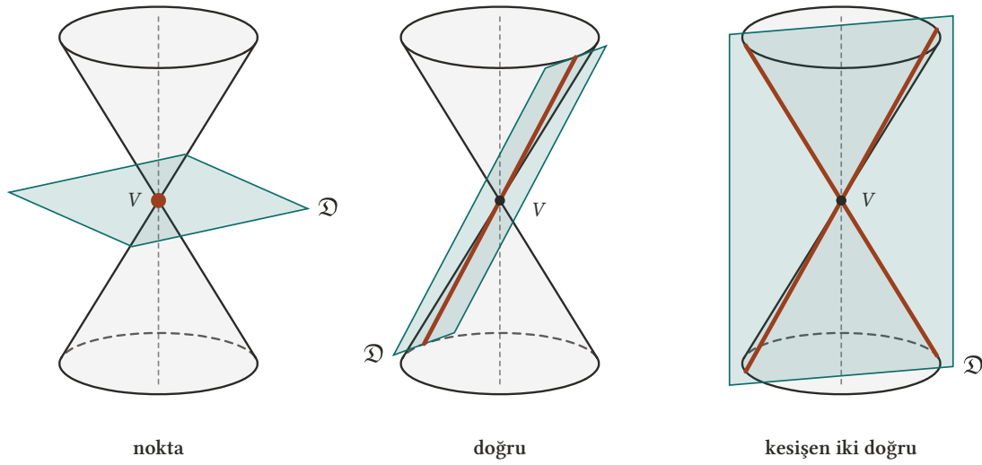
Şekil 18.3: Düzlem koninin köşesinden geçerse yozlaşmış konikler çıkar: yalnız köşe V, bir ana doğru ya da köşede kesişen iki ana doğru.
