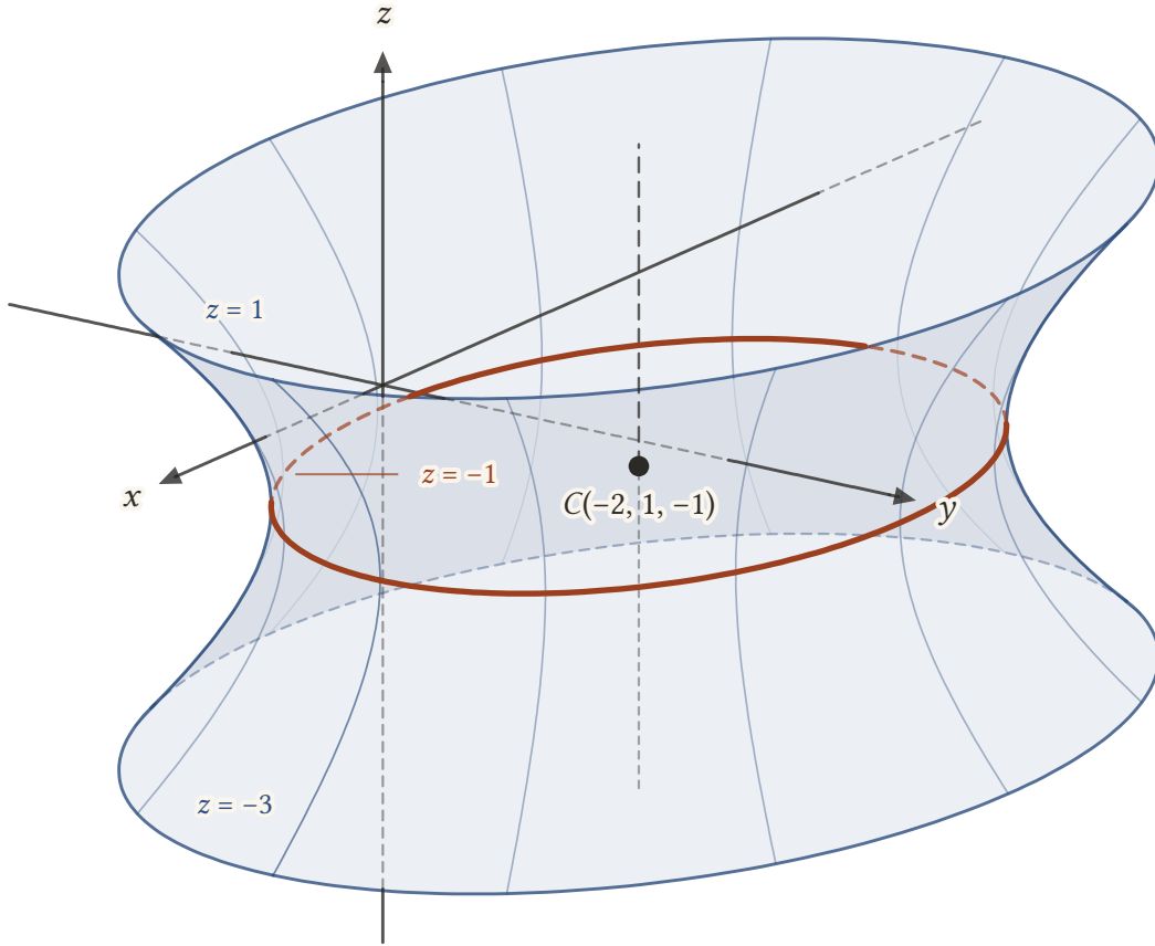
Şekil 23.32: Tek kanatlı hiperboloid (x+2)^2/12 + (y-1)^2/6 - (z+1)^2/4 = 1, -3 \leq z \leq 1 . Merkez C(-2, 1, -1) ; eksen C 'den geçen düşey kesikli doğrudur. Bel elipsi (kırmızı) z = -1 düzleminde, yarı eksenleri 2\sqrt{3} ve \sqrt{6} 'dır.
