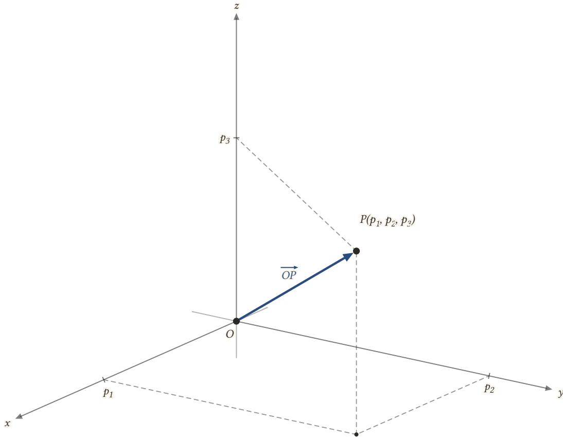
Şekil 7.7: P noktasının konum vektörü, başlangıç noktasından P 'ye çizilen oktur; kesikli çizgiler P 'nin koordinatlarını eksenler üzerinde okutur.
