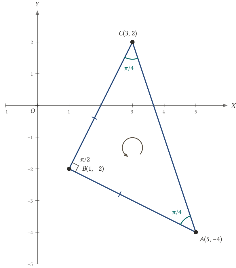
Şekil 2.27: A(5, -4) , B(1, -2) , C(3, 2) üçgeninin iç açıları: B 'de \pi/2 , A ve C 'de \pi/4 . Köşeler saat yönünün tersine A , C , B sırasıyla dolaşılır; çentikler |AB| = |BC| eşitliğini gösterir.
