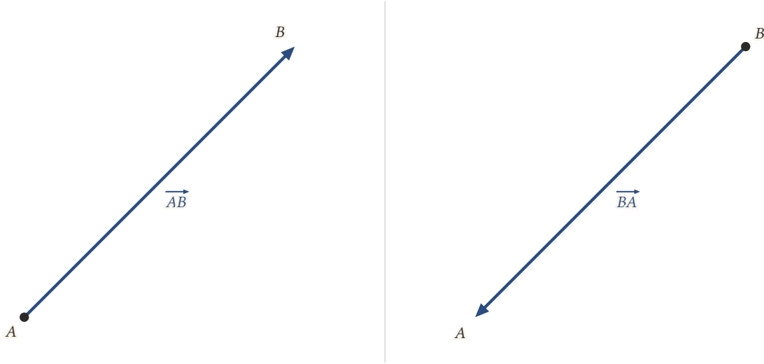
Şekil 7.1: Aynı doğru parçası üzerinde iki farklı yönlü doğru parçası: solda ok B 'yi, sağda A 'yı gösterir.
