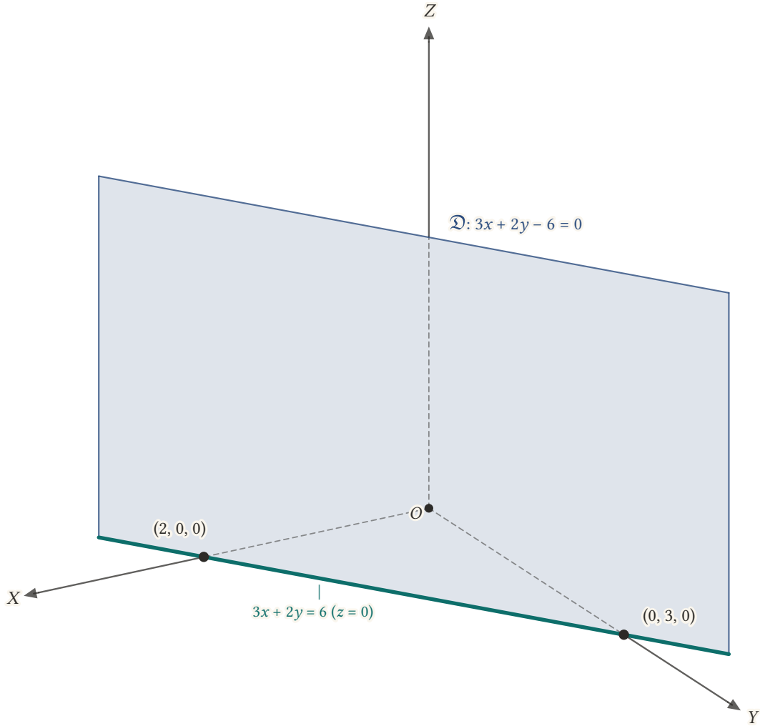
Şekil 13.14: 3x + 2y - 6 = 0 düzlemi, XY -düzlemindeki izi 3x + 2y = 6 üzerinde dikilen bir duvardır. Z -eksenine paraleldir ama onu kesmez: eksen duvarın arkasında kalır (kesikli).
