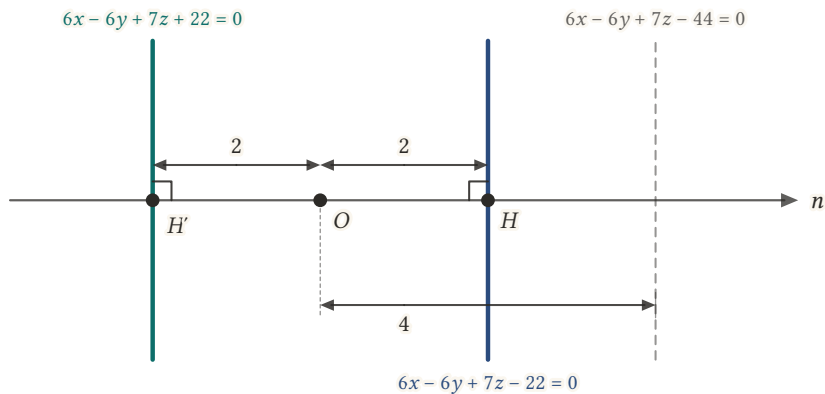
Şekil 13.20: Normal doğrultusundaki kesit: düzlemler n 'ye dik doğrular olarak görünür. Orijinin iki yanında, ona 2 birim uzaklıkta iki paralel düzlem vardır; kesikli doğru, orijine uzaklığı 4 olan verilen düzlemdir.
