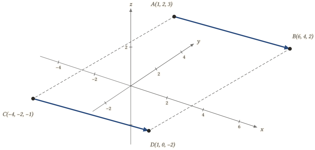
Şekil 7.6: AB ile CD aynı vektörü temsil ettiğinden ABDC bir paralelkenardır; kesikli kenarlar AC ve BD dir.
