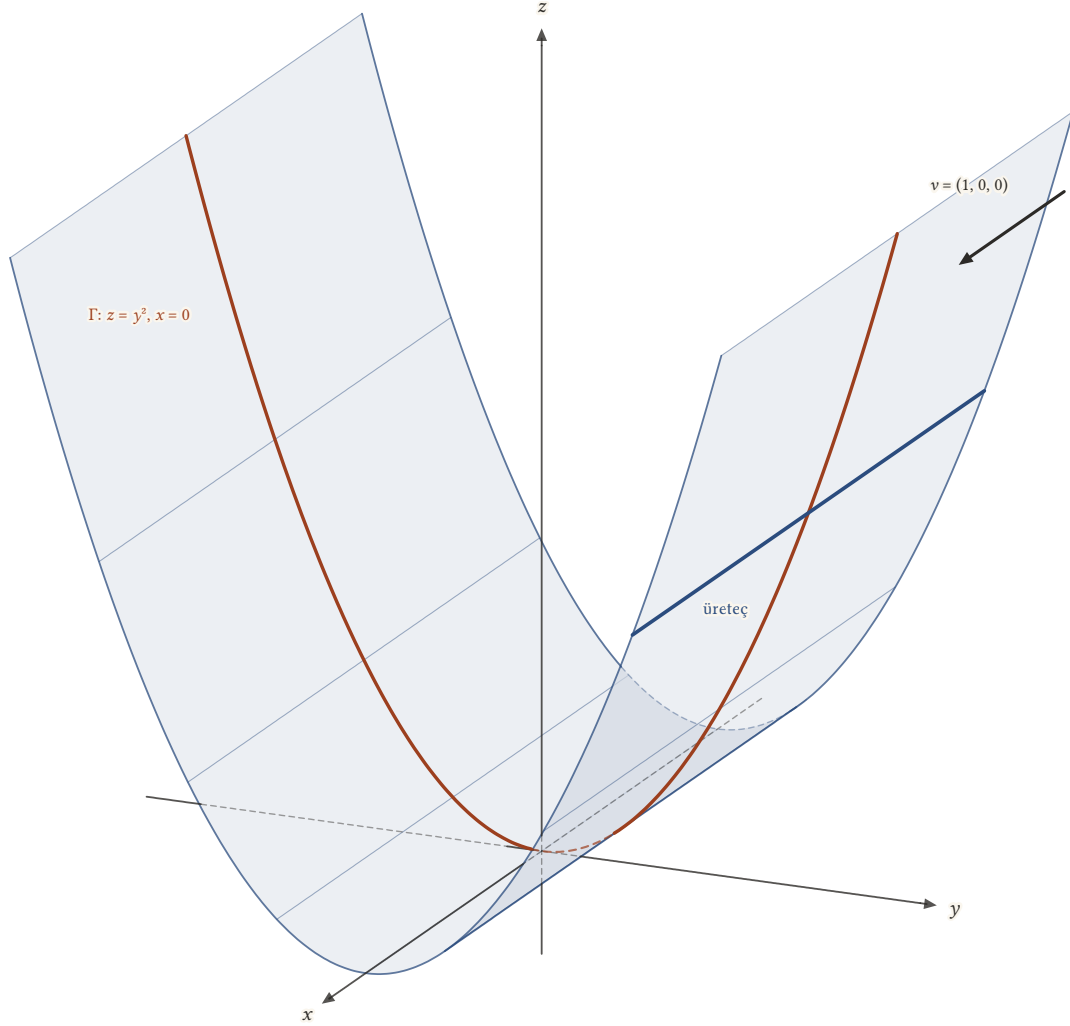
Şekil 23.7: Parabolik silindir z = y^2 ( -2 \leq x \leq 2 parçası): yz -düzlemindeki \Gamma parabolü (kırmızı) x -ekseni doğrultusunda kaydırılır; üreteçler v = (1, 0, 0) 'a paraleldir.
