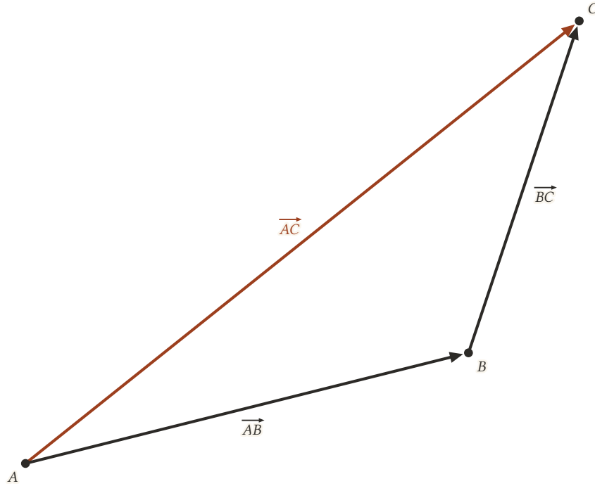
Şekil 7.9: Üçgen kuralı: A'dan B'ye, oradan C'ye gitmek, doğrudan A'dan C'ye gitmekle aynı yer değiştirir.
