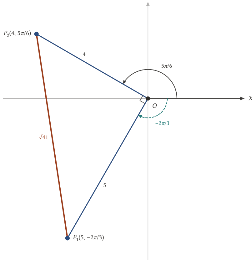
Şekil 5.23: (5, -2\pi/3) saat yönünde ölçülen açıyla bulunur. İki yarıçap arasındaki açı 3\pi/2 - \pi = \pi/2 olduğundan uzaklık \sqrt{(25 + 16)} = \sqrt{41} 'dir.
