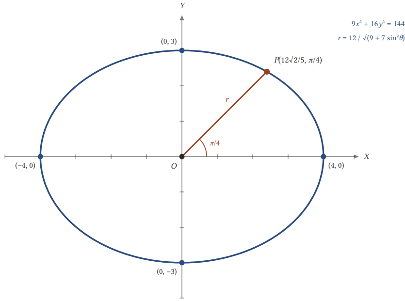
Şekil 5.31: 9x^2 + 16y^2 = 144 elipsi ve \theta = \pi/4 yönündeki kutupsal yarıçap: r = 12\sqrt{2}/5 , yani P = (12/5, 12/5) .
