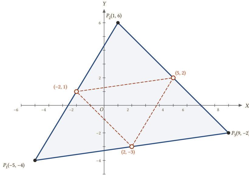
Şekil 1.28: Kenar orta noktaları (-2, 1) , (5, 2) ve (2, -3) olan üçgenin köşeleri P_1(-5, -4) , P_2(1, 6) ve P_3(9, -2) 'dir.
