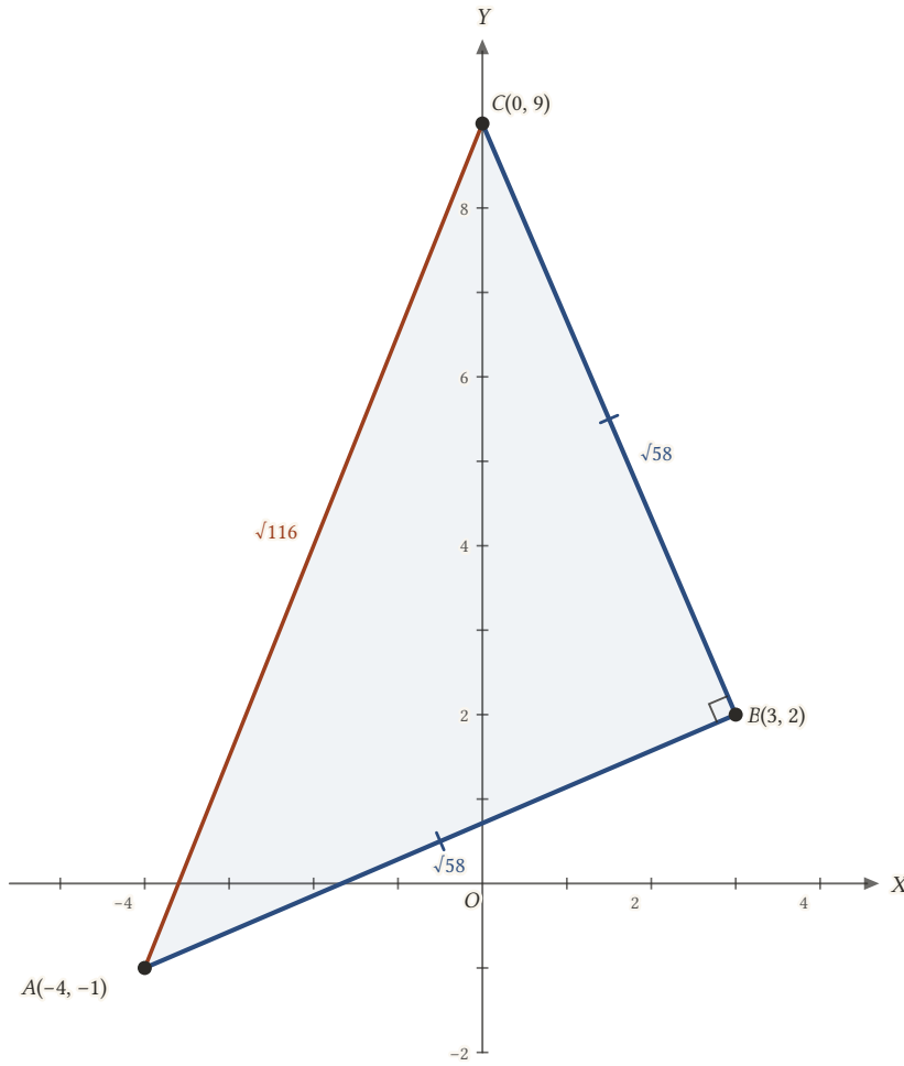
Şekil 1.15: 58 + 58 = 116 olduğundan B açısı diktir; eşit dik kenarlar üçgeni ikizkenar dik üçgen yapar.
