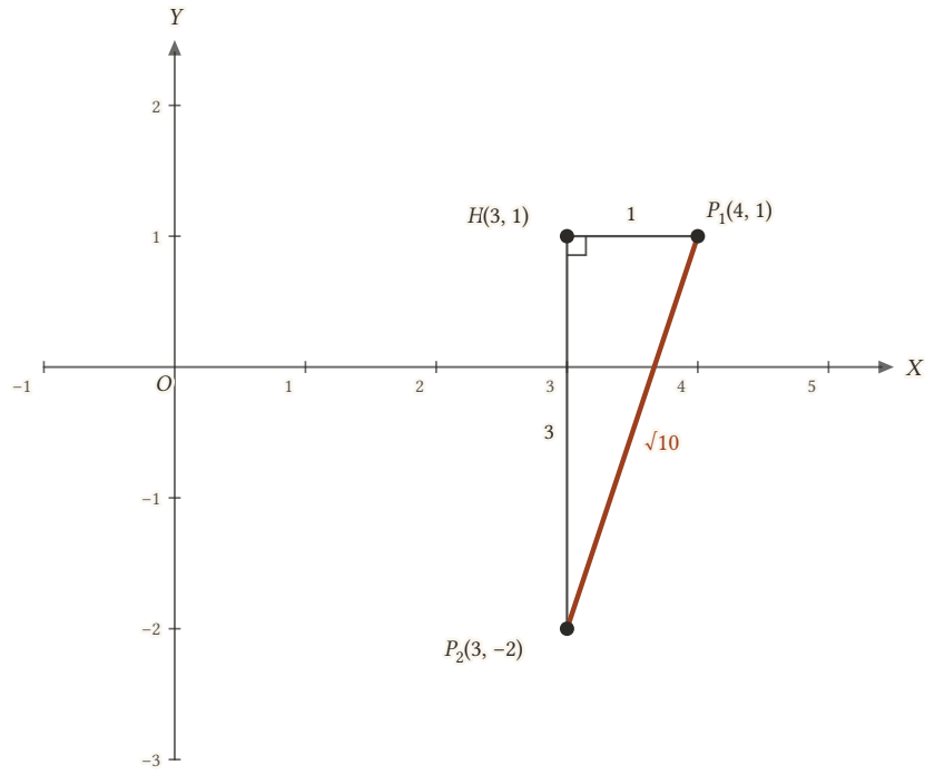
Şekil 1.7: Dik kenarları 1 ve 3 olan dik üçgenin hipotenüsü |P_1P_2| = \sqrt{10} 'dur.
