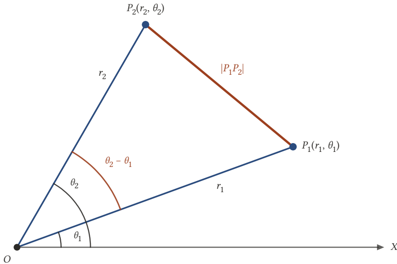
Şekil 5.10: Kutupsal koordinatlarda uzaklık: P_1OP_2 üçgeninde kenarlar r_1 , r_2 ve aradaki açının kosinüsü \cos(\theta_2 - \theta_1) 'dir; |P_1P_2| kosinüs teoremiyle bulunur.
