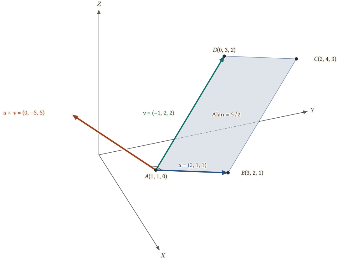
Şekil 9.7: A(1, 1, 0) , B(3, 2, 1) , C(2, 4, 3) , D(0, 3, 2) köşeli paralelkenar. A 'dan çıkan kısa ok u \times v = (0, -5, 5) vektörünün 0,4 katıdır; paralelkenarın düzlemine diktir ve uzunluğu alanı, 5\sqrt{2} 'yi verir.
