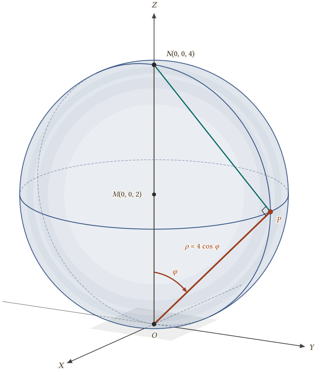
Şekil 22.11: \rho = 4 \cos \varphi küresi: merkezi M(0, 0, 2) , yarıçapı 2, XY -düzlemine O 'da teğet. ON bir çap olduğundan OPN üçgeni P 'de diktir ve |OP| = 4 \cos \varphi olur (şekilde P(0, 2, 2) , \varphi = \pi/4 ).
