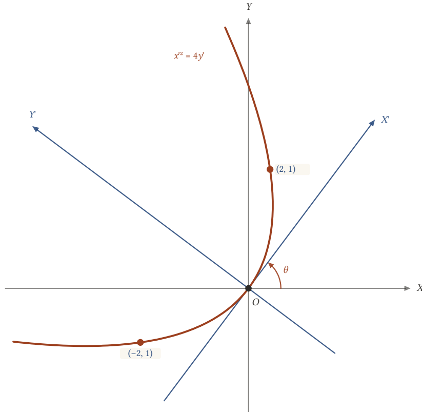
Şekil 17.28: Eksenler \arctan(4/3) döndürülünce 9x^2 + 24xy + 16y^2 + 80x - 60y = 0 eğrisinin denklemi x'^2 = 4y' olur; parabolün eksen Y' -eksenidir. İşaretli noktaların yanındaki sayılar yeni (x', y') koordinatlarıdır.
