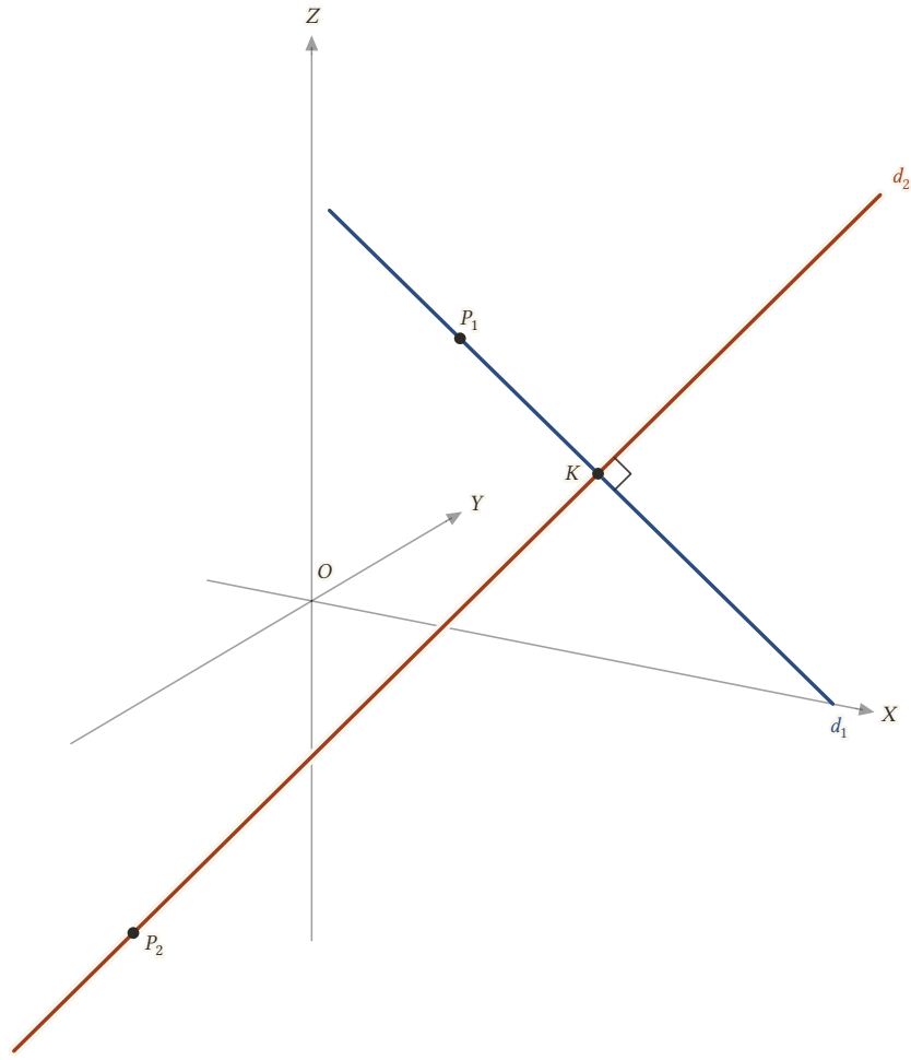
Şekil 11.2: d_1 ile d_2 doğruları K(28/9, -17/27, 17/9) noktasında dik kesişir: \langle v_1, v_2 \rangle = 0 , \theta = \pi/2 .
