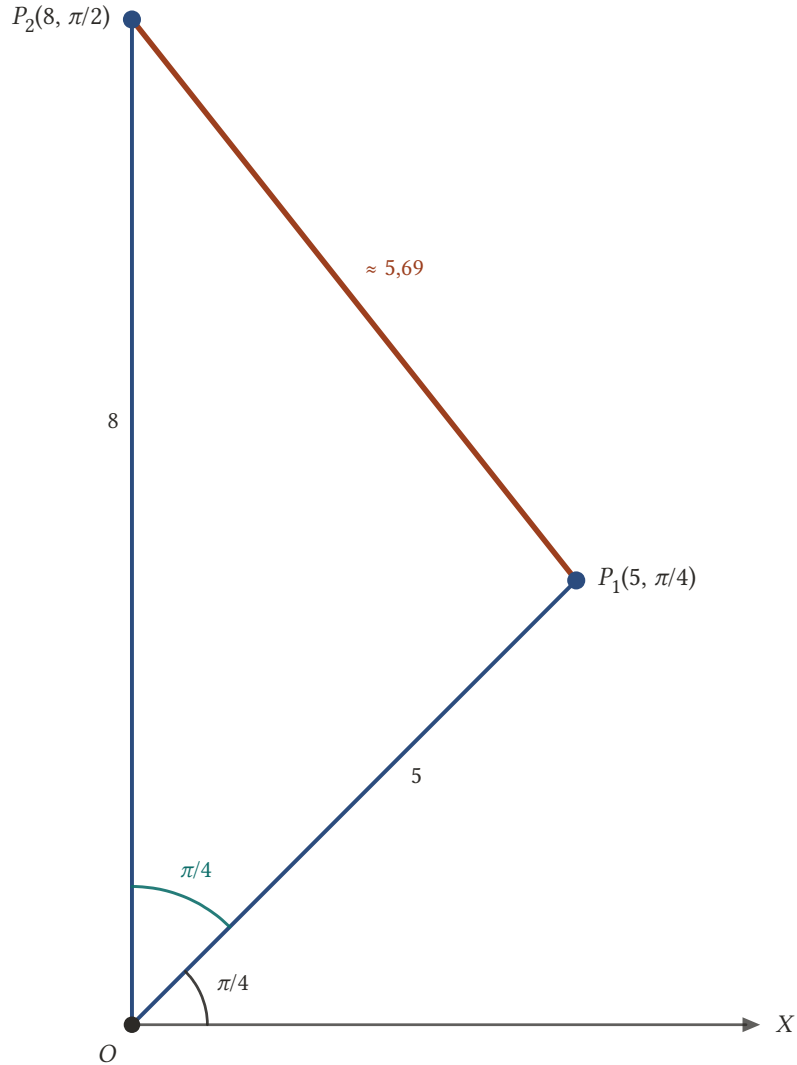
Şekil 5.22: (5, \pi/4) ile (8, \pi/2) arasındaki açı \pi/4 'tür; uzaklık \sqrt{89 - 40\sqrt{2}} \approx 5,69 .
