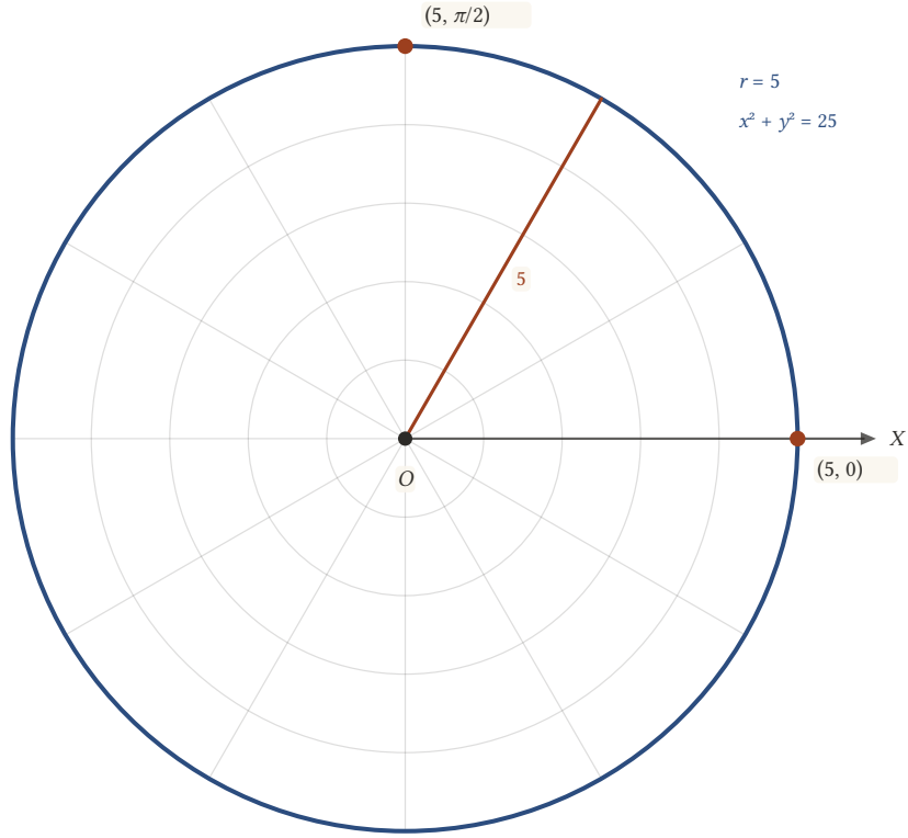
Şekil 5.30: Kutup merkezli, 5 yarıçaplı çember: kutupsal denklemi r = 5 , dik denklemi x^2 + y^2 = 25 .
