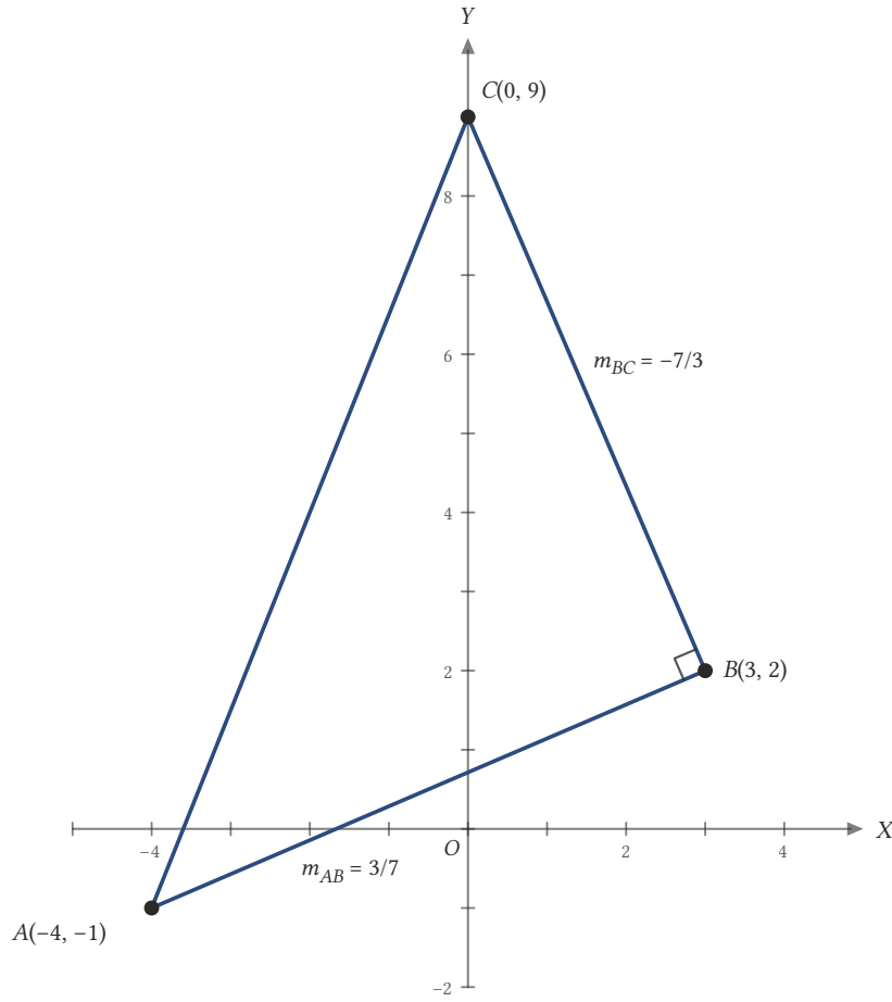
Şekil 2.19: A(-4, -1) , B(3, 2) , C(0, 9) üçgeninde m_{AB} \cdot m_{BC} = -1 ; üçgen B köşesinde dik açıdır.
