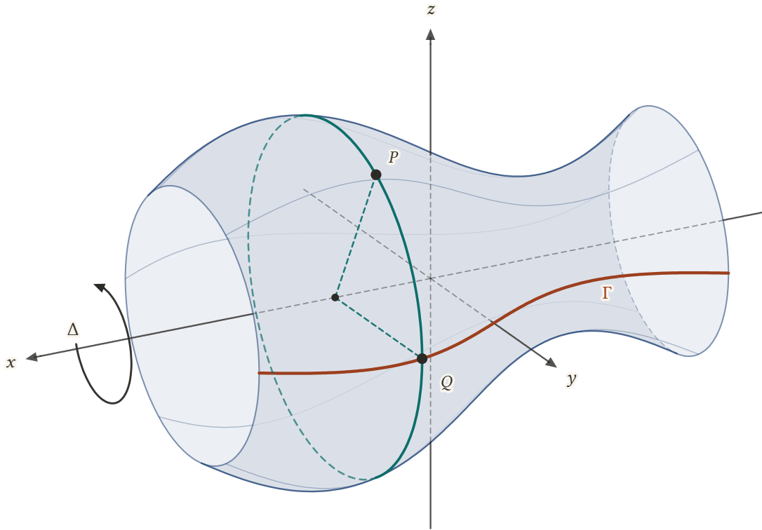
Şekil 23.11: Dönel yüzey: xy -düzlemindeki \Gamma eğrisi (kırmızı) \Delta = x -ekseni etrafında döndürülür. \Gamma 'nın her Q noktası, merkezi eksen üzerinde olan ve eksene dik bir düzlemde kalan bir çember (yeşil) çizer; bu çemberin P noktalarının eksene uzaklığı Q 'nunkine eşittir.
