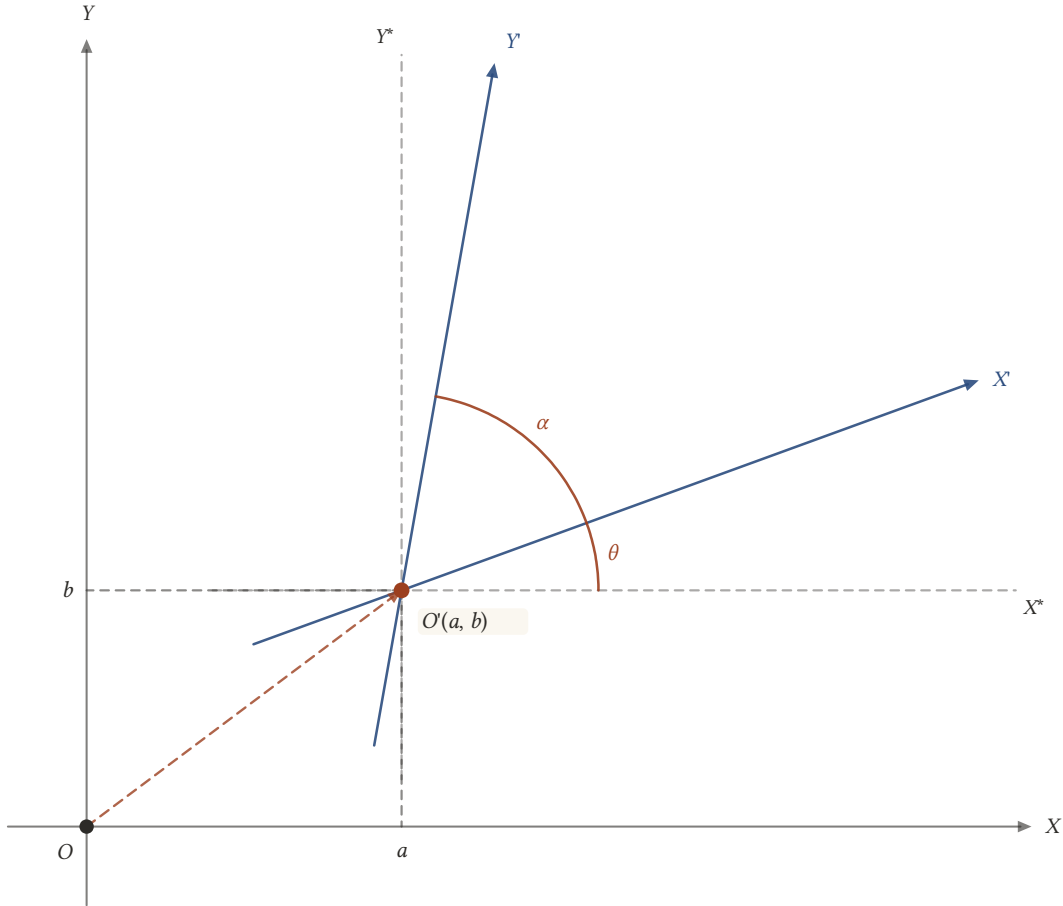
Şekil 17.18: Başlangıçlar farklıysa XY önce O'(a, b) 'ye ötelenip X^*Y^* elde edilir; X^*Y^* ile eğik X'Y' sisteminin başlangıcı ortaktır.
