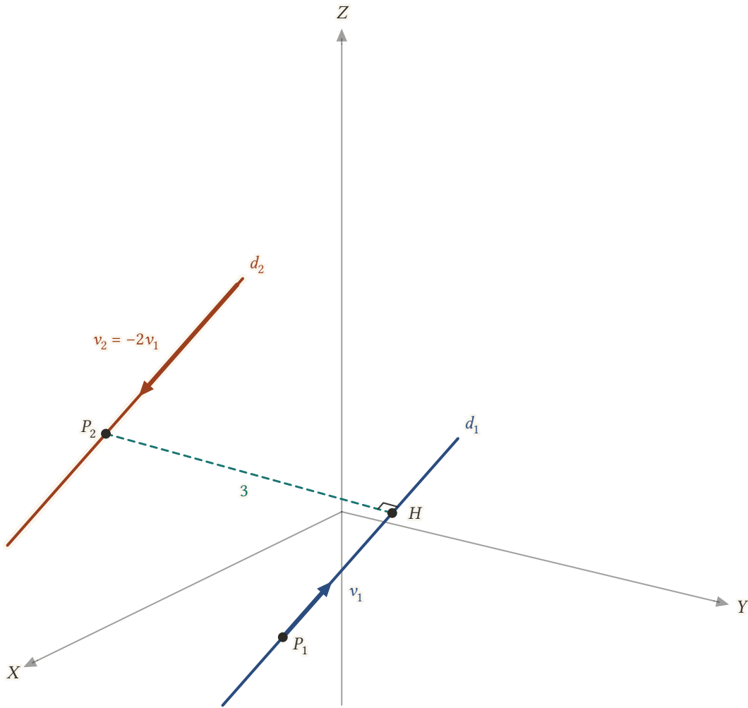
Şekil 11.9: Paralel ve farklı iki doğru: v_2 = -2v_1 ters yönde ve iki kat uzundur, P_2(4, 0, 2) ise d_1 üzerinde değildir. P_2 'den d_1 'e inilen dikmenin ayağı H(2, 2, 1) , uzunluğu 3'tür.
