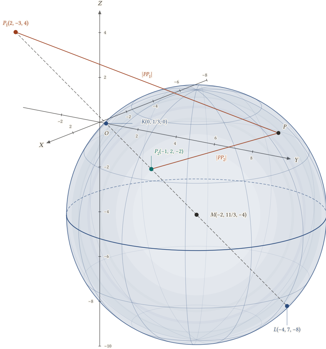
Şekil 6.16: P_1 'e uzaklığı P_2 'ye uzaklığının 2 katı olan noktalar, merkezi M(-2, 11/3, -4) ve yarıçapı 2\sqrt{70}/3 \approx 5,58 olan küreyi oluşturur. P_1P_2 doğrusu M 'den geçer ve küreyi K ile L noktalarında keser; küre üzerindeki her P için |PP_1| = 2|PP_2| .
