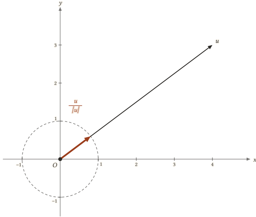
Şekil 7.15: u = (4, 3) ve aynı ışın üzerindeki birim vektör u/\|u\| = (0,8; 0,6) ; birim vektörün ucu birim çemberin üzerindedir.
