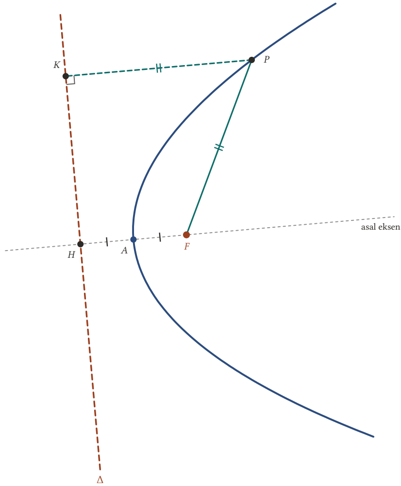
Şekil 20.1: Parabolün öğeleri: odak F, doğrultman \Delta , köşe A. Her P noktası için |PF| = |PK| ; köşe HF parçasının orta noktasıdır.
