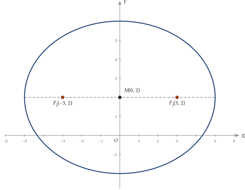
Şekil 18.26: Odakları (-3, 2) , (3, 2) ve asal eksen uzunluğu 10 olan elips: x^2/25 + (y-2)^2/16 = 1 .
