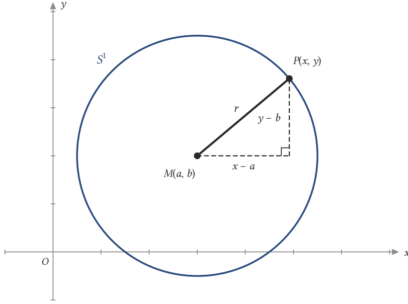
Şekil 4.2: P(x, y) ile M(a, b) arasındaki uzaklık, dik kenarları |x - a| ve |y - b| olan dik üçgenin hipotenüsüdür; P çember üzerindeyse bu uzaklık r 'dir.
