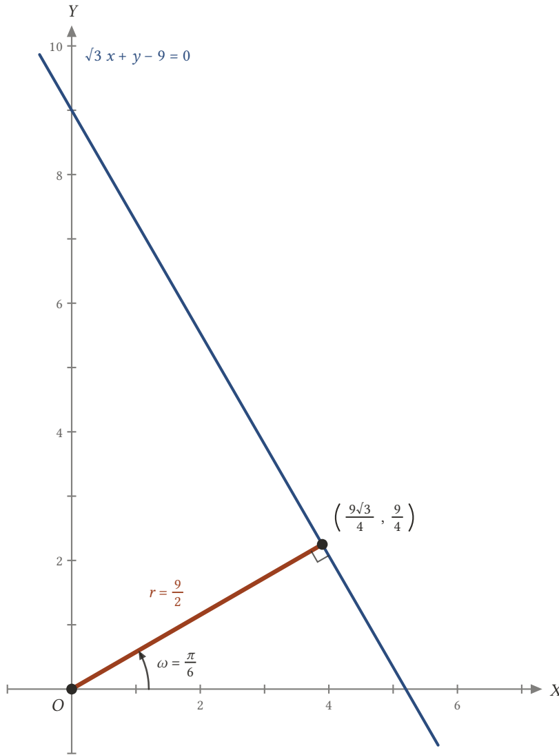
Şekil 3.16: \sqrt{3}x + y - 9 = 0 doğrusuna orijinden inen dikmenin ayağı (9\sqrt{3}/4, 9/4) 'tür: r = 9/2 , \omega = \pi/6 .
