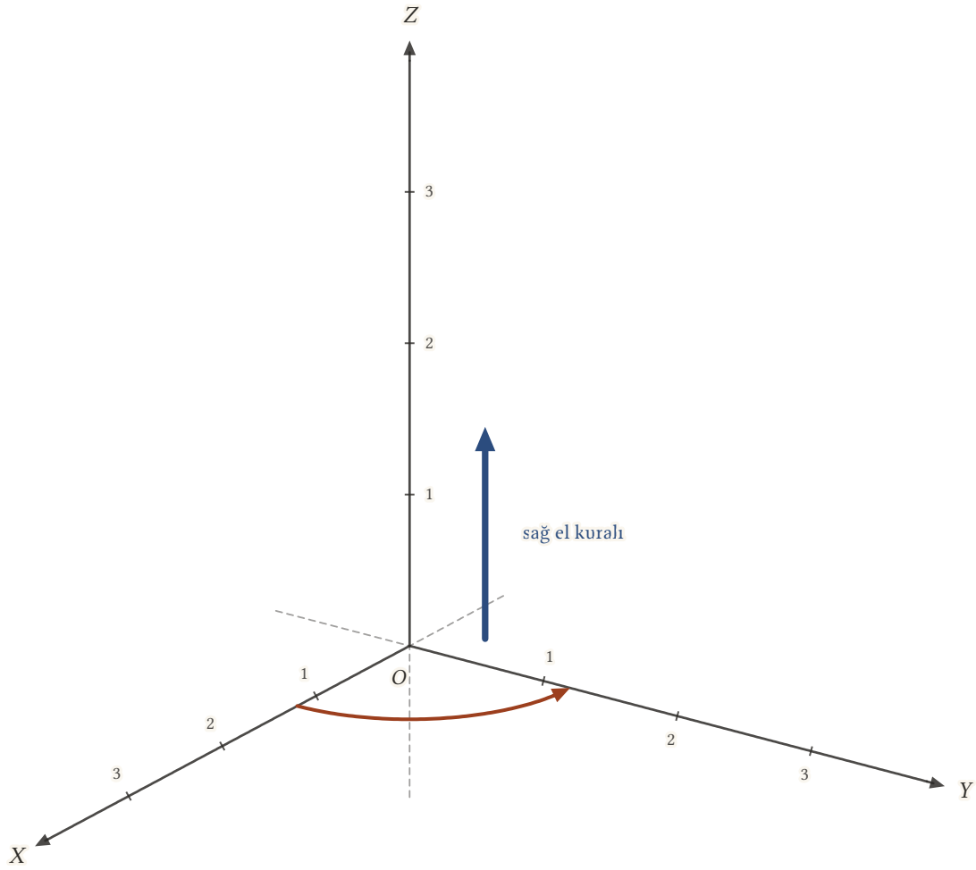
Şekil 6.1: Sağ el kuralına göre yönlendirilmiş eksenler: X-ekseni okuyucuya doğru (sol aşağı), Y-ekseni sağa, Z-ekseni yukarı. Pozitif X-ekseninden pozitif Y-eksenine kıvrılan parmaklar (turuncu ok) başparmağı pozitif Z-ekseni yönüne (mavi ok) getirir. Eksenlerin negatif kısımları kesiklidir.
