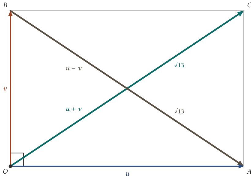
Şekil 8.17: u = (3, 0, 0) ve v = (0, 2, 0) dik olduğundan paralelkenar bir dikdörtgendir; iki köşegenin uzunluğu da \sqrt{13} 'tür.
