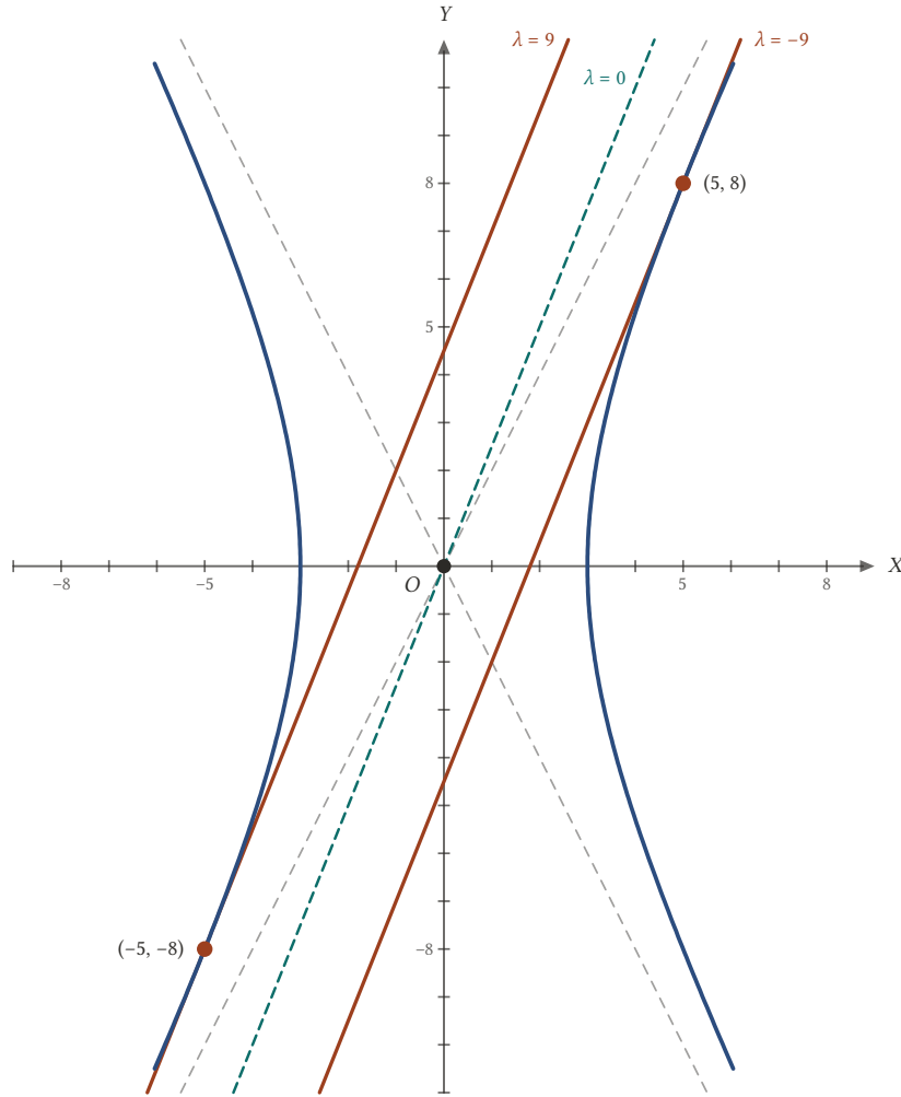
Şekil 19.24: \lambda = \pm 9 'da doğru hiperbole teğet; -9 < \lambda < 9 iken hiperbolü kesmez.
