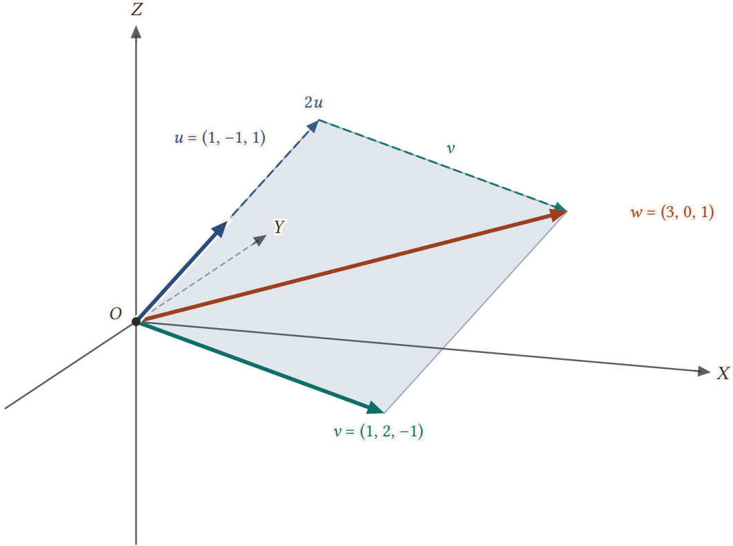
Şekil 9.14: m = 0 için u = (1, -1, 1) , v = (1, 2, -1) , w = (3, 0, 1) aynı düzlemindedir: paralelkenar kuralıyla w = 2u + v .
