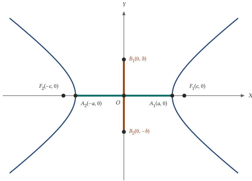
Şekil 19.4: Asal eksen uzunluğu 2a , yedek eksen uzunluğu 2b ; B_1 ve B_2 hiperbolün üzerinde değildir.
