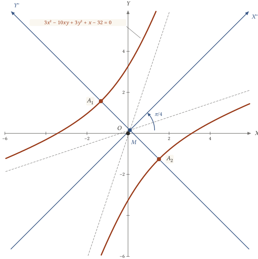
Şekil 21.14: d = 16 > 0 , D = 2045/4 > 0 : konik, asal eksenini Y'' -ekseni olan bir hiperboldür.
