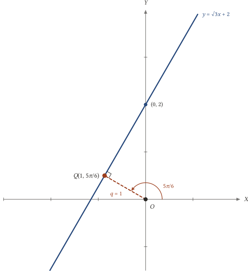
Şekil 5.18: y = \sqrt{3}x + 2 doğrusu için kutuptan inilen dikmenin ayağı Q(1, 5\pi/6) ; normal denklem r \cos(\theta - 5\pi/6) = 1 .
