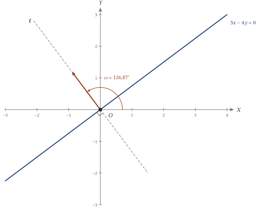
Şekil 3.17: Orijinden geçen 3x - 4y = 0 doğrusu ( r = 0 ). \ell doğruya dik olan doğrudur; seçilen işaret onun üst yarı düzlemdeki ışığını verir: \omega \approx 126,87^\circ .
