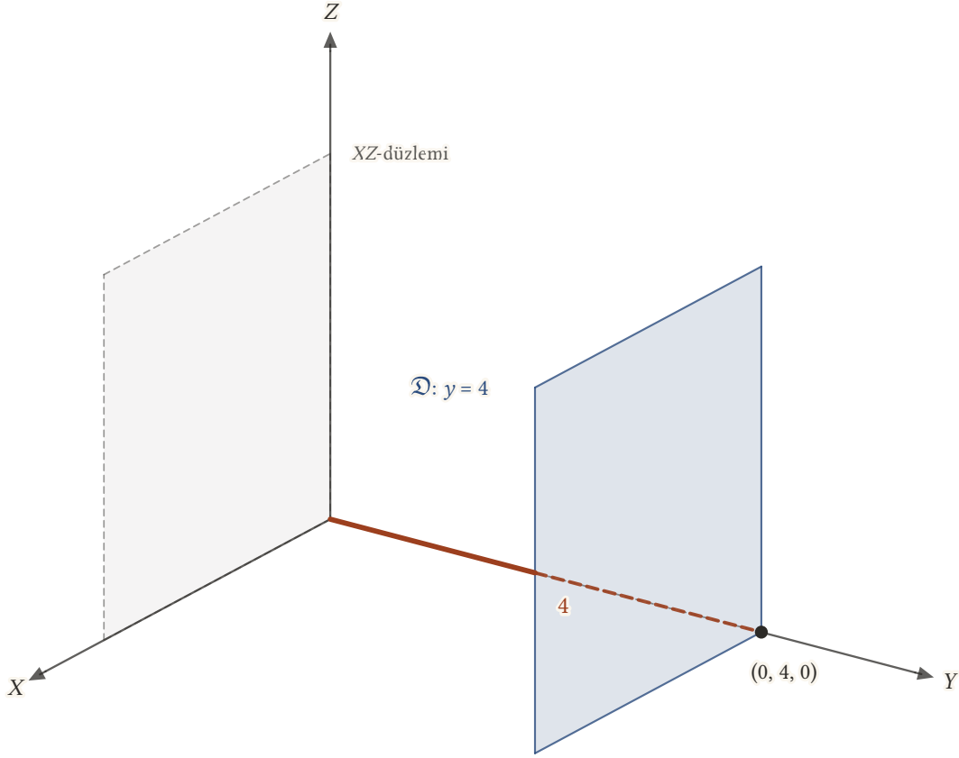
Şekil 13.15: y = 4 düzlemi XZ -düzlemine paraleldir: XZ -düzleminin Y -ekseni boyunca 4 birim kaydırılmışıdır ve Y -eksenini (0, 4, 0) 'da dik keser.
