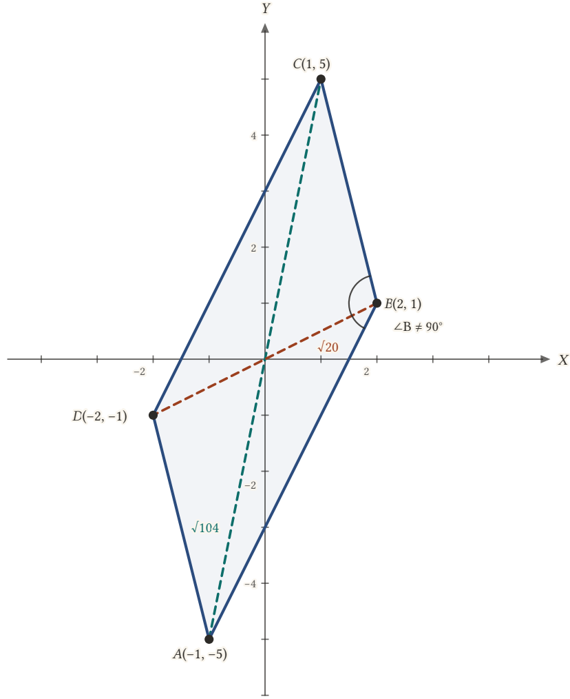
Şekil 1.36: Köşegenler eşit değildir ( \sqrt{104} \neq \sqrt{20} ) ve B açısı dik değildir; ABCD bir dikdörtgen değildir.
