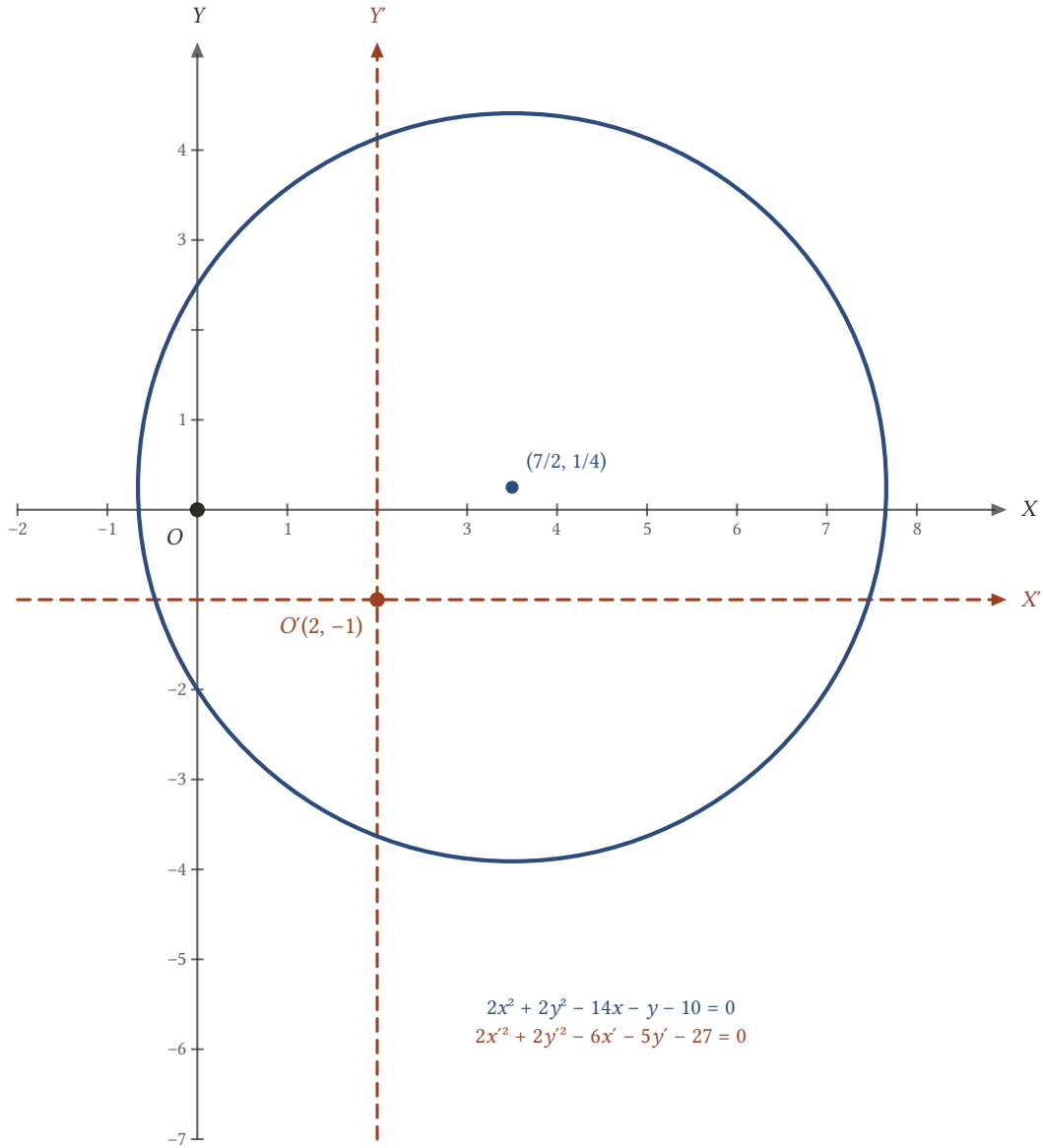
Şekil 16.19: Yeni başlangıç noktası O'(2, -1) çemberin merkezi (7/2, 1/4) değildir; bu yüzden yeni denklemde birinci dereceden terimler kalır.
