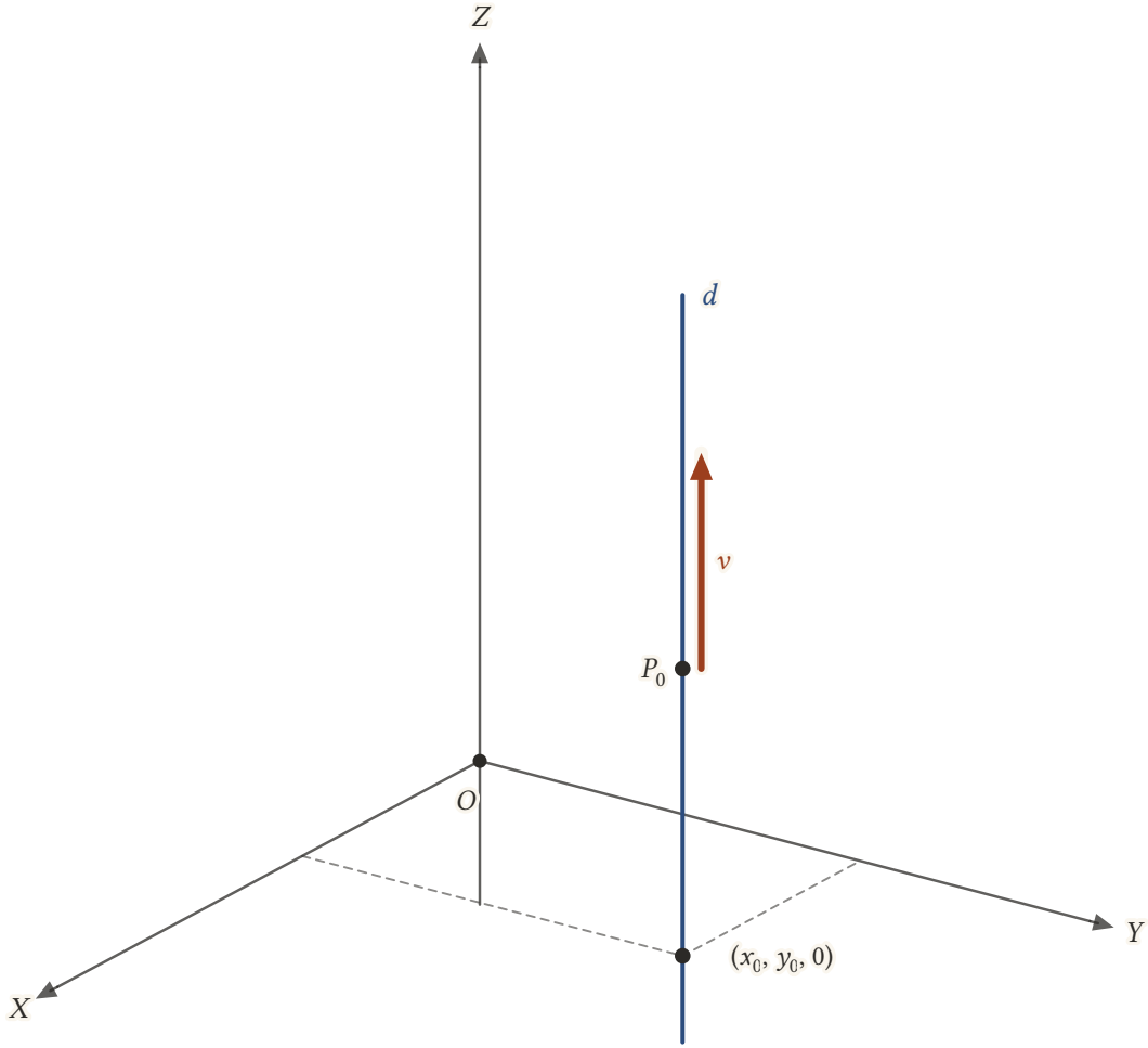
Şekil 10.14: Doğrultmanı Z eksenine paralel olan d doğrusu, XY düzlemindeki (x_0, y_0, 0) noktasından dikey olarak geçer; üzerinde x = x_0 ve y = y_0 sabittir.
