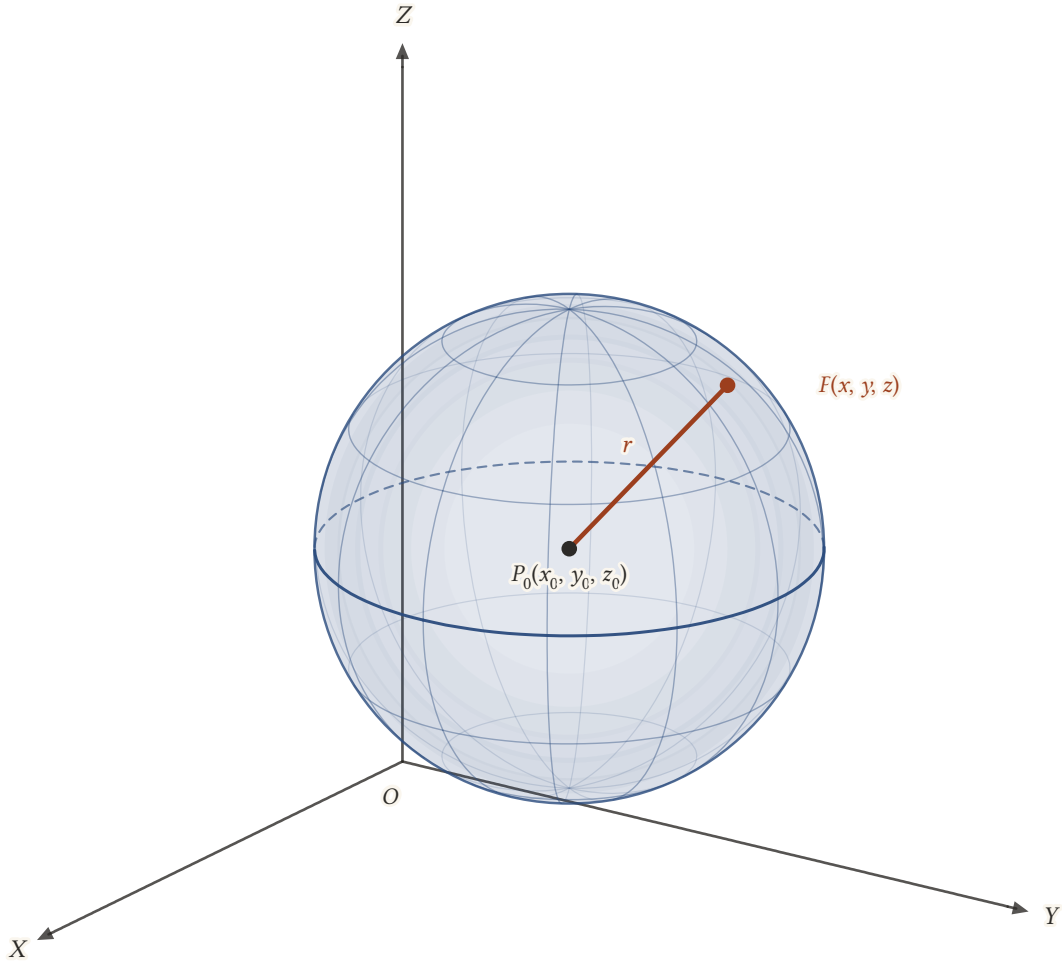
Şekil 6.12: P_0 noktasına uzaklığı r olan P noktaları, merkezi P_0 ve yarıçapı r olan küreyi oluşturur. Koyu çember kürenin ekvatorudur; arkada kalan yarısı kesiklidir.
