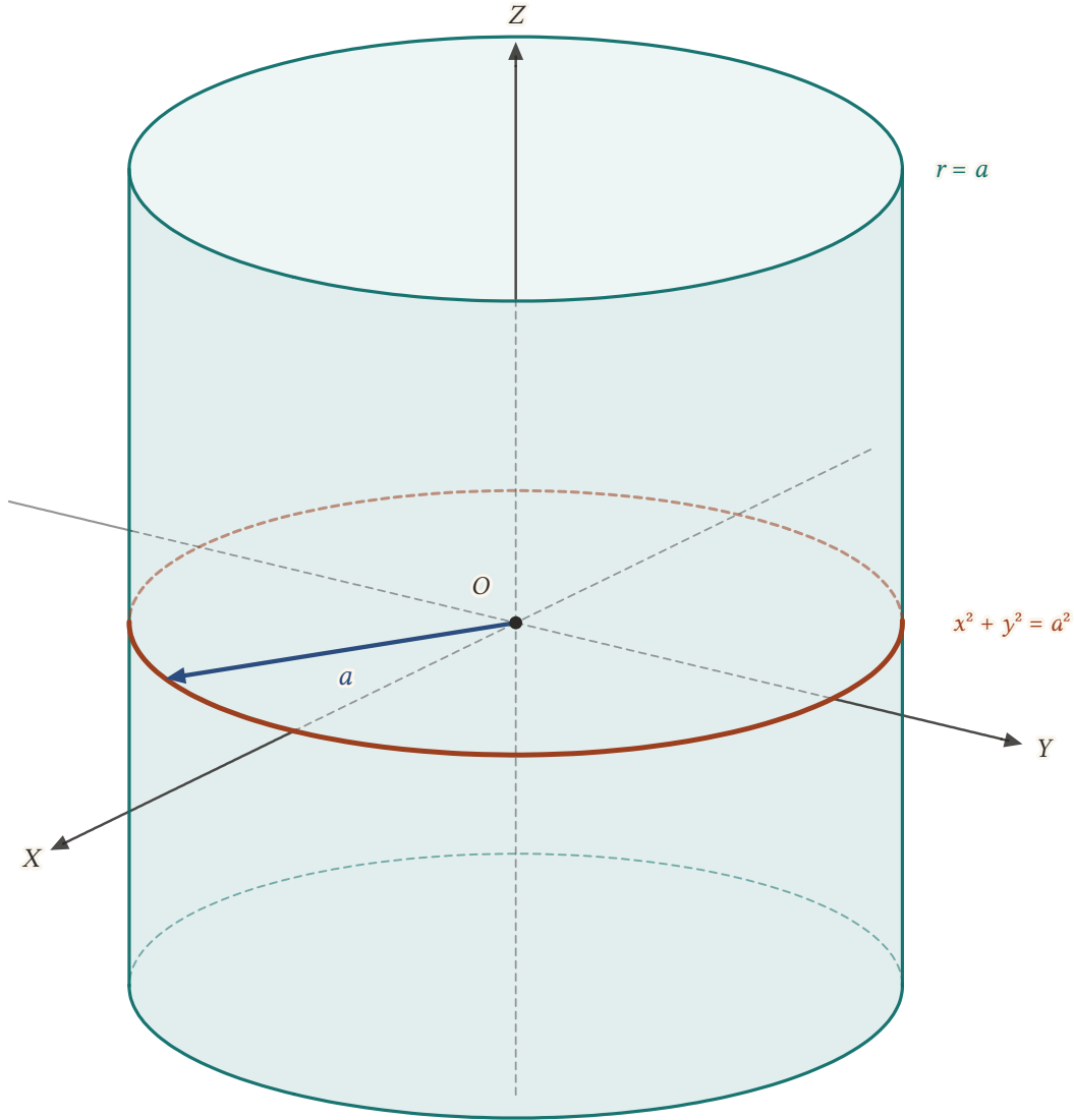
Şekil 22.2: r = a denkleminin grafiği: eksen Z -ekseni, yarıçapı a olan dik dairesel silindir (şekilde a = 2 ve -2 \leq z \leq 2,5 parçası). Kalın çember XY -düzlemindeki x^2 + y^2 = a^2 çemberidir; silindirin arkasında kalan çizgiler kesiklidir.
