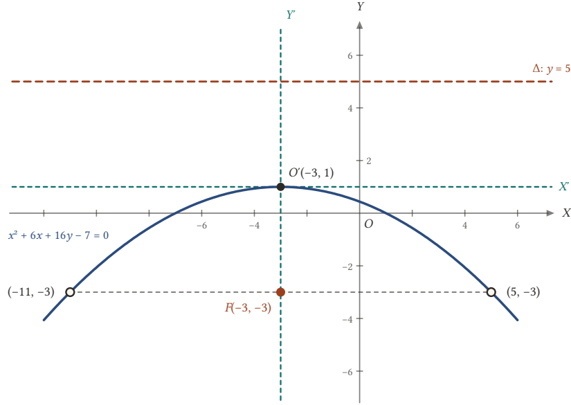
Şekil 20.16: Köşe O'(-3, 1) 'e öteleme denklemi x'^2 = -16y' yapar; parabol aşağı açılır, odak F(-3, -3) , doğrultman y = 5 .
