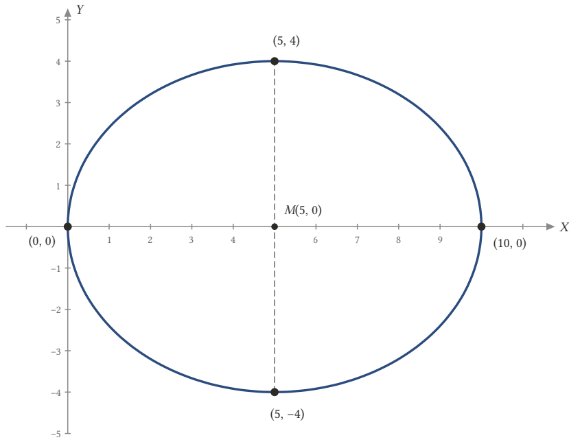
Şekil 18.27: Köşeleri (0, 0) , (10, 0) , (5, 4) , (5, -4) olan elipsin merkezi M(5, 0) : (x - 5)^2/25 + y^2/16 = 1 .
