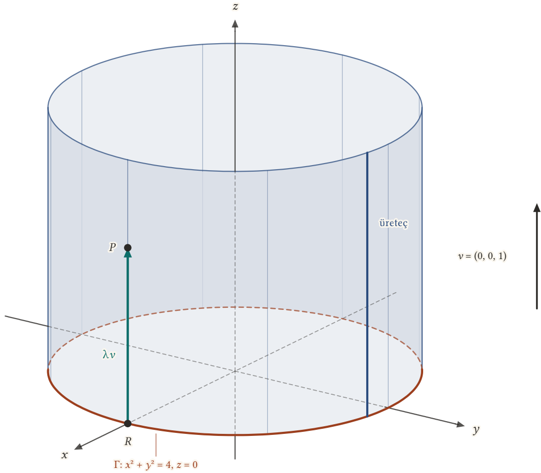
Şekil 23.4: Dayanak eğrisi xy -düzlemindeki \Gamma: x^2 + y^2 = 4 çemberi (kırmızı) olan ve üreteçleri v = (0, 0, 1) doğrultusunda olan dik dairesel silindir ( 0 \leq z \leq 3 parçası). P = R + \lambda v noktası, \Gamma üzerindeki R(2, 0, 0) noktasından geçen üreteçtedir.
