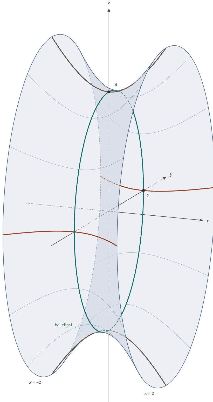
Şekil 23.28: Ekseni x -ekseni olan tek kanatlı hiperboloid -x^2/4 + y^2/9 + z^2/16 = 1 , |x| \leq 2 . Bel elipsi x = 0 düzleminde (yeşil; yarı eksenler 3 ve 4); x = \pm 2 'deki uç elipslerin yarı eksenleri 3\sqrt{2} ve 4\sqrt{2} 'dir. z = 0 ve y = 0 düzlemlerindeki izler hiperboldür (kırmızı ve kahverengi).
