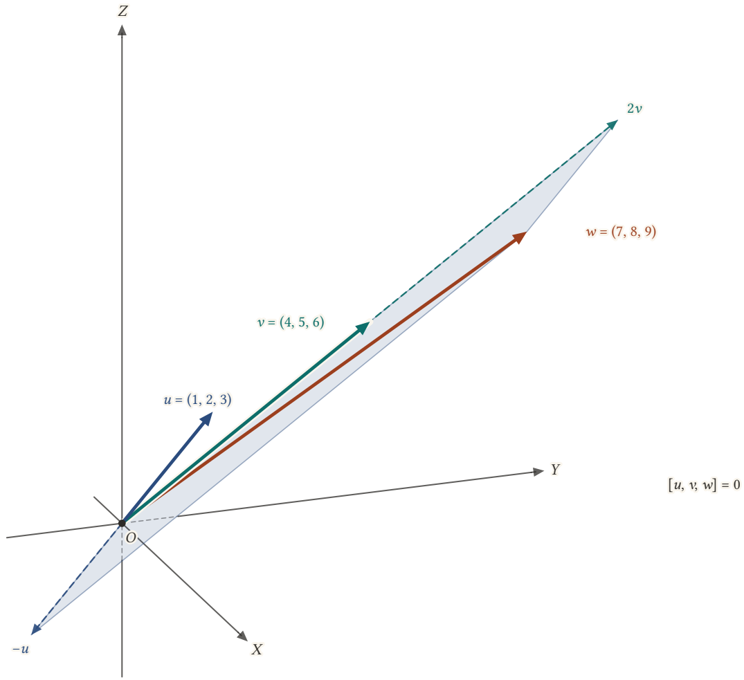
Şekil 9.11: u = (1, 2, 3) , v = (4, 5, 6) , w = (7, 8, 9) aynı düzlemindedir: w , -u ile 2v üzerine kurulan paralelkenarın köşegenidir, yani w = 2v - u .
