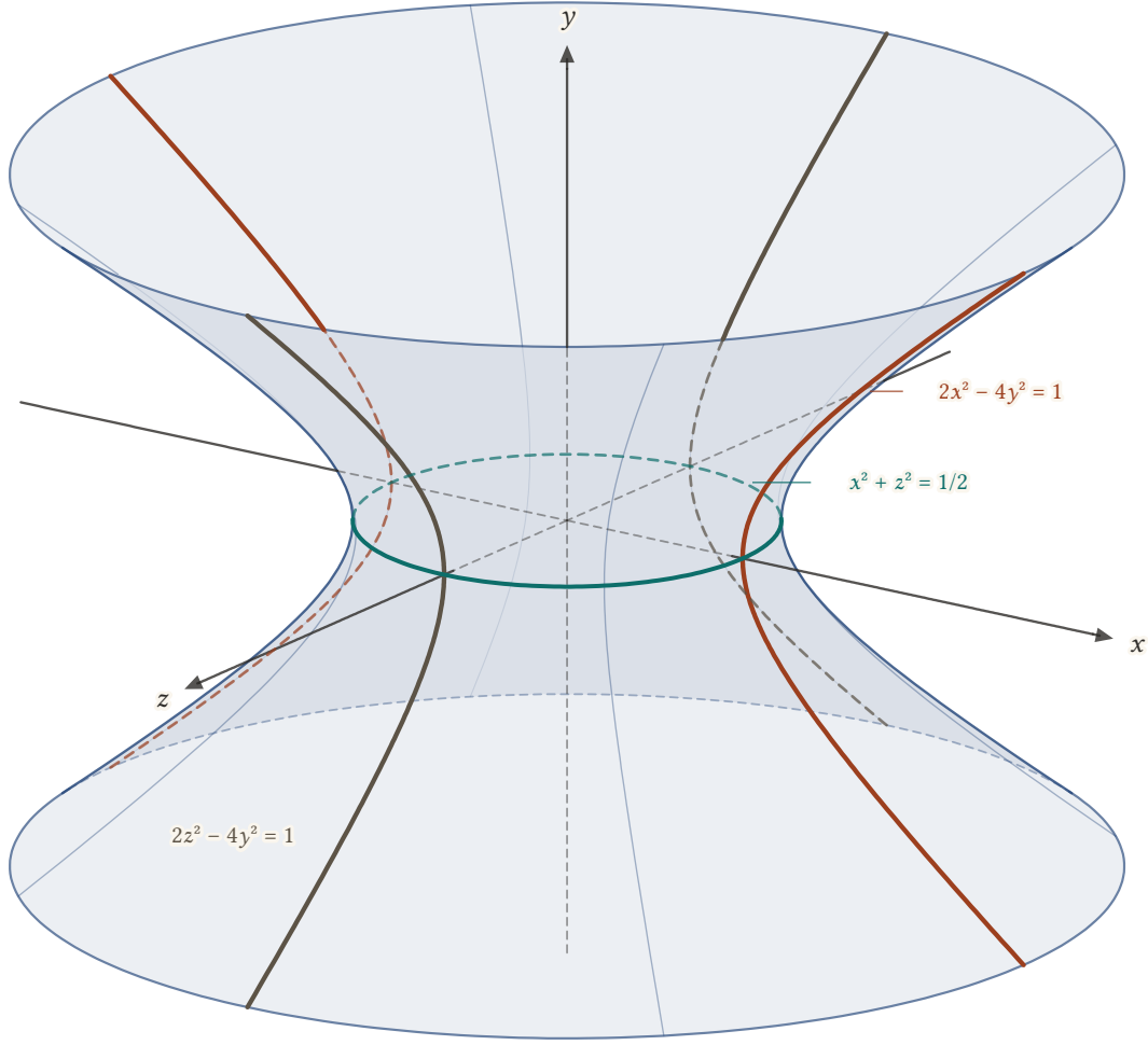
Şekil 23.15: Tek kanatlı dönel hiperboloid 2x^2 - 4y^2 + 2z^2 = 1 , -1,2 \leq y \leq 1,2 ( y -ekseni dikey). Bel çemberi x^2 + z^2 = 1/2 (yeşil); xy -düzlemindeki 2x^2 - 4y^2 = 1 hiperbolü (kırmızı) üretectir, yz -düzlemindeki iz 2z^2 - 4y^2 = 1 hiperbolüdür.
