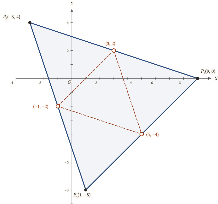
Şekil 1.37: Kenar orta noktaları (3, 2) , (-1, -2) ve (5, -4) olan üçgenin köşeleri P_1(9, 0) , P_2(-3, 4) ve P_3(1, -8) 'dir.
