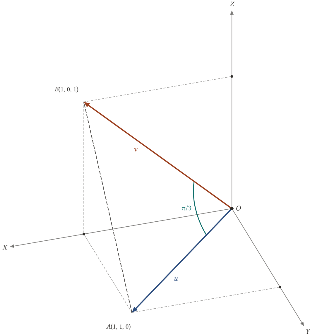
Şekil 8.4: u = (1, 1, 0) ve v = (1, 0, 1) başlangıç noktasından çizilir. O, A, B noktaları kenar uzunluğu \sqrt{2} olan bir eşkenar üçgenin köşeleridir; bu yüzden u ile v arasındaki açı \pi/3 'tür.
