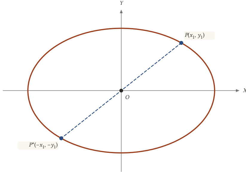
Şekil 21.7: Elipsin her noktasının O 'ya göre simetriği de elips üzerindedir.
