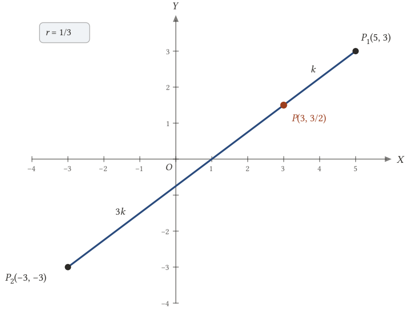
Şekil 2.8: P_1(5, 3) ve P_2(-3, -3) uç noktalı parçayı r = 1/3 oranında bölen nokta P(3, 3/2) ; P , P_2 'ye P_1 'e olduğundan üç kat uzaktır.
