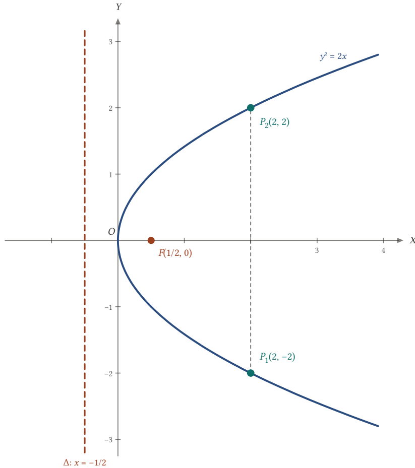
Şekil 20.6: P_1 ile P_2 X -eksenine göre simetrik olduğundan asal eksen X -eksenidir; parabol y^2 = 2x .
