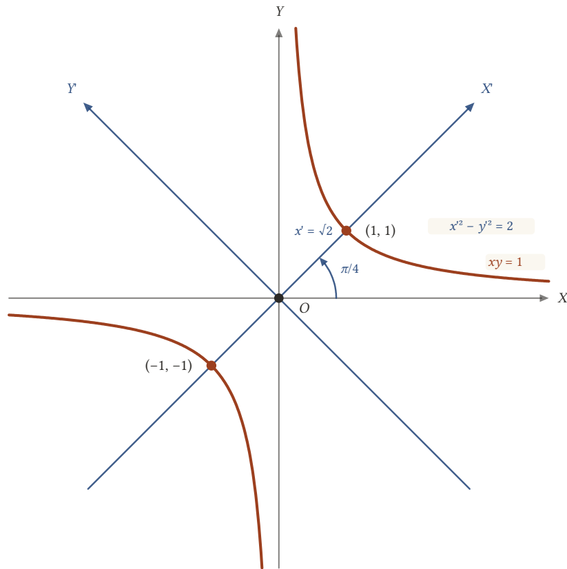
Şekil 17.14: Eksenler \pi/4 döndürülünce xy = 1 eğrisinin denklemi x'^2 - y'^2 = 2 olur; eğri yeni eksenlere göre simetrik durur.
