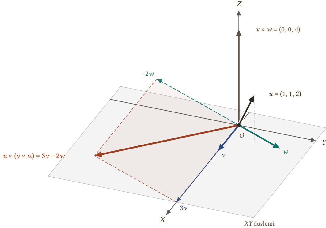
Şekil 9.3: u \times (v \times w) = (4, -4, 0) , XY düzleminde kalır: 3v ile -2w üzerine kurulan kesikli paralelkenarın köşegenidir, yani 3v - 2w 'ye eşittir. v \times w = (0, 0, 4) ise düzleme diktir.
