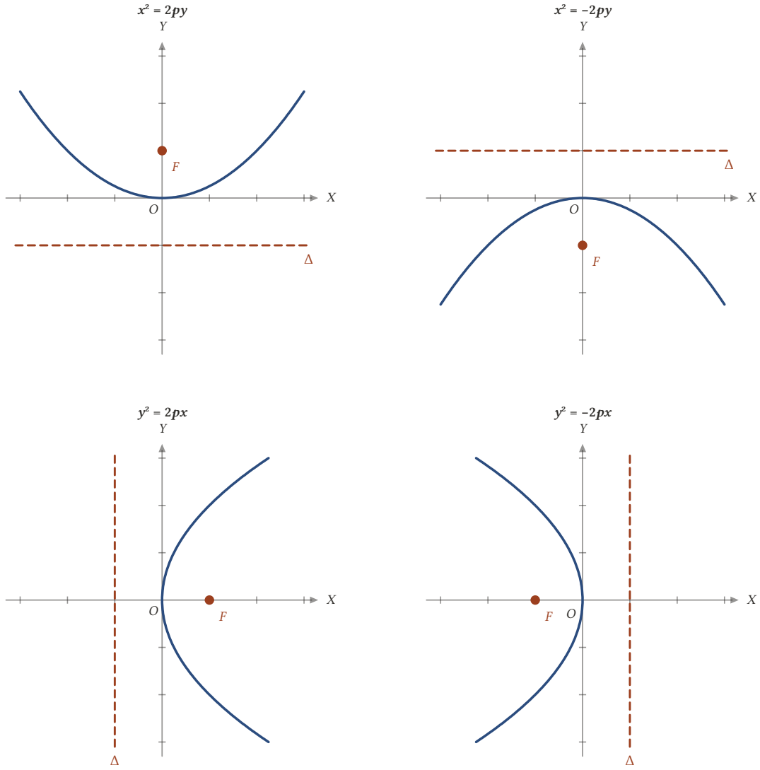
Şekil 20.3: Köşesi başlangıç noktasında olan parabolün dört konumu ( p = 2 ): birinci dereceden geçen değişken asal eksenini söyler, işaret açılma yönünü belirler.
