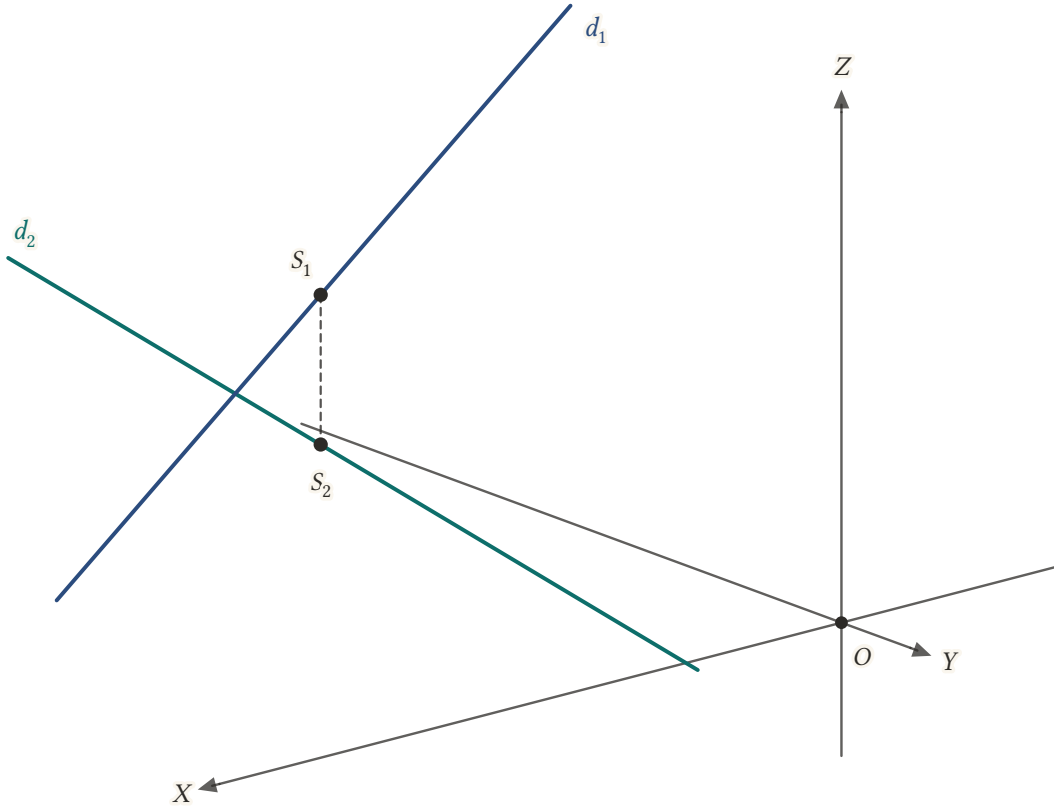
Şekil 10.11: Dik fakat kesişmeyen d_1 ve d_2 doğruları. S_1 ile S_2 aynı dikey doğru üzerindedir; d_1, d_2 'nin 9/8 birim üstünden geçer.
