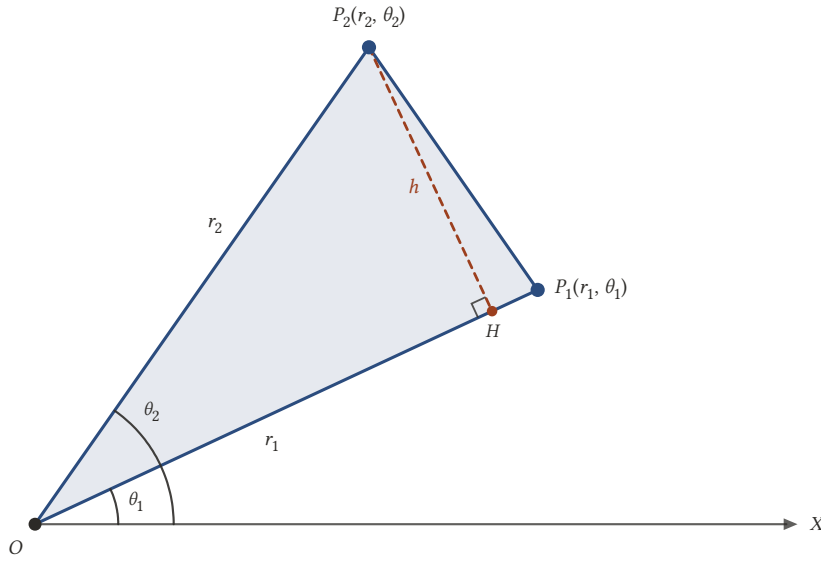
Şekil 5.12: Kutupsal koordinatlarda üçgenin alanı: taban |OP_1| = r_1 , yükseklik h = r_2 \sin(\theta_2 - \theta_1) .
