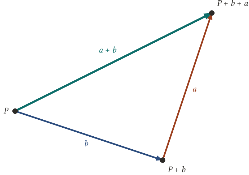
Şekil 16.3: Önce b, sonra a kadar ötelemek, a + b kadar tek bir ötelemeye eşittir.
