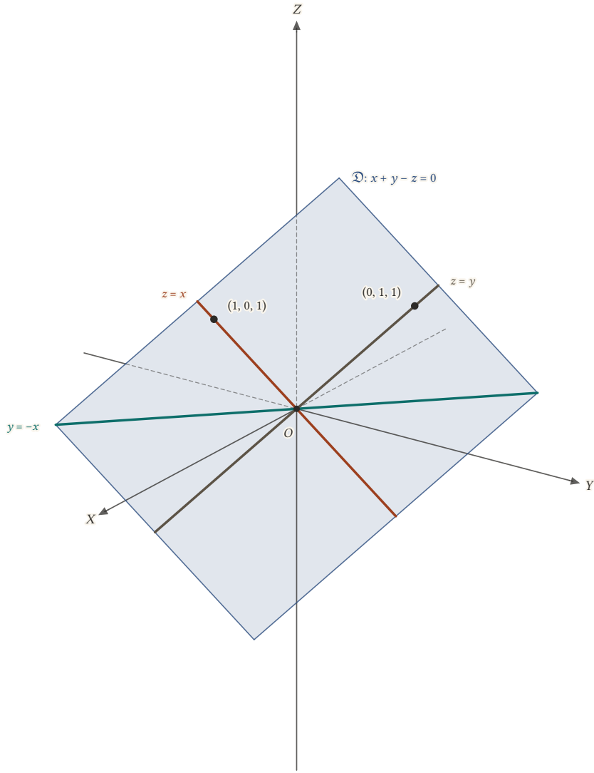
Şekil 13.12: x + y - z = 0 düzlemi orijinden geçer; onu üç iziyle çizeriz: XY -düzleminde y = -x , XZ -düzleminde z = x , YZ -düzleminde z = y . Yama, |x|, |y| \leq 1,2 olan parçadır.
