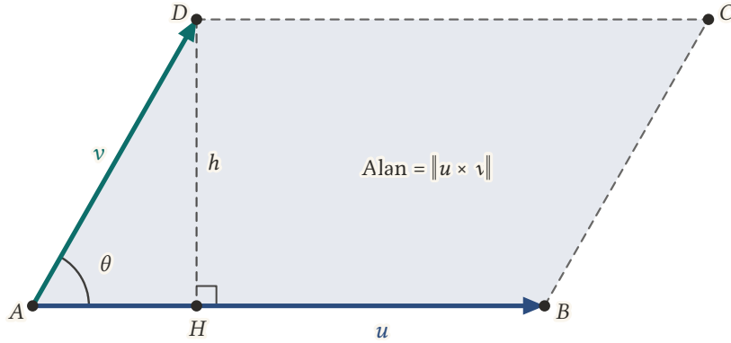
Şekil 9.6: ABCD paralelkenarında taban |AB| = \|u\| , yükseklik h = |DH| = \|v\| \sin \theta 'dir; alan \|u\| h = \|u \times v\| olur.
