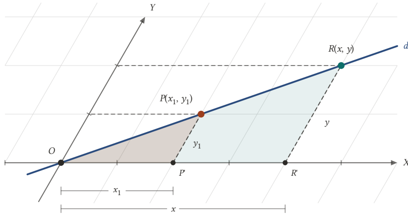
Şekil 5.19: Eğik sistemde başlangıçtan geçen d doğrusu: OPP ve OR'R üçgenleri benzer olduğundan x/x_1 = y/y_1 , yani y = mx .
