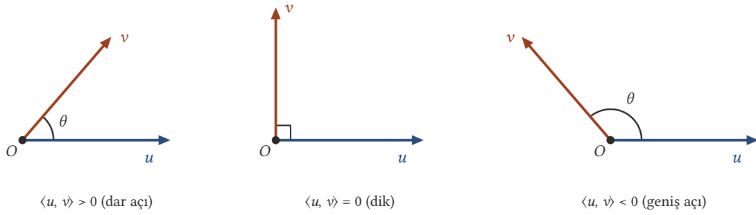
Şekil 8.6: İç çarpımın işareti açığı belirler: pozitifse açı dar, sıfırsa dik, negatifse geniştir.
