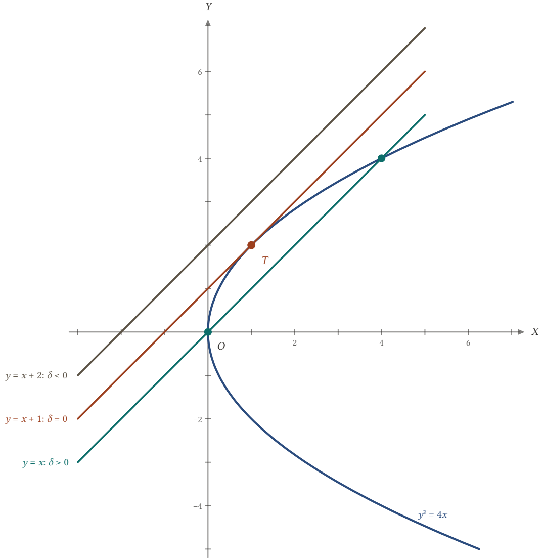
Şekil 20.10: y^2 = 4x parabolü ve eğimi 1 olan üç doğru: \delta = 4p(p - 2mn) = 8(2 - 2n) işaretine göre kesen, teğet (değme noktası T(1, 2) ) ve kesmeyen doğru.
