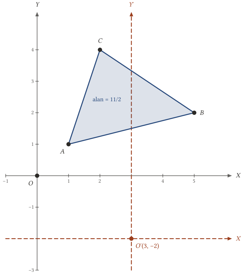
Şekil 16.12: ABC üçgeninin alanı eski sistemde de, eksenler (3, -2) kadar ötelendikten sonra da 11/2 'dir.
