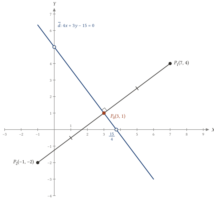
Şekil 3.5: P_1P_2 parçasının orta dikmesi: \bar{d} doğrusu orta nokta P_0(3, 1) 'den geçer ve parçaya diktir. Eşitlik çentikleri iki yarının eşit olduğunu gösterir.
