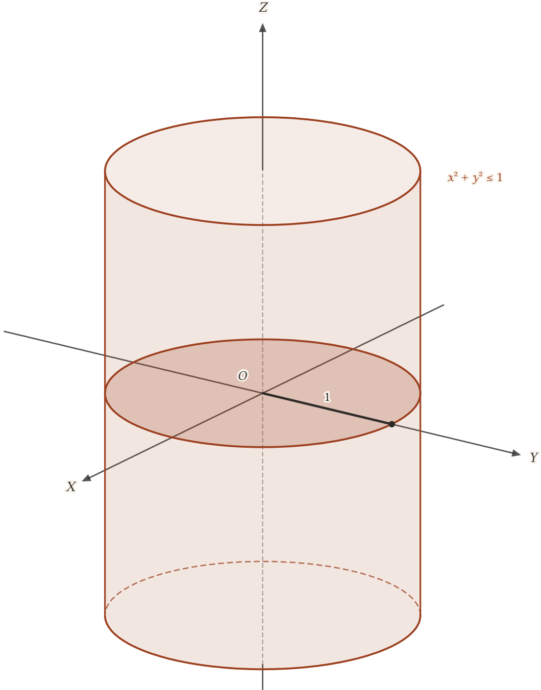
Şekil 6.9: x^2 + y^2 \leq 1 kümesi: Z-ekseni çevresindeki, yarıçapı 1 olan dolu silindir ( -1,5 \leq z \leq 1,5 parçası). Koyu taralı daire XY-düzlemindeki kesittir; aynı daire her yükseklikte tekrarlanır.
