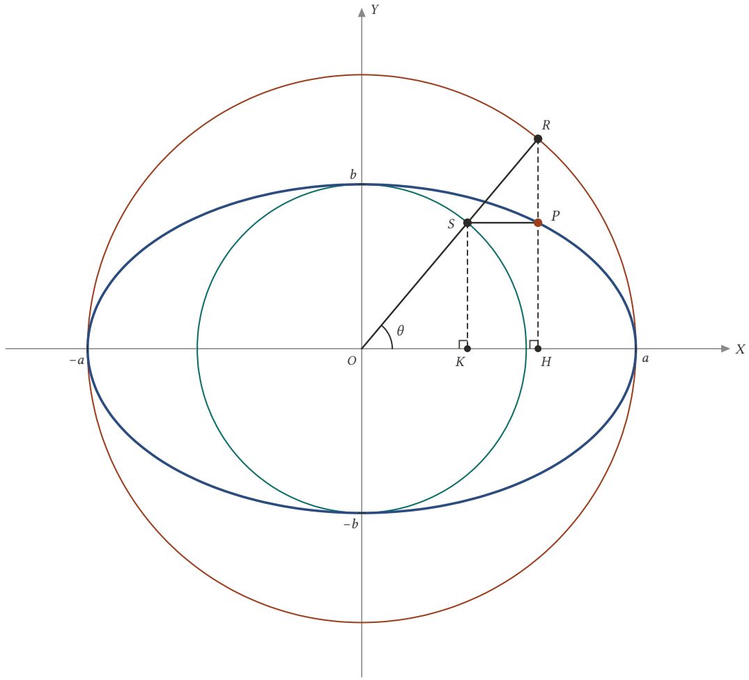
Şekil 18.21: P'nin apsisi R'den, ordinatı S'den gelir: P = (a \cos \theta, b \sin \theta) .
