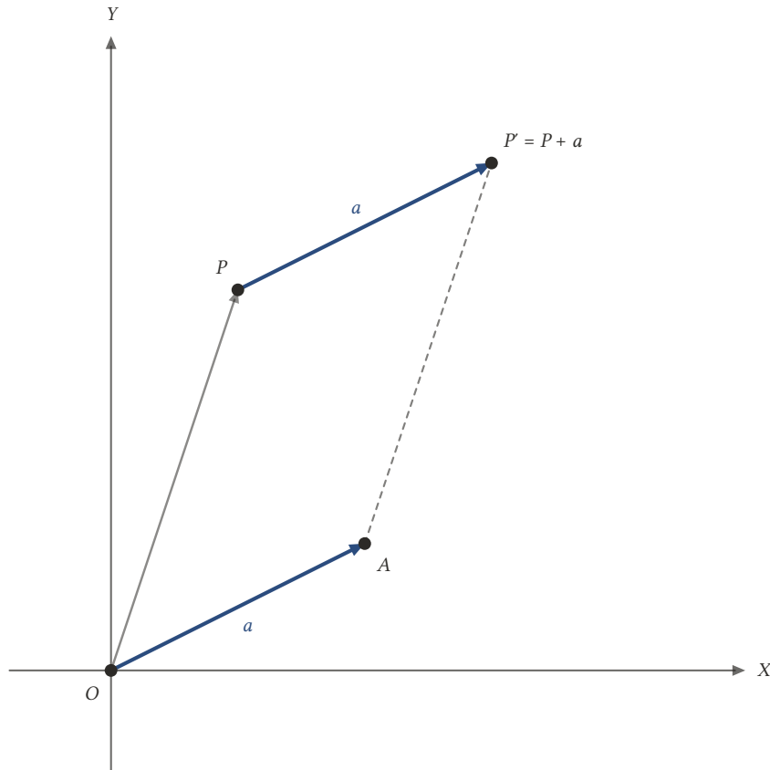
Şekil 16.1: f_a ötelenmesi P noktasını a = \overrightarrow{OA} vektörü kadar kaydırır: OA ve PP' okları paralel ve eşit uzunluktadır.
