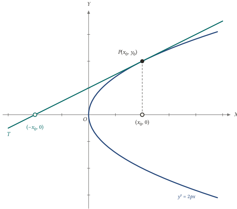
Şekil 20.8: y^2 = 2px parabolünün P(x_0, y_0) noktasındaki teğeti y_0 y = p(x + x_0) ; teğet X -eksenini (-x_0, 0) 'da keser (çizimde p = 1 , P(2, 2) ).
