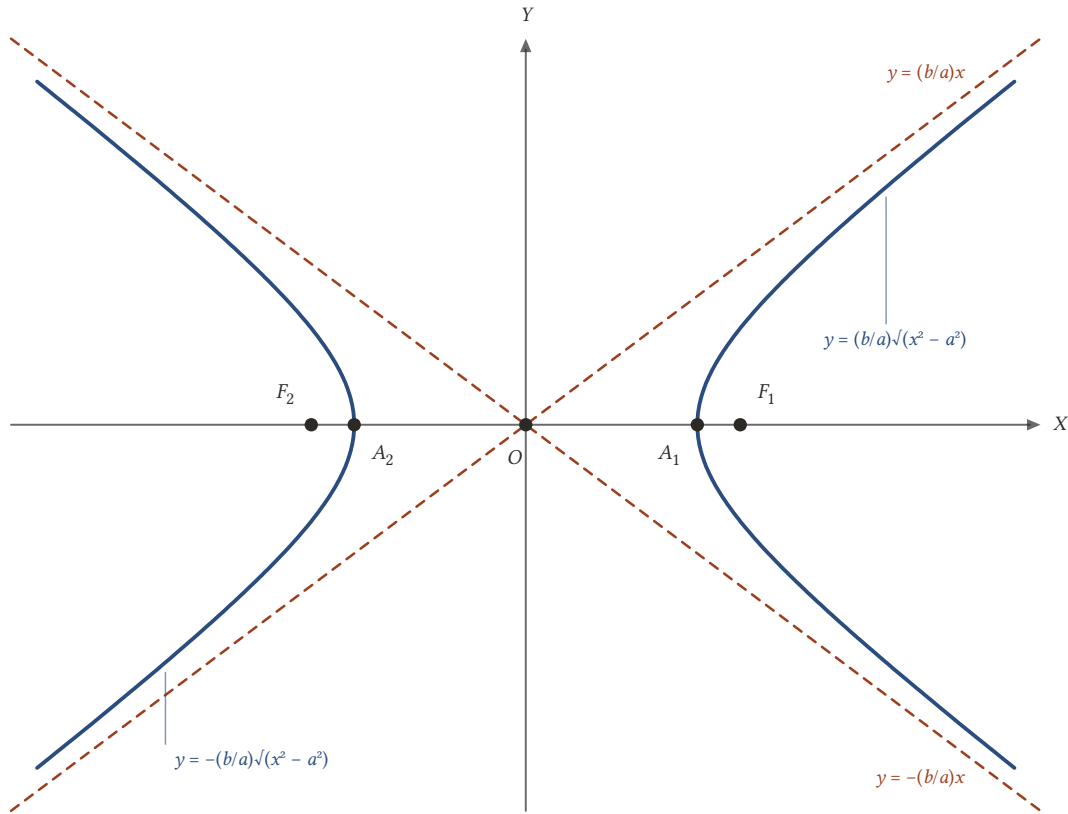
Şekil 19.3: Kollar uzaklaştıkça merkezden geçen iki asimptota yaklaşır.
