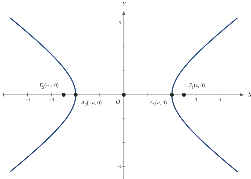
Şekil 19.2: Merkezi O, asal eksen X-ekseni olan hiperbol: köşeler (\pm a, 0) , odaklar (\pm c, 0) .
