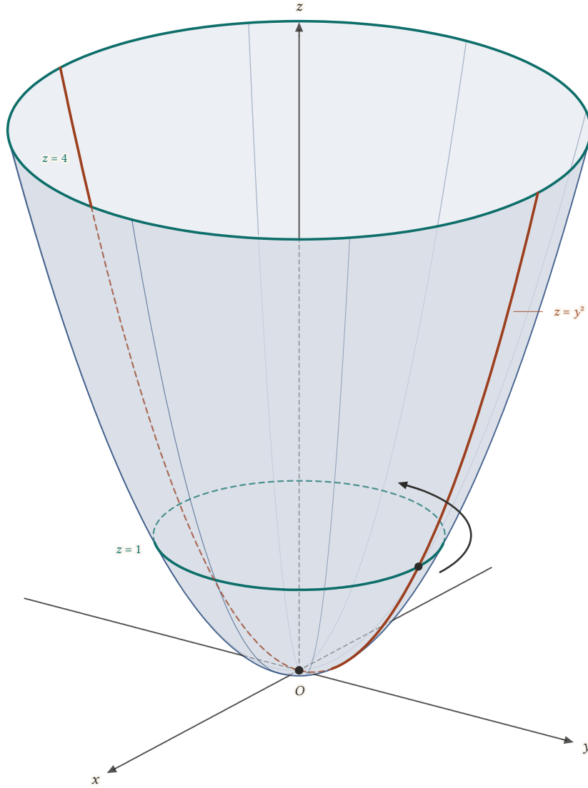
Şekil 23.34: yz -düzlemindeki z = y^2 parabolünün (kırmızı) z -ekseni etrafında döndürülmesiyle oluşan dönel paraboloid z = x^2 + y^2 , 0 \leq z \leq 4 . z = 1 ve z = 4 izleri yarıçapları 1 ve 2 olan çemberlerdir (yeşil); ok, (0, 1, 1) noktasının dönerken izlediği yolu gösterir.
