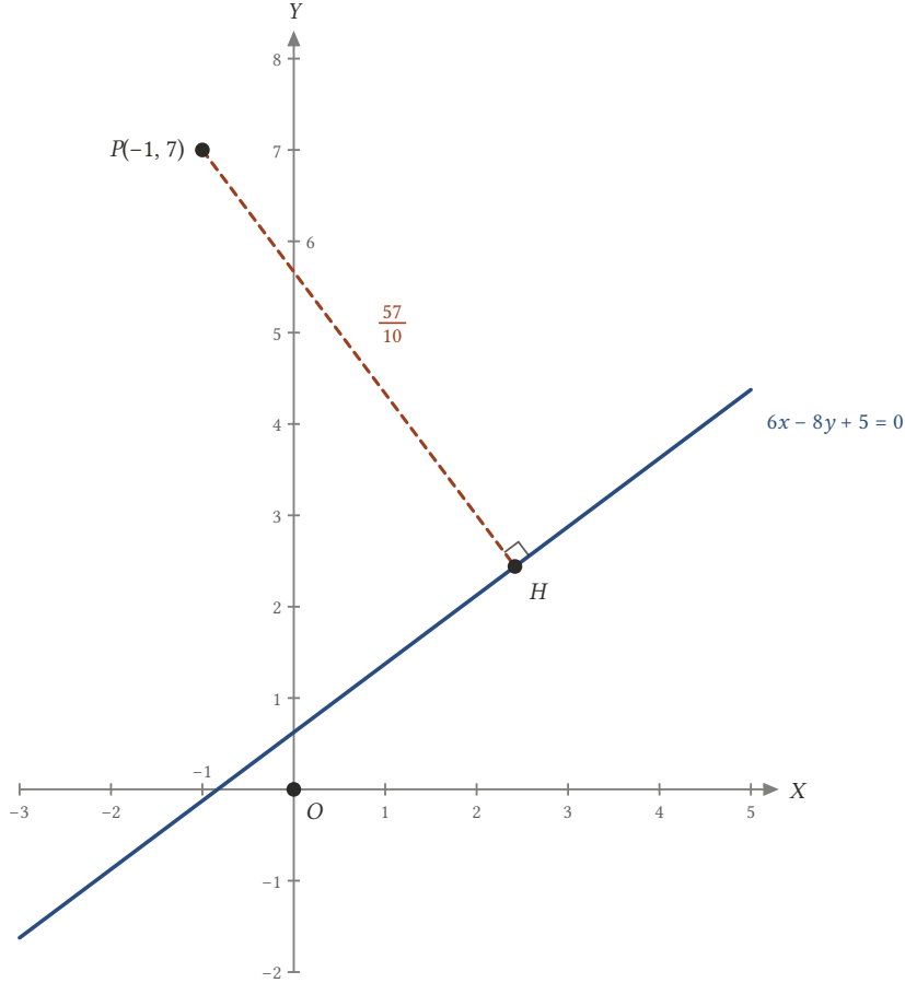
Şekil 3.18: P(-1, 7) noktasının 6x - 8y + 5 = 0 doğrusuna uzaklığı |PH| = 57/10 'dur; s > 0 olduğundan P ile orijin doğrunun farklı taraflarındadır.
