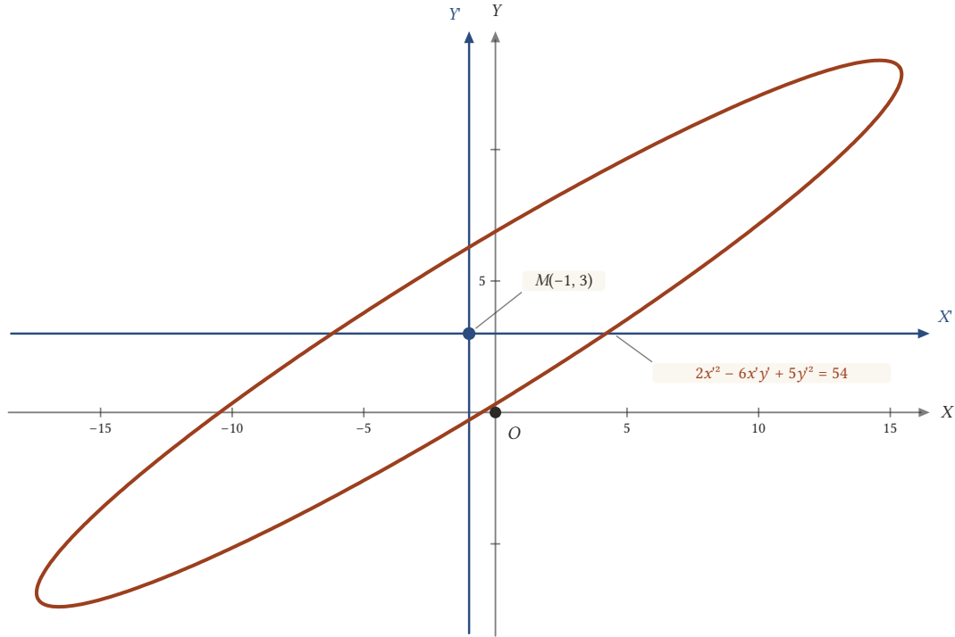
Şekil 21.19: Elipsin merkezi M(-1, 3) ; eksenler M 'ye ötelenince birinci dereceden terimler kaybolur.
