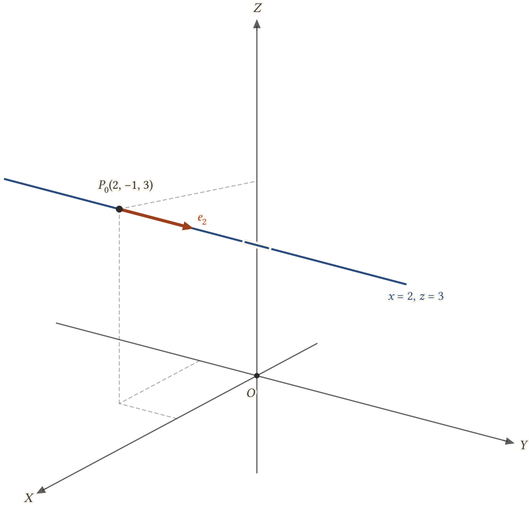
Şekil 12.17: P_0(2, -1, 3) noktasından geçen ve Y -eksenine paralel olan doğru; doğrultmanı e_2 'dir.
