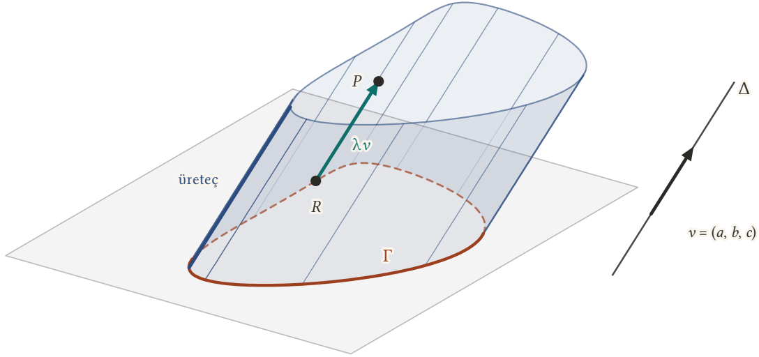
Şekil 23.3: Silindir: dayanak eğrisi \Gamma (kırmızı) boyunca kayan ve \Delta doğrusuna (doğrultman vektörü v ) paralel kalan doğrular, yani üreteçler yüzeyi örer. \Gamma üzerindeki R noktasının üretecindeki her P noktası için RP = \lambda v olur.
