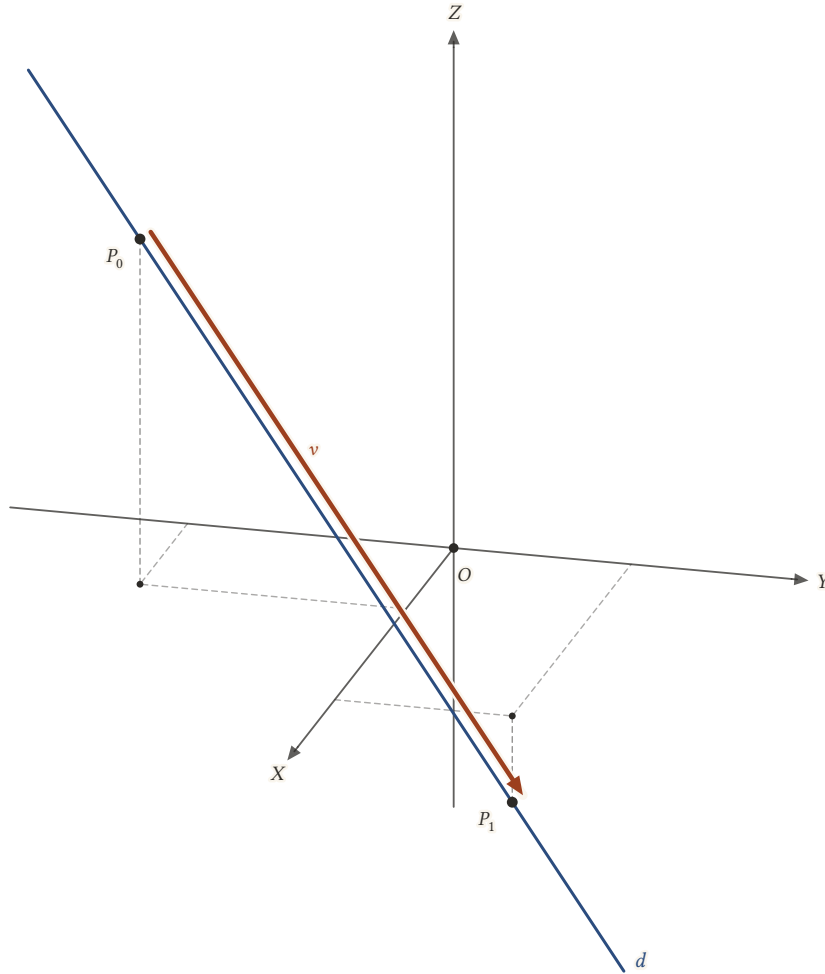
Şekil 10.6: P_0 = (2, -3, 4) ile P_1 = (5, 2, -1) noktalarından geçen doğru ve doğrultmanı v = (3, 5, -5) . Kesikli çizgiler noktaları XY düzlemine bağlar.
