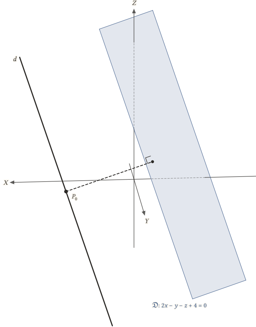
Şekil 14.7: d doğrusu düzleme paraleldir ( \langle n, v \rangle = 0 ) ama P_0(2, 1, 0) düzlemde değildir; doğru düzlemin yanından geçer ve onu hiç kesmez. Kesikli çizgi P_0 'dan düzleme inen dikmedir.
