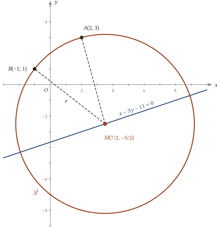
Şekil 4.7: Merkezi M(7/2, -5/2) ve yarıçapı \sqrt{65/2} olan çember A ile B 'den geçer; merkezi x - 3y - 11 = 0 doğrusu üzerindedir.
