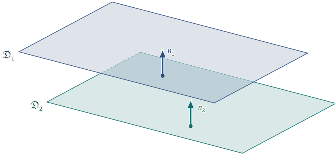
Şekil 13.1: Paralel iki düzlem: normal vektörleri n_1 ile n_2 aynı doğrultudadır. Alttaki düzlemin üsttekinin arkasında kalan kenarları kesiklidir.
