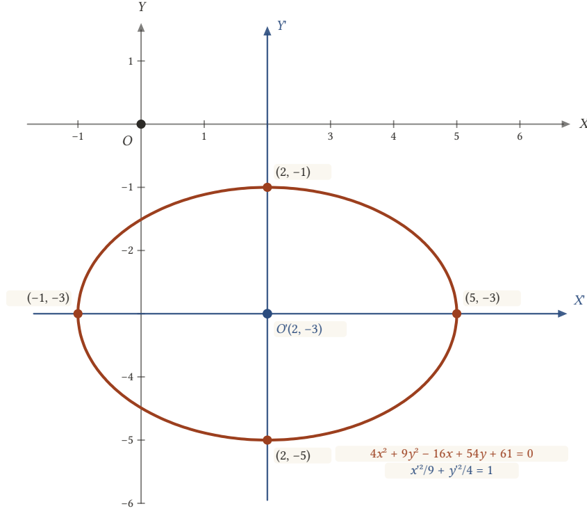
Şekil 21.1: Eksenler O'(2, -3) 'e ötelenince birinci dereceden terimler kaybolur ve elipsin standart denklemi ortaya çıkar.
