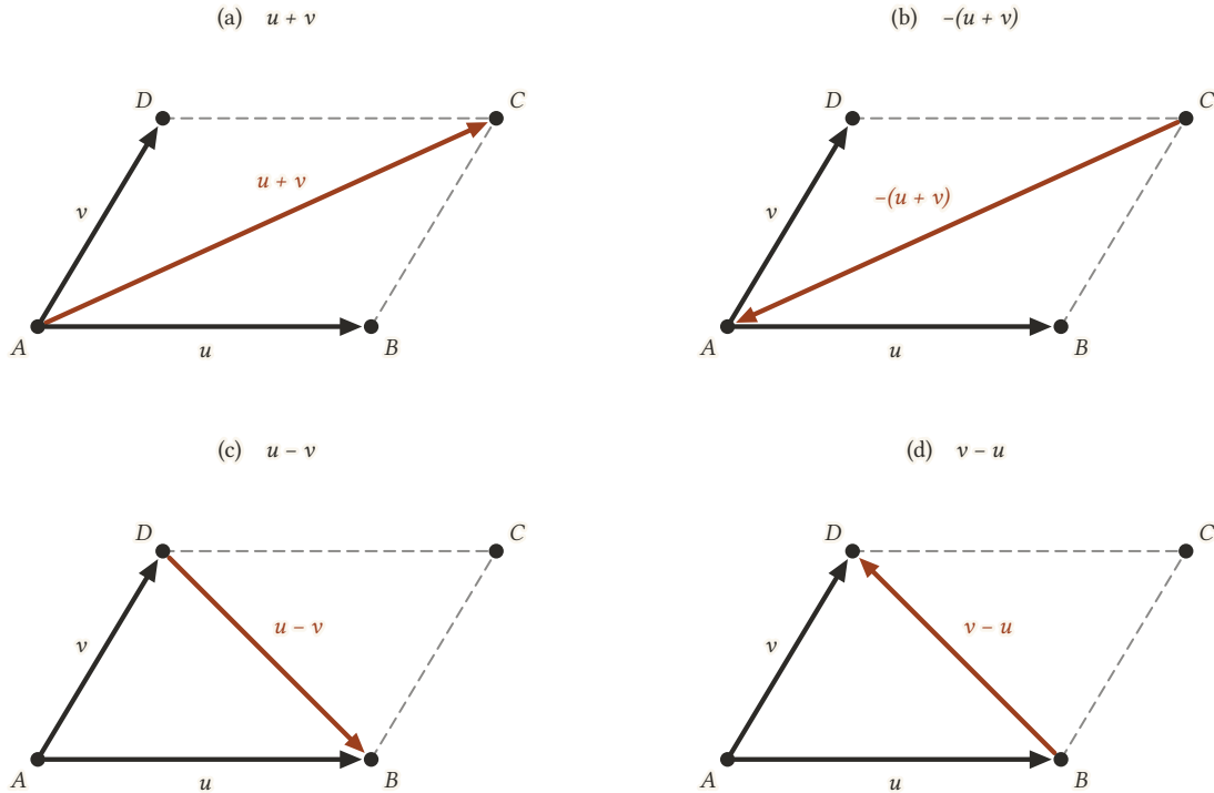
Şekil 7.13: u ve v üzerine kurulan paralelkenarın köşegen vektörleri: (a) AC = u + v , (b) CA = -(u + v) , (c) DB = u - v , (d) BD = v - u .
