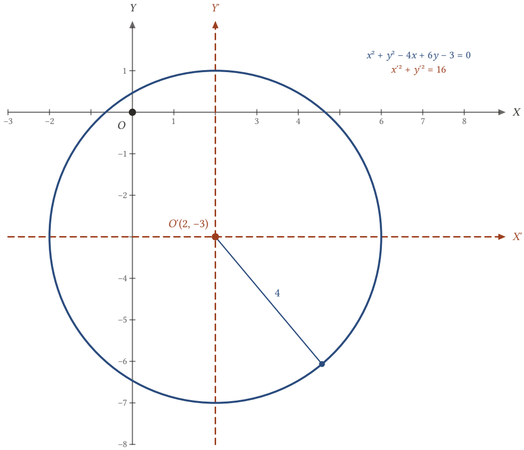
Şekil 16.14: Eksenler çemberin merkezi O'(2, -3) noktasına ötelenince denklem x'^2 + y'^2 = 16 olur.
