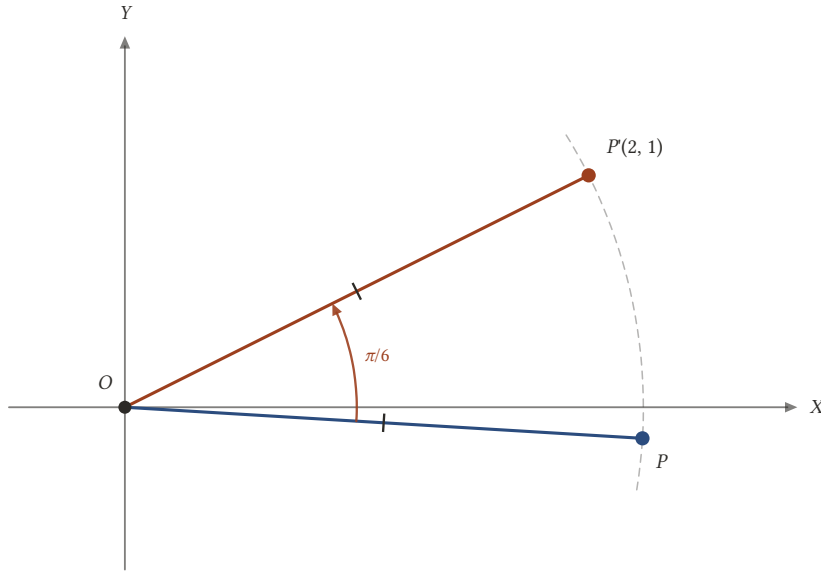
Şekil 17.20: O etrafında \pi/6 döndürülünce P(2, 1) 'e giden nokta P((2\sqrt{3}+1)/2, (\sqrt{3}-2)/2) 'dir; |OP| = \sqrt{5} .
