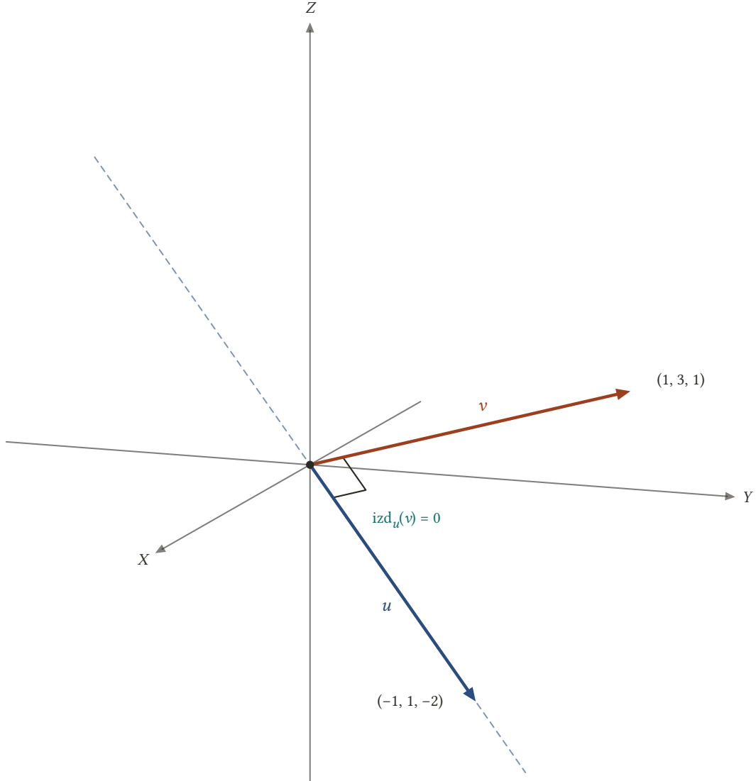
Şekil 8.9: v = (1, 3, 1) , u = (-1, 1, -2) doğrultusuna diktir. v 'nin ucundan u doğrultusuna inen dikmenin ayağı başlangıç noktasıdır; izdüşüm sıfır vektörüdür.
