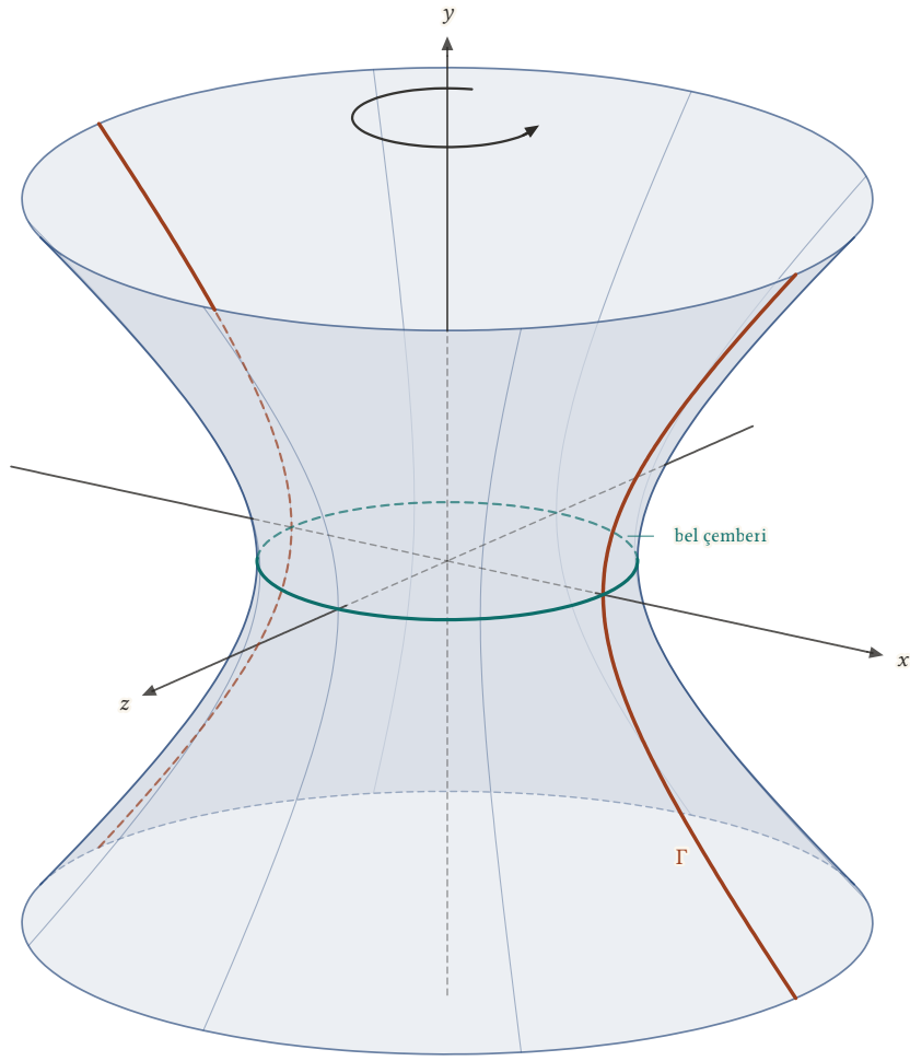
Şekil 23.14: a = b = 1 için x^2 - y^2 = 1 hiperbolünün (kırmızı, \Gamma ) y -ekseni etrafında döndürülmesiyle oluşan tek kanatlı hiperboloid x^2 - y^2 + z^2 = 1 , -2 \leq y \leq 2 . Yeşil çember y = 0 'daki bel çemberidir; uçlardaki çemberlerin yarıçapı \sqrt{5} 'tir.
