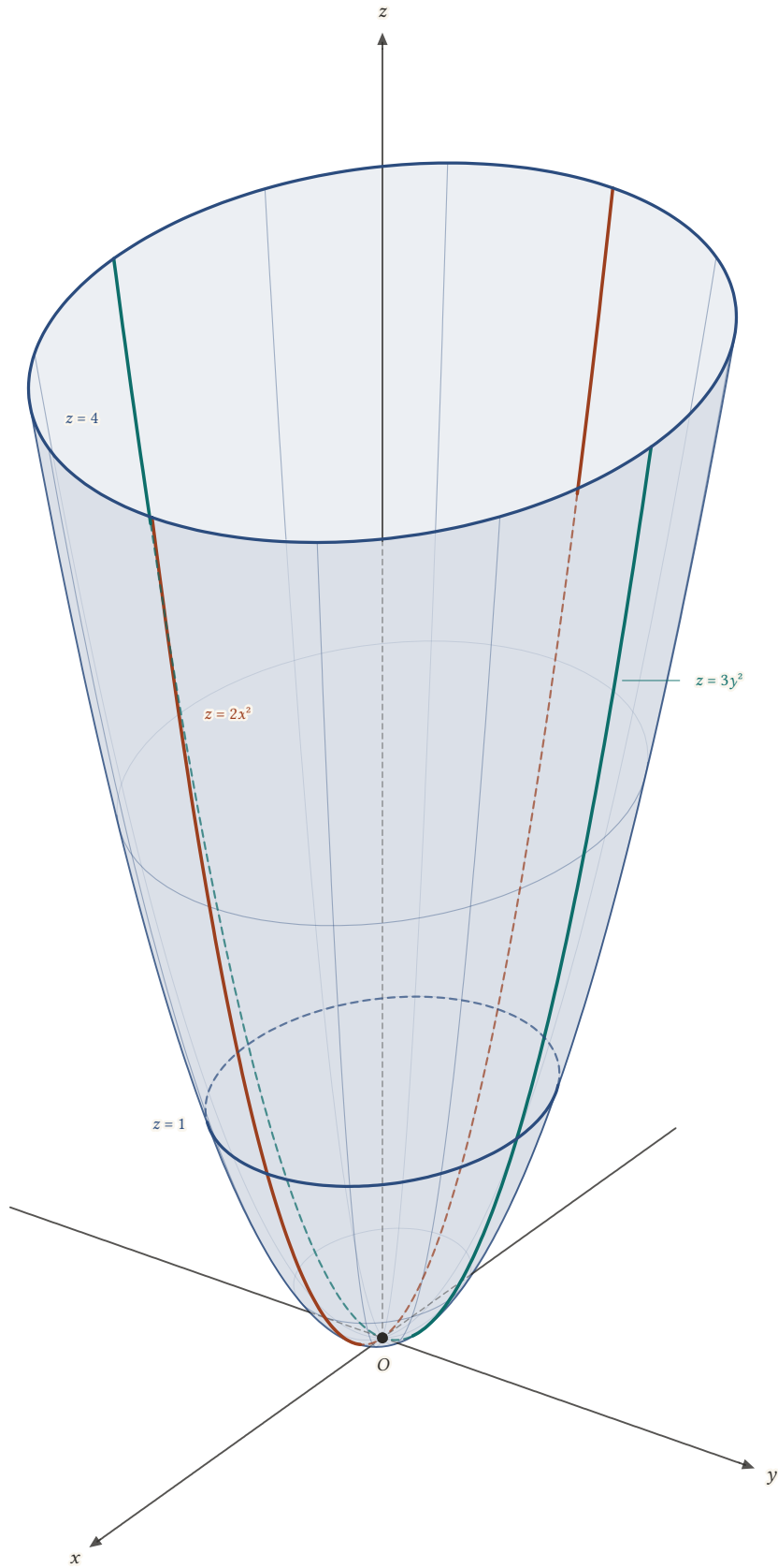
Şekil 23.19: Eliptik paraboloid 2x^2 + 3y^2 = z , 0 \leq z \leq 4 . xz - ve yz -düzlemlerindeki izler z = 2x^2 (kırmızı) ve z = 3y^2 (yeşil) parabolleridir; z = 1 ve z = 4 düzlemlerindeki izler elipstir. Köşe O 'dur.
