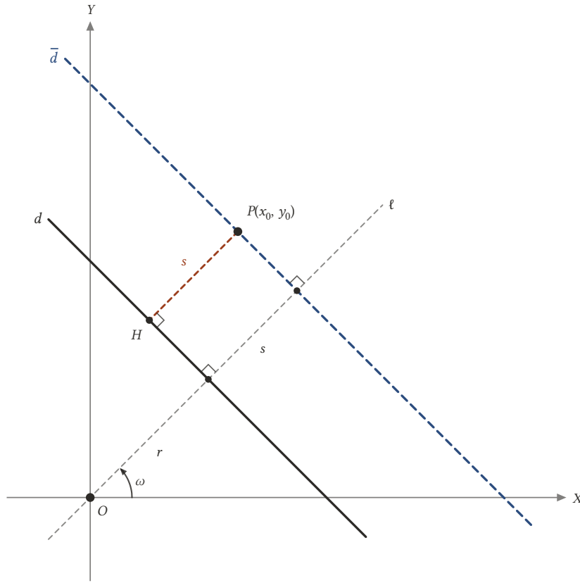
Şekil 3.11: Birinci konum: P, d'nin orijinle karşı tarafındadır. P'den geçen paralel \bar{d} , \ell dikmesini Q_{r+s} 'de keser; P'nin d'ye uzaklığı iki paralel arasındaki s uzaklığıdır.
