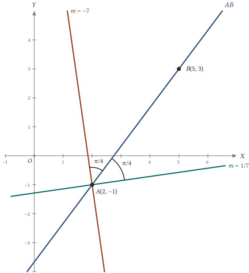
Şekil 2.31: AB doğrusuyla \pi/4 'lük açı yapan iki yön vardır: eğimi -7 ve eğimi 1/7 olan doğrular (burada A 'dan geçecek biçimde çizildi). Bu iki doğru birbirine diktir.
