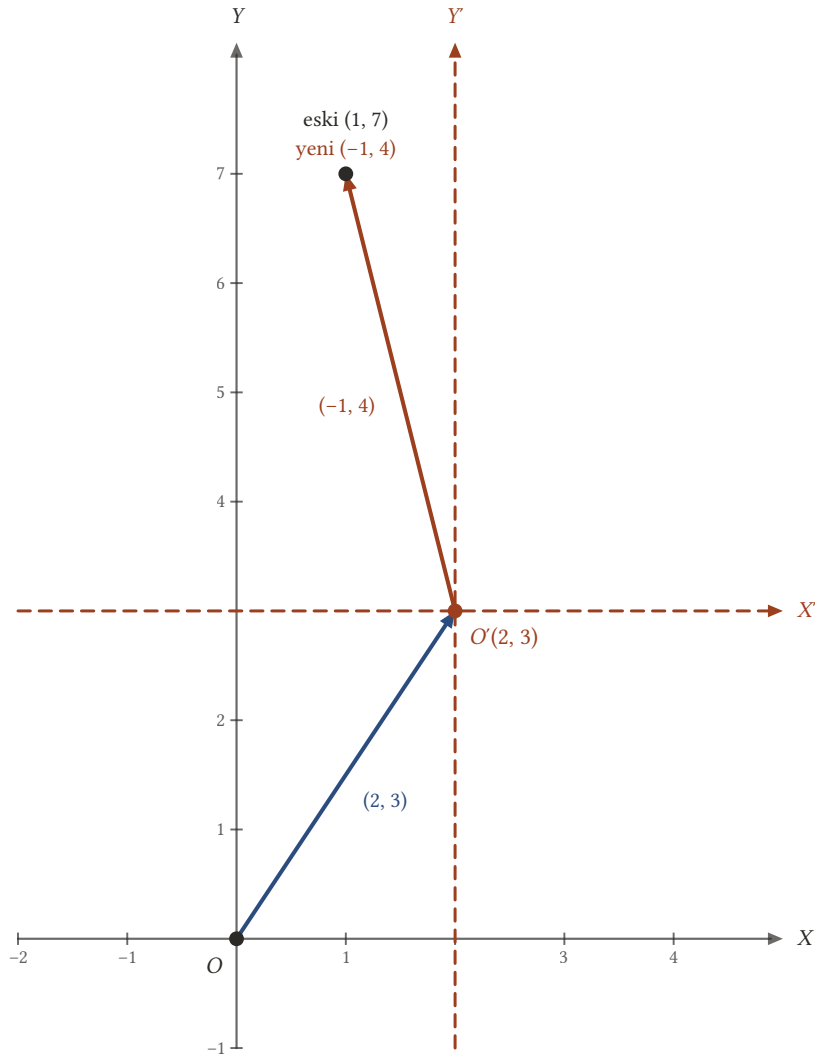
Şekil 16.10: Yeni koordinatları (-1, 4) olan nokta, eski sistemde (2, 3) + (-1, 4) = (1, 7) noktasıdır.
