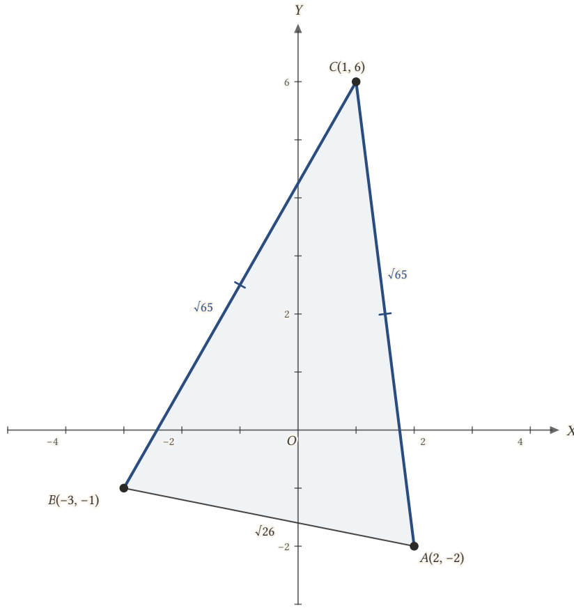
Şekil 1.13: |BC| = |CA| = \sqrt{65} : tepe noktası C olan ikizkenar üçgen.
