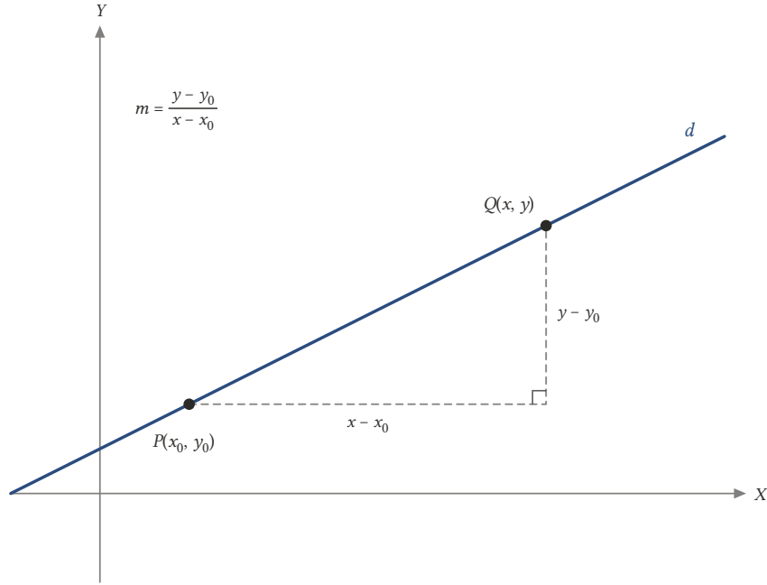
Şekil 3.1: Nokta-eğim denklemi: d doğrusu üzerindeki her Q(x, y) noktası için P den Q ya giden parçanın eğimi aynı m sayıdır. Kesikli dik üçgenin kenarları x - x_0 ve y - y_0 'dur.
