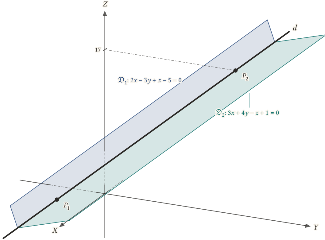
Şekil 13.4: İki düzlemin arakesit doğrusu d , ortak noktalar P_1(1, -1, 0) ve P_2(0, 4, 17) 'den geçer; iki şerit, düzlemlerin d 'yi içeren parçalarıdır. Şekil sığsın diye Z -ekseni dörtte bir ölçekle çizilmiştir.
