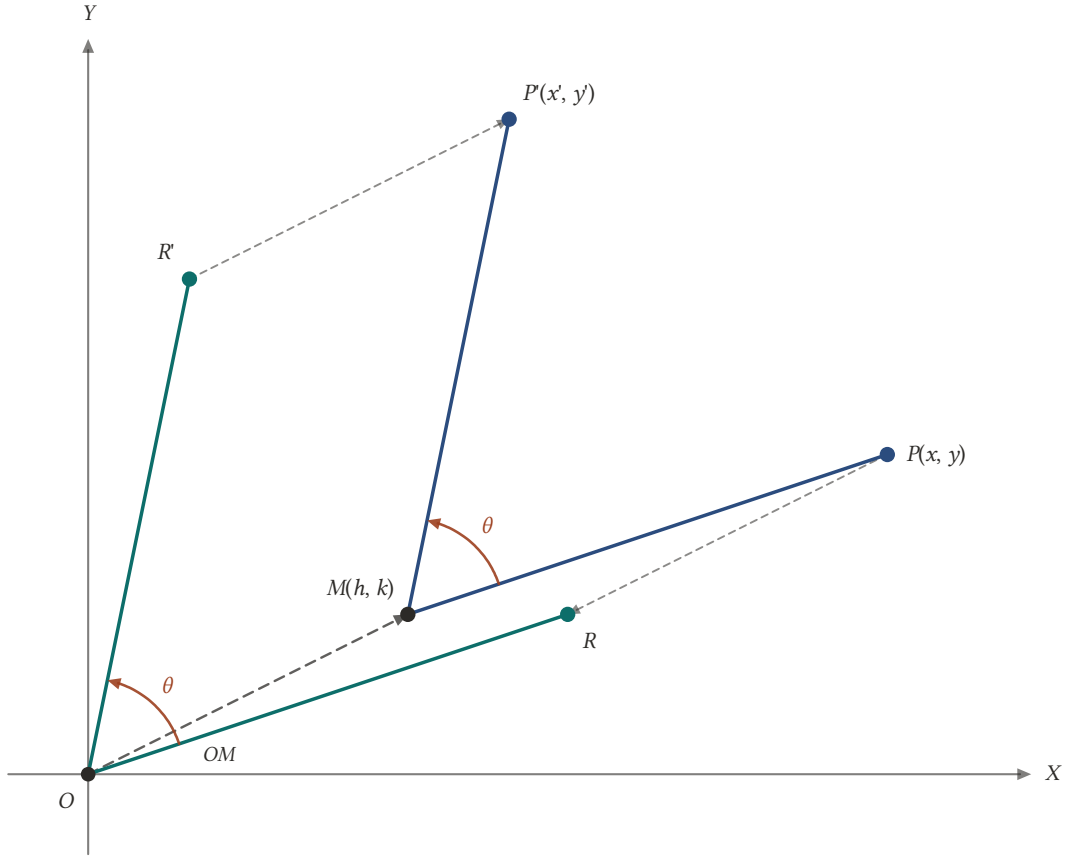
Şekil 17.5: P önce -OM kadar ötelenip R' 'ye, R başlangıç etrafında \theta döndürülüp R' 'ne, R' de OM kadar ötelenip P' 'ne götürülür.
