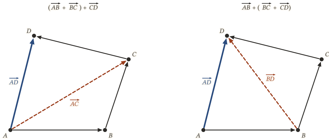
Şekil 7.20: Solda önce AB ile BC birleştirilip AC , sağda önce BC ile CD birleştirilip BD bulunur; iki yol da A 'dan D 'ye varır.
