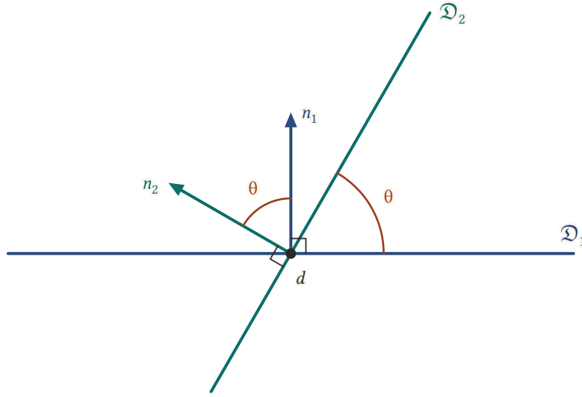
Şekil 13.7: Arakesit doğrusuna dik bir kesit: d bir nokta, düzlemler iki doğru, normaller bu doğrulara dik iki ok olarak görünür. Normaller arasındaki açı ile doğrular arasındaki açı aynı \theta açısıdır.
