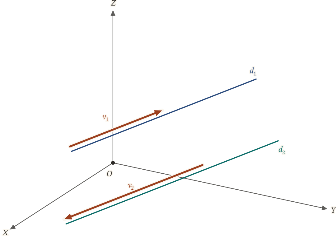
Şekil 10.8: Doğrultmanları paralel olan d_1 ve d_2 doğruları. Burada v_2 = -1,5 v_1 olduğundan iki doğrultman zıt yönlüdür; doğrular yine paraleldir.
