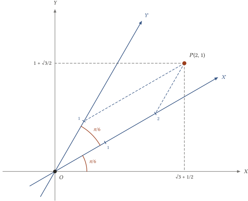
Şekil 17.17: \theta = \alpha = \pi/6 olan eğik sistemde paralel koordinatları (2, 1) olan noktanın dik koordinatları (\sqrt{3} + 1/2, 1 + \sqrt{3}/2) 'dir.
