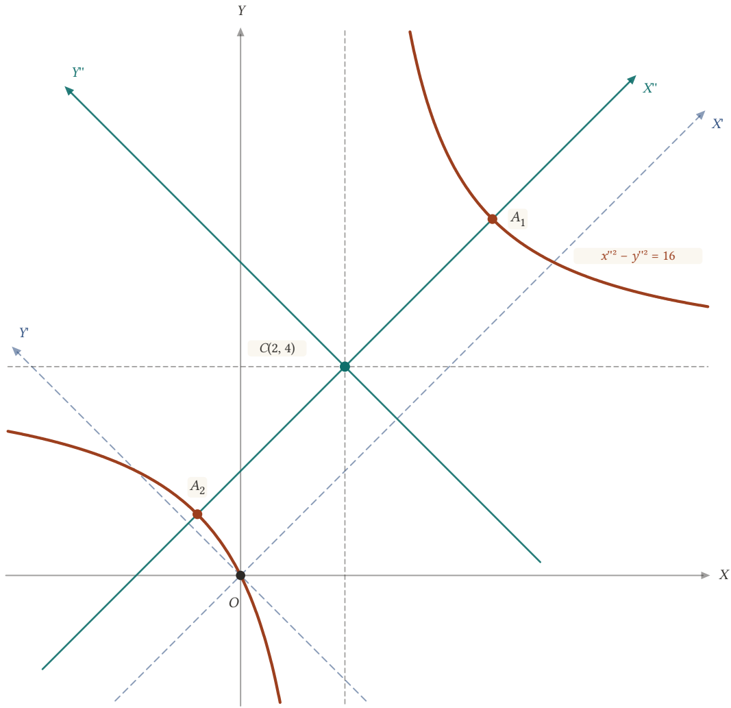
Şekil 21.13: Eksenler merkez C(2, 4) 'e ötelenince ikizkenar hiperbolün standart denklemi x''^2 - y''^2 = 16 elde edilir.
