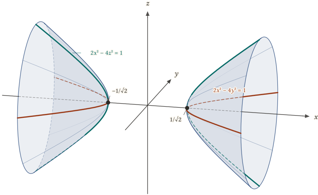
Şekil 23.17: İki kanatlı dönel hiperboloid 2x^2 - 4y^2 - 4z^2 = 1 , |x| \leq 2 : xy -düzlemindeki iz 2x^2 - 4y^2 = 1 (kırmızı), xz -düzlemindeki iz 2x^2 - 4z^2 = 1 (yeşil); x = \pm 2 'deki uç çemberlerin yarıçapı \sqrt{7/2} 'dir. Köşeler (\pm 1/\sqrt{2}, 0, 0) noktalarıdır.
