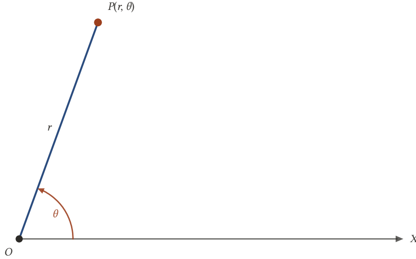
Şekil 5.5: Kutupsal koordinatlar: r = |OP| kutuptan uzaklık, \theta de kutupsal eksenden OP ye saat yönünün tersine ölçülen açıdır.
