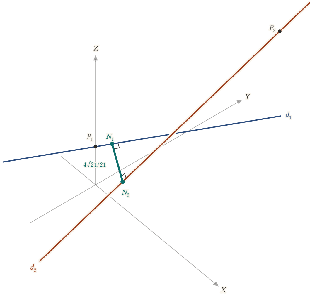
Şekil 11.17: Aykırı d_1 ve d_2 doğrularının ortak dikmesinin ayakları N_1(1/7, 2/7, 1) ve N_2(19/21, -2/21, 17/21) ; aralarındaki uzaklık 4\sqrt{21}/21 \approx 0,87 'dir.
