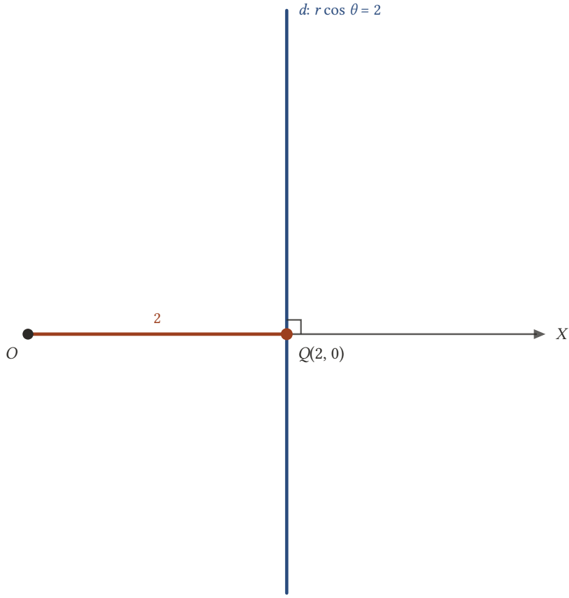
Şekil 5.32: r \cos \theta = 2 doğrusu: kutuptan inilen dikmenin ayağı Q(2, 0) 'dır ve doğru kutupsal eksene diktir, yani x = 2 .
