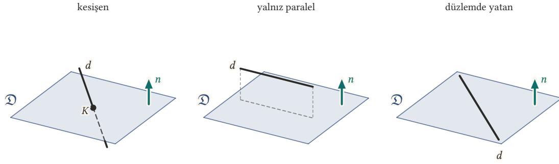
Şekil 14.1: Bir doğru ile bir düzlem: solda doğru düzlemi tek bir K noktasında deler (düzlemin arkasında kalan parçası kesikli), ortada düzleme paraleldir ve onu hiç kesmez (kesikli çizgi, doğrunun düzlemdeki dik izdüşümüdür), sağda tamamen düzlemin içinde yatar.
