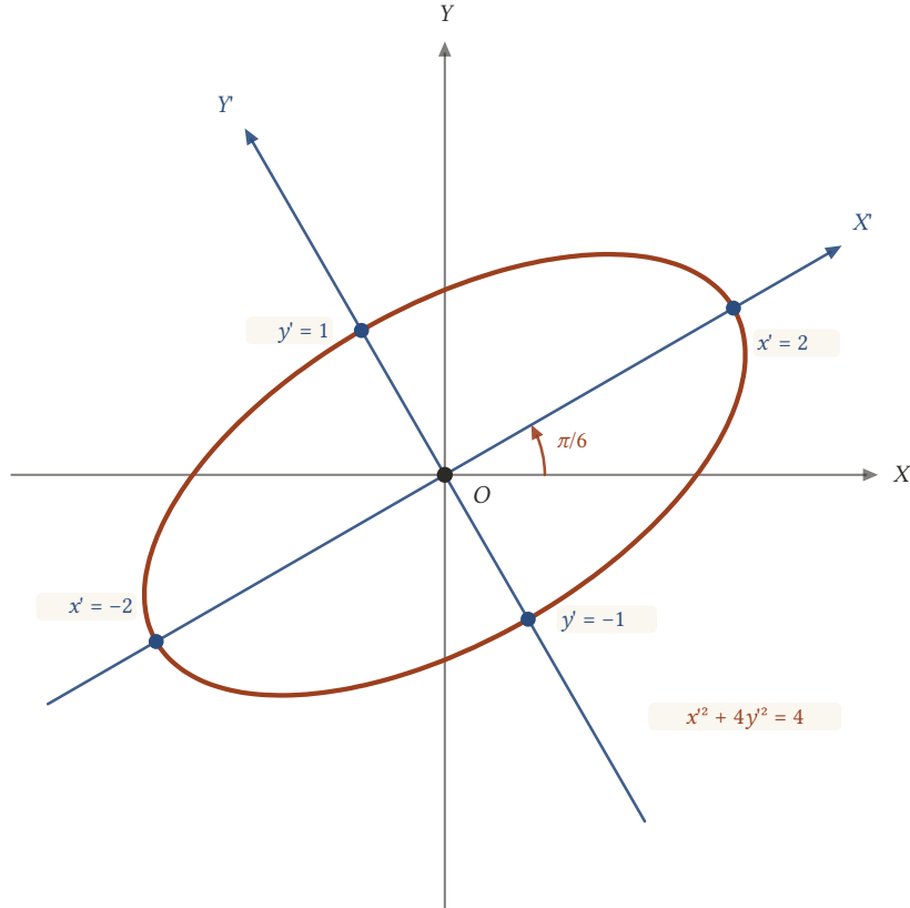
Şekil 17.23: 7x^2 - 6\sqrt{3}xy + 13y^2 = 16 eğrisi, eksenler \pi/6 döndürülünce x'^2 + 4y'^2 = 4 denklemiyle yazılır.
