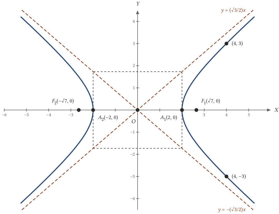
Şekil 19.18: 3x^2 - 4y^2 = 12 hiperbolü, temel dikdörtgeni ve asimptotları.
