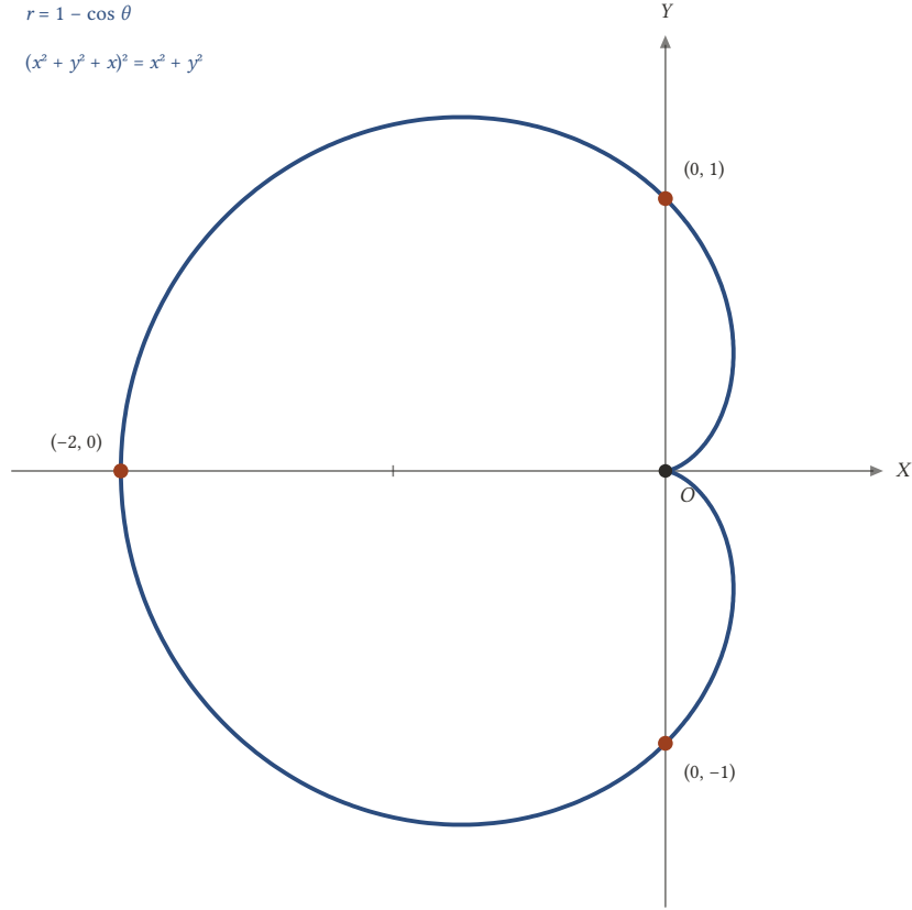
Şekil 5.28: r = 1 - \cos \theta kardiodi. Eğri kutupta sivri bir uç yapar ve sola doğru açılır; dik koordinatlardaki denklemi (x^2 + y^2 + x)^2 = x^2 + y^2 'dir.
