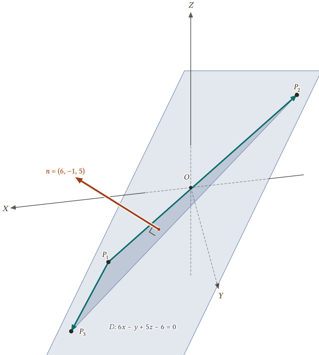
Şekil 12.22: P_1(2, 1, -1) , P_2(-2, 2, 4) , P_3(3, 2, -2) noktalarından geçen 6x - y + 5z - 6 = 0 düzlemi ve normali (0,3 katı, üçgenin ağırlık merkezinden).
