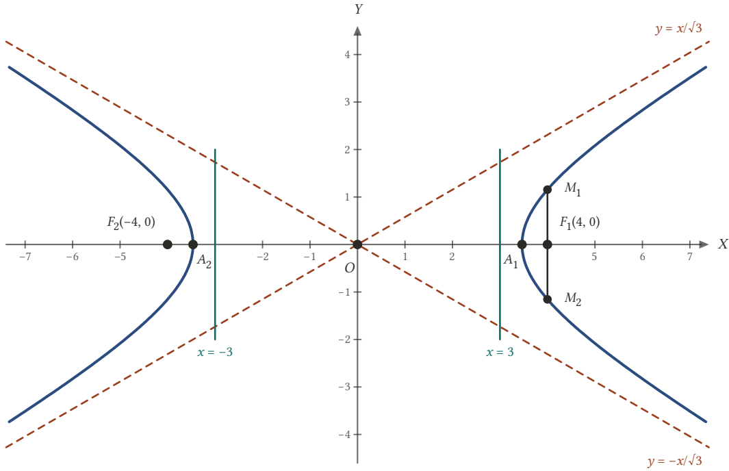
Şekil 19.20: x^2/12 - y^2/4 = 1 : odaklar (\pm 4, 0) , asimptotlar y = \pm x/\sqrt{3} , doğrultmanlar x = \pm 3 .
