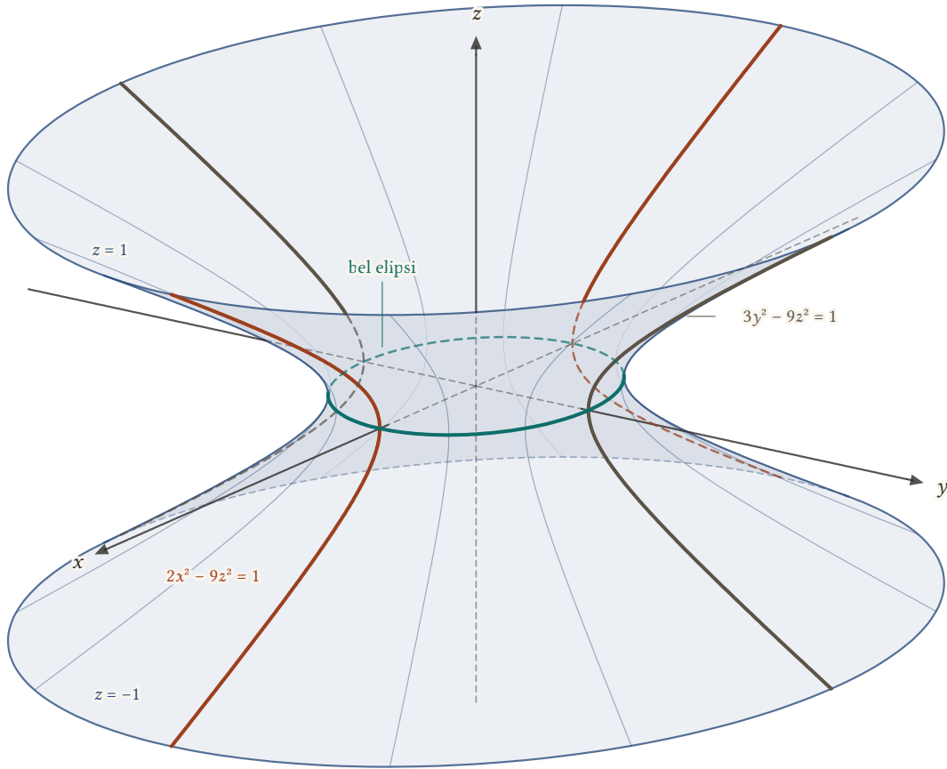
Şekil 23.21: Tek kanatlı hiperboloid 2x^2 + 3y^2 - 9z^2 = 1 , |z| \leq 1 . z = 0 'daki bel elipsi 2x^2 + 3y^2 = 1 (yeşil), z = \pm 1 'deki uç elipsler 2x^2 + 3y^2 = 10 'dur; xz - ve yz -düzlemlerindeki izler 2x^2 - 9z^2 = 1 (kırmızı) ve 3y^2 - 9z^2 = 1 hiperbolleridir.
