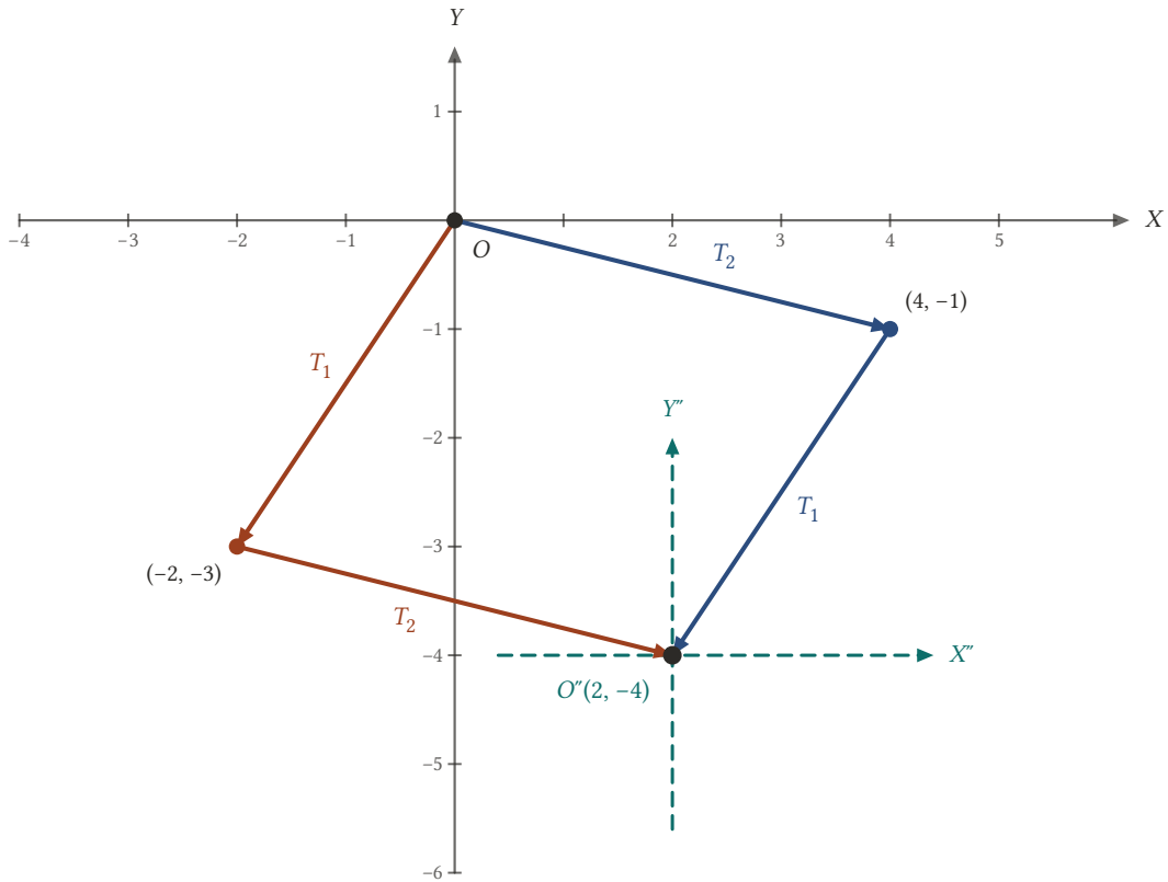
Şekil 16.23: Başlangıç noktası önce T_2 sonra T_1 ile de, önce T_1 sonra T_2 ile de aynı O''(2, -4) noktasına taşınır.
