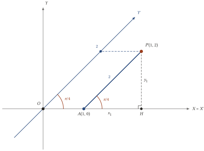
Şekil 17.25: Eksen açısı \pi/4 olan eğik sistemde P(1, 2) noktası; AHP dik üçgeninden x_1 = y_1 = \sqrt{2} ve P(1 + \sqrt{2}, \sqrt{2}) bulunur.
