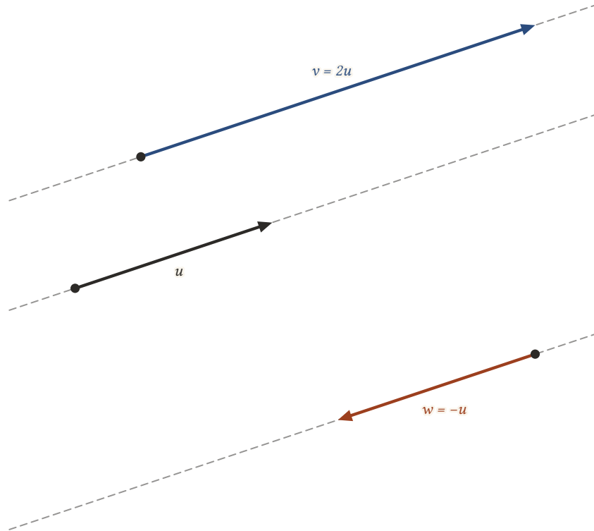
Şekil 7.14: u, v = 2u ve w = -u paralel doğrular üzerindedir; v ile u aynı yönlü, w ile u zıt yönlüdür.
