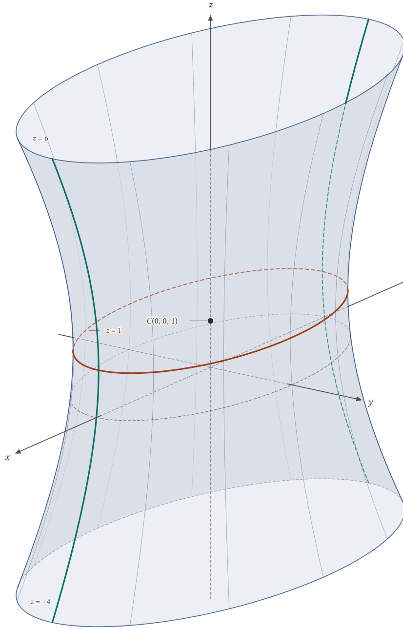
Şekil 23.29: Merkezi C(0, 0, 1) olan tek kanatlı hiperboloid x^2/16 + y^2/4 - (z - 1)^2/25 = 1 , -4 \leq z \leq 6 . Bel elipsi (kırmızı) z = 1 düzleminde, yani xy -düzleminin bir birim üstündedir (soluk kesikli elips yüzeyin z = 0 izidir); yeşil eğriler y = 0 düzlemindeki hiperbolün kollarıdır.
