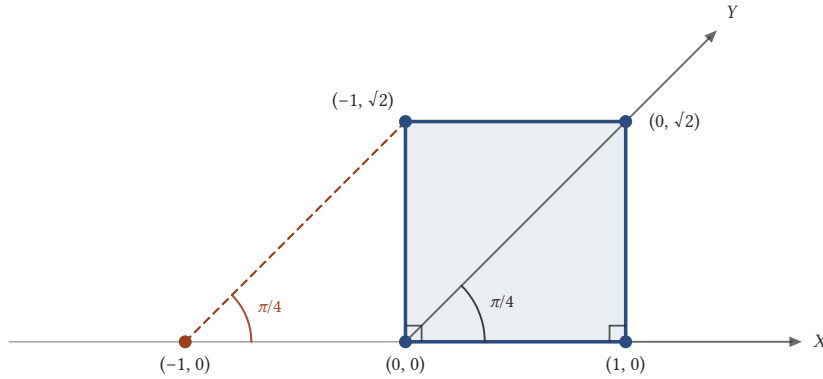
Şekil 5.4: \alpha = \pi/4 olan eğik sistemde kenarı 1 olan kare. Köşelerin yanındaki sayılar paralel koordinatlarıdır; C 'den Y -eksenine çizilen paralel X -eksenini (-1, 0) 'da keser.
