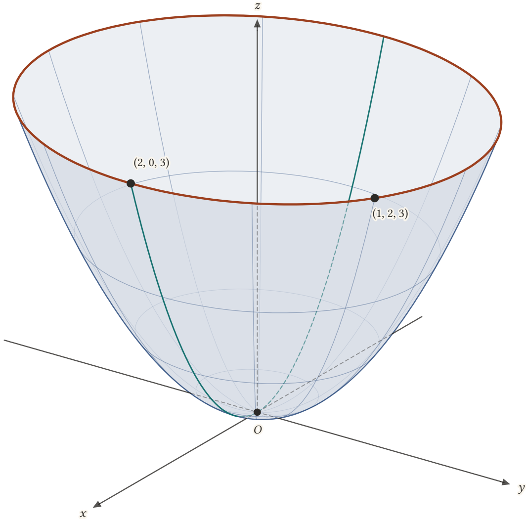
Şekil 23.31: Eliptik paraboloid 12x^2 + 9y^2 = 16z , 0 \leq z \leq 3 . Verilen (2, 0, 3) ve (1, 2, 3) noktaları z = 3 izi olan x^2/4 + y^2/(16/3) = 1 elipsinin (kırmızı) üzerindedir; yeşil eğri xz -düzlemindeki z = (3/4)x^2 parabolüdür.
