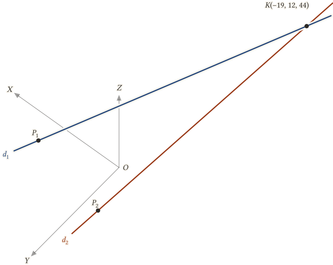
Şekil 11.16: d_1 ile d_2 K(-19, 12, 44) noktasında kesişir. Doğrultman vektörleri neredeyse paralel olduğundan doğrular kesişim noktasına çok yavaş yaklaşır; eksenler başlangıç noktası çevresinde, ölçek için çizilmiştir.
