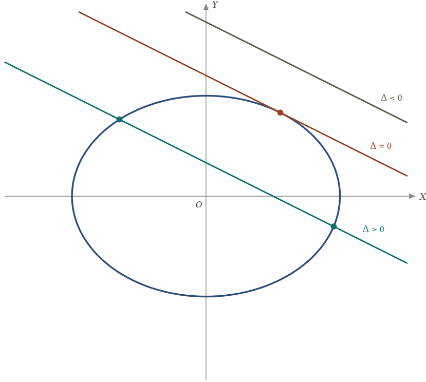
Şekil 18.15: x^2/16 + y^2/9 = 1 elipsi ve eğimi -1/2 olan üç doğru: n = 1 iken iki ortak nokta, n = \sqrt{13} iken teğet, n = 5,2 iken ortak nokta yok.
