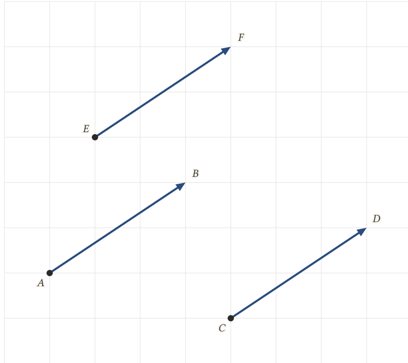
Şekil 7.4: Aynı vektörün üç temsalcisi: AB, CD ve EF okları aynı yönde ve aynı uzunluktadır; her biri sağa 3, yukarı 2 birim gider.
