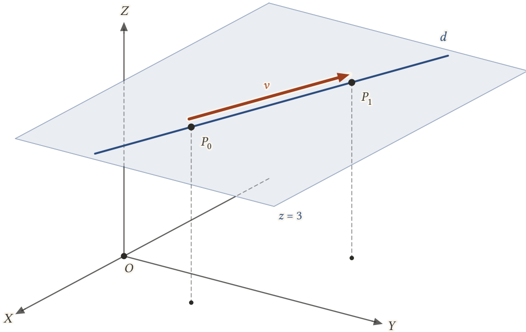
Şekil 10.7: Doğrultmanı v = (-3, 1, 0) olan doğru, kotu 3 olan noktalardan oluşan z = 3 düzleminde yatar; P_0 ve P_1 'den XY düzlemine inen kesikli çizgilerin ikisi de 3 birimdir.
