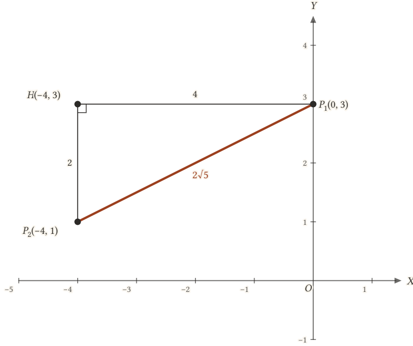
Şekil 1.23: Dik kenarları 4 ve 2 olan dik üçgenin hipotenüsü \sqrt{20} = 2\sqrt{5} 'tir.
