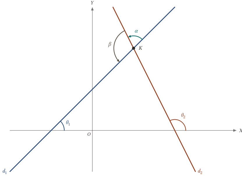
Şekil 2.24: d_1 ve d_2 doğrularının eğim açıları \theta_1, \theta_2 ; kesişim noktasındaki yönlendirilmiş açılar \alpha ve \beta . Üçgenin dış açısı olarak \theta_2 = \theta_1 + \alpha 'dır.
