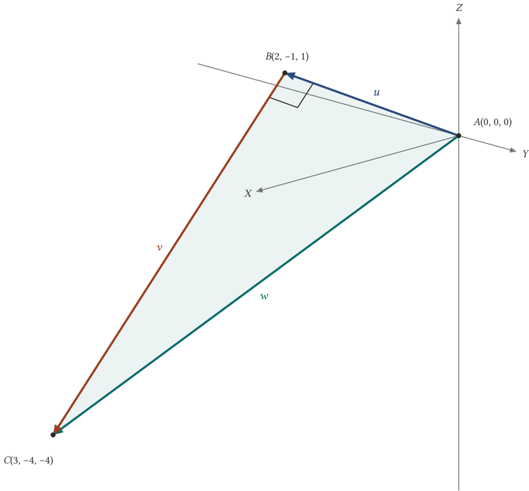
Şekil 8.14: u + v = w olduğundan üç vektör ABC üçgeninin kenarlarıdır; \langle u, v \rangle = 0 olduğundan B köşesindeki açı diktir.
