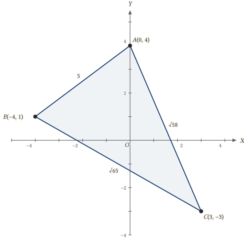
Şekil 1.11: Kenarları 5, \sqrt{65} ve \sqrt{58} olan üçgenin çevresi 5 + \sqrt{65} + \sqrt{58} 'dir.
