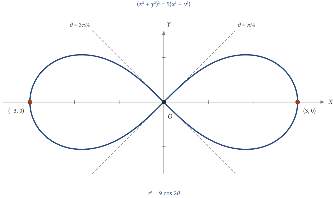
Şekil 5.29: r^2 = 9 \cos 2\theta Bernoulli lemniskatı. Eğri yalnız kutupsal eksenle en çok \pi/4 açı yapan yönlerde ve bunların ters yönlerinde bulunur.
