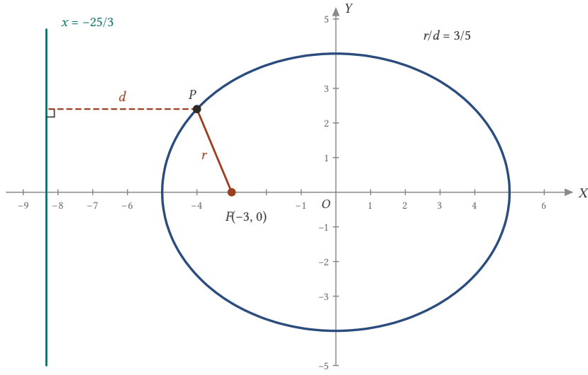
Şekil 18.23: F(-3, 0) noktasına ve x = -25/3 doğrusuna uzaklıklarının oranı 3/5 olan noktalar x^2/25 + y^2/16 = 1 elipsini oluşturur.
