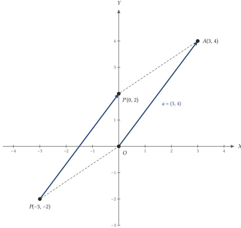
Şekil 16.2: a = (3, 4) ötelemesi P(-3, -2) noktasını P'(0, 2) noktasına taşır.
