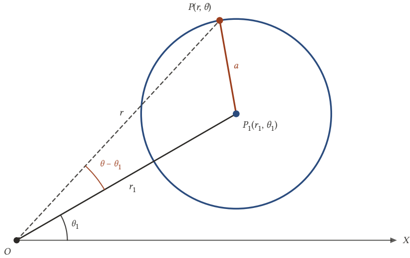
Şekil 5.24: P_1(r_1, \theta_1) merkezli, a yarıçaplı çember: POP_1 üçgeninde kosinüs teoremi çemberin kutupsal denklemini verir.
