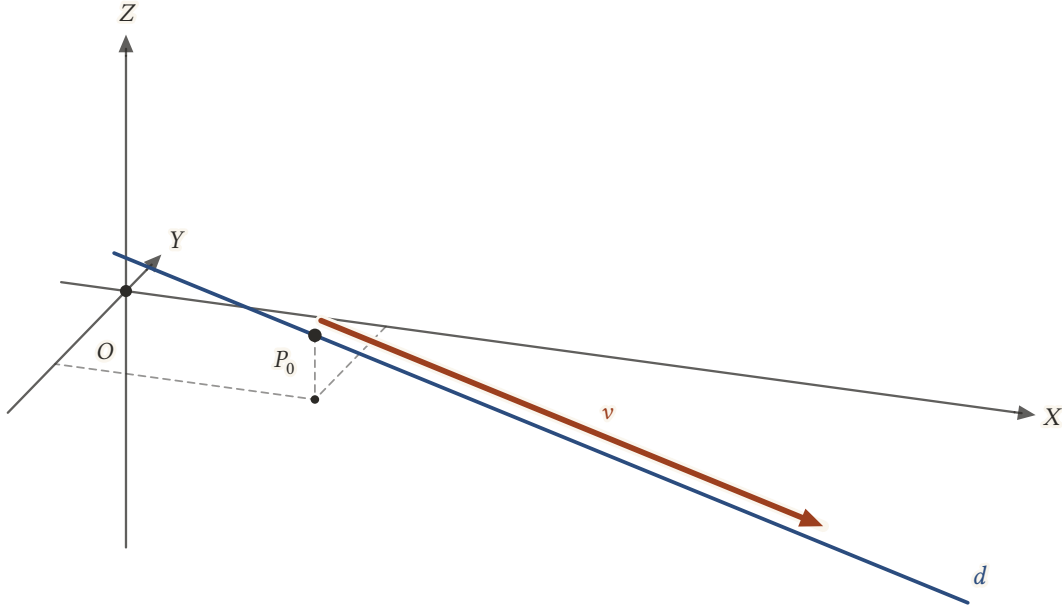
Şekil 10.2: P_0 = (4, -3, 1) noktasından geçen ve v = (7, 2, -3) vektörüne paralel olan d doğrusu. Kesikli çizgiler P_0 'ın XY düzlemindeki izdüşümünü gösterir.
