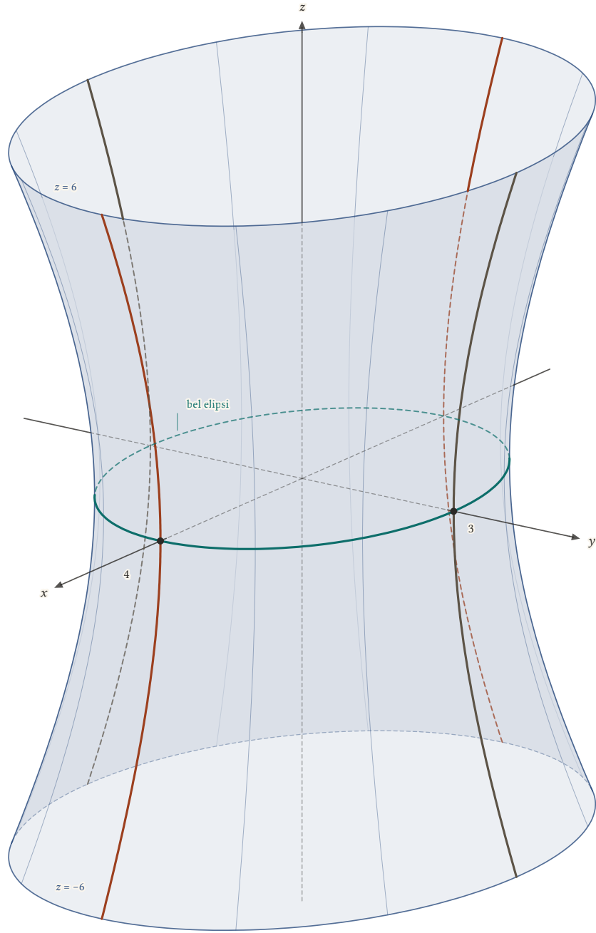
Şekil 23.27: Tek kanatlı hiperboloid x^2/16 + y^2/9 - z^2/36 = 1, |z| \leq 6 . Bel elipsi (yeşil) eksenleri 4 ve 3'te keser; z = \pm 6 'daki uç elipslerin yarı eksenleri 4\sqrt{2} ve 3\sqrt{2} 'dir. y = 0 ve x = 0 düzlemlerindeki izler hiperboldür (kırmızı ve kahverengi).
