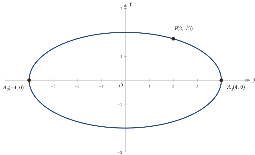
Şekil 18.8: Uzak köşeleri (\pm 4, 0) olan ve P(2, \sqrt{3}) noktasından geçen elips: x^2/16 + y^2/4 = 1 .
