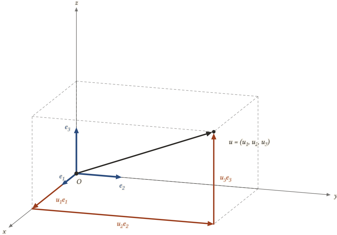
Şekil 7.16: u = (u_1, u_2, u_3) , eksenler boyunca uç uca eklenen u_1 e_1, u_2 e_2 ve u_3 e_3 oklarının toplamıdır.
