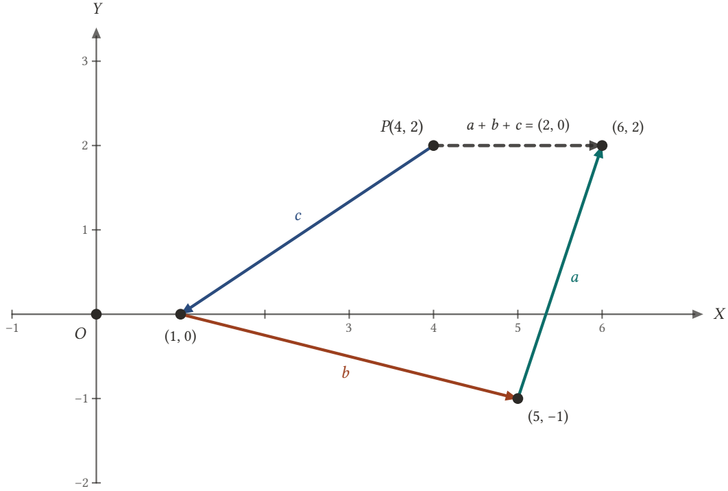
Şekil 16.15: P(4, 2) noktasına sırasıyla c , b ve a ötelemeleri uygulanır; sonuç, a + b + c = (2, 0) kadar tek ötelemenin verdiği (6, 2) noktasıdır.
