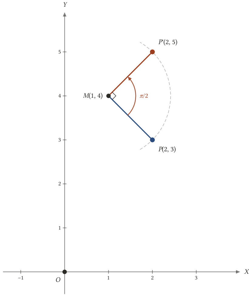
Şekil 17.6: P(2, 3) , M(1, 4) etrafında \pi/2 döndürülünce P(2, 5) olur; MP ile MP' eşit uzunlukta ve diktir.
