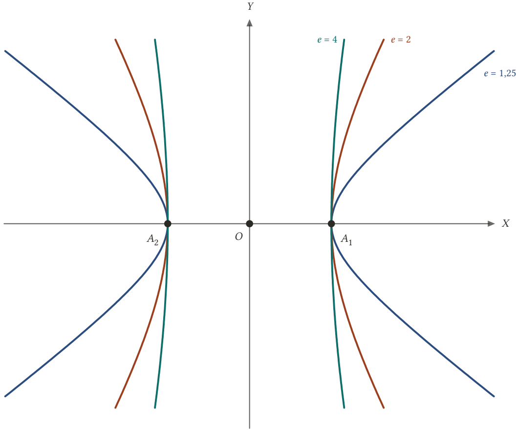
Şekil 19.14: Köşeler aynıken e büyüdükçe asimptotlar dikleşir ve kollar açılır; e 1'e yaklaştıkça kollar asal eksene doğru kapanır.
