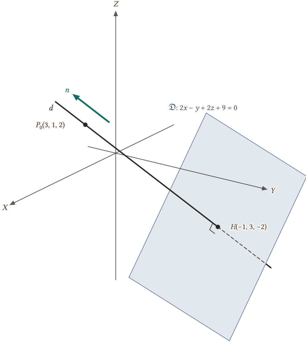
Şekil 14.6: d 'nin doğrultman vektörü düzlemin normali n = (2, -1, 2) 'dir; doğru düzleme diktir ve onu H(-1, 3, -2) 'de keser. H , P_0(3, 1, 2) 'dan düzleme inen dikmenin ayağıdır.
