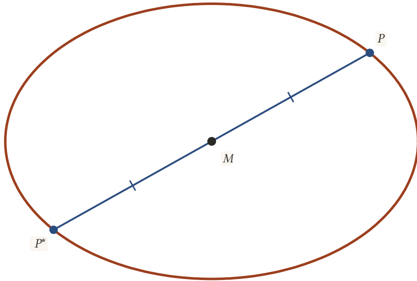
Şekil 21.6: M , koniğin merkezidir: koniğin her P noktasının M 'ye göre simetriği P^* de konik üzerindedir.
