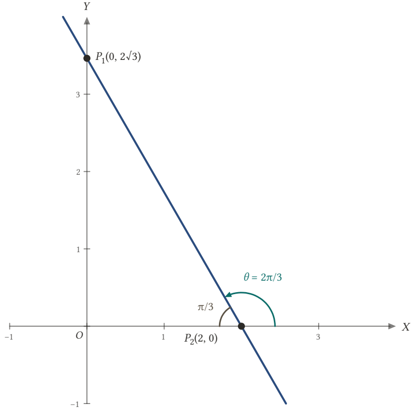
Şekil 2.14: P_1(0, 2\sqrt{3}) ve P_2(2, 0) 'dan geçen doğrunun eğimi -\sqrt{3} 'tür; doğru X -ekseninin negatif yönüyle \pi/3 'lük açı yapar, eğim açısı \theta = 2\pi/3 'tür.
