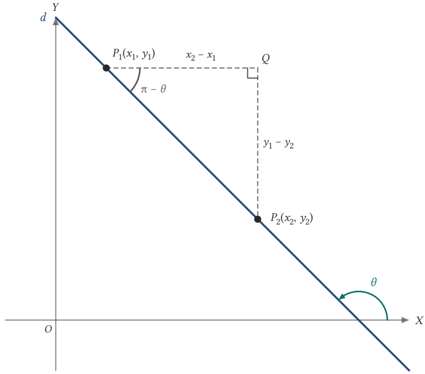
Şekil 2.12: Geniş eğim açısında P_1QP_2 üçgeninin P_1 köşesindeki iç açısı \pi - \theta 'dir; \tan(\pi - \theta) = -\tan \theta olduğundan formül yine aynı çıkar.
