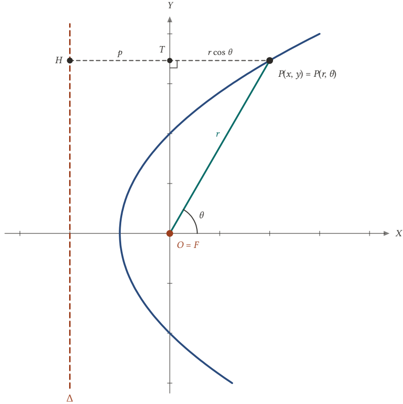
Şekil 20.12: Kutup odakta: |PF| = r ve |PH| = p + r \cos \theta . |PF| = e|PH| koşulu r = ep/(1 - e \cos \theta) verir (çizimde p = 2 , e = 1 ).
