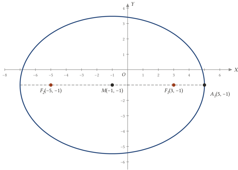
Şekil 18.32: Merkezi M(-1, -1) , uzak köşesi A_1(5, -1) , dış merkezliği 2/3 olan elips: (x + 1)^2/36 + (y + 1)^2/20 = 1 .
