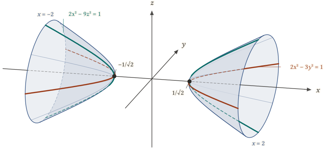
Şekil 23.22: İki kanatlı hiperboloid 2x^2 - 3y^2 - 9z^2 = 1 , |x| \leq 2 : xy -düzlemindeki iz 2x^2 - 3y^2 = 1 (kırmızı), xz -düzlemindeki iz 2x^2 - 9z^2 = 1 (yeşil); x = \pm 2 düzlemlerindeki uç elipsler 3y^2 + 9z^2 = 7 'dir. Yüzey yz -düzlemini kesmez.
