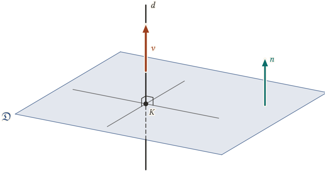
Şekil 14.3: Düzleme dik doğru: d 'nin doğrultman vektörü v , düzlemin normali n ile aynı doğrultudadır. Bu yüzden d , düzlemin K 'dan geçen her doğrusuna diktir; şekilde bunlardan ikisi gösterilmiştir.
