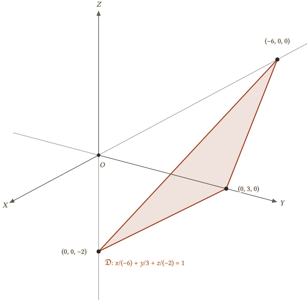
Şekil 13.11: x - 2y + 3z + 6 = 0 düzlemi eksenleri (-6, 0, 0) , (0, 3, 0) ve (0, 0, -2) noktalarında keser; üçgen X ve Z eksenlerinin negatif yanlarına uzanır. Eksenlerin negatif kısımları soluktur.
