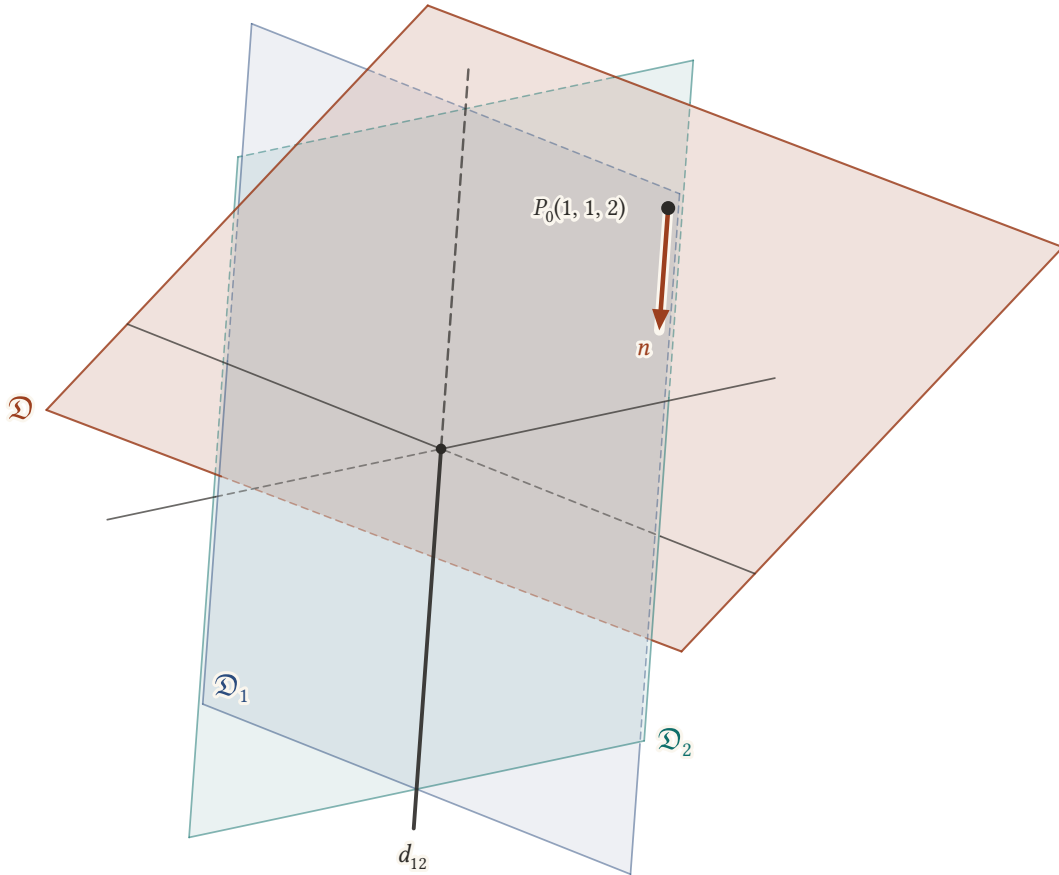
Şekil 13.21: P_0(1, 1, 2) 'den geçen ve iki düzleme birden dik olan düzlem: normal n = (1, 3, -1) , d_{12} arakesit doğrusuna paraleldir; bu yüzden düzlem d_{12} 'ye diktir ve iki düzlemi ince çizgiler boyunca keser.
