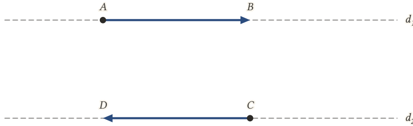
Şekil 7.3: AB ile CD aynı doğrultulu ama ters yönlüdür: biri sağ, öteki solu gösterir.
