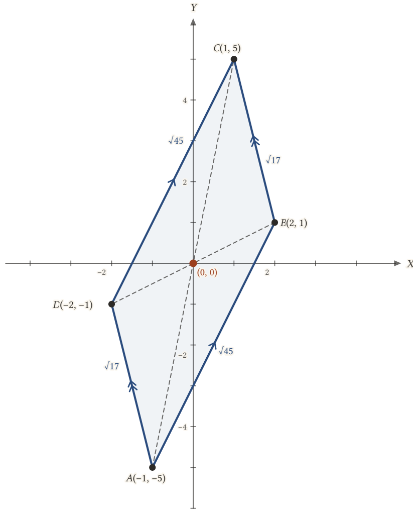
Şekil 1.34: Karşılıklı kenarlar paraleldir (eğimler 2 ve -4) ve eşittir; köşegenler birbirini (0, 0)'da ortalar.
