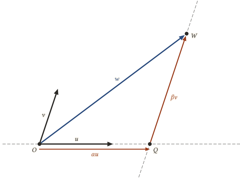
Şekil 7.18: W 'den v 'ye paralel çizilen doğru, u doğrusunu Q 'da keser; böylece w = \alpha u + \beta v olur.
