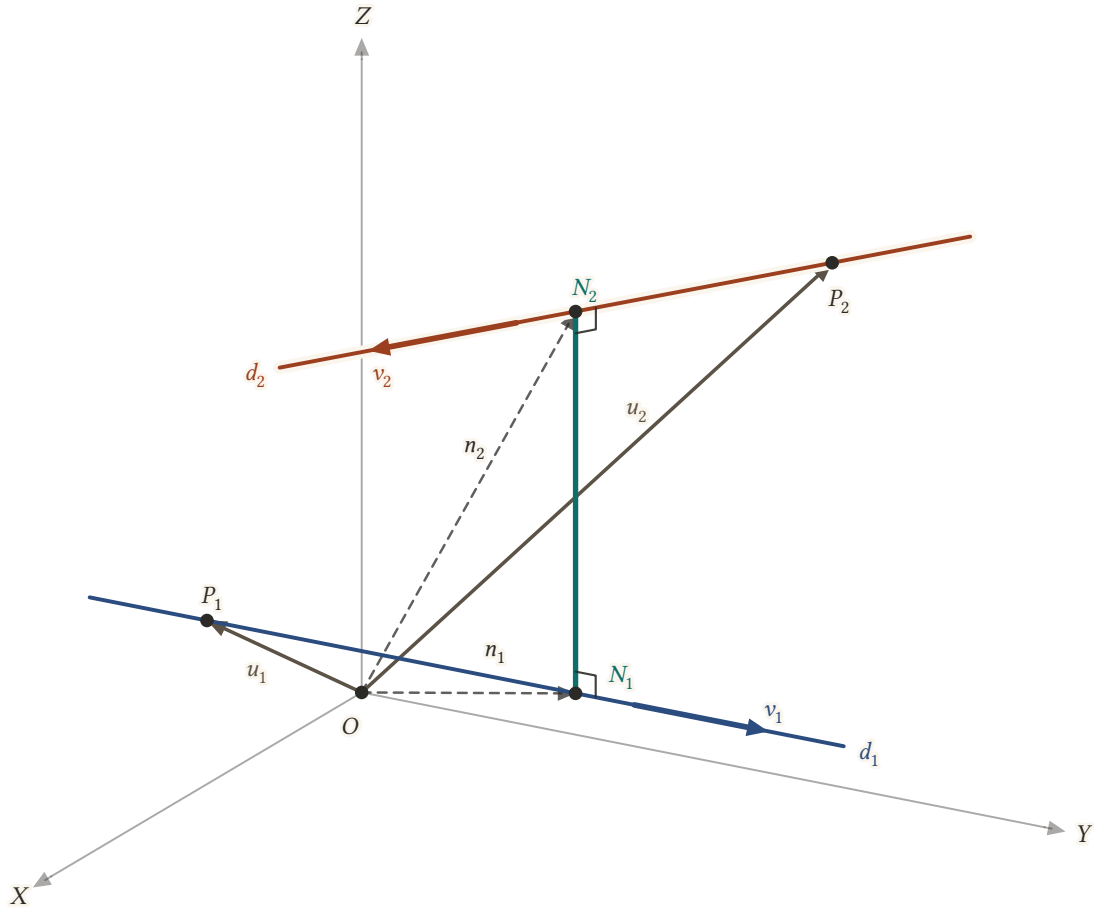
Şekil 11.11: N_1N_2 ortak dikmesi d_1 'e ve d_2 'ye diktir. u_1, u_2 doğrulardaki P_1, P_2 noktalarının, n_1, n_2 ise ayakların konum vektörleridir.
