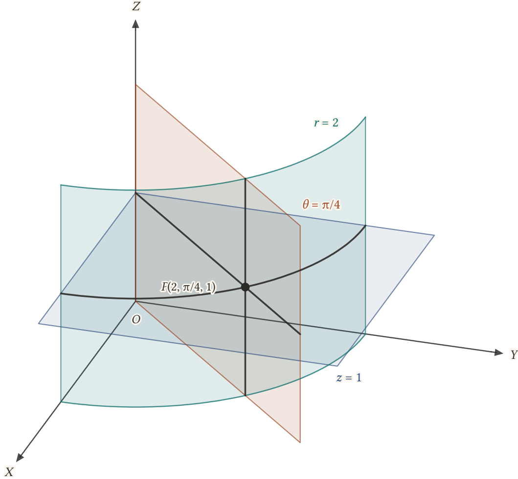
Şekil 22.4: Silindirik koordinat yüzeyleri: r = 2 silindiri, \theta = \pi/4 yarım düzlemi ve z = 1 düzlemi (birinci bölgedeki parçaları). Koyu çizgiler ikişer ikişer kesişimlerdir; üçü birden yalnız silindirik koordinatları (2, \pi/4, 1) olan P(\sqrt{2}, \sqrt{2}, 1) noktasında buluşur.
