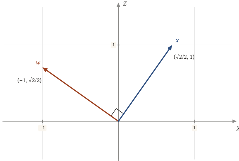
Şekil 8.3: w ile x 'in ikinci bileşeni 0 olduğundan ikisi de XZ -düzleminde yatar. Bu düzlemde çizildiklerinde aralarındaki açının dik olduğu görülür.
