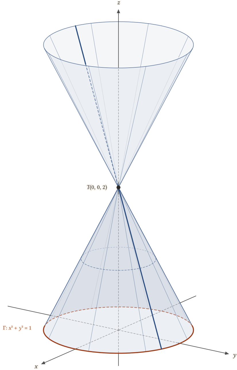
Şekil 23.9: Dik dairesel koni 4x^2 + 4y^2 = (2 - z)^2 , 0 \leq z \leq 4 . Üreteçler dayanak çemberi \Gamma 'dan (kırmızı) T(0, 0, 2) tepe noktasından geçerek üst kanada uzanır; kesikli ara çember z = 1 kesitidir (yarıçap 1/2 ).
