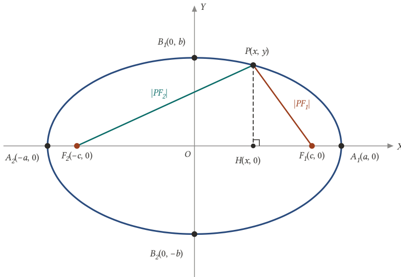
Şekil 18.7: P 'den X -eksenine inen dikmenin ayağı H ; PHF_1 ve PHF_2 dik üçgenlerinde Pisagor bağıntısı |PF_1| ve |PF_2| 'yi x cinsinden verir.
