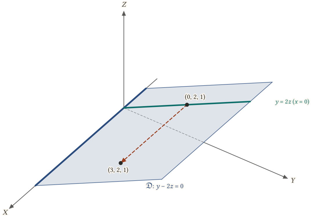
Şekil 13.13: y - 2z = 0 düzlemi X -eksenini içerir (kalın mavi). YZ -düzlemindeki izi y = 2z doğrusudur; düzlem bu izin X -ekseni doğrultusunda kaydırılmasıyla oluşur: (0, 2, 1) düzlemdeyse (3, 2, 1) de düzlemde.
