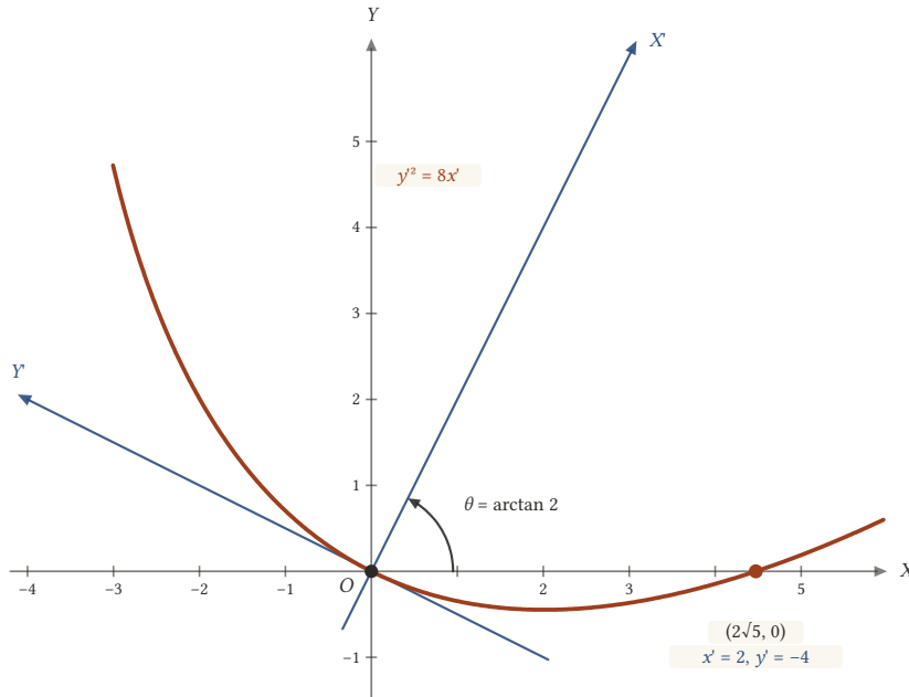
Şekil 21.11: Eksenler \arctan 2 kadar döndürülünce 4x^2 - 4xy + y^2 - 8\sqrt{5}x - 16\sqrt{5}y = 0 parabolü y'^2 = 8x' olur; parabolün eksen y = 2x doğrusudur.
