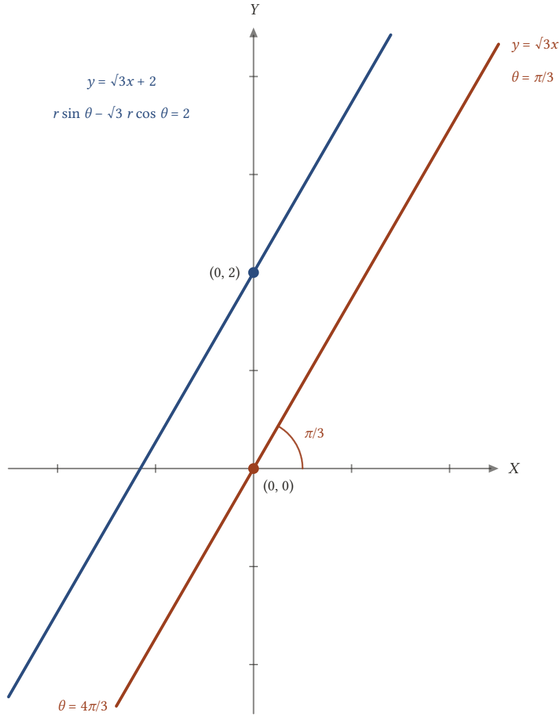
Şekil 5.9: Paralel iki doğru: y = \sqrt{3}x + 2 kutuptan geçmez, kutupsal denklemi r \sin \theta - \sqrt{3} r \cos \theta = 2 'dir. Kutuptan geçen y = \sqrt{3}x doğrusu ise \theta = \pi/3 ve \theta = 4\pi/3 yarı doğrularının birleşimidir.
