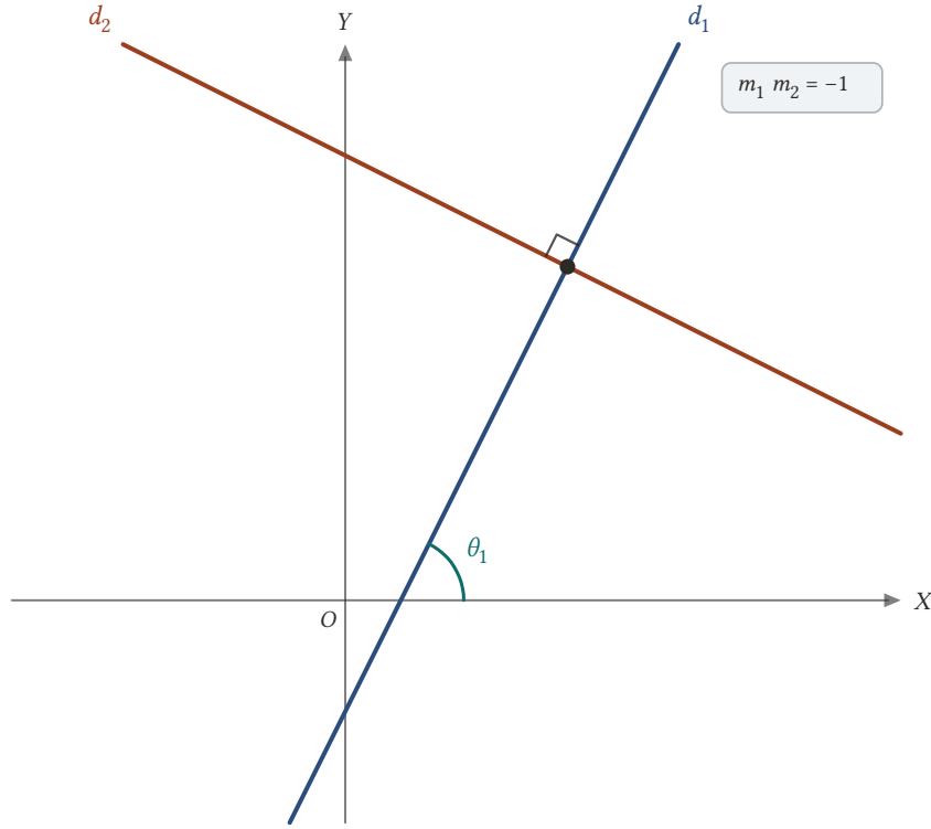
Şekil 2.18: Dik d_1 (eğim 2) ve d_2 (eğim -1/2 ) doğruları (2, 3) noktasında dik açıyla kesişir; eğimlerinin çarpımı -1 'dir.
