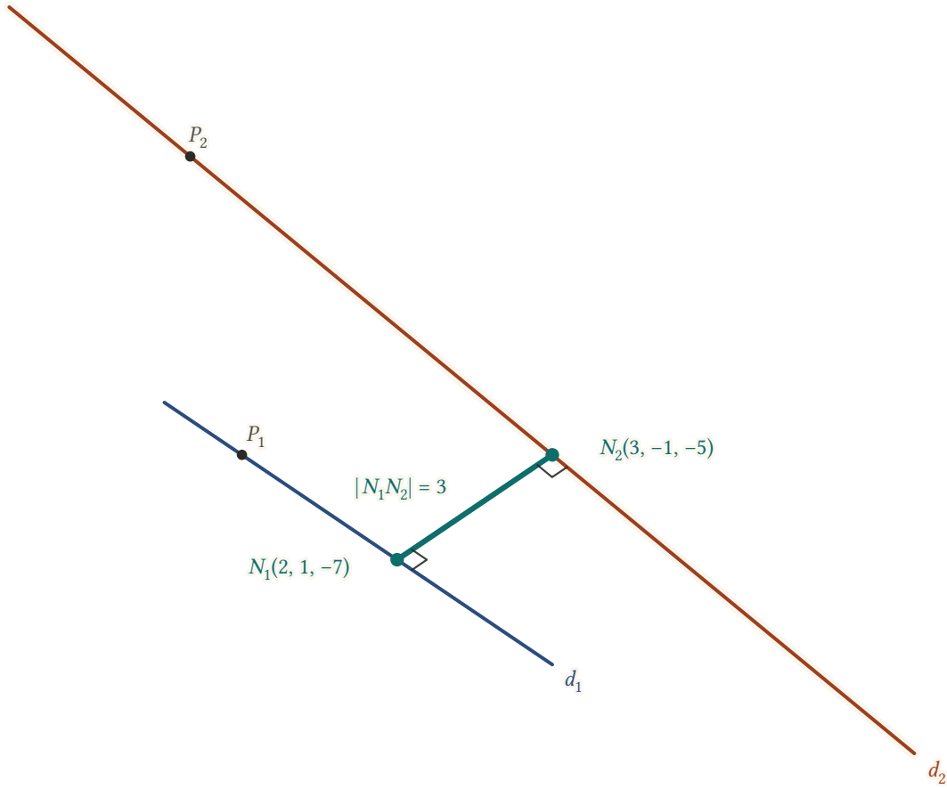
Şekil 11.14: Aykırı d_1 ve d_2 doğrularının ortak dikmesi N_1(2, 1, -7) ile N_2(3, -1, -5) arasındadır; iki doğruya da diktir ve uzunluğu 3'tür.
