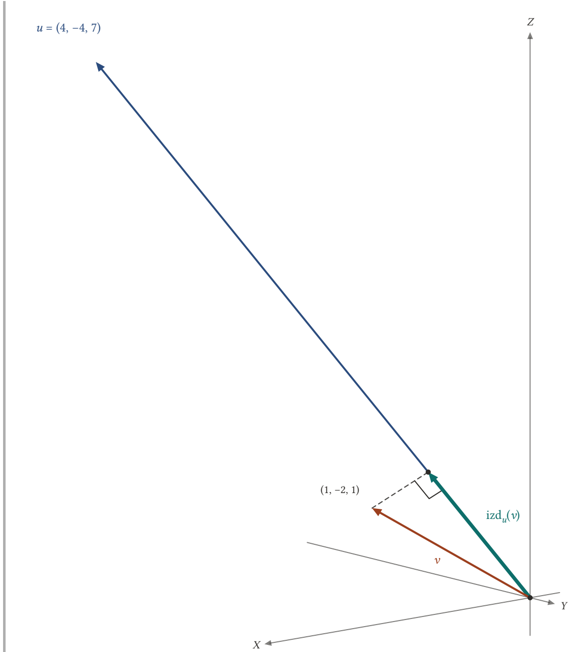
Şekil 8.20: v = (1, -2, 1) 'nin u = (4, -4, 7) üzerine izdüşümü \text{izd}_u(v) = (76/81, -76/81, 133/81) 'dir; bileşen 19/81 pozitif olduğundan izdüşüm u ile aynı yönlüdür.
