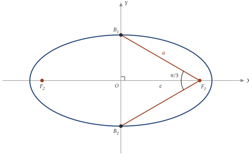
Şekil 18.30: F_1 odağı yedek eksen \pi/3 açısı altında görülür; OF_1B_1 dik üçgeninde \cos(\pi/6) = c/a = e = \sqrt{3}/2 .
