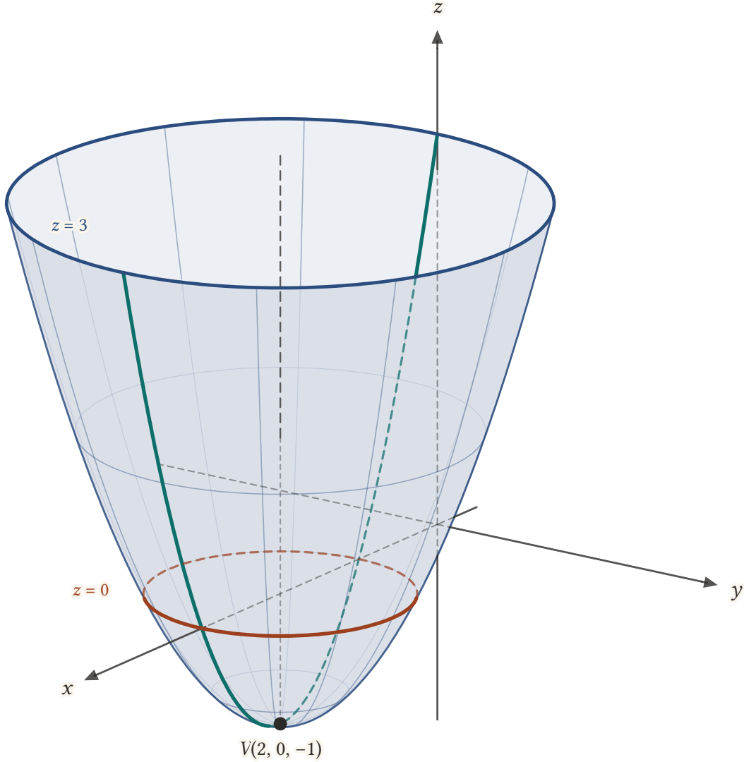
Şekil 23.25: Dönel paraboloid (x - 2)^2 + y^2 = z + 1 , -1 \leq z \leq 3 . Köşe V(2, 0, -1) , eksen köşeden geçen düşey kesikli doğrudur. z = 3 izi yarıçapı 2, z = 0 izi (kırmızı) yarıçapı 1 olan çemberdir; yeşil eğri y = 0 düzlemindeki z = (x - 2)^2 - 1 parabolüdür.
