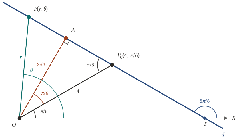
Şekil 5.26: P_0(4, \pi/6) 'dan geçen ve kutupsal eksenle 5\pi/6 açı yapan d doğrusu. Kutuptan inilen dikmenin ayağı A(2\sqrt{3}, \pi/3) ; denklem r \cos(\theta - \pi/3) = 2\sqrt{3} .
