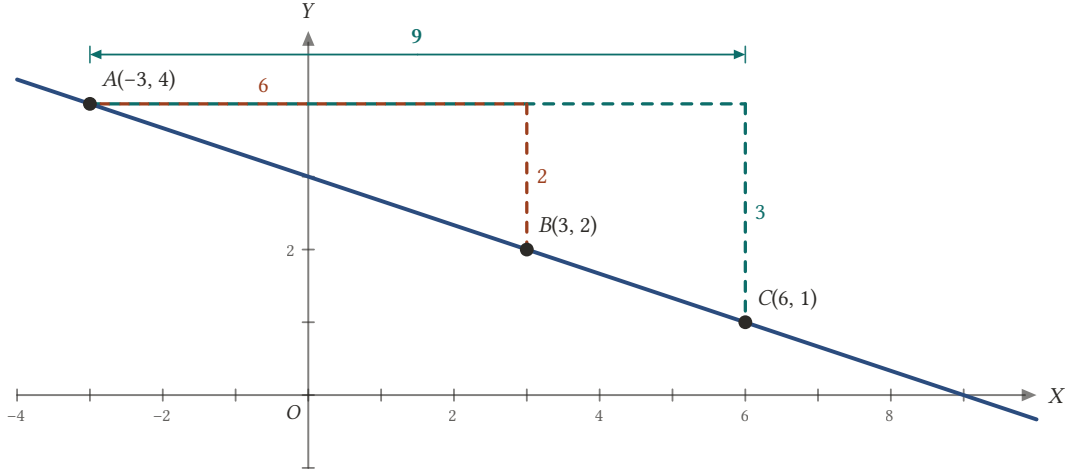
Şekil 2.16: A 'dan başlayan iki eğim üçgeni: turuncu üçgende düşey değişim / yatay değişim = 2/6 , yeşil üçgende 3/9 . Eğimler eşit ( -1/3 ) olduğundan A , B , C aynı doğru üzerindedir.
