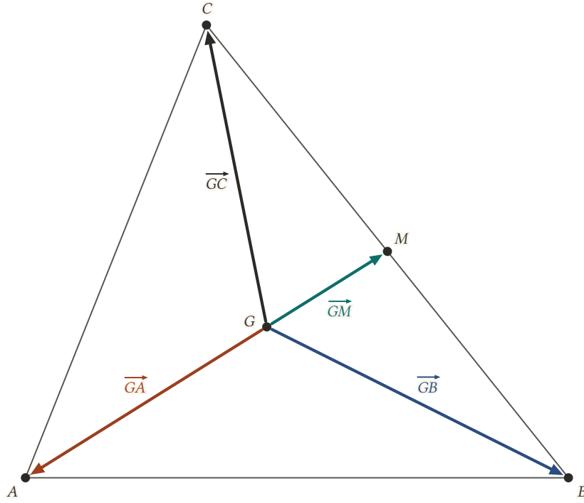
Şekil 7.21: G ağırlık merkezinden köşelere giden vektörler; M , BC 'nin orta noktasıdır ve GA = -2 GM , GB + GC = 2 GM olur.
