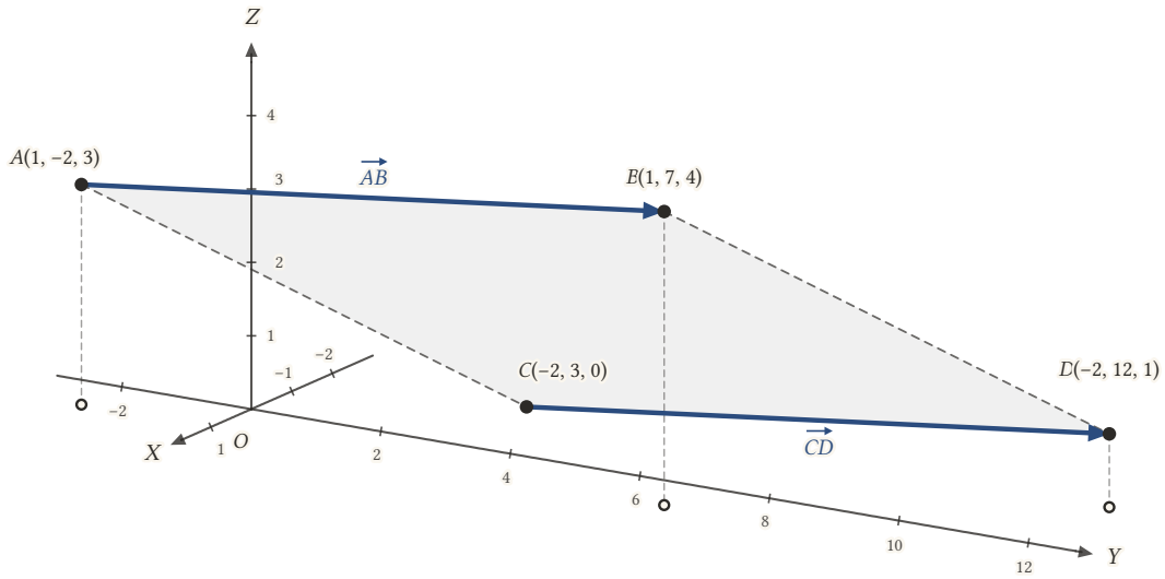
Şekil 6.19: A 'dan B 'ye ve C 'den D 'ye giden oklar aynı (0, 9, 1) koordinat değişimini taşır: paraleldir ve uzunlukları \sqrt{82} 'dir. ABDC bir paralelkenardır.
