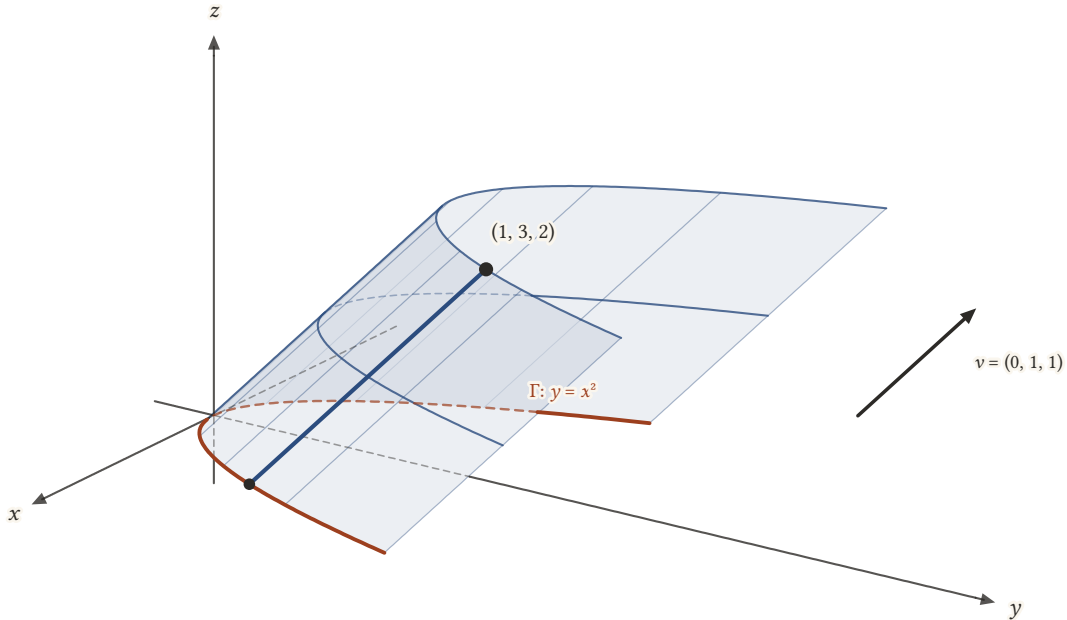
Şekil 23.35: Eğik parabolik silindir y - z = x^2 , |x| \leq 1,6 , 0 \leq z \leq 2 . Dayanak parabolü \Gamma (kırmızı) xy -düzleminindedir; z = 1 ve z = 2 kesitleri y doğrultusunda kaymış y = x^2 + 1 ve y = x^2 + 2 parabolleridir. Kalın üreteç (1, 1, 0) 'dan v = (0, 1, 1) doğrultusunda (1, 3, 2) 'ye gider.
