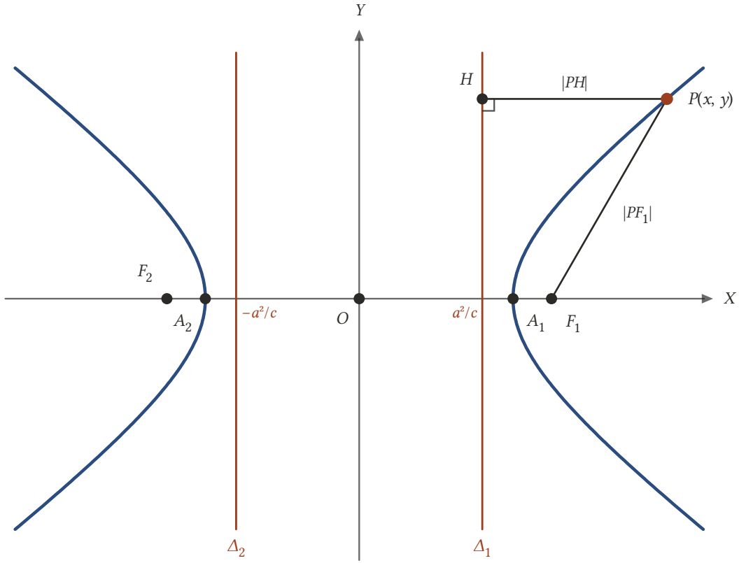
Şekil 19.15: Hiperbolün her noktasında |PF_1| = e \cdot |PH| .
