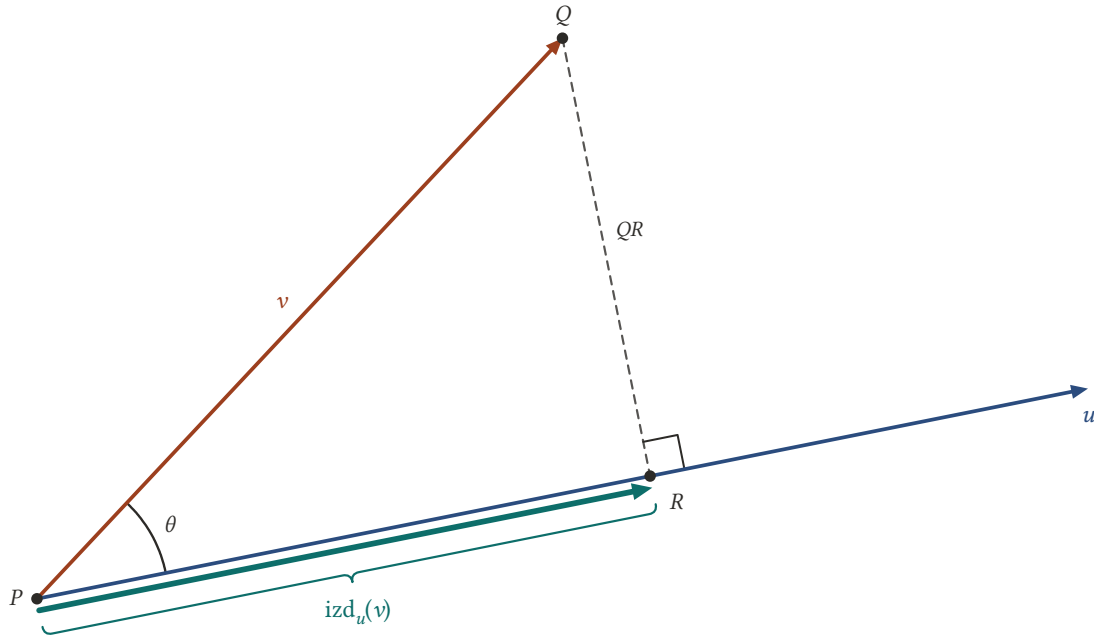
Şekil 8.7: P den çizilen v 'nin ucu Q 'dan u doğrultusuna dikme inilir; dikmenin ayağı R 'dir. P den R 'ye giden vektör v 'nin u üzerine dik izdüşümü \text{izd}_u(v) 'dir.
