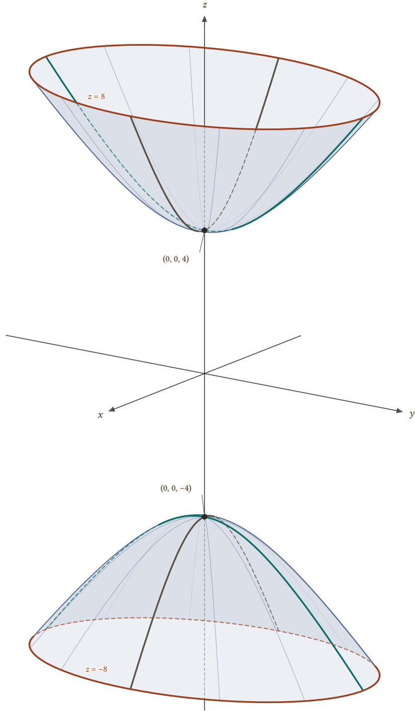
Şekil 23.30: Ekseni z -ekseni olan iki kanatlı hiperboloid -x^2/4 - y^2/9 + z^2/16 = 1 , 4 \leq |z| \leq 8 . Köşeler (0, 0, \pm 4) ; z = \pm 8 'deki uç elipsler x^2/4 + y^2/9 = 3 'tür (kırmızı). x = 0 ve y = 0 düzlemlerindeki izler hiperboldür (yeşil ve kahverengi); -4 < z < 4 şeridinde yüzey yoktur.
