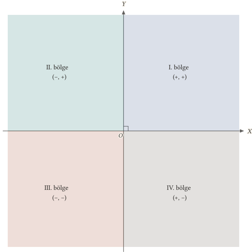
Şekil 1.3: Eksenler düzlemi dört bölgeye ayırır; parantez içindeki işaretler sırasıyla apsisin ve ordinatın işaretidir. Bölgeler saat yönünün tersine I'den IV'e sıralanır.
