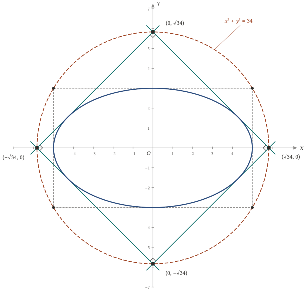
Şekil 18.18: x^2/25 + y^2/9 = 1 elipsinin eğimi \pm 1 olan dört teğeti bir kare oluşturur; karenin köşeleri ve 10 \times 6 dikdörtgenin köşeleri Monge çemberi x^2 + y^2 = 34 üzerindedir.
